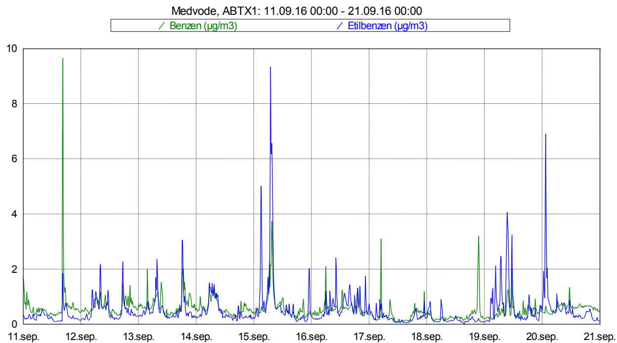
Slika 4: Imisijske koncentracije benzena in etilbenzena med 11. 9. 2016 in 20. 9. 2016.
