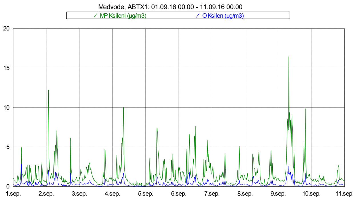
Slika 12: Imisijske koncentracije M&P in O ksilena med vključno 1. 9. 2016 in 10. 9. 2016.
