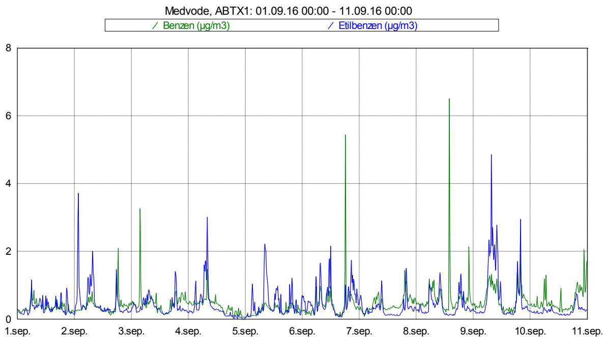
Slika 3: Imisijske koncentracije benzena in etilbenzena med vključno 1. 9. 2016 in 10. 9. 2016.
