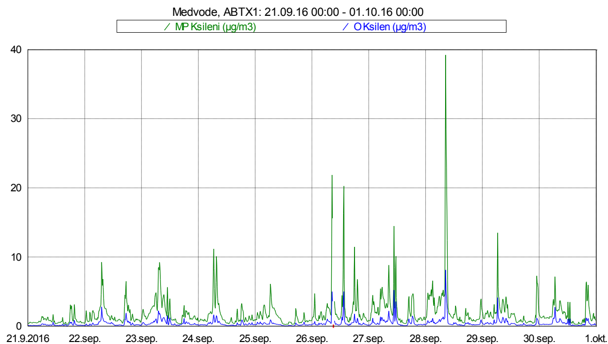
Slika 14: Imisijske koncentracije M&P in O ksilena med 21. 9. 2016 in 30. 9. 2016.
