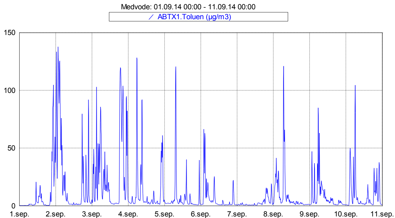
Slika 8: Imisijske koncentracije toluena med vključno 1. 9. 2014 in 10. 9. 2014.
