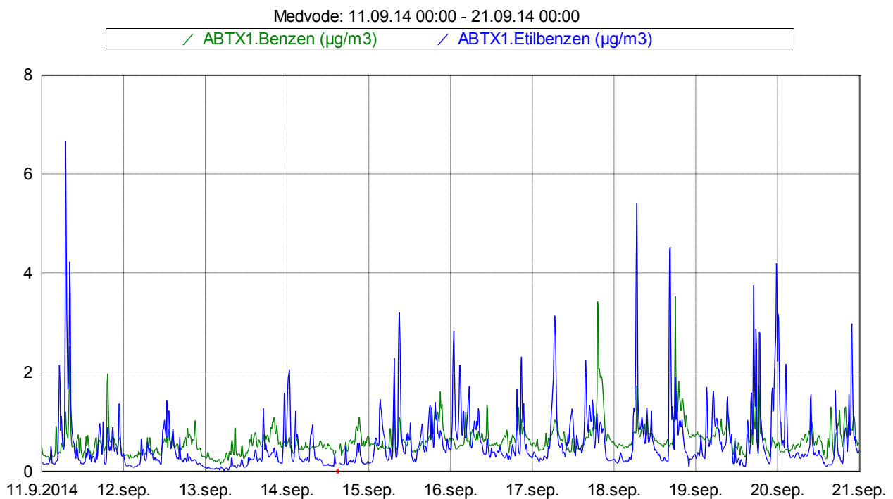
Slika 4: Imisijske koncentracije benzena in etilbenzena med 11. 9. 2014 in 20. 9. 2014.
