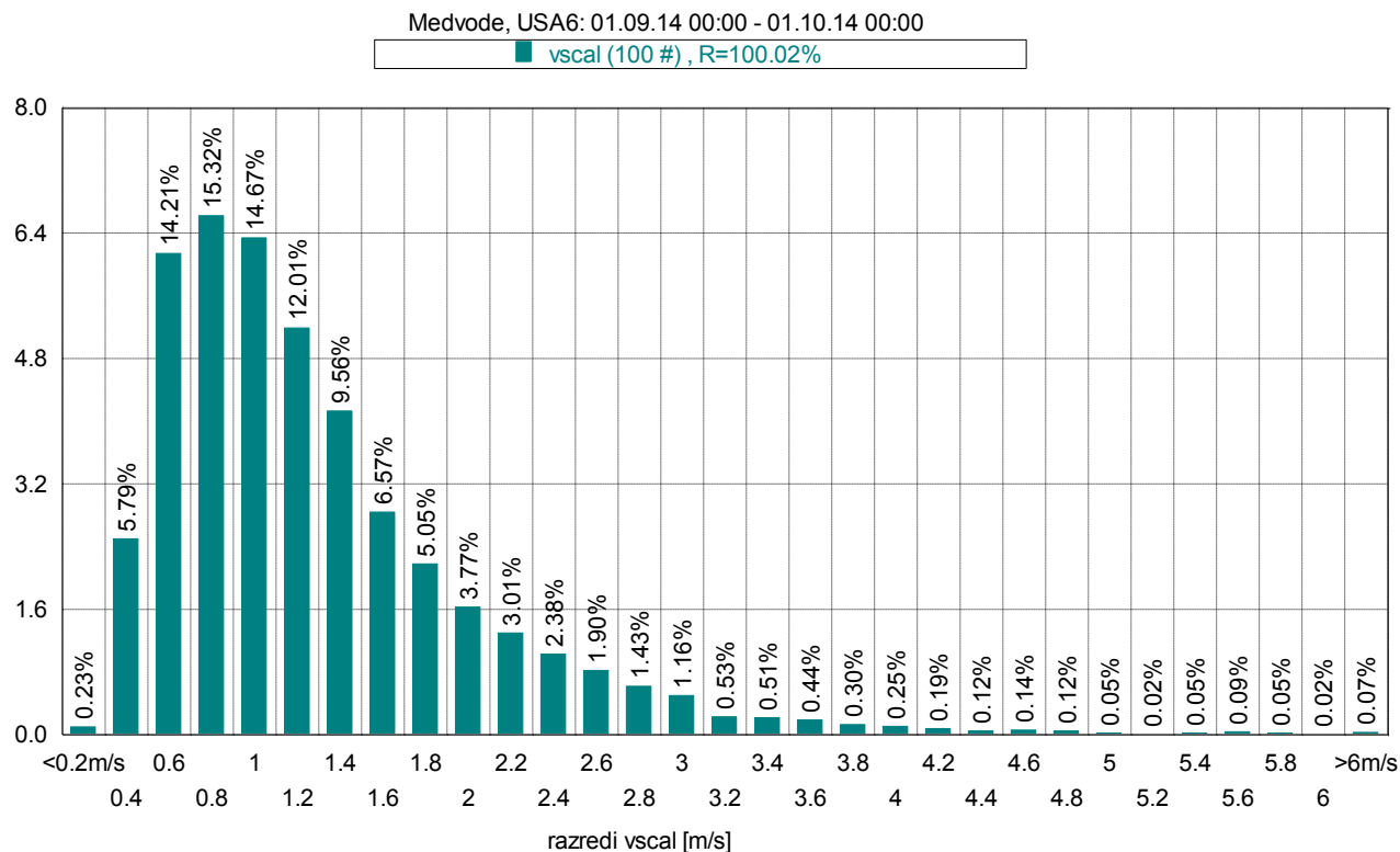
Slika 20: Frekvenčna porazdelitev po hitrosti vetra, september 2014.
