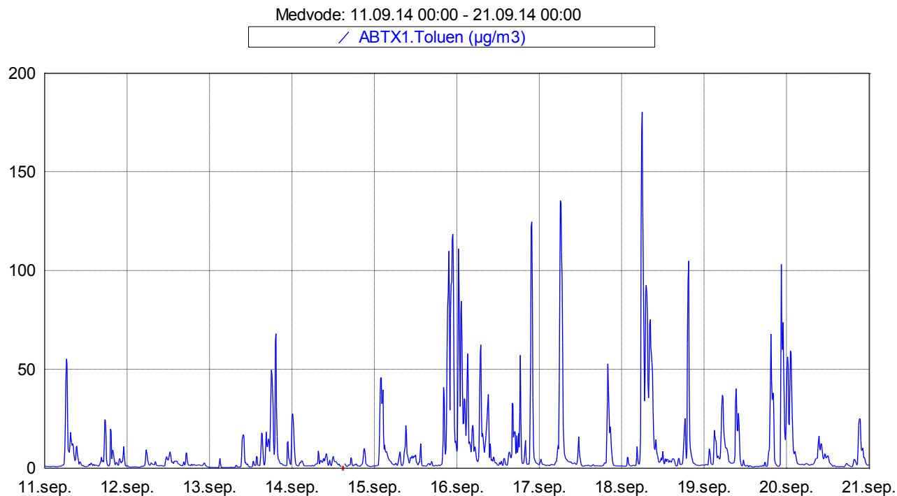
Slika 9: Imisijske koncentracije toluena med 11. 9. 2014 in 20. 9. 2014.
