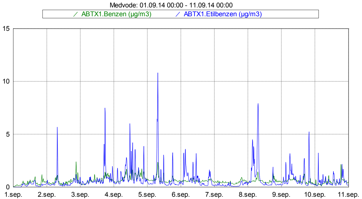
Slika 3: Imisijske koncentracije benzena in etilbenzena med vključno 1. 9. 2014 in 10. 9. 2014.
