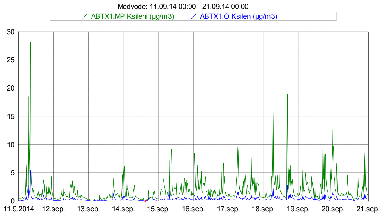
Slika 13: Imisijske koncentracije M&P in O ksilena med 11. 9. 2014 in 20. 9. 2014.
