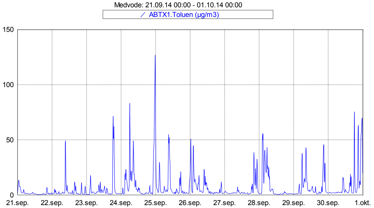
Slika 10: Imisijske koncentracije toluena med 21. 9. 2014 in 30. 9. 2014.
