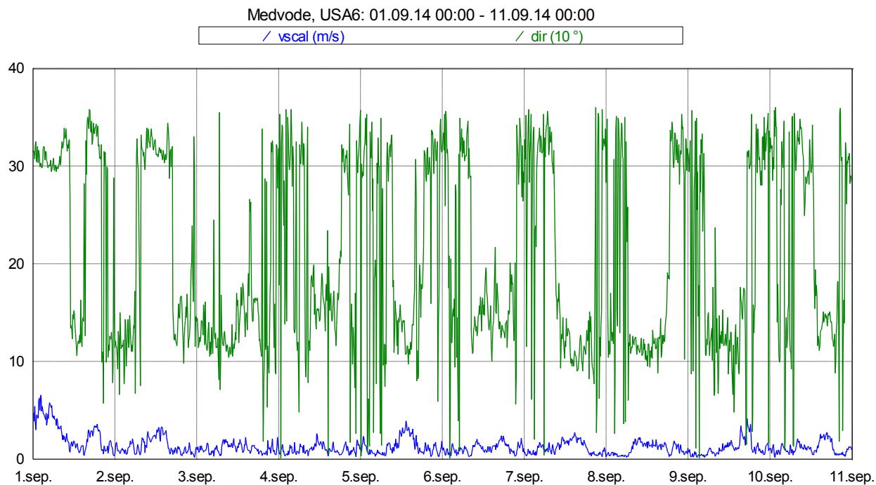
Slika 16: Smer in hitrost vetra med 1. 9. 2014 in 10. 9. 2014.
