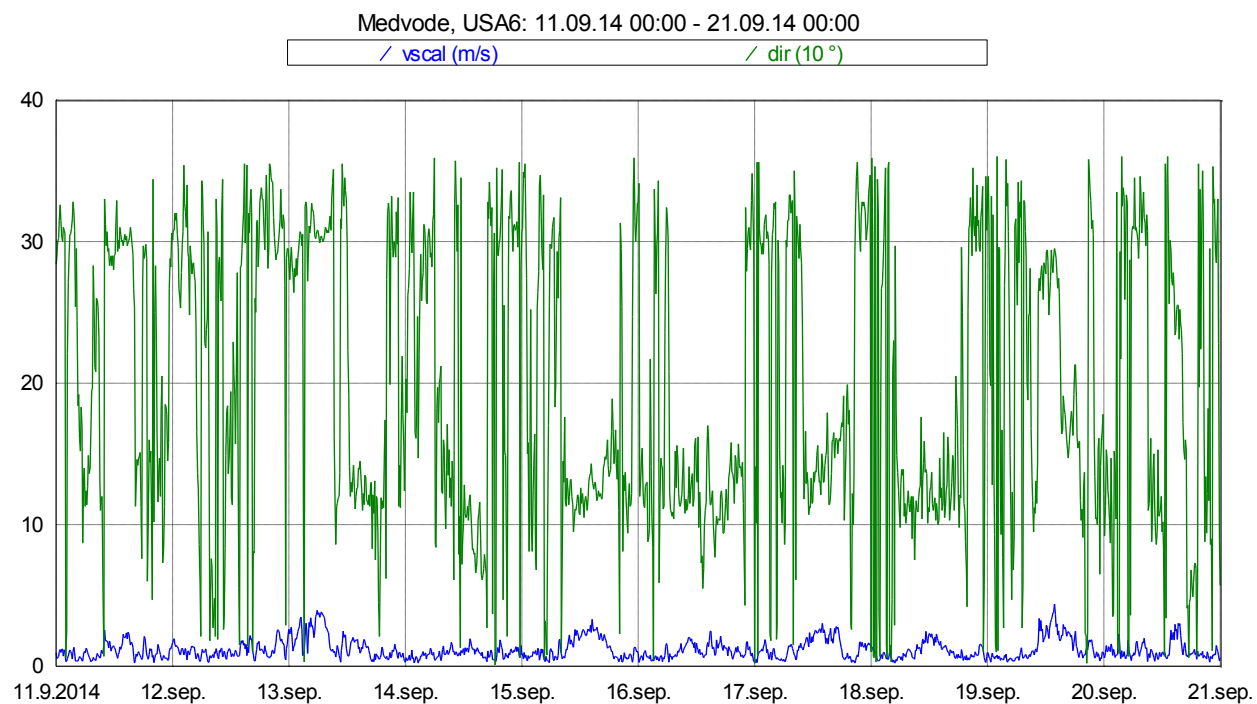
Slika 17: Smer in hitrost vetra med 11. 9. 2014 in 20. 9. 2014.
