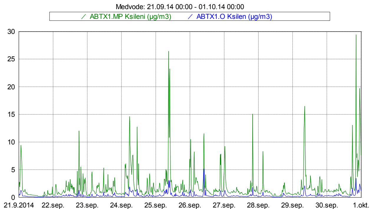
Slika 14: Imisijske koncentracije M&P in O ksilena med 21. 9. 2014 in 30. 9. 2014.
