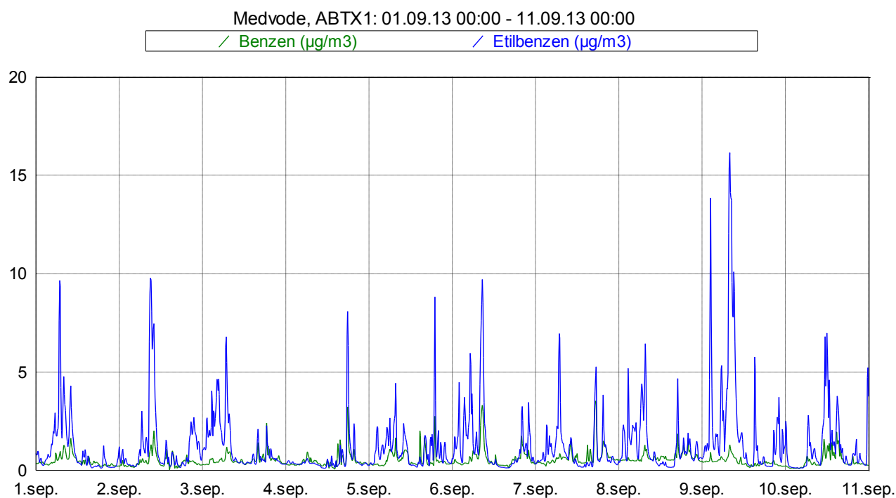
Slika 3: Imisijske koncentracije benzena in etilbenzena med vključno 1. 9. 2013 in 10. 9. 2013.
