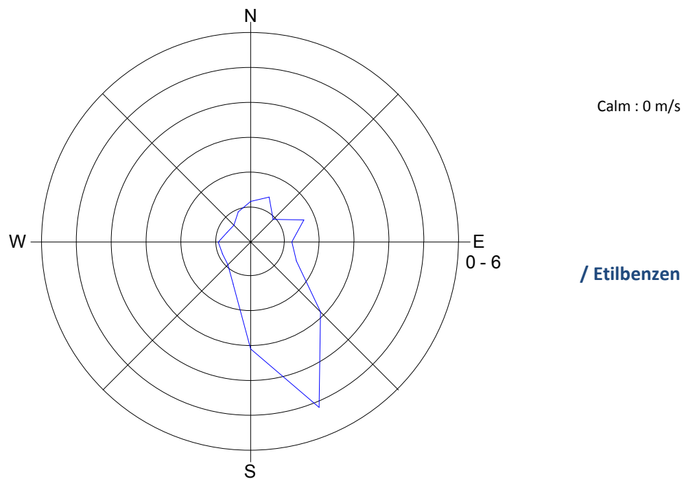
Slika 6: Roža onesnaženosti – benzen (zgoraj) in etilbenzen (spodaj), september 2013.
