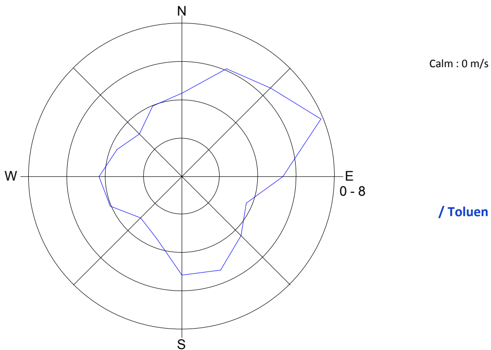
Slika 10: Roža onesnaženost - toluen, september 2013.
