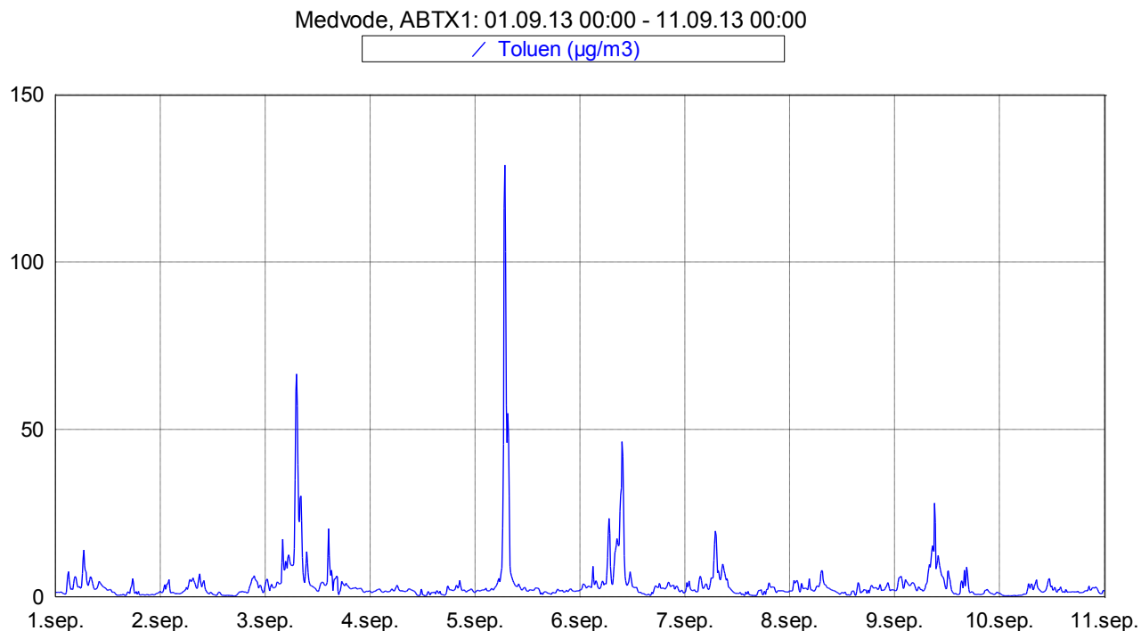
Slika 7: Imisijske koncentracije toluena med vključno 1. 9. 2013 in 11. 9. 2013.
