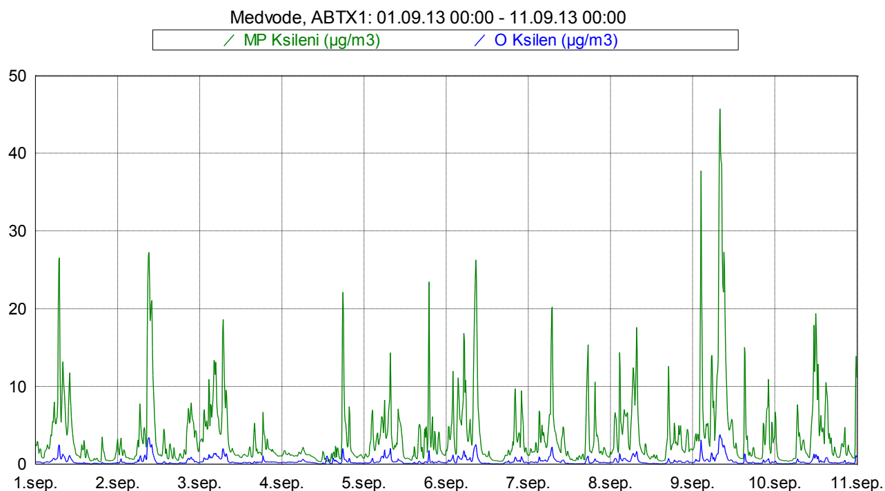
Slika 11: Imisijske koncentracije M&P in O ksilena med vključno 1. 9. 2013 in 10. 9. 2013.
