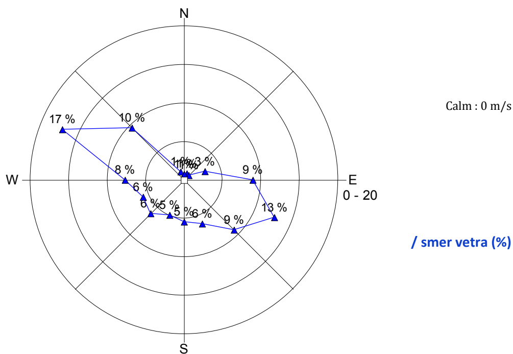
Slika 18: Roža vetrov, september 2013.
