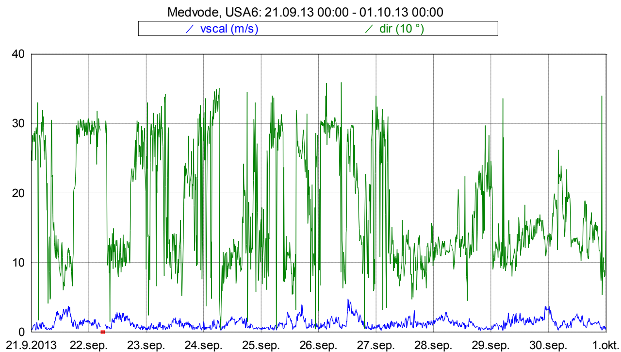
Slika 17: Smer in hitrost vetra med 21. 9. 2013 in 30. 9. 2013.
