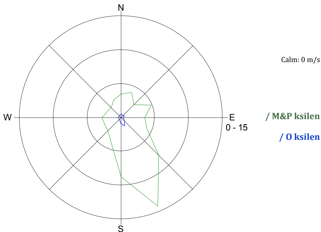
Slika 14: Roža onesnaženosti - M & P ksilen in O ksilen, september 2013.
