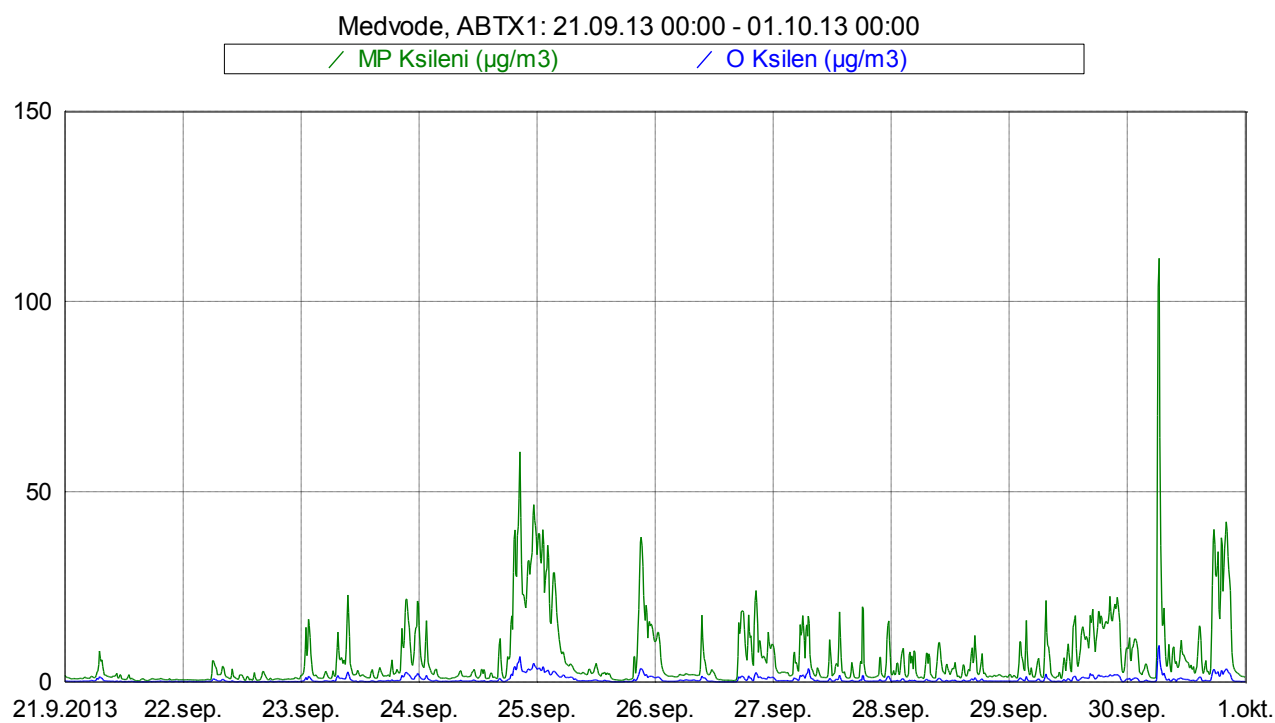
Slika 13: Imisijske koncentracije M&P in O ksilena med 21. 9. 2013 in 30. 9. 2013.
