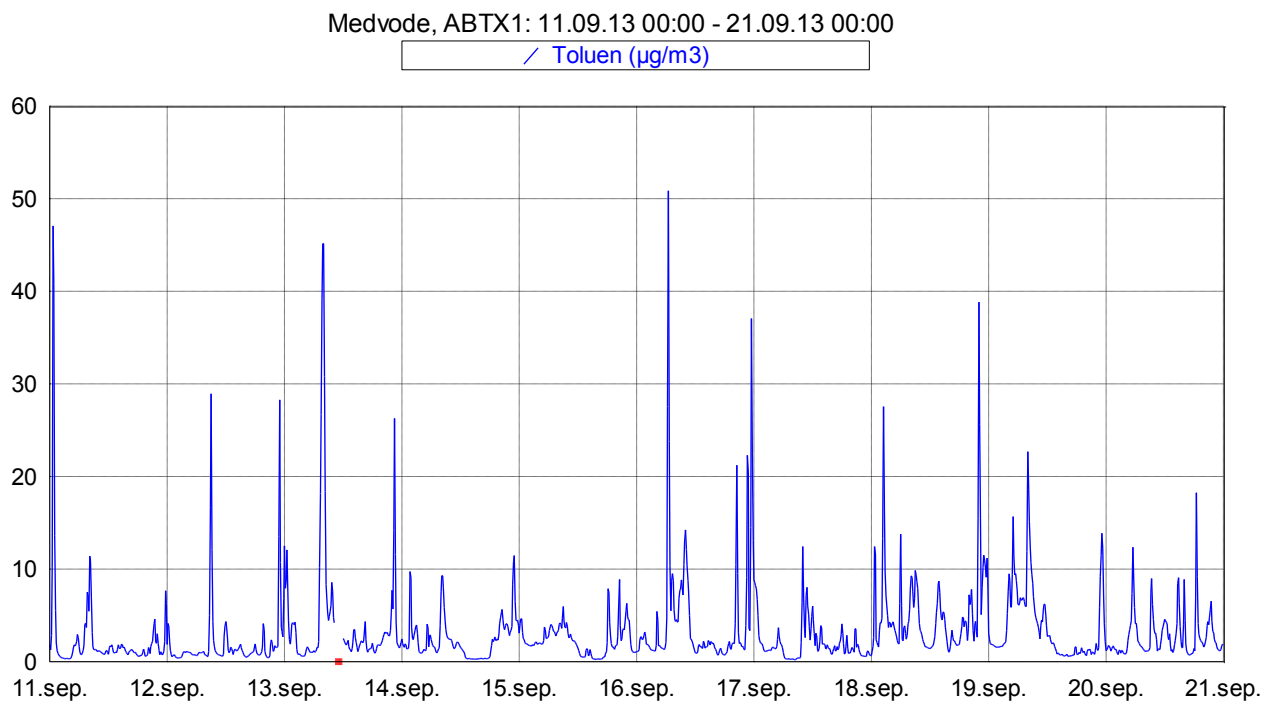
Slika 8: Imisijske koncentracije toluena med 11. 9. 2013 in 20. 9. 2013.
