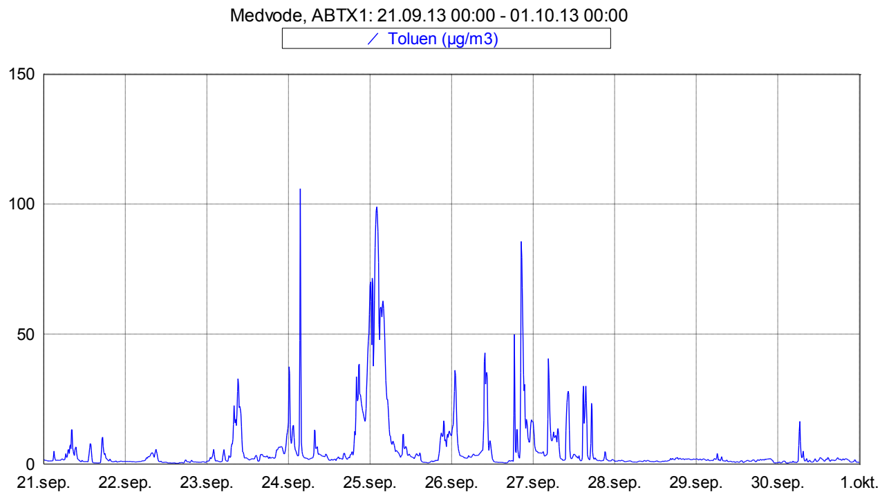
Slika 9: Imisijske koncentracije toluena med 21. 9. 2013 in 30. 9. 2013.
