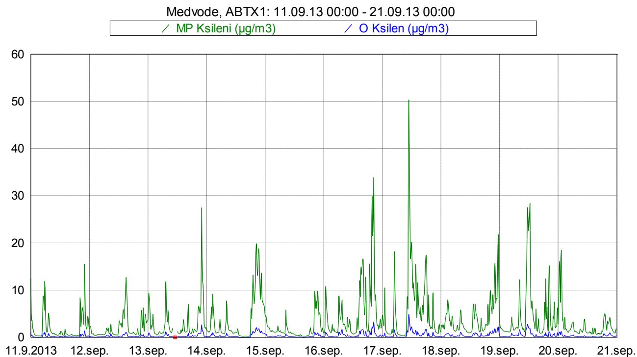
Slika 12: Imisijske koncentracije M&P in O ksilena med 11. 9. 2013 in 20. 9. 2013.
