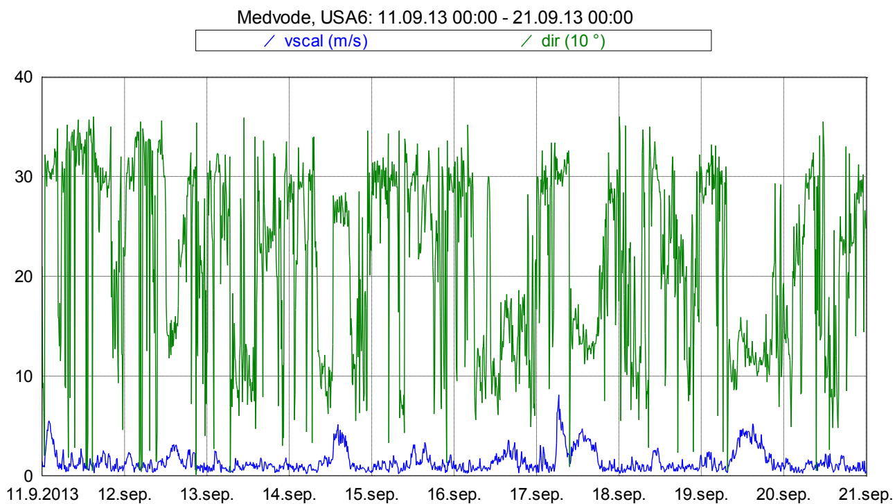
Slika 16: Smer in hitrost vetra med 11. 9. 2013 in 20. 9. 2013.
