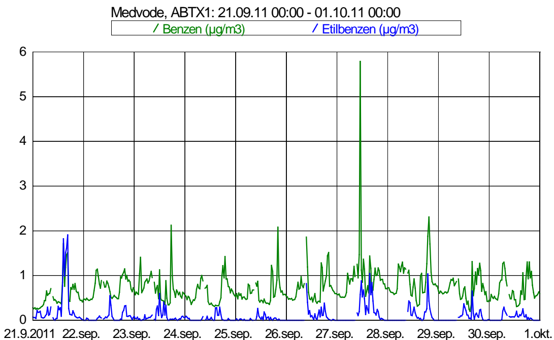
Slika 5: Imisijske koncentracije benzena in etilbenzena med 21. 9. 2011 in 1. 10. 2011.
