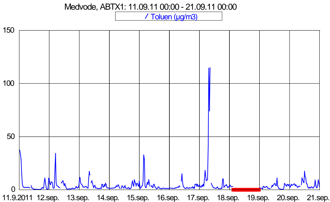
Slika 8: Imisijske koncentracije toluena med 11. 9. 2011 in 20. 9. 2011.
