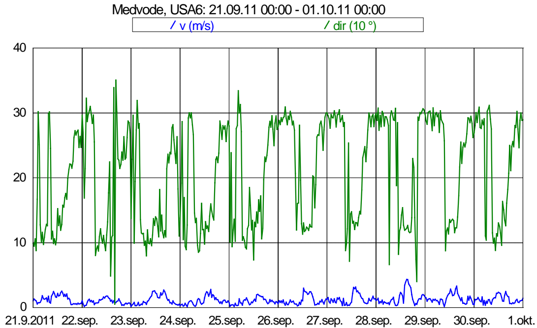
Slika 17: Smer in hitrost vetra med 21. 9. 2011 in 1. 10. 2011.
