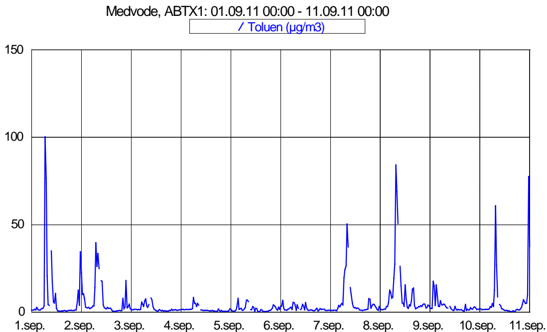
Slika 7: Imisijske koncentracije toluena med 1. 9. 2011 in 10. 9. 2011.
