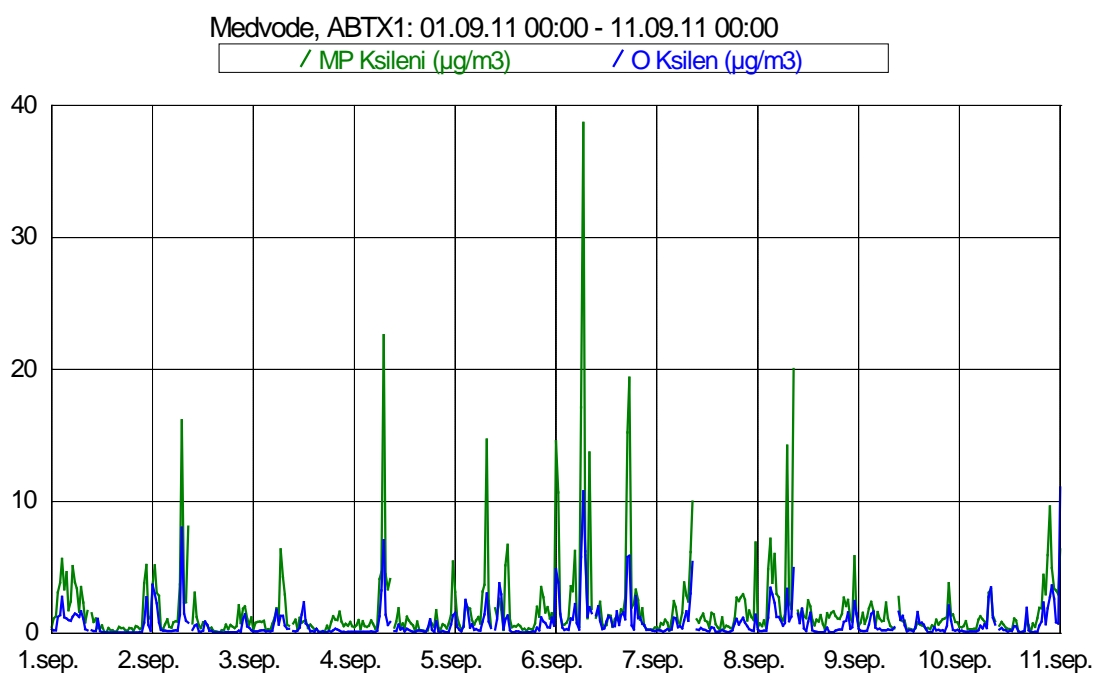
Slika 11: Imisijske koncentracije M&P in O ksilena med 1. 9. 2011 in 10. 10. 2011.
