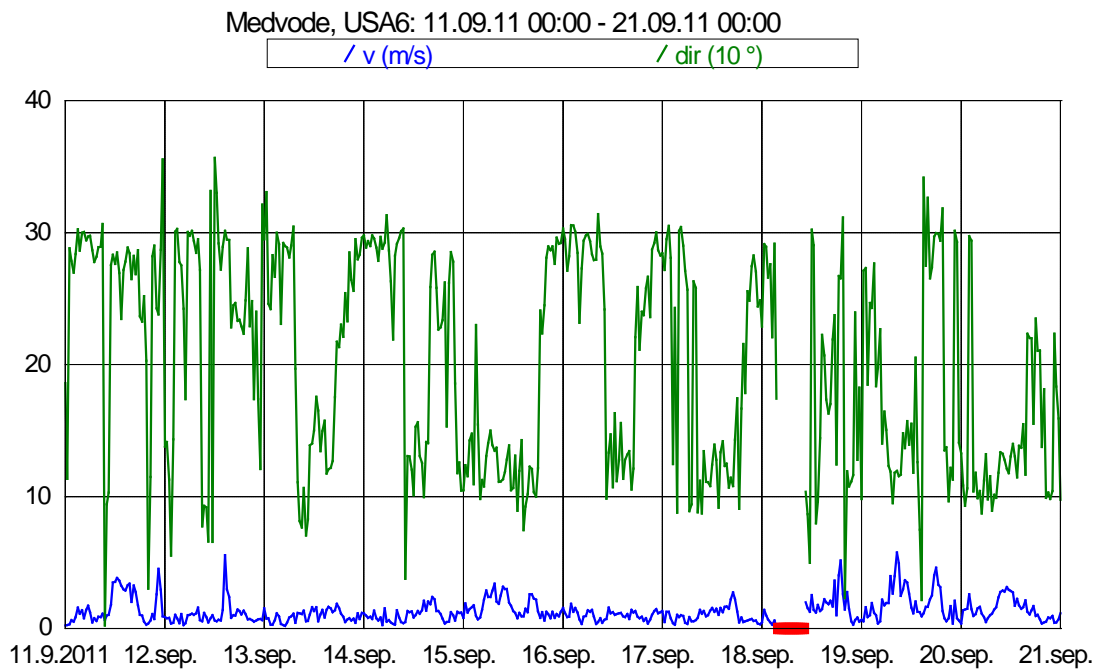
Slika 16: Smer in hitrost vetra med 11. 9. 2011 in 20. 9. 2011.
