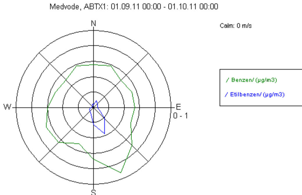
Slika 6: Roža onesnaženosti - benzen in etilbenzen, september 2011.
