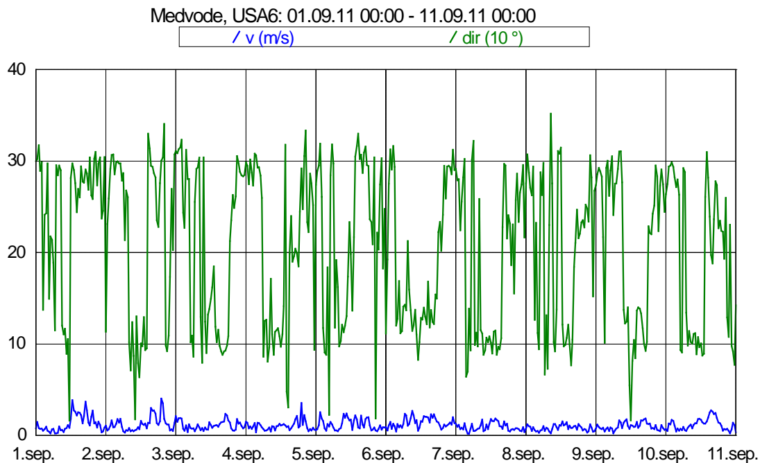
Slika 15: Smer in hitrost vetra med 1. 9. 2011 in 10. 9. 2011.
