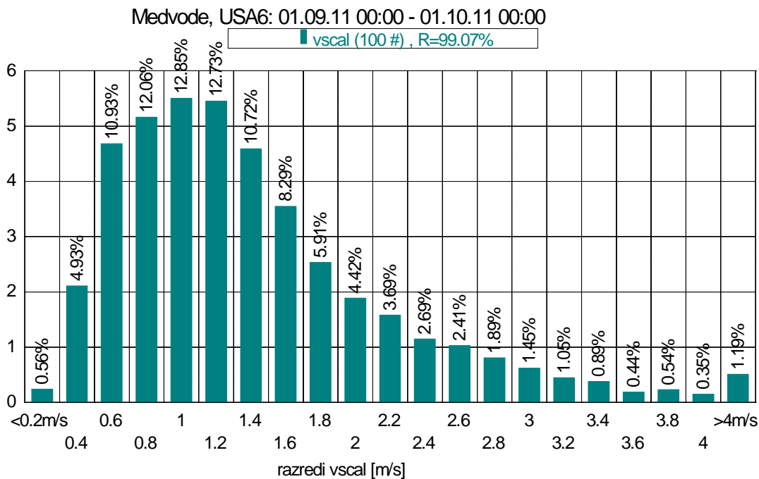
Slika 19: Frekvenčna porazdelitev- pogostost hitrosti vetra po razredih hitrosti, sep. 2011.
