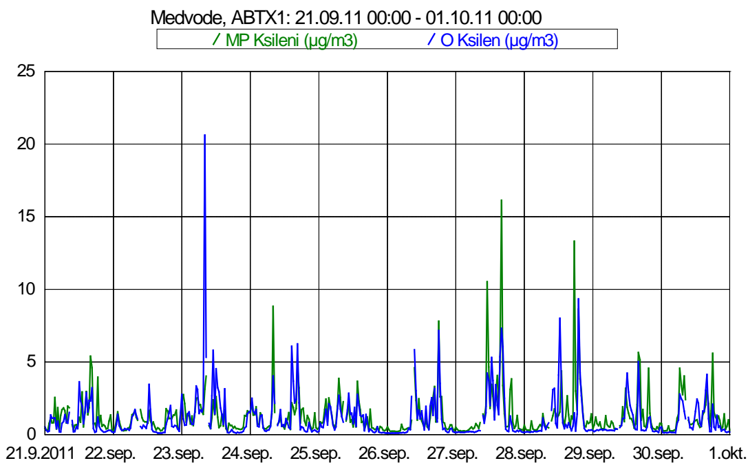
Slika 13: Imisijske koncentracije M&P in O ksilena med 21. 9. 2011 in 1. 10. 2011.
