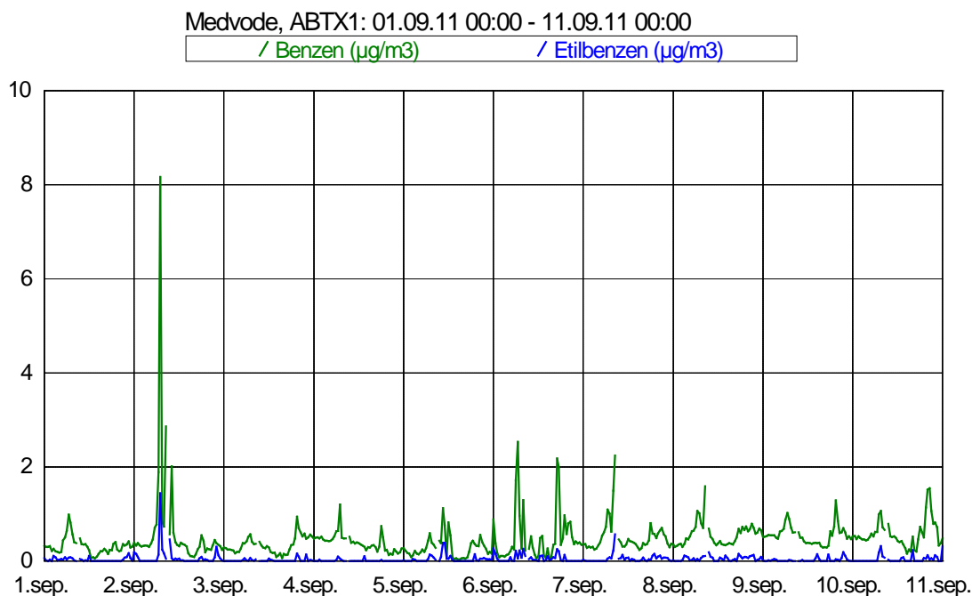
Slika 3: Imisijske koncentracije benzena in etilbenzena med 1. 9. 2011 in 10. 9. 2011.
