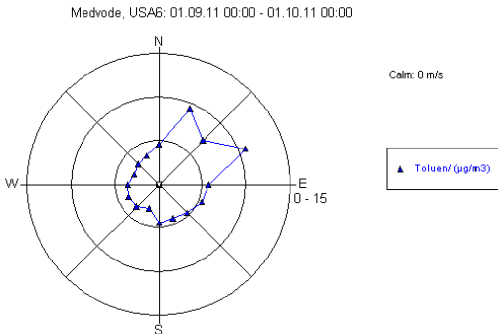
Slika 10: Roža onesnaženost - toluen, september 2011.
