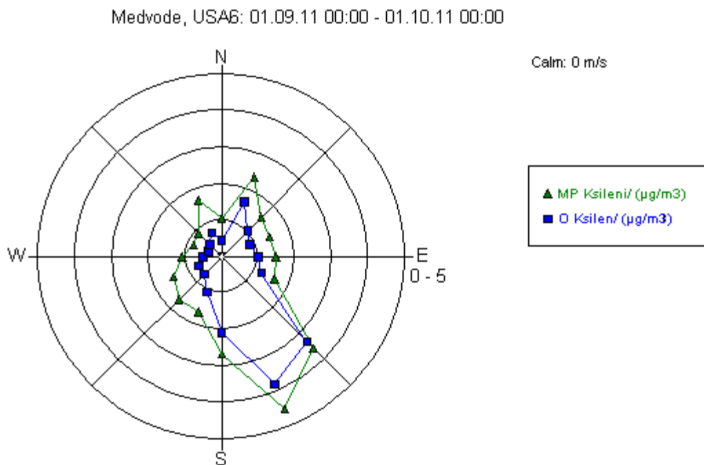
Slika 14: Roža onesnaženosti - M & P ksilen in O ksilen, september 2011.
