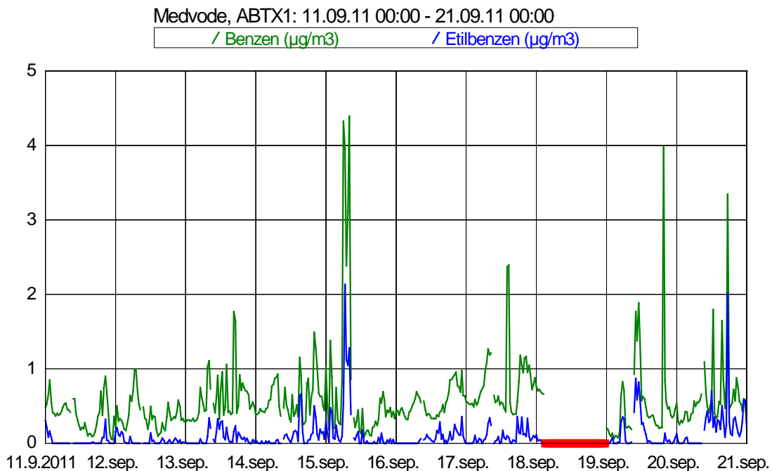
Slika 4: Imisijske koncentracije benzena in etilbenzena med 11. 9. 2011 in 20. 9. 2011.
