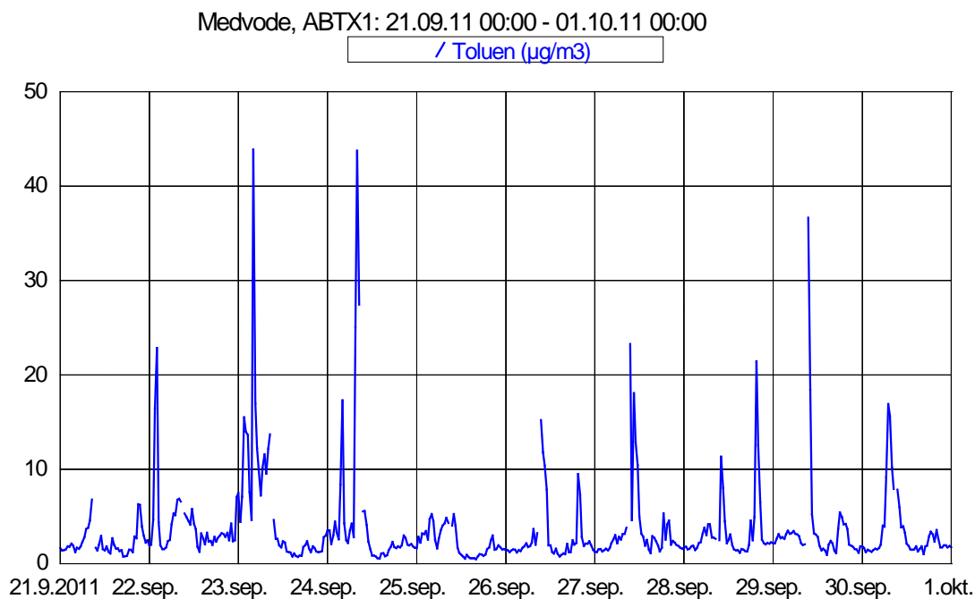
Slika 9: Imisijske koncentracije toluena med 21. 9. 2011 in 1. 10. 2011.
