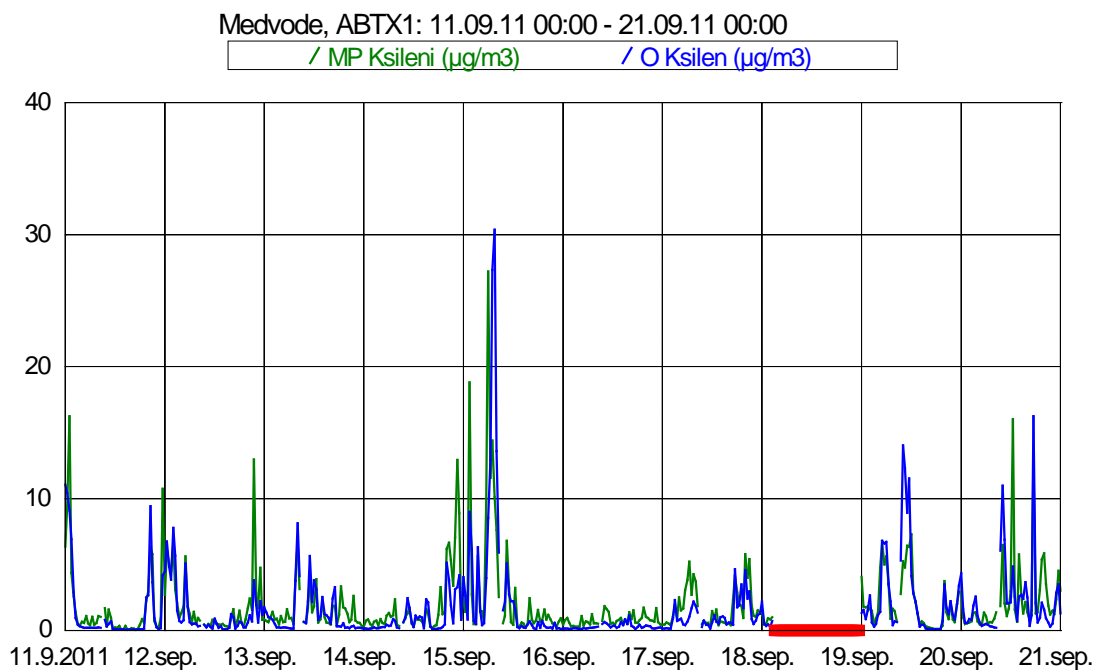
Slika 12: Imisijske koncentracije M&P in O ksilena med 11. 9. 2011 in 20. 10. 2011.
