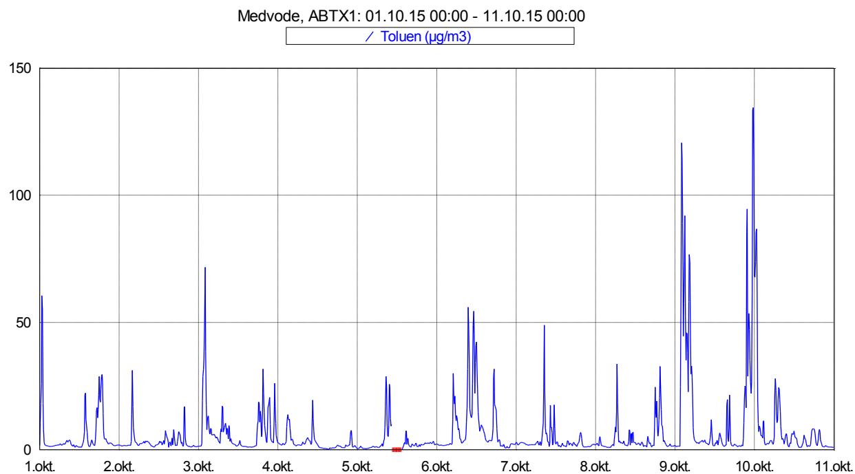
Slika 8: Imisijske koncentracije toluena med vključno 1. 10. 2015 in 10. 10. 2015.
