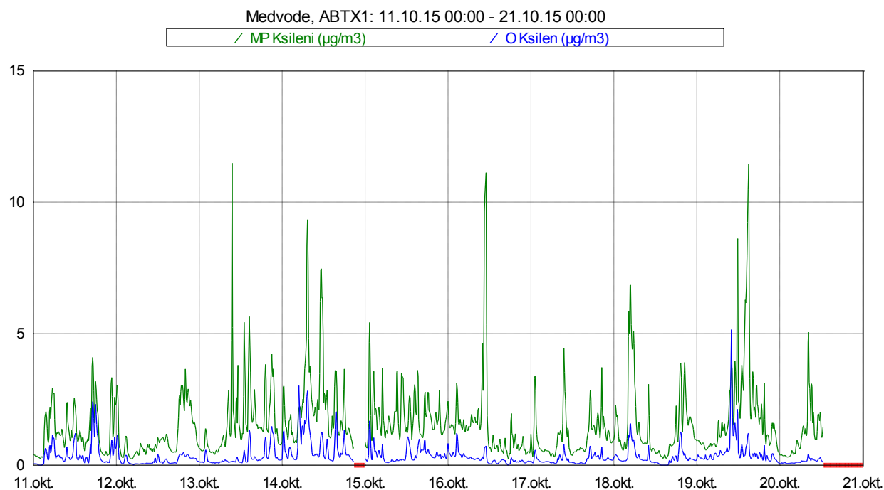
Slika 13: Imisijske koncentracije M&P in O ksilena med 11. 10. 2015 in 20. 10. 2015.
