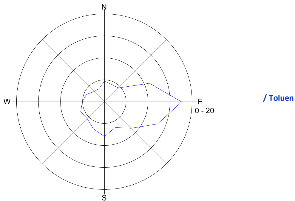
Slika 11: Roža onesnaženost - toluen, oktober 2015.
