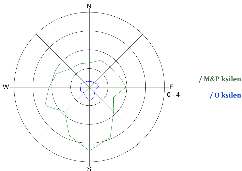
Slika 15: Roža onesnaženosti - M & P ksilen in O ksilen, oktober 2015.
