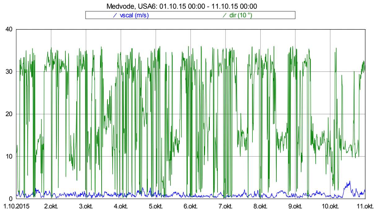
Slika 16: Smer in hitrost vetra med 1. 10. 2015 in 10. 10. 2015.
