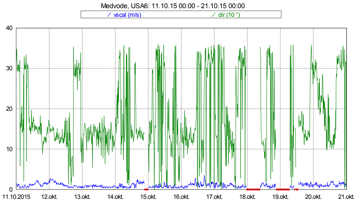
Slika 17: Smer in hitrost vetra med 11. 10. 2015 in 20. 10. 2015.
