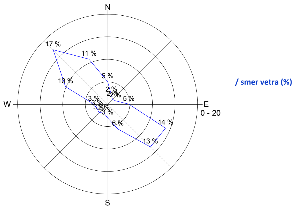
Slika 19: Roža vetrov, oktober 2015.
