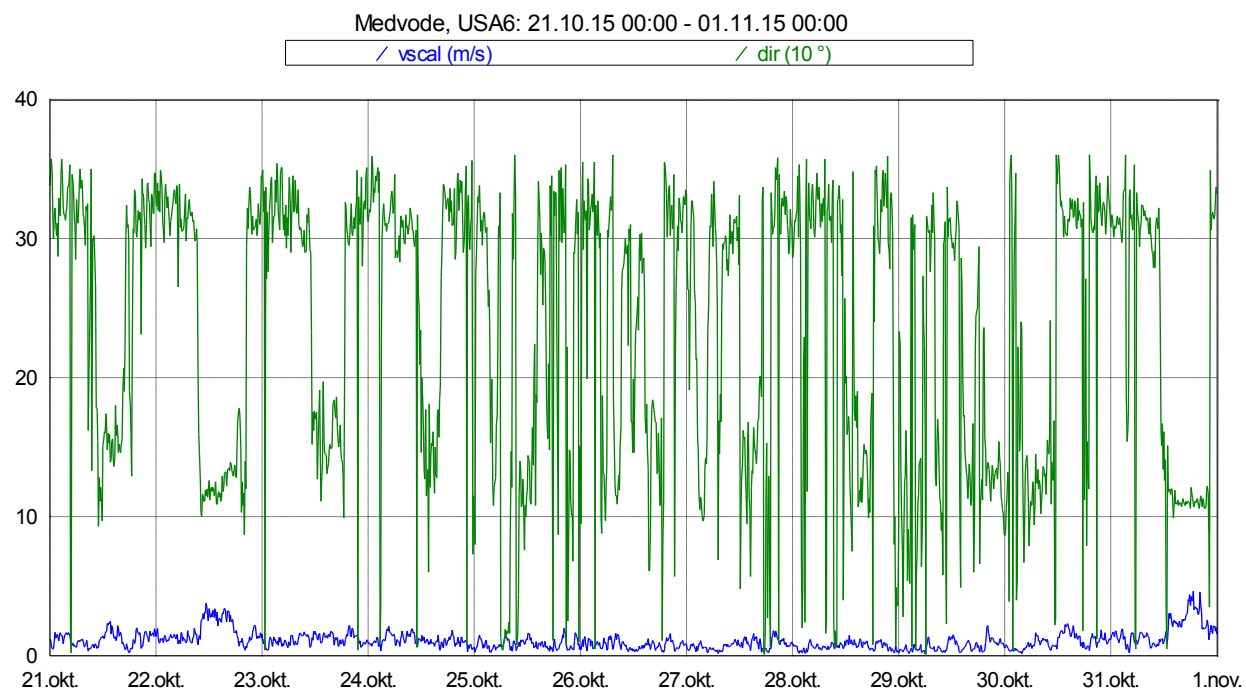
Slika 18: Smer in hitrost vetra med 21. 10. 2015 in 31. 10. 2015.
