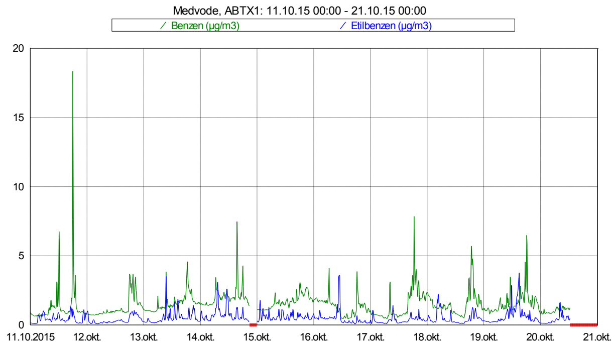
Slika 4: Imisijske koncentracije benzena in etilbenzena med 11. 10. 2015 in 20. 10. 2015.
