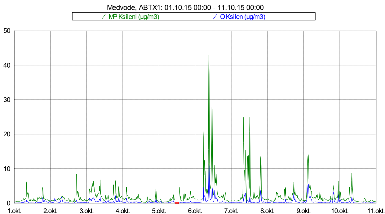
Slika 12: Imisijske koncentracije M&P in O ksilena med vključno 1. 10. 2015 in 10. 10. 2015.
