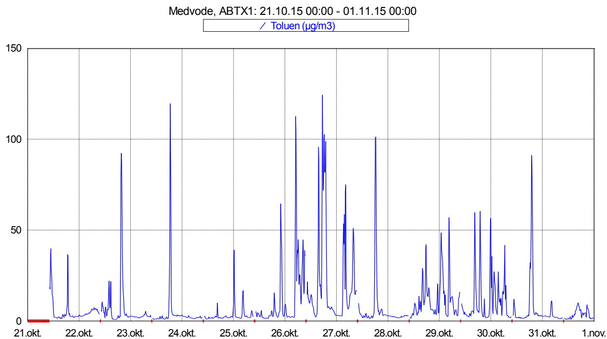
Slika 10: Imisijske koncentracije toluena med 21. 10. 2015 in 31. 10. 2015.
