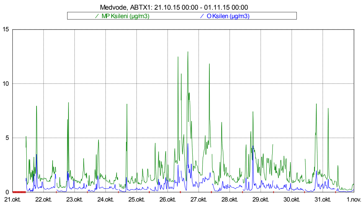
Slika 14: Imisijske koncentracije M&P in O ksilena med 21. 10. 2015 in 31. 10. 2015.
