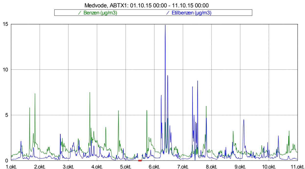
Slika 3: Imisijske koncentracije benzena in etilbenzena med vključno 1. 10. 2015 in 10. 10. 2015.
