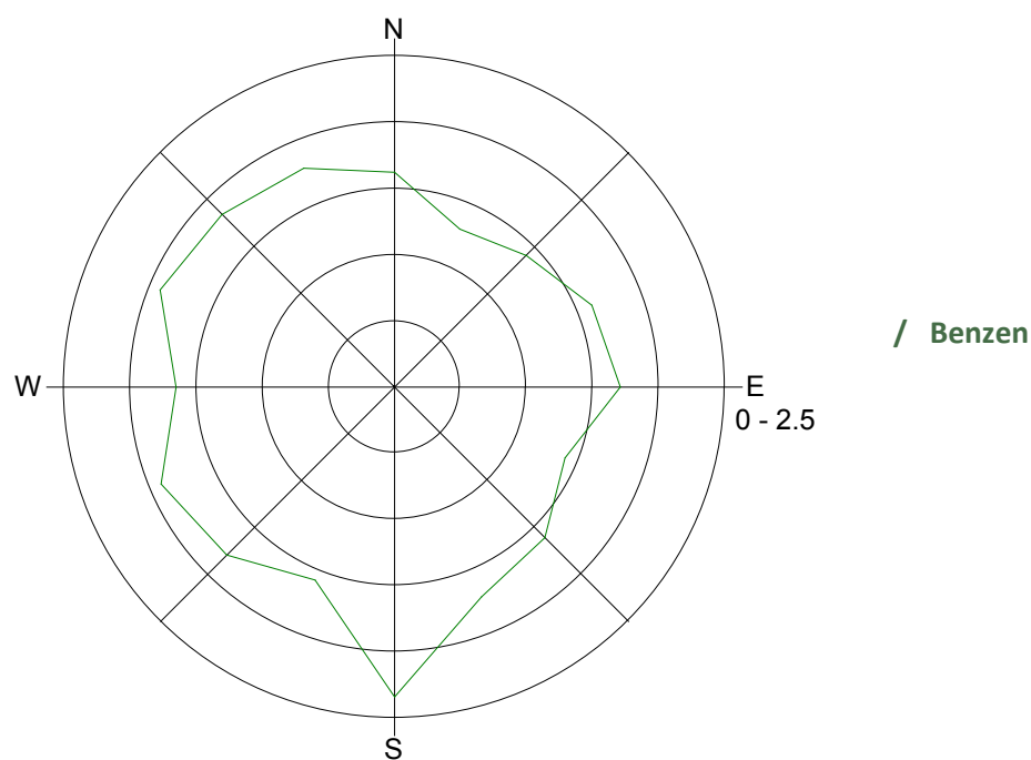
Slika 6: Roža onesnaženosti – benzen, oktober 2015.
