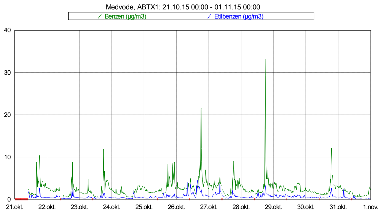
Slika 5: Imisijske koncentracije benzena in etilbenzena med 21. 10. 2015 in 31. 10. 2015.
