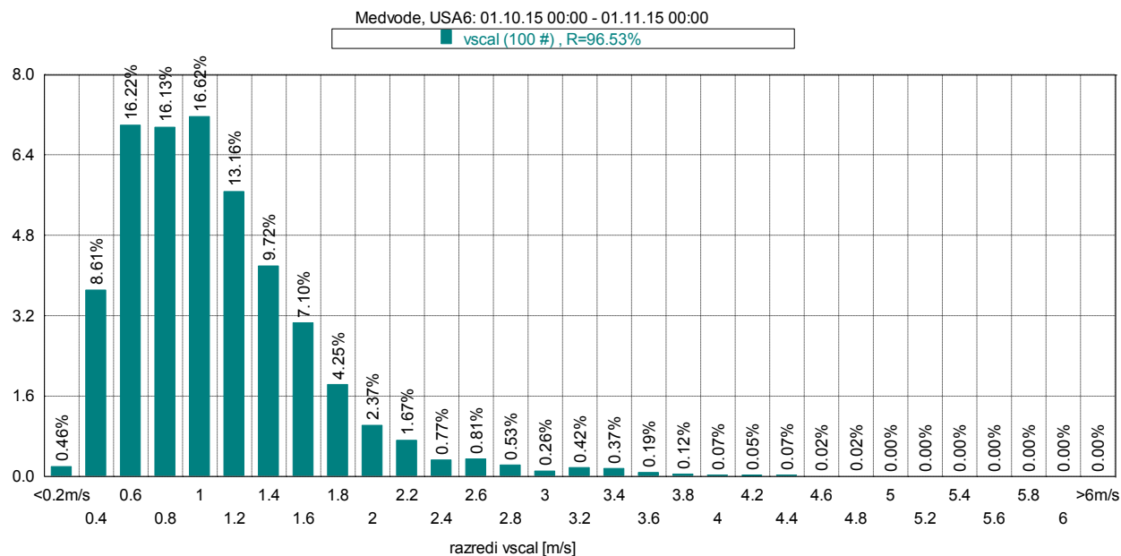
Slika 20: Frekvenčna porazdelitev po hitrosti vetra, oktober 2015.
