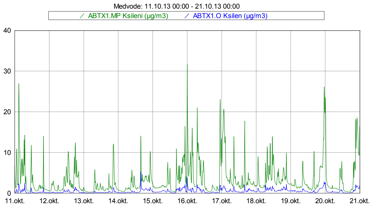
Slika 13: Imisijske koncentracije M&P in O ksilena med 11. 10. 2013 in 20. 10. 2013.
