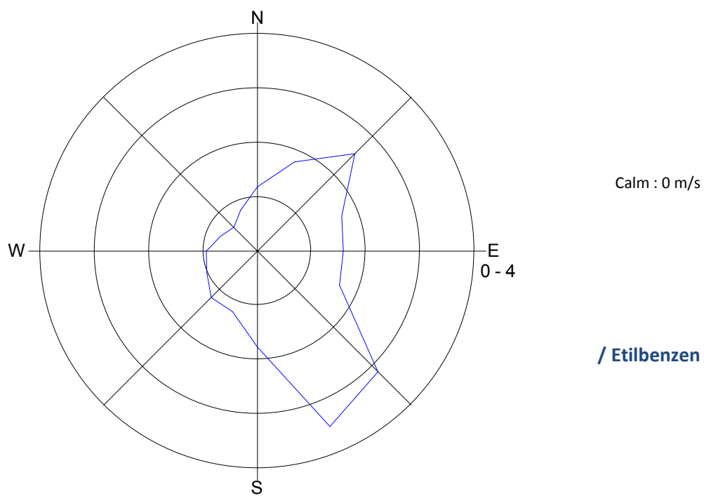
Slika 6: Roža onesnaženosti – benzen (zgoraj) in etilbenzen (spodaj), oktober 2013.
