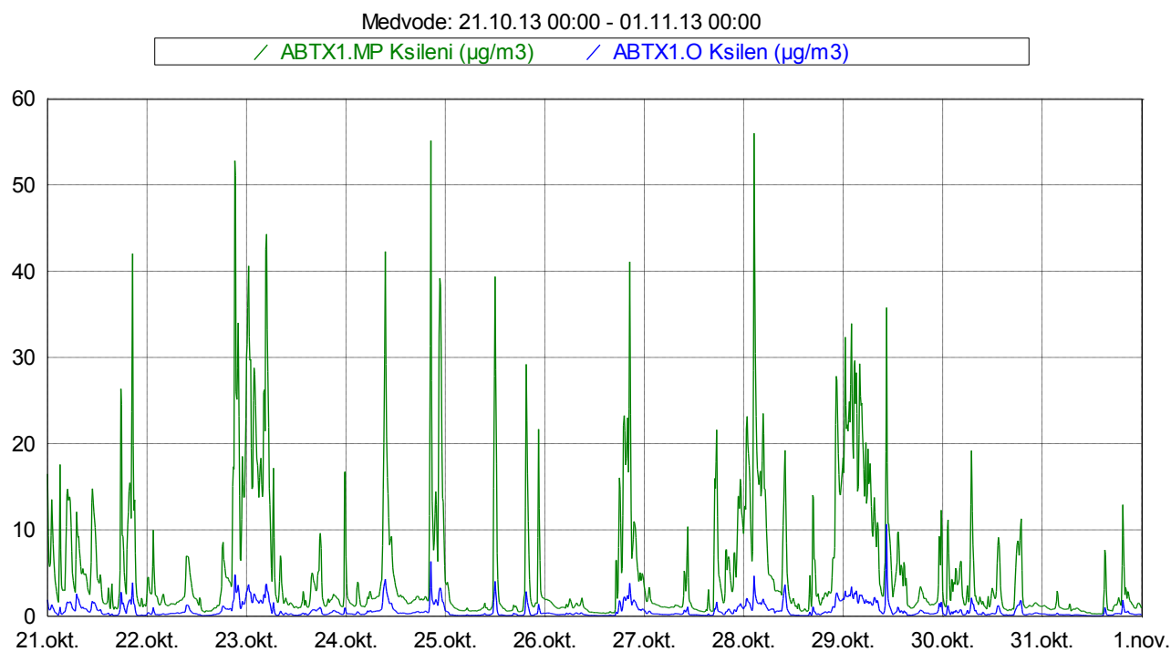
Slika 14: Imisijske koncentracije M&P in O ksilena med 21. 10. 2013 in 31. 10. 2013.
