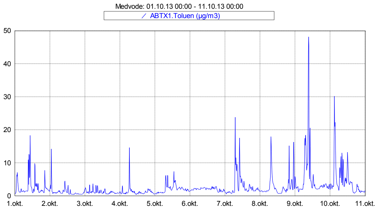
Slika 7: Imisijske koncentracije toluena med vključno 1. 10. 2013 in 10. 10. 2013.
