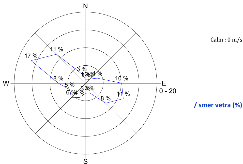
Slika 20: Roža vetrov, oktober 2013.
