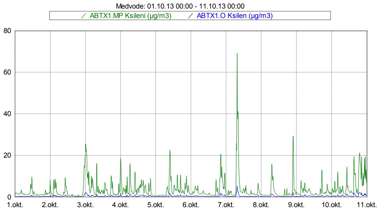
Slika 12: Imisijske koncentracije M&P in O ksilena med vključno 1. 10. 2013 in 10. 10. 2013.
