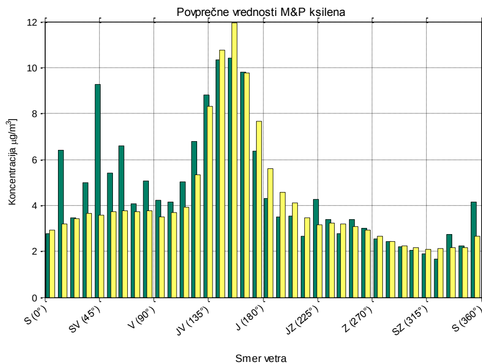
Slika 16: Primerjava povprečnih vrednosti M&P ksilena oktobra 2013 in v obdobju 2012-2013 po smereh vetra.
