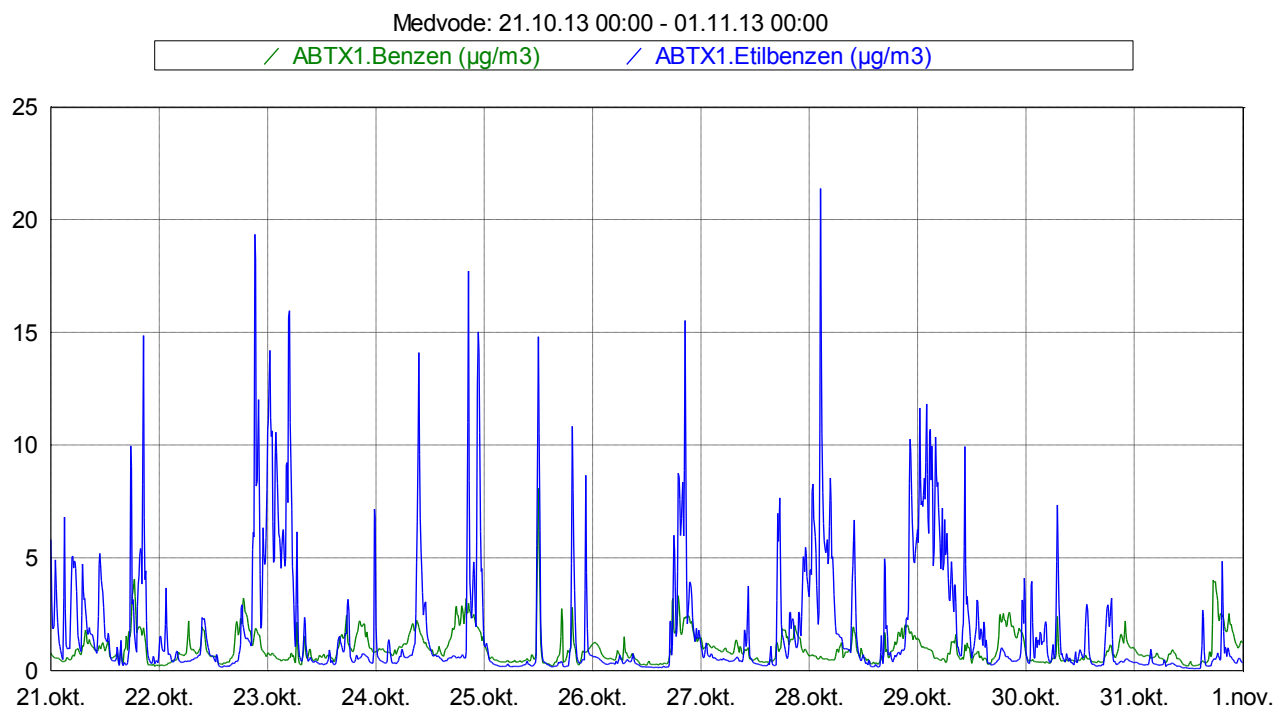
Slika 5: Imisijske koncentracije benzena in etilbenzena med 21. 10. 2013 in 31. 10. 2013.
