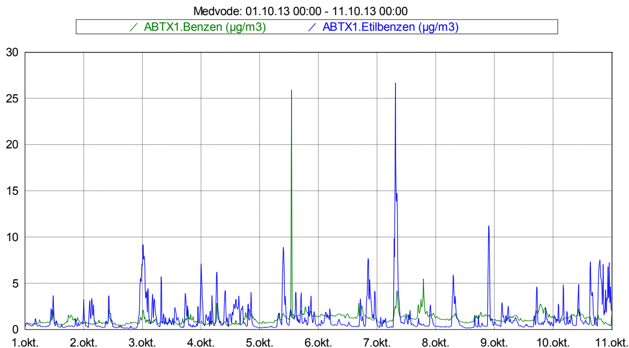
Slika 3: Imisijske koncentracije benzena in etilbenzena med vključno 1. 10. 2013 in 10. 10. 2013.
