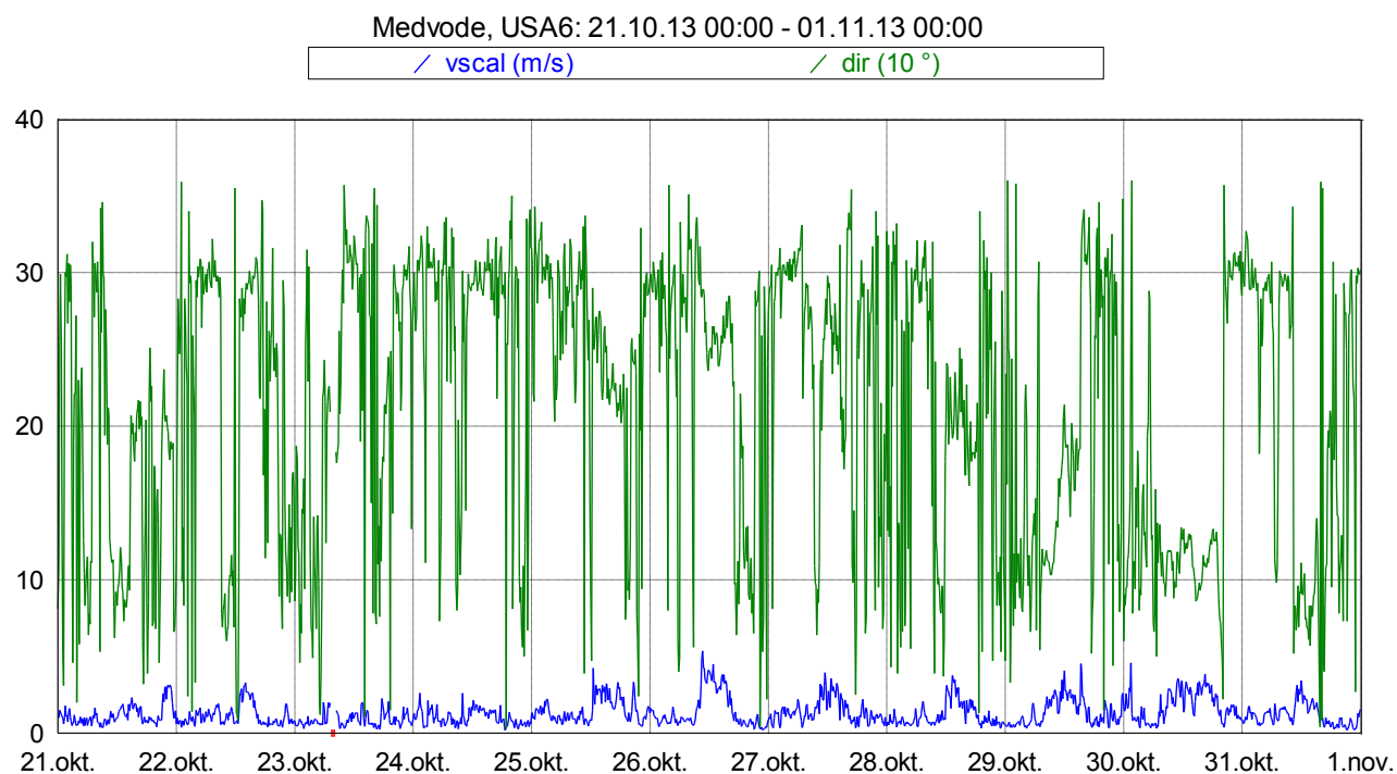
Slika 19: Smer in hitrost vetra med 21. 10. 2013 in 31. 10. 2013.
