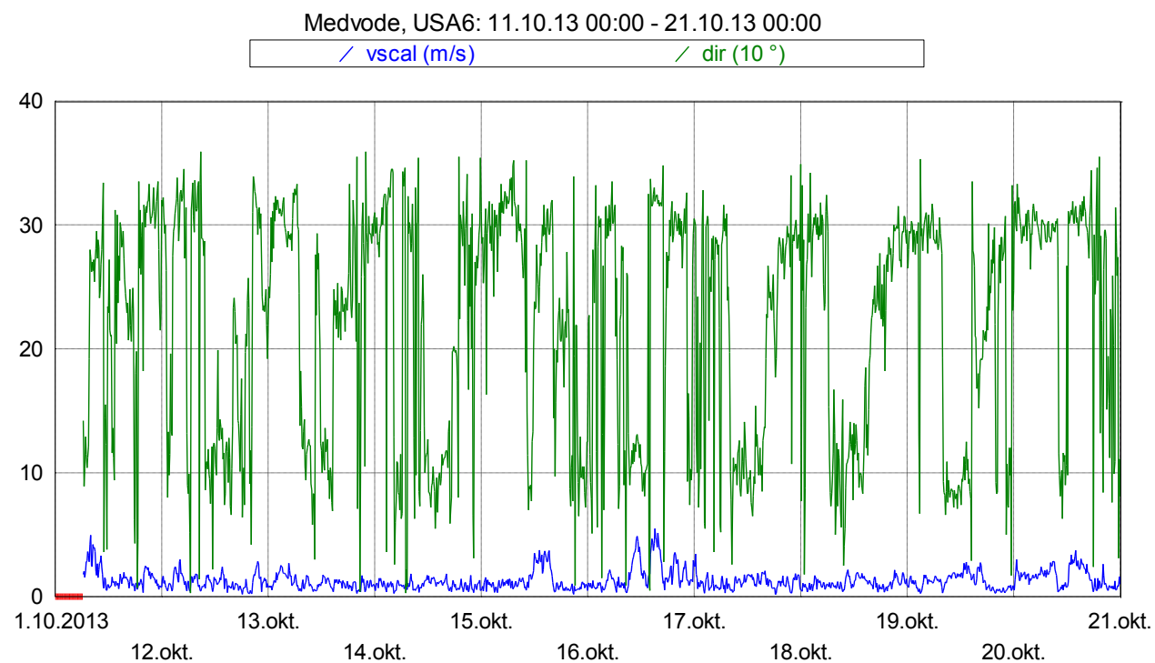
Slika 18: Smer in hitrost vetra med 11. 10. 2013 in 20. 10. 2013.
