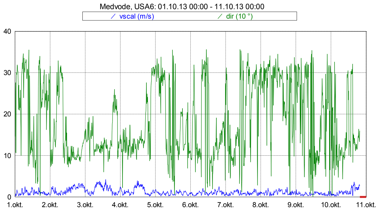
Slika 17: Smer in hitrost vetra med 1. 10. 2013 in 10. 10. 2013.
