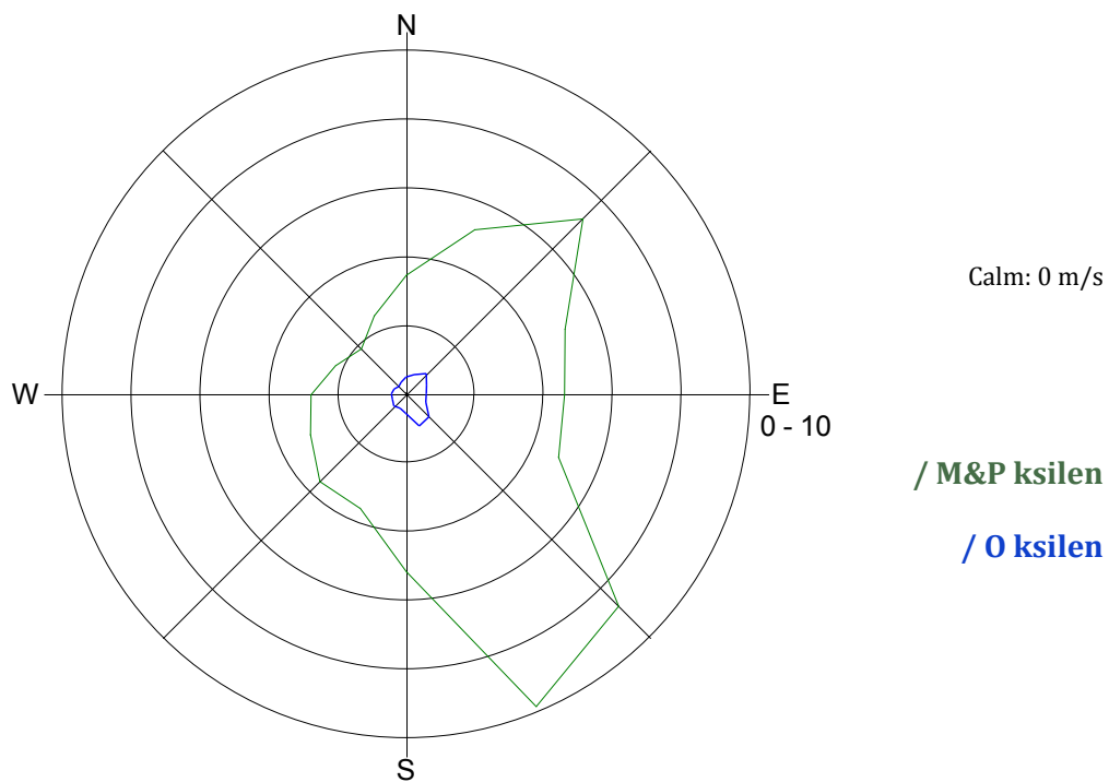
Slika 15: Roža onesnaženosti - M & P ksilen in O ksilen, oktober 2013.
