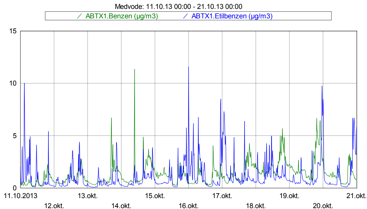
Slika 4: Imisijske koncentracije benzena in etilbenzena med 11. 10. 2013 in 20. 10. 2013.
