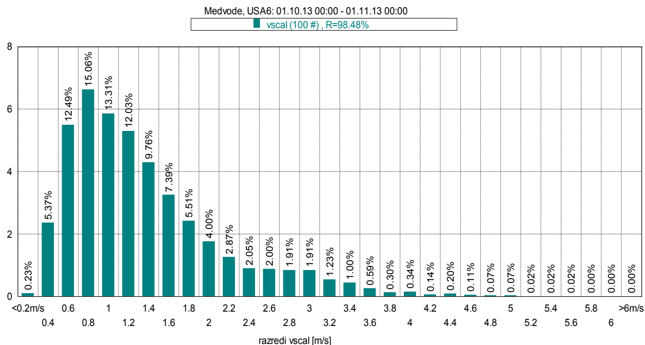
Slika 21: Frekvenčna porazdelitev po hitrosti vetra, oktober 2013.
