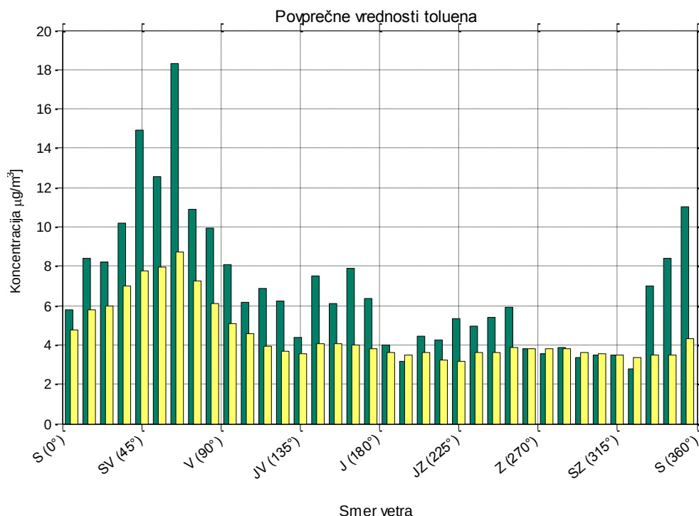
Slika 11: Primerjava povprečnih vrednosti toluena oktobra 2013 in v obdobju 2012-2013 po smereh vetra.
