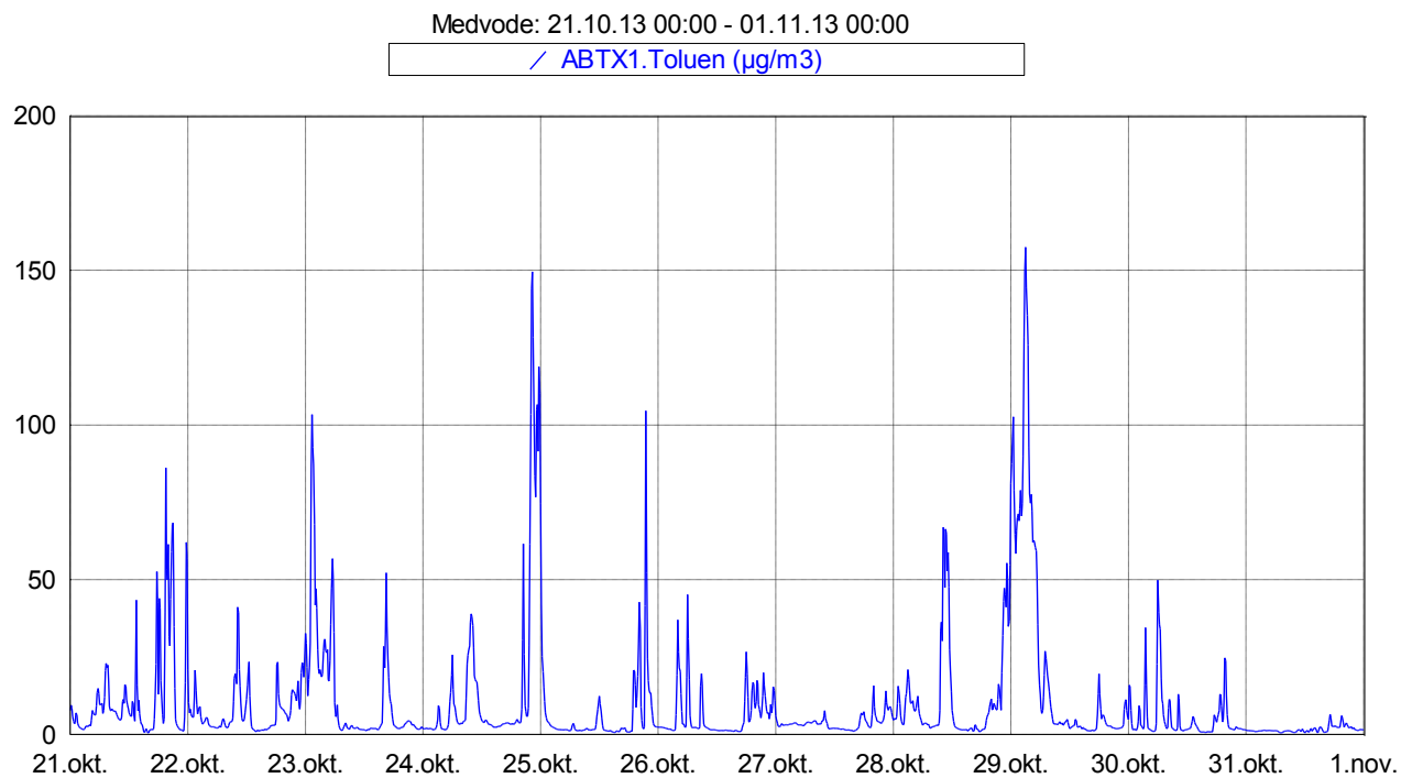
Slika 9: Imisijske koncentracije toluea med 21. 10. 2013 in 31. 10. 2013.
