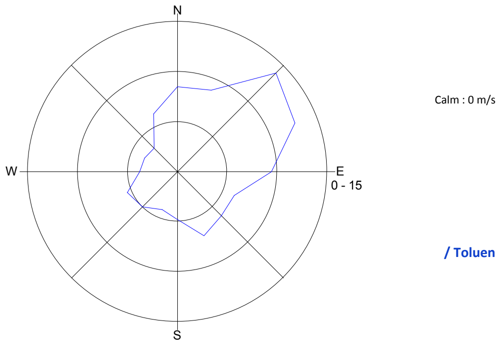
Slika 10: Roža onesnaženost - toluen, oktober 2013.
