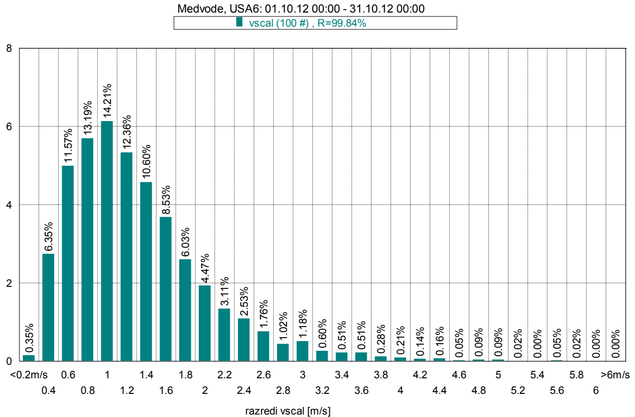
Slika 19: Frekvenčna porazdelitev po hitrosti vetra, oktober 2012.
