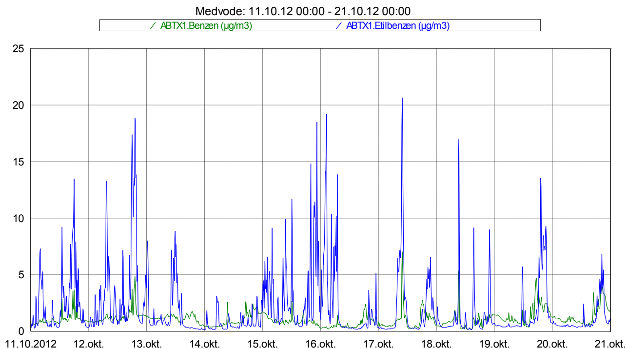
Slika 4: Imisijske koncentracije benzena in etilbenzena med 11. 10. 2012 in 21. 10. 2012.
