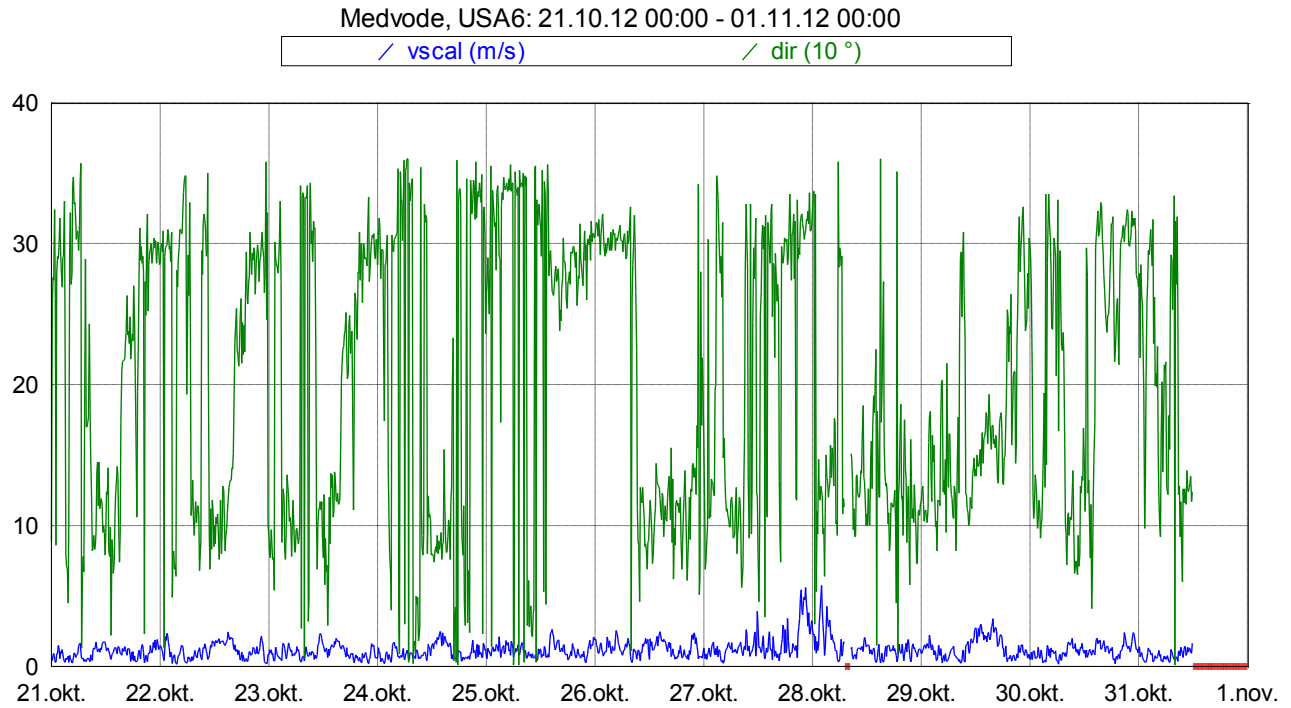
Slika 17: Smer in hitrost vetra med 21. 10. 2012 in 31. 10. 2012.
