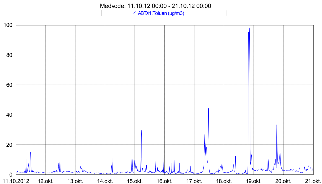
Slika 8: Imisijske koncentracije toluena med 11. 10. 2012 in 21. 10. 2012.
