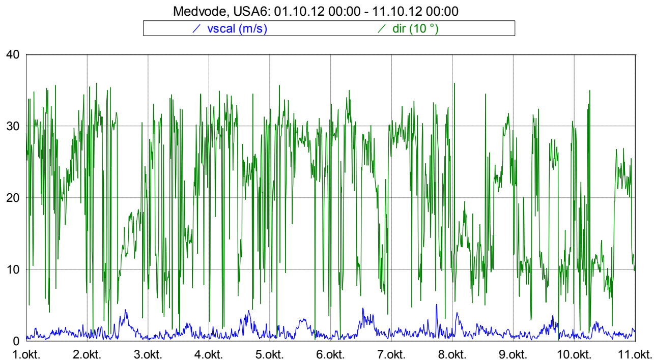
Slika 15: Smer in hitrost vetra med 1. 10. 2012 in 11. 10. 2012.
