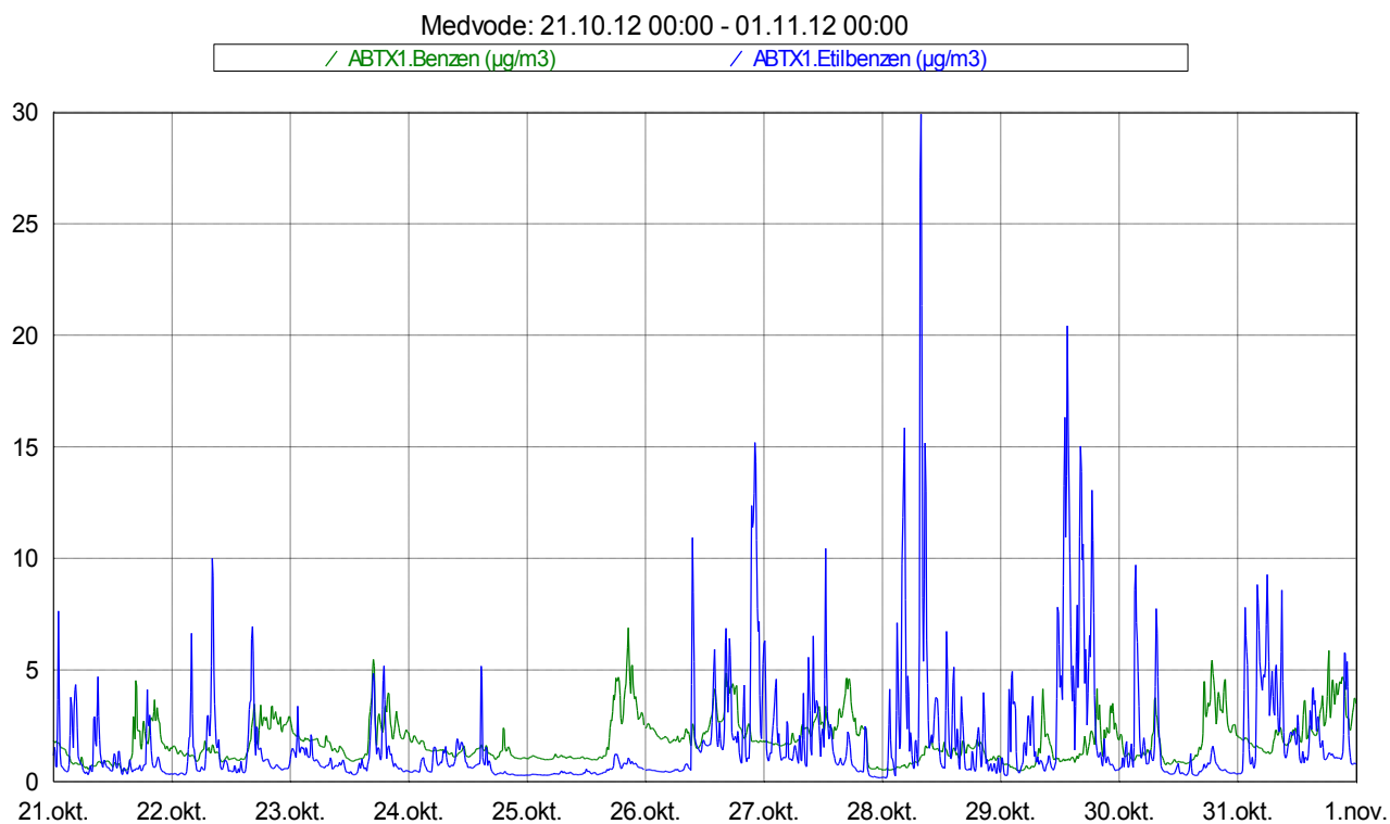
Slika 5: Imisijske koncentracije benzena in etilbenzena med 21. 10. 2012 in 31. 10. 2012.
