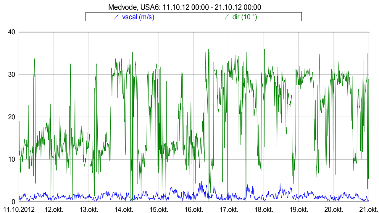
Slika 16: Smer in hitrost vetra med 11. 10. 2012 in 21. 10. 2012.
