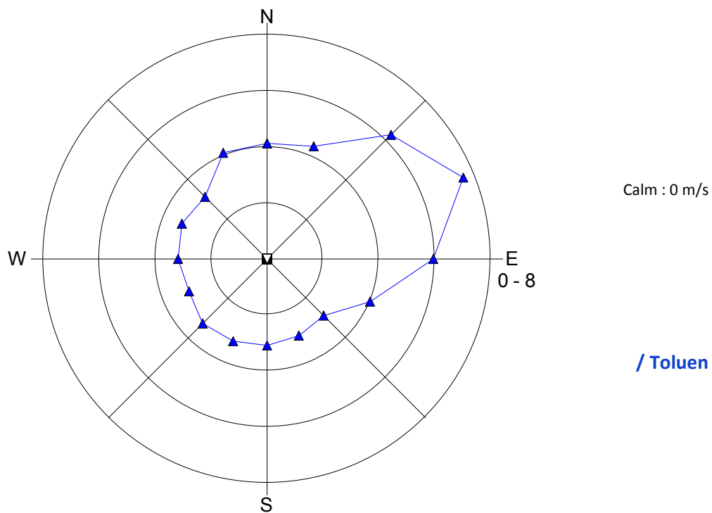
Slika 10: Roža onesnaženost - toluen, oktober 2012.
