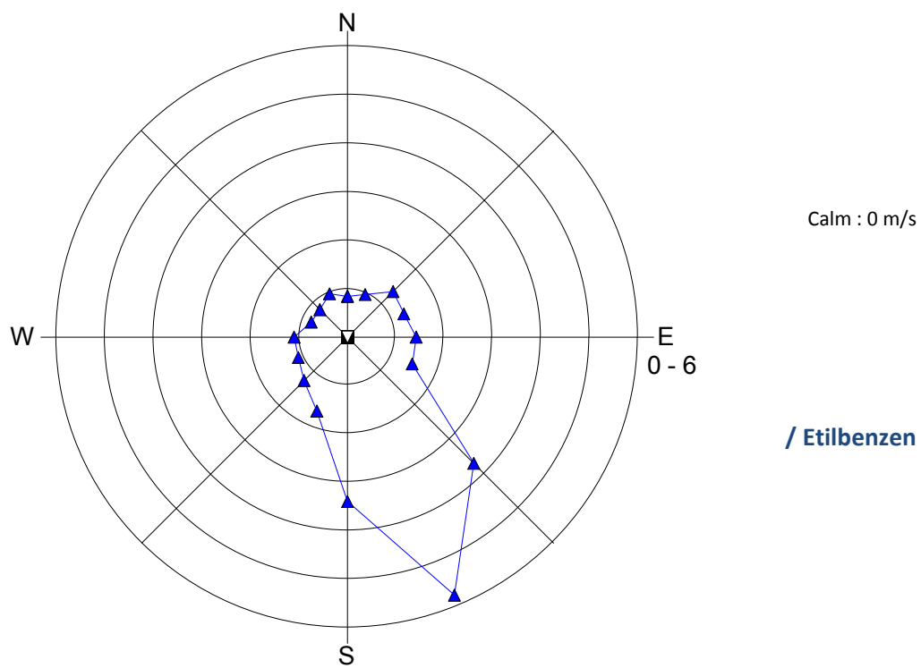
Slika 6: Roža onesnaženosti – benzen (zgoraj) in etilbenzen (spodaj), oktober 2012.
