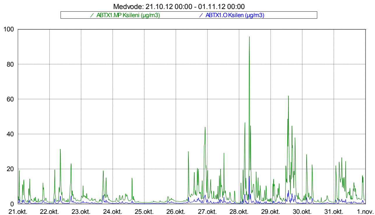
Slika 13: Imisijske koncentracije M&P in O ksilena med 21. 10. 2012 in 31. 10. 2012.
