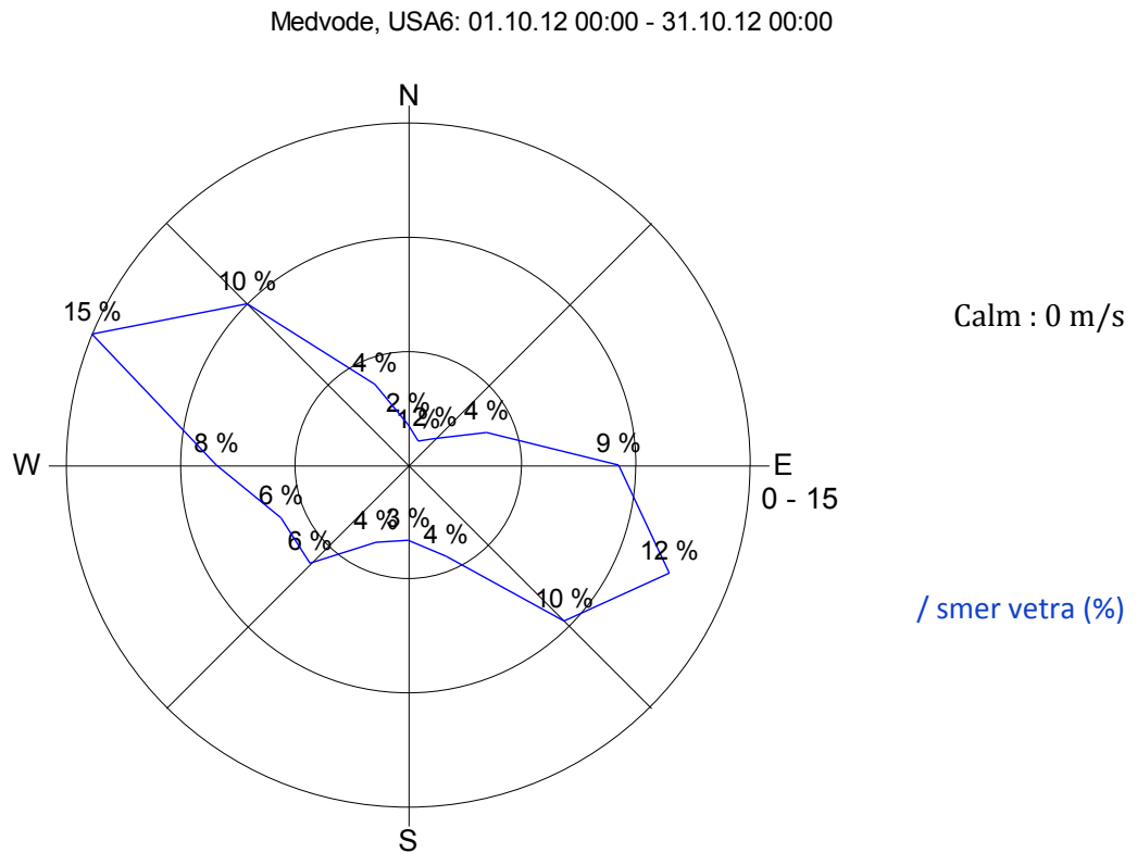
Slika 18: Roža vetrov, oktober 2012.
