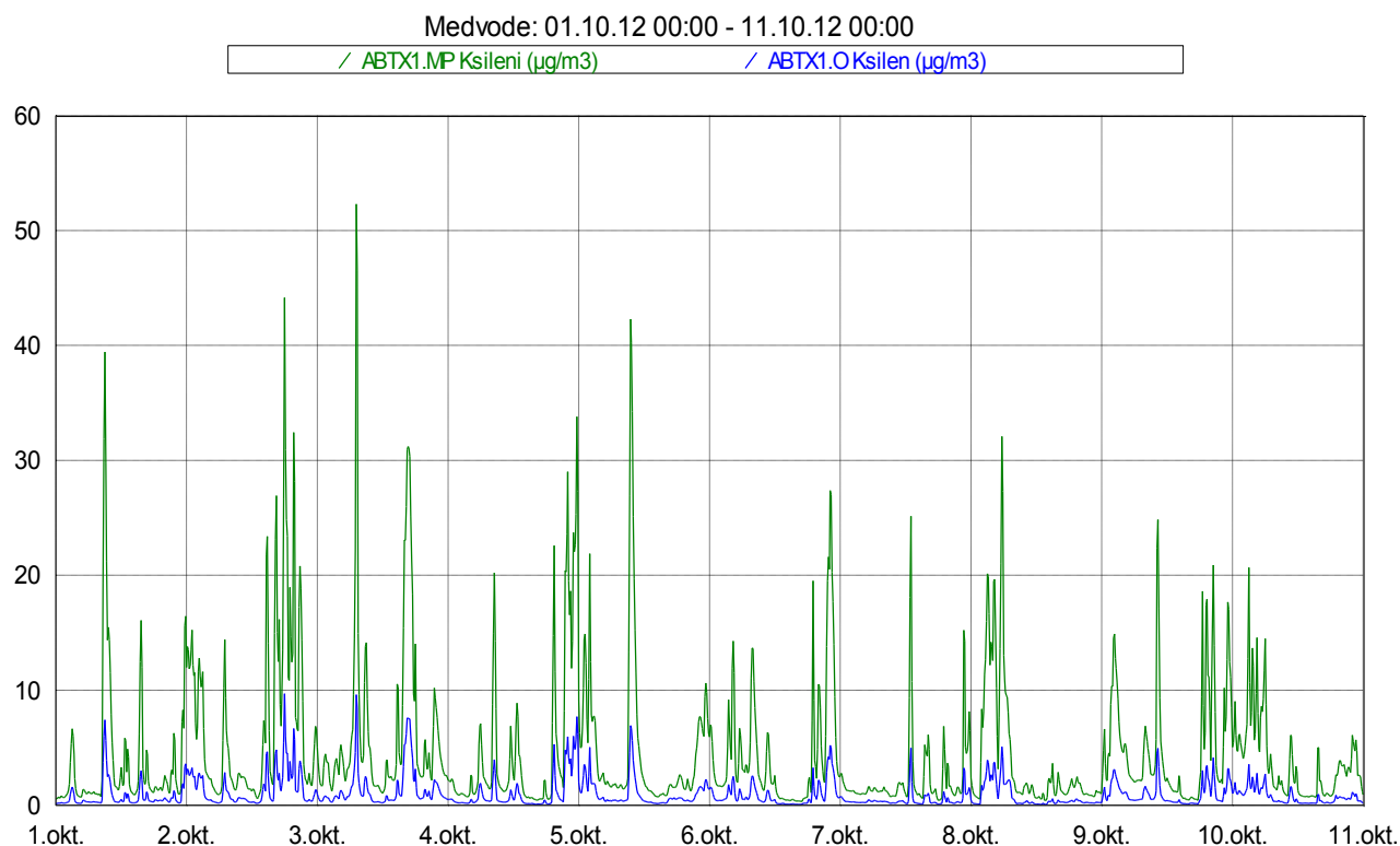
Slika 11: Imisijske koncentracije M&P in O ksilena med vključno 1. 10. 2012 in 11. 10. 2012.
