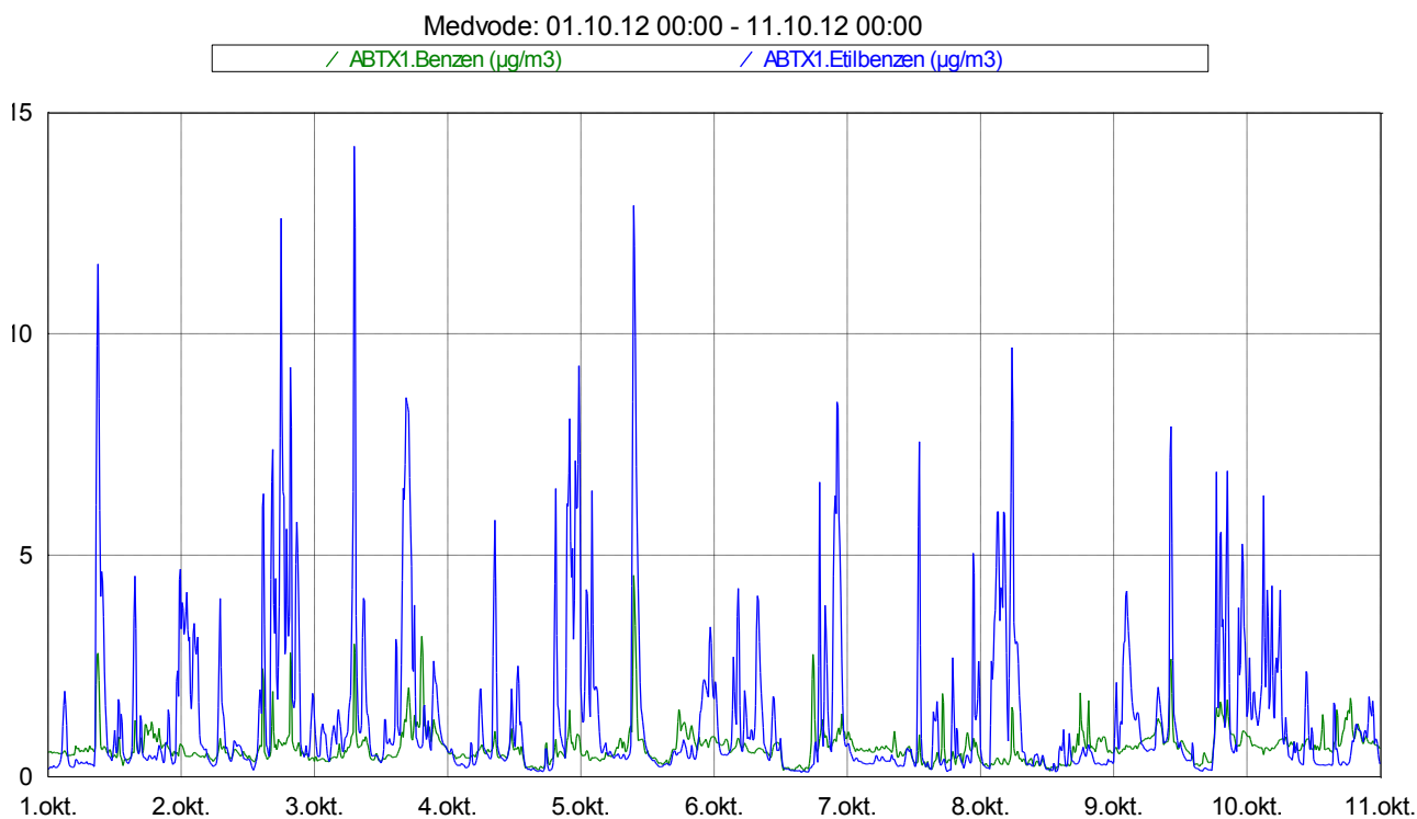
Slika 3: Imisijske koncentracije benzena in etilbenzena med vključno 1. 10. 2012 in 11. 10. 2012.
