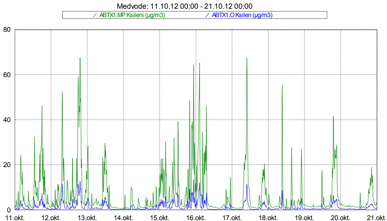
Slika 12: Imisijske koncentracije M&P in O ksilena med 11. 10. 2012 in 21. 10. 2012.
