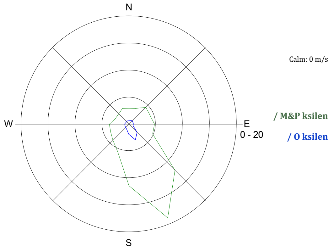
Slika 14: Roža onesnaženosti - M & P ksilen in O ksilen, oktober 2012.
