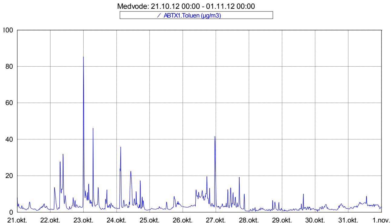
Slika 9: Imisijske koncentracije toluena med 21. 10. 2012 in 31. 10. 2012.
