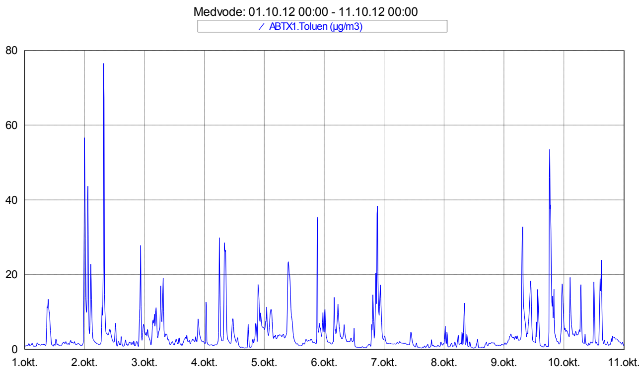
Slika 7: Imisijske koncentracije toluena med vključno 1. 10. 2012 in 11. 10. 2012.
