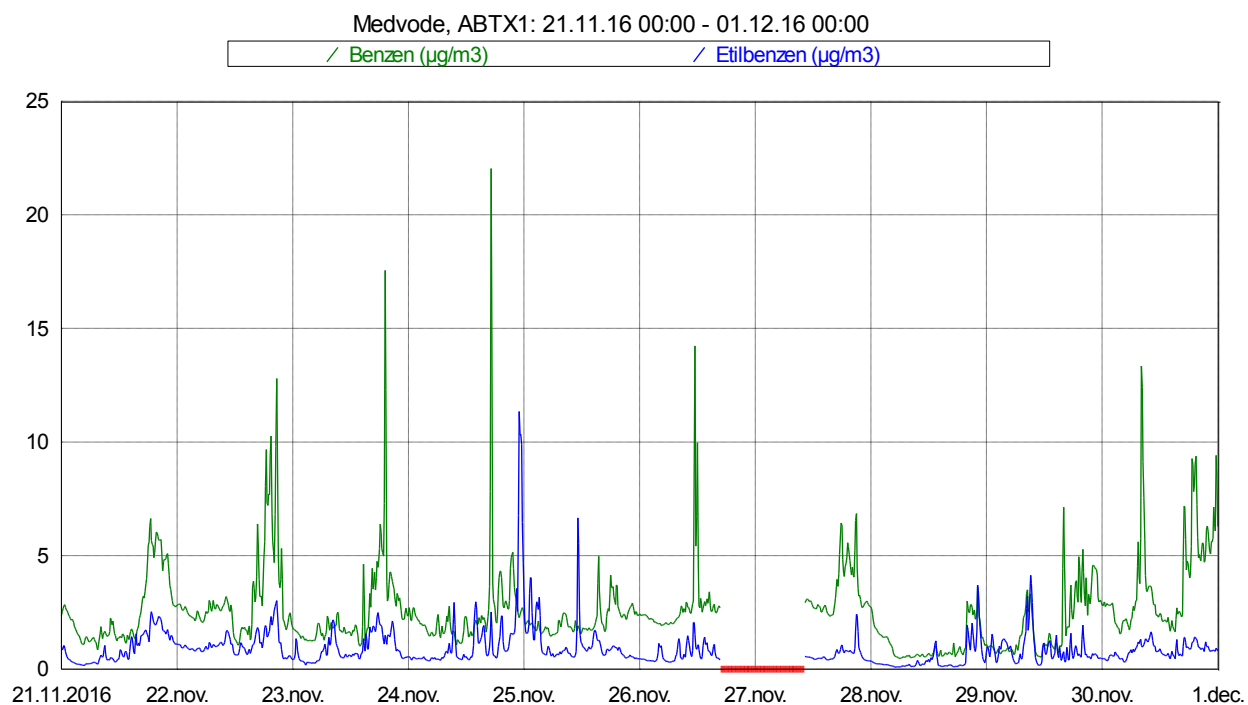
Slika 5: Imisijske koncentracije benzena in etilbenzena med 21. 11. 2016 in 30. 11. 2016.
