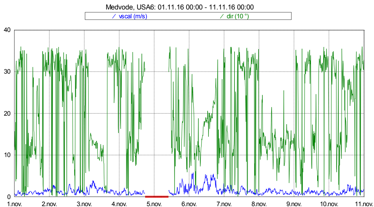
Slika 16: Smer in hitrost vetra med 1. 11. 2016 in 10. 11. 2016.
