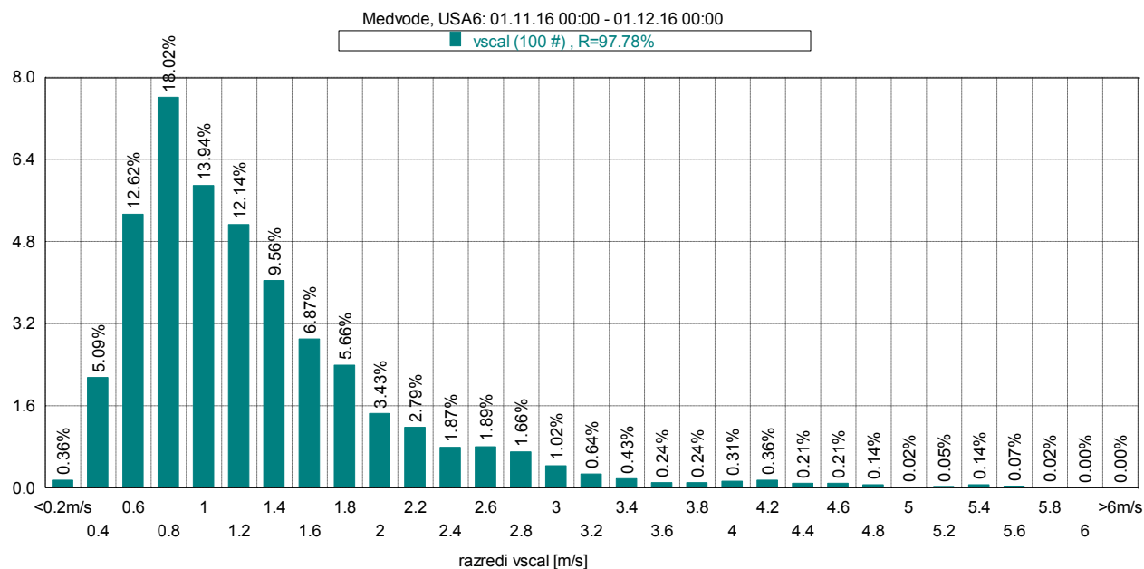
Slika 20: Frekvenčna porazdelitev po hitrosti vetra, november 2016.
