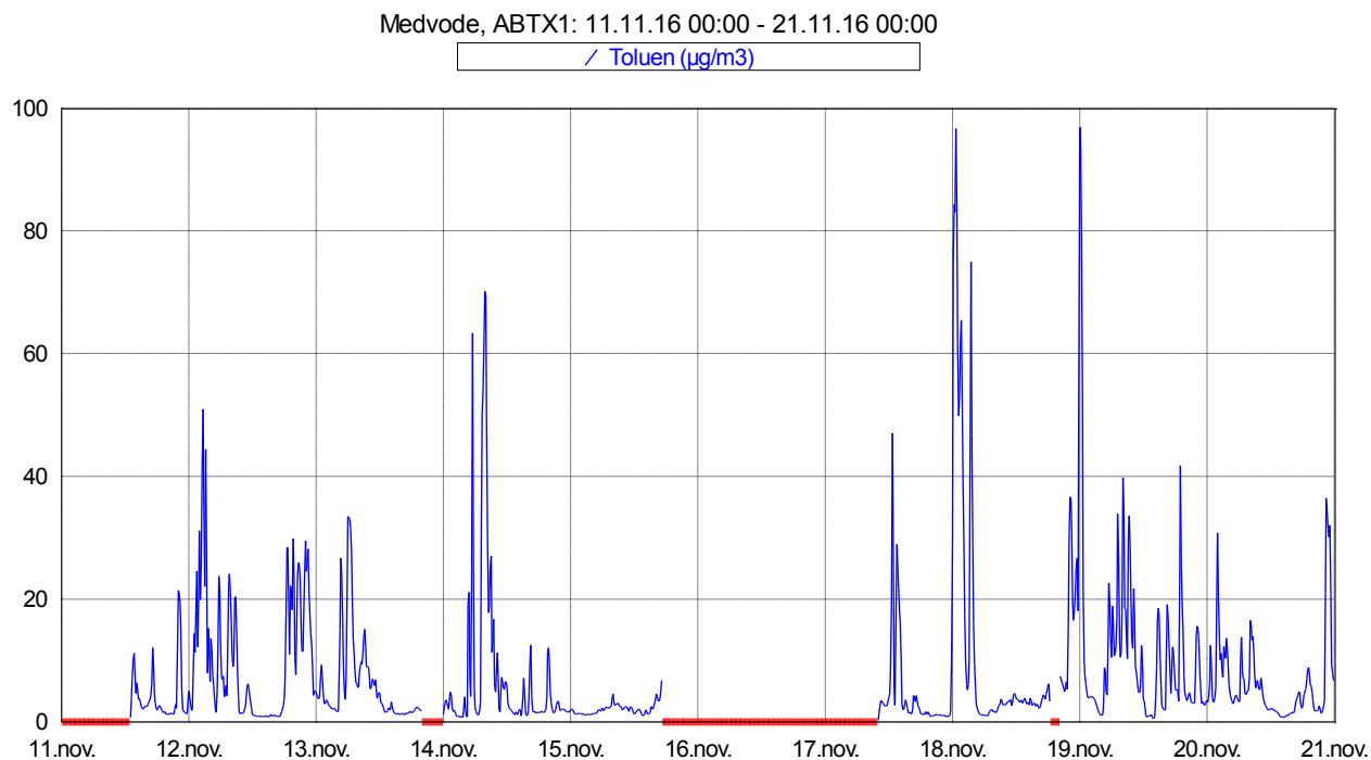
Slika 9: Imisijske koncentracije toluena med 11. 11. 2016 in 20. 11. 2016.
