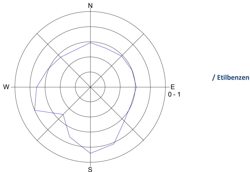
Slika 7: Roža onesnaženosti – etilbenzen, november 2016.
