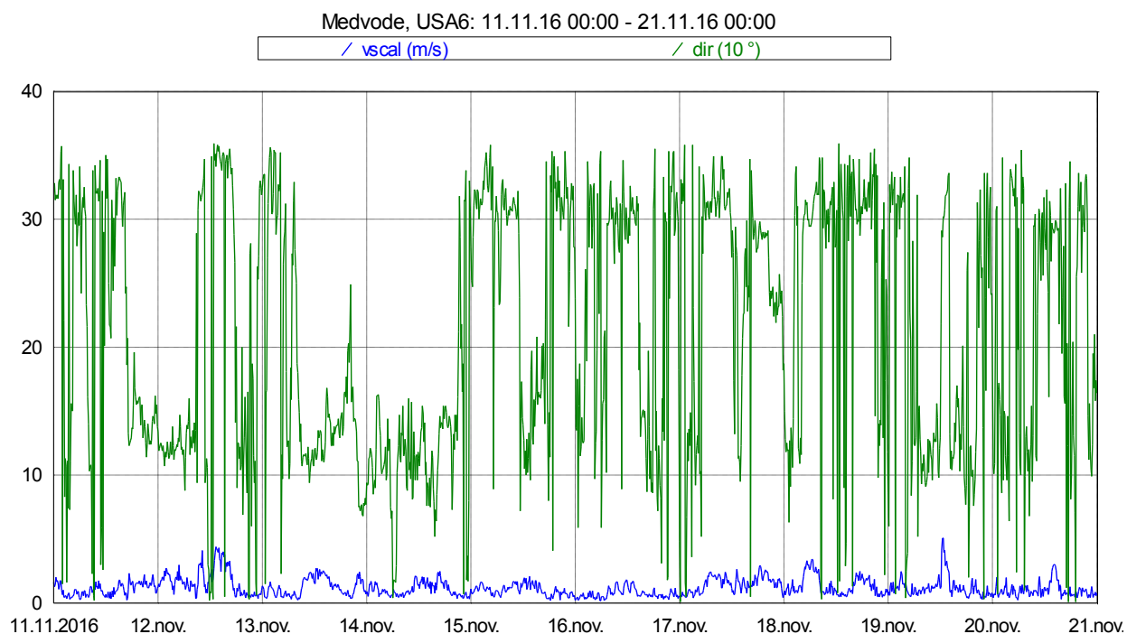
Slika 17: Smer in hitrost vetra med 11. 11. 2016 in 20. 11. 2016.
