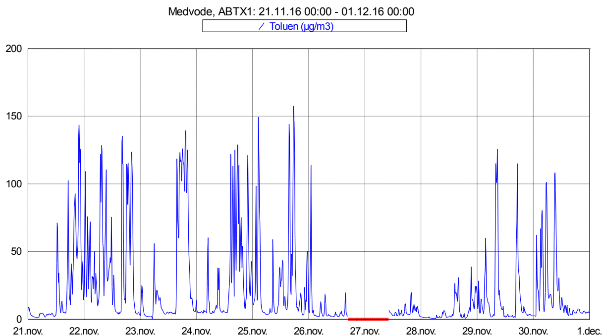
Slika 10: Imisijske koncentracije toluea med 21. 11. 2016 in 30. 11. 2016.
