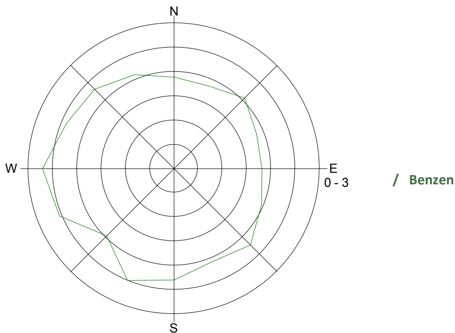
Slika 6: Roža onesnaženosti – benzen, november 2016.
