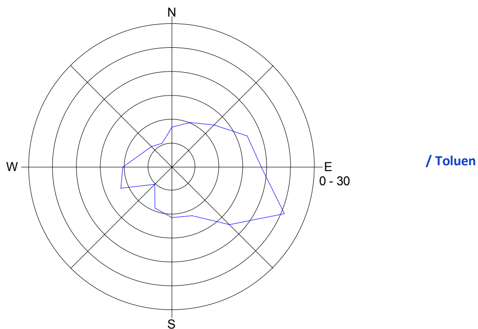
Slika 11: Roža onesnaženost - toluen, november 2016.
