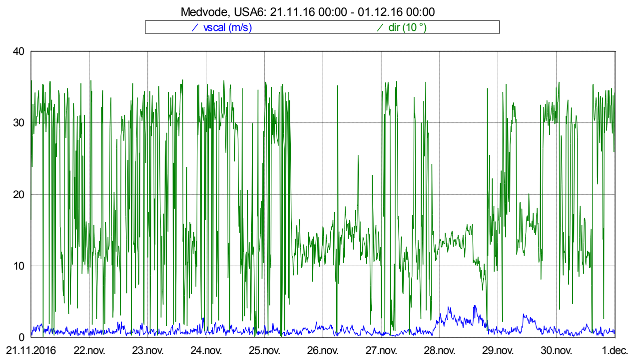
Slika 18: Smer in hitrost vetra med 21. 11. 2016 in 30. 11. 2016.
