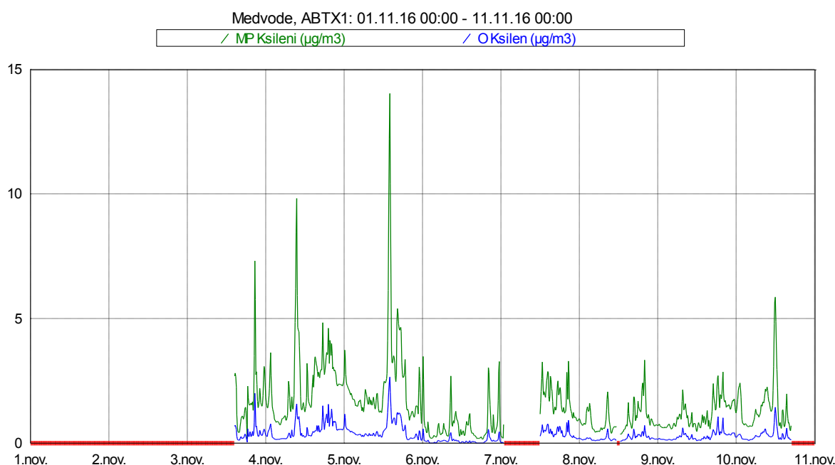
Slika 12: Imisijske koncentracije M&P in O ksilena med vključno 1. 11. 2016 in 10. 11. 2016.
