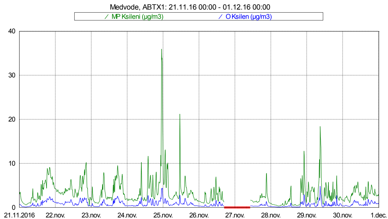
Slika 14: Imisijske koncentracije M&P in O ksilena med 21. 11. 2016 in 30. 11. 2016.
