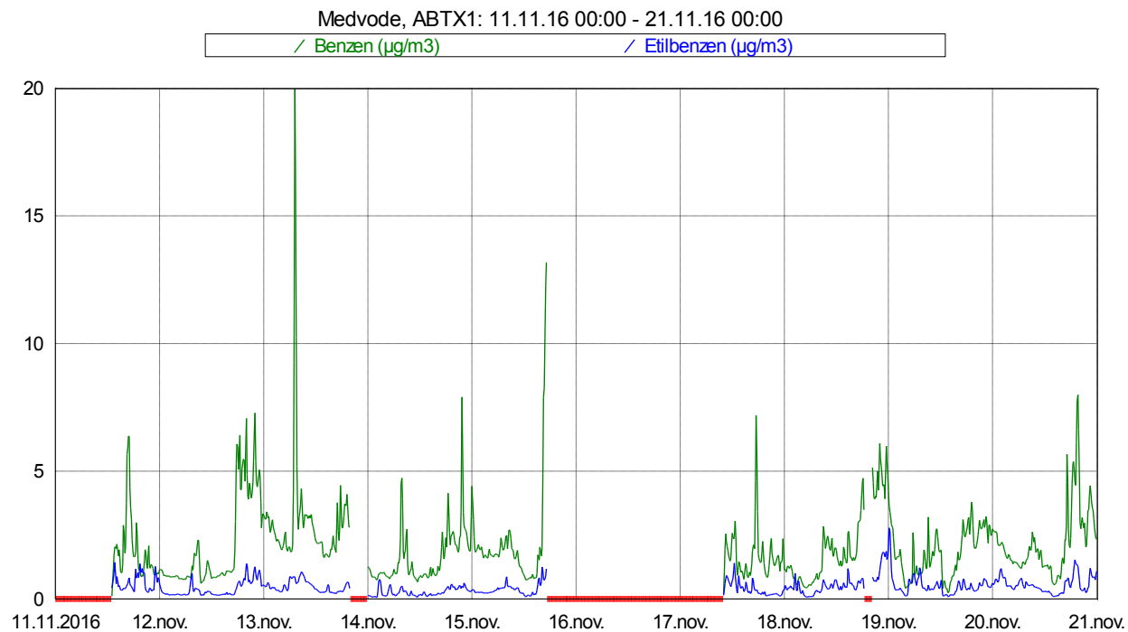
Slika 4: Imisijske koncentracije benzena in etilbenzena med 11. 11. 2016 in 20. 11. 2016.
