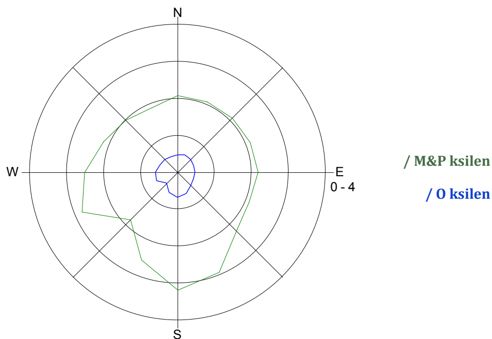
Slika 15: Roža onesnaženosti - M & P ksilen in O ksilen, november 2016.
