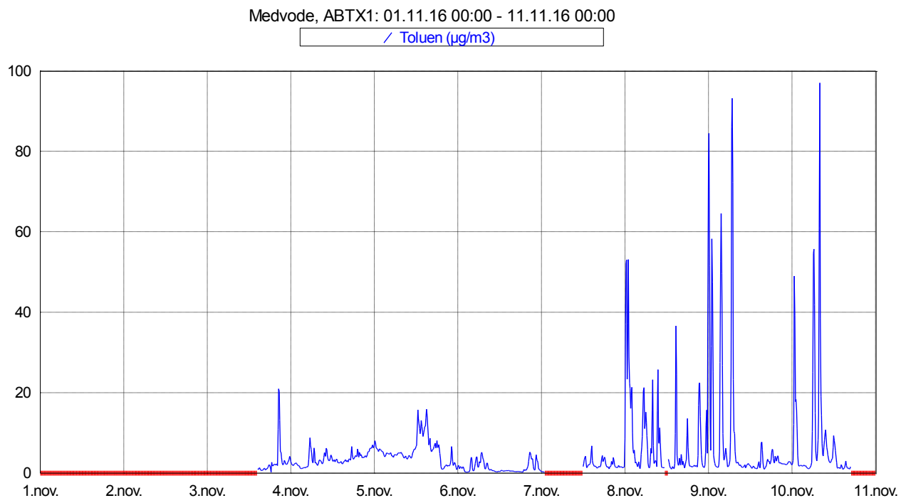
Slika 8: Imisijske koncentracije toluena med vključno 1. 11. 2016 in 10. 11. 2016.
