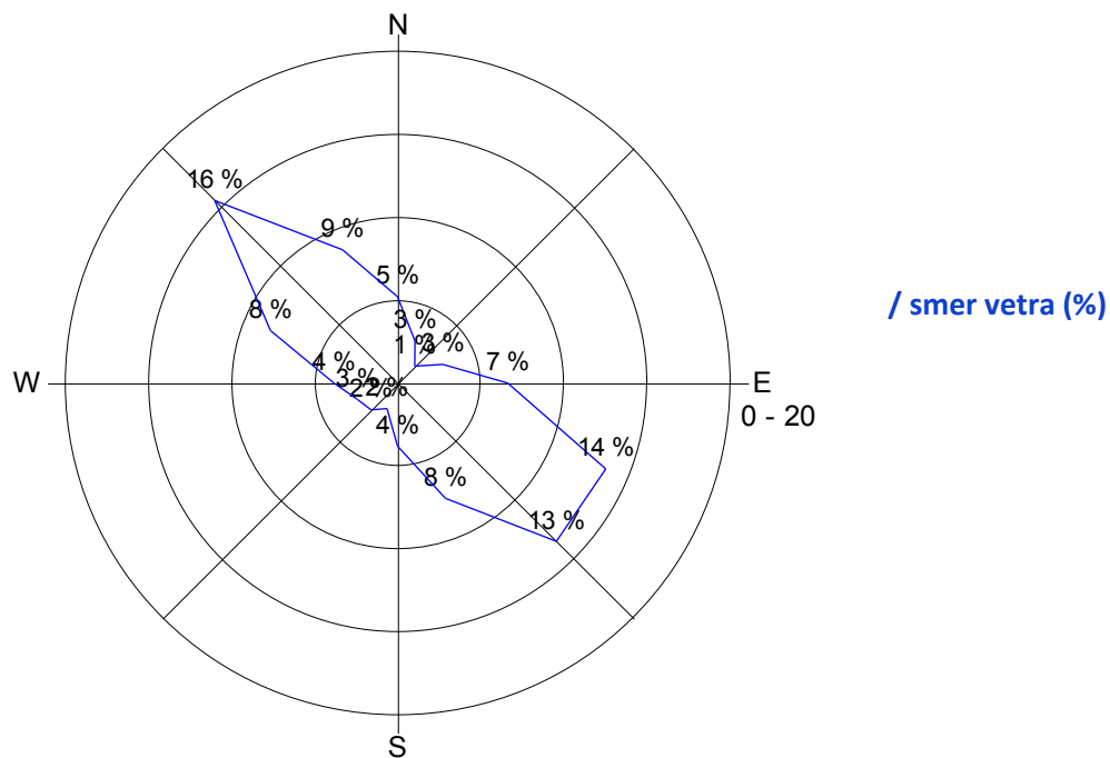
Slika 19: Roža vetrov, november 2016.
