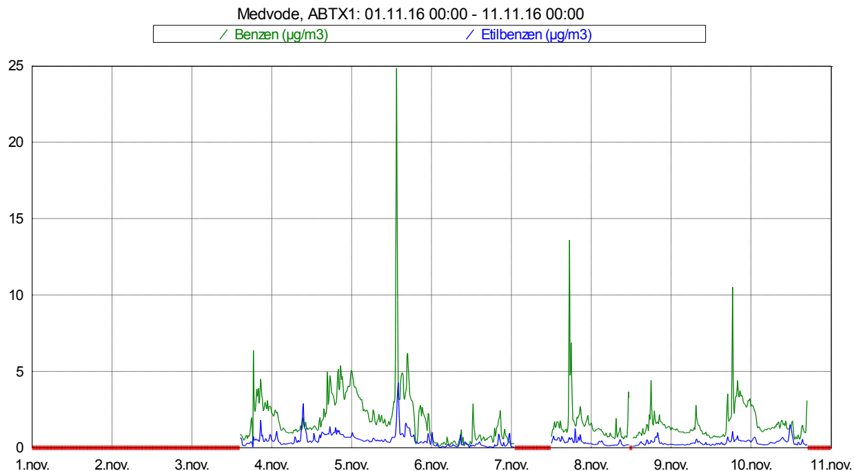
Slika 3: Imisijske koncentracije benzena in etilbenzena med vključno 1. 11. 2016 in 10. 11. 2016.
