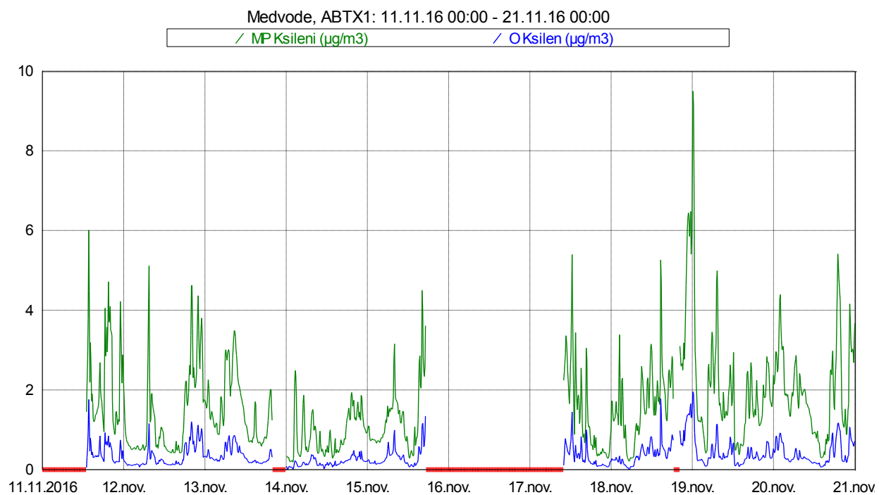
Slika 13: Imisijske koncentracije M&P in O ksilena med 11. 11. 2016 in 20. 11. 2016.
