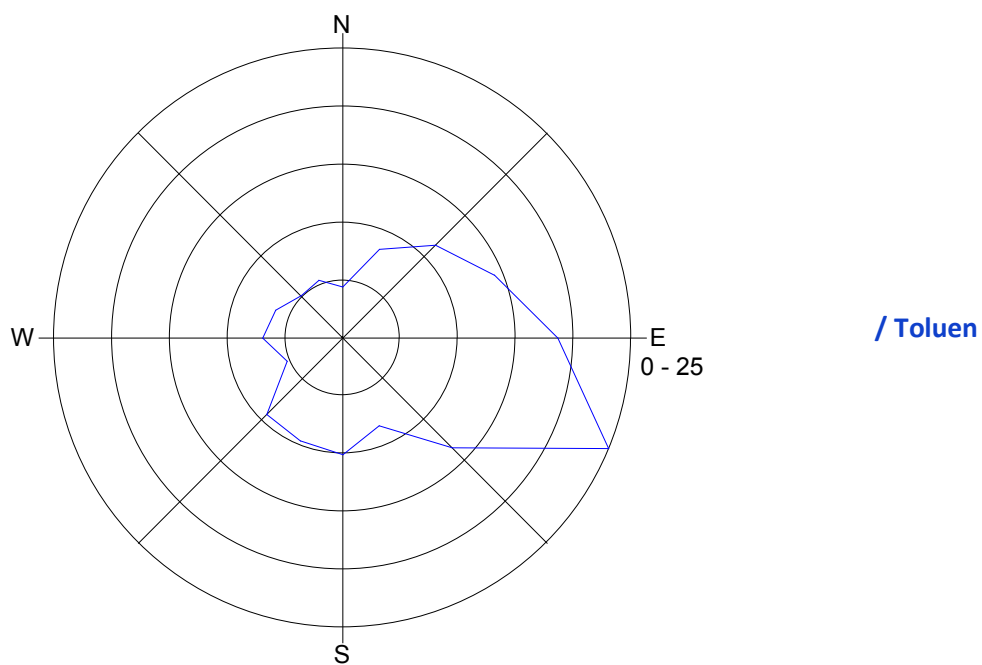
Slika 11: Roža onesnaženost - toluen, november 2015.
