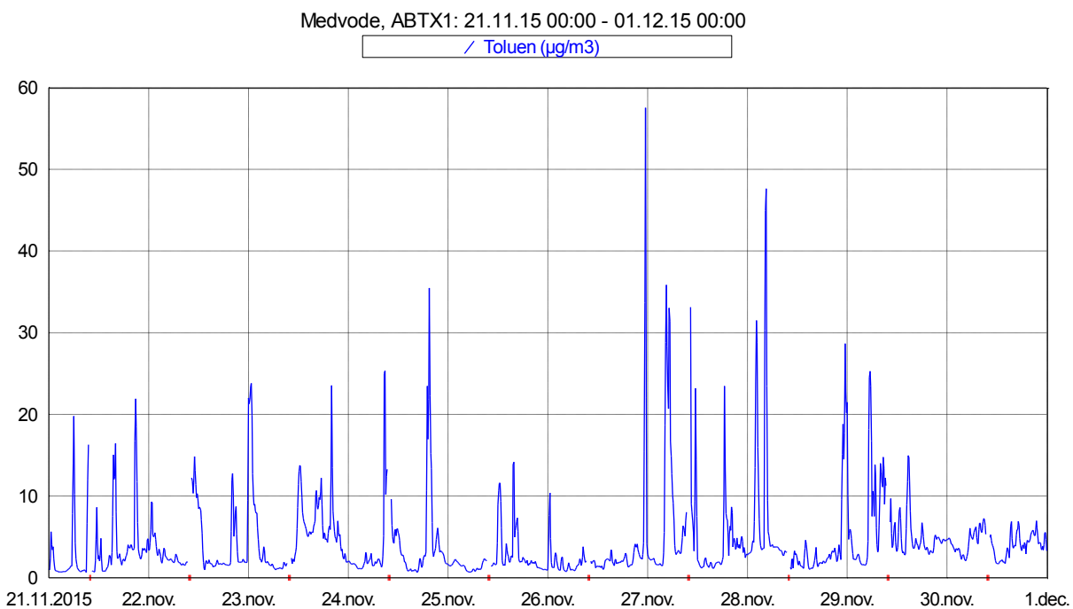
Slika 10: Imisijske koncentracije toluenta med 21. 11. 2015 in 30. 11. 2015.
