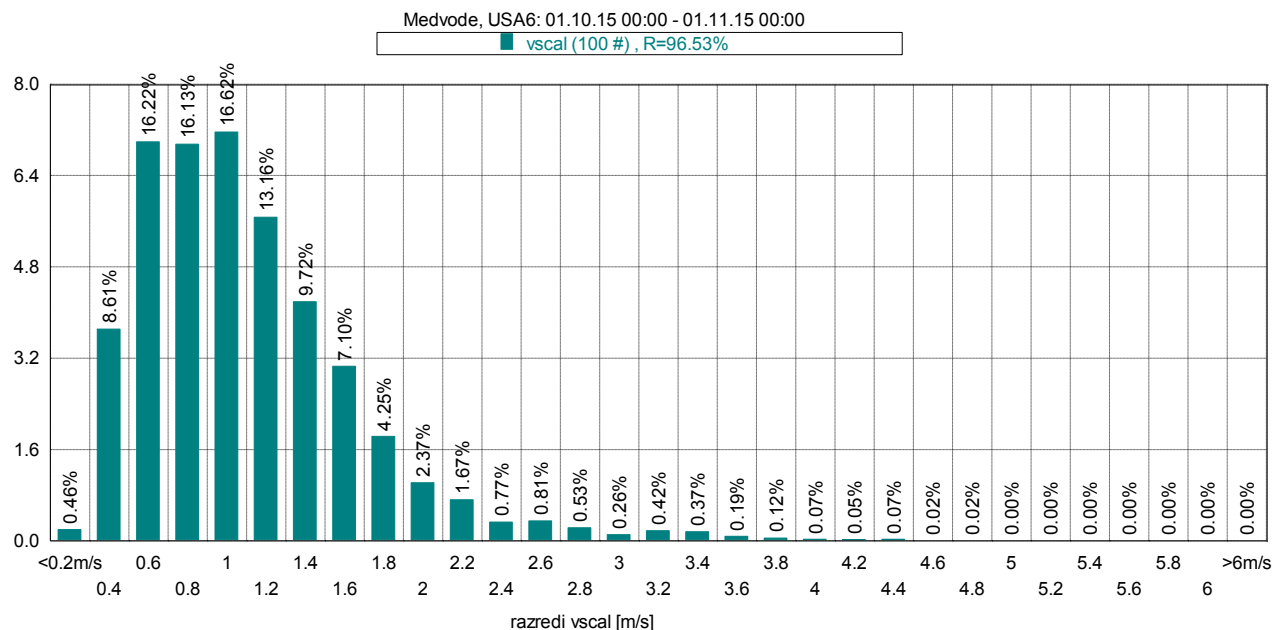
Slika 20: Frekvenčna porazdelitev po hitrosti vetra, november 2015.
