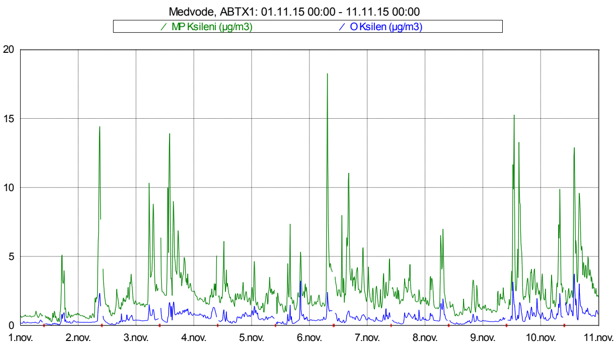
Slika 12: Imisijske koncentracije M&P in O ksilena med vključno 1. 11. 2015 in 10. 11. 2015.
