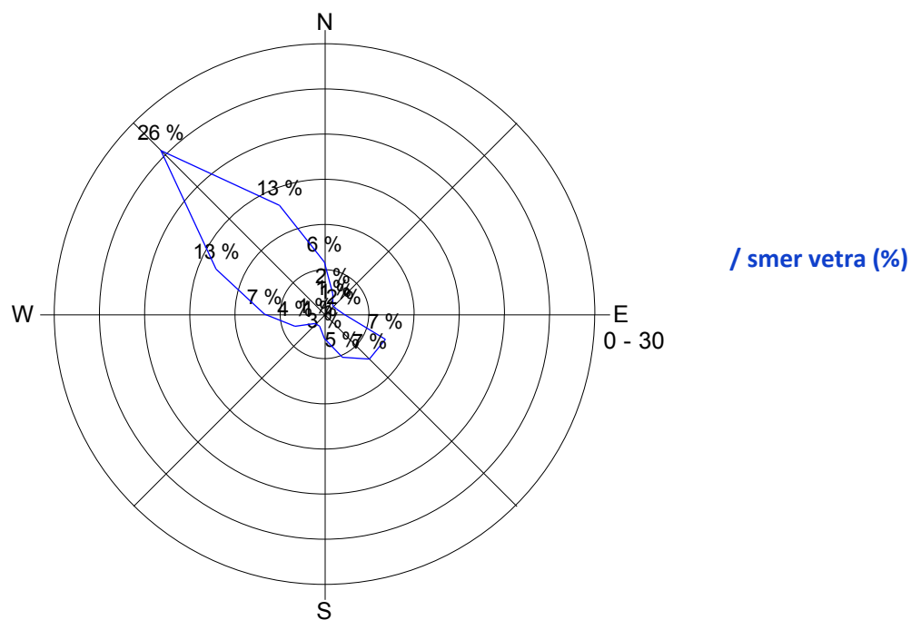
Slika 19: Roža vetrov, november 2015.
