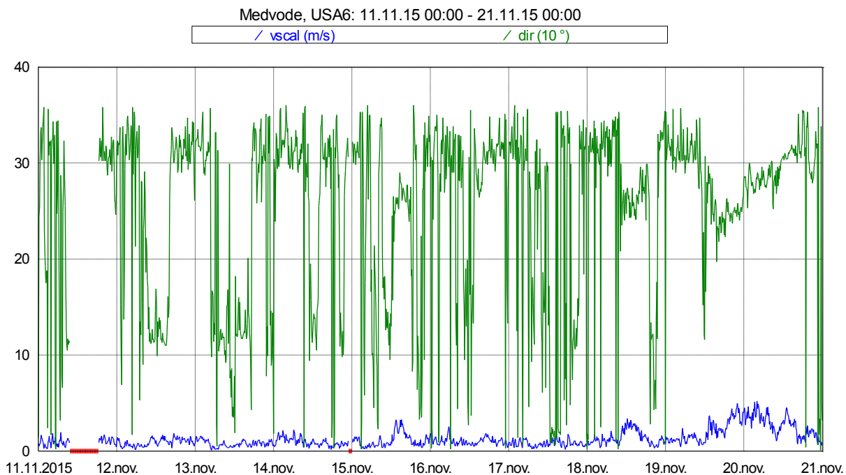
Slika 17: Smer in hitrost vetra med 11. 11. 2015 in 20. 11. 2015.
