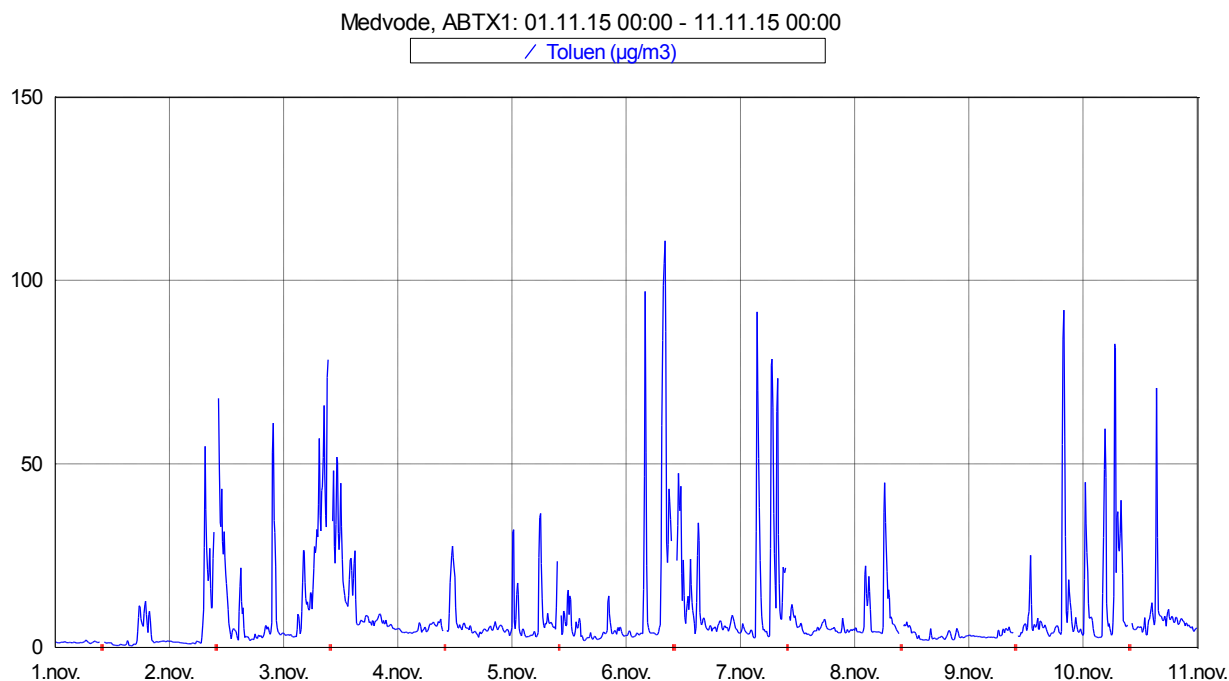
Slika 8: Imisijske koncentracije toluena med vključno 1. 11. 2015 in 10. 11. 2015.
