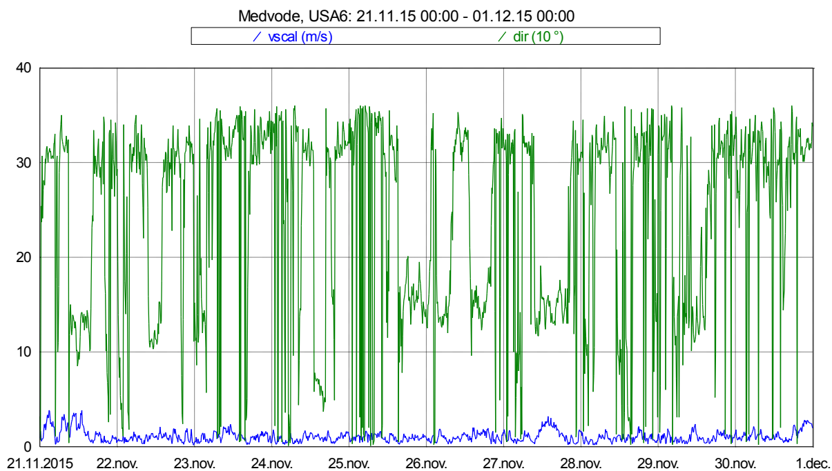
Slika 18: Smer in hitrost vetra med 21. 11. 2015 in 30. 11. 2015.
