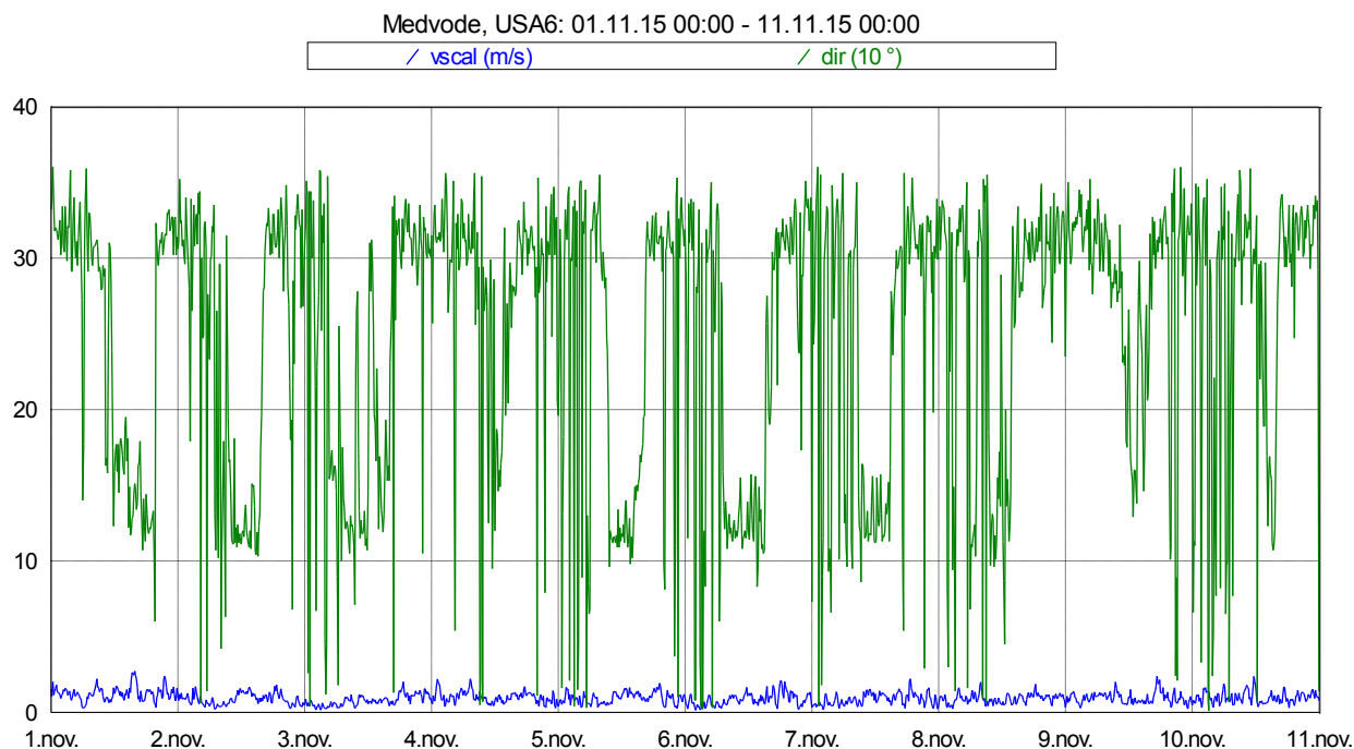
Slika 16: Smer in hitrost vetra med 1. 11. 2015 in 10. 11. 2015.
