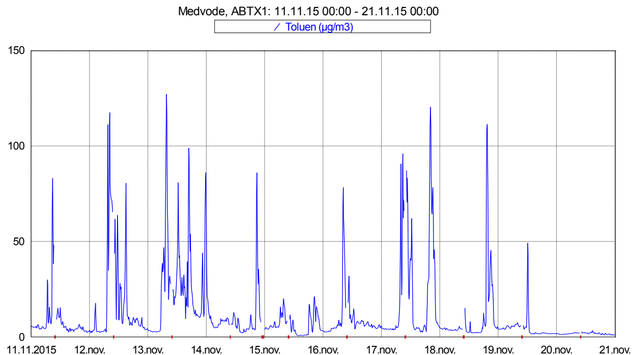
Slika 9: Imisijske koncentracije toluena med 11. 11. 2015 in 20. 11. 2015.
