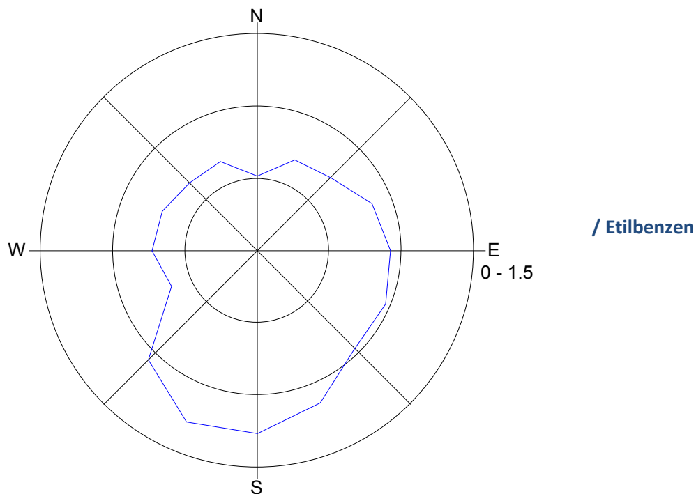
Slika 7: Roža onesnaženosti – etilbenzen, november 2015.
