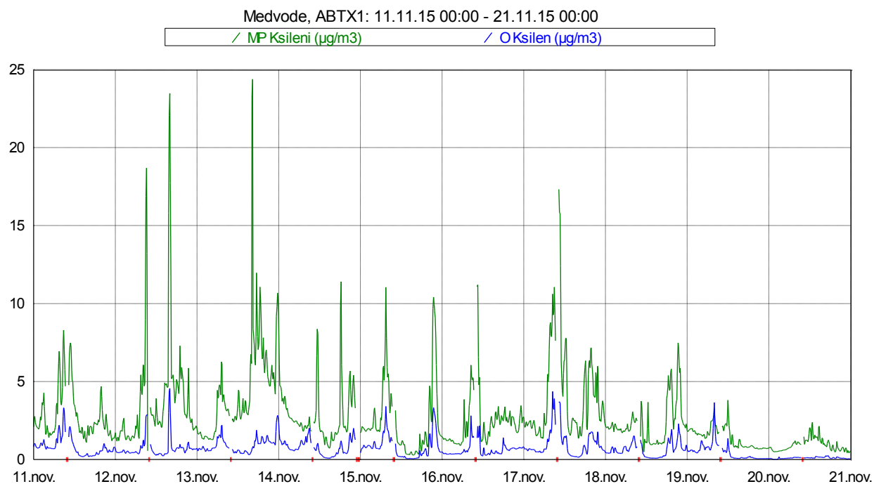
Slika 13: Imisijske koncentracije M&P in O ksilena med 11. 11. 2015 in 20. 11. 2015.
