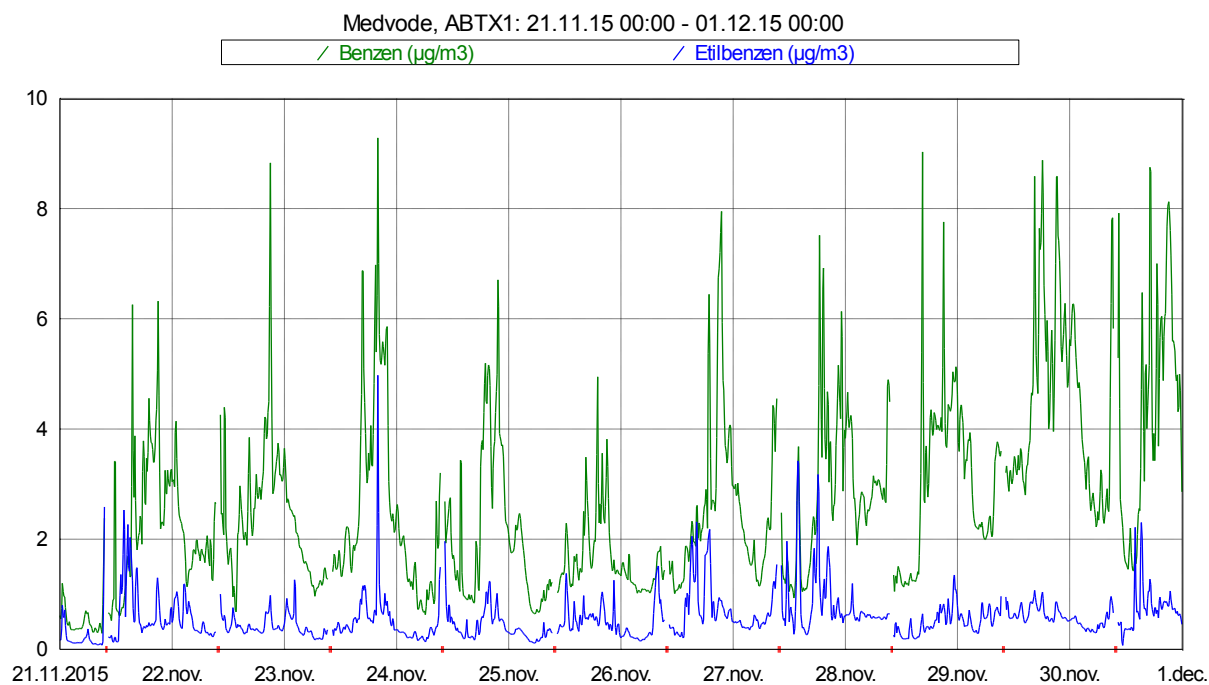
Slika 5: Imisijske koncentracije benzena in etilbenzena med 21. 11. 2015 in 30. 11. 2015.
