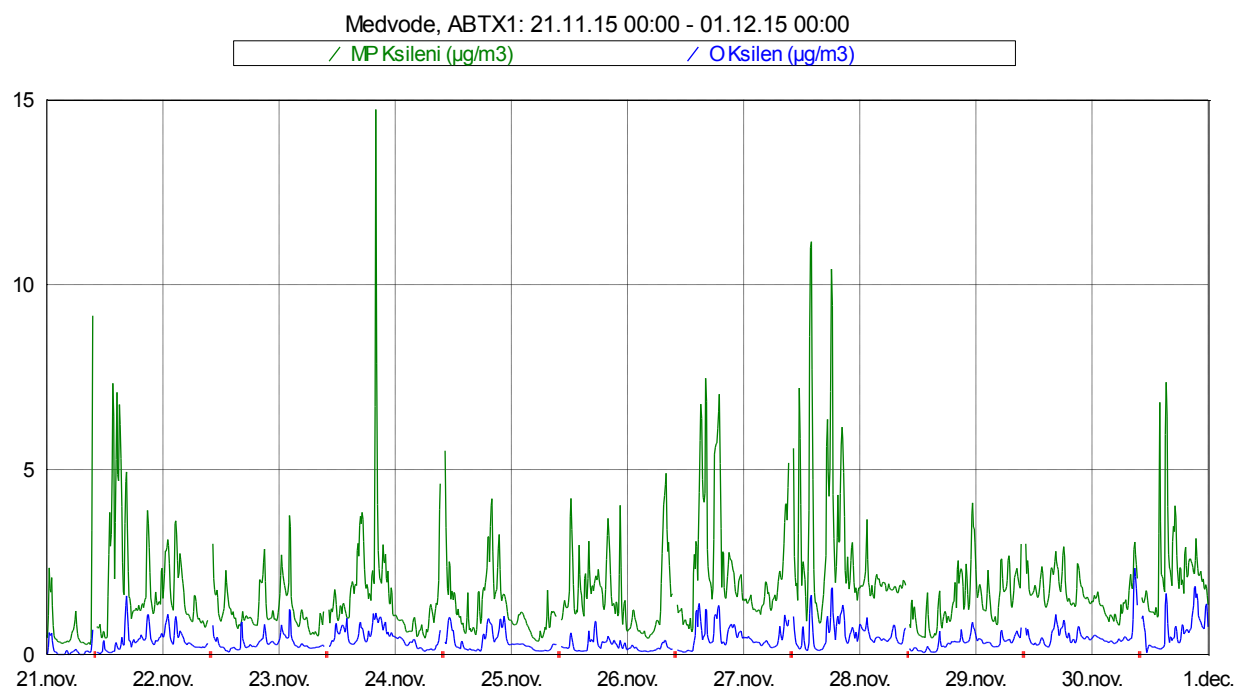
Slika 14: Imisijske koncentracije M&P in O ksilena med 21. 11. 2015 in 30. 11. 2015.
