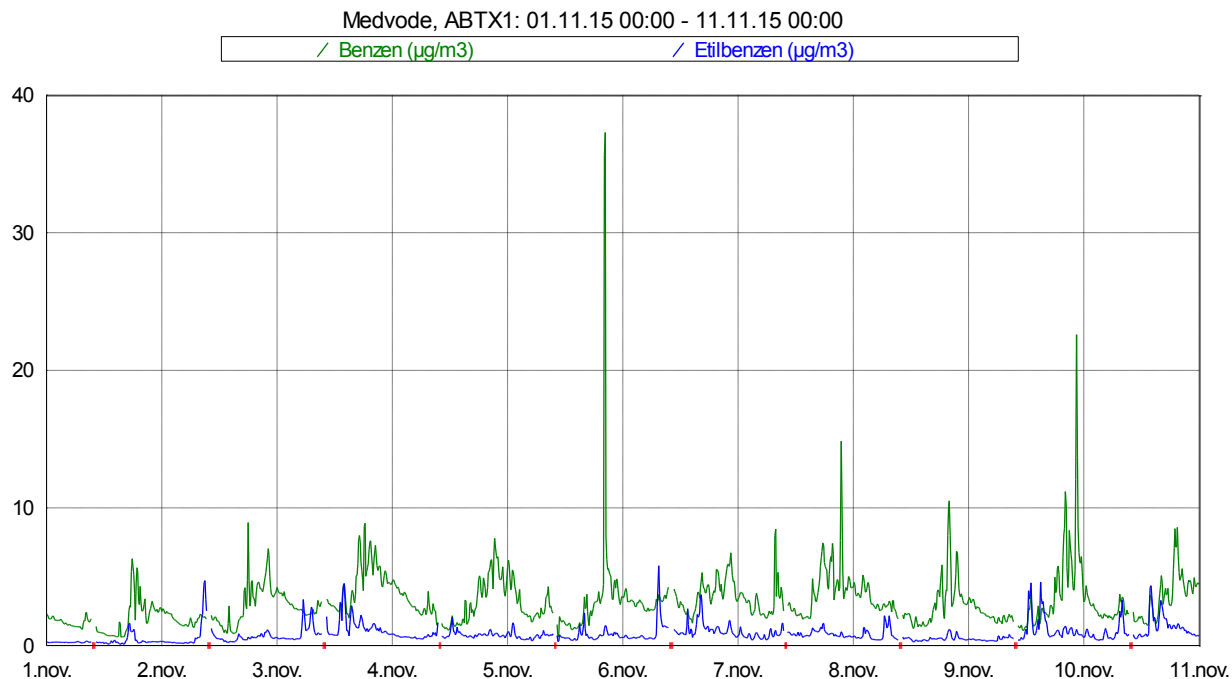
Slika 3: Imisijske koncentracije benzena in etilbenzena med vključno 1. 11. 2015 in 10. 11. 2015.
