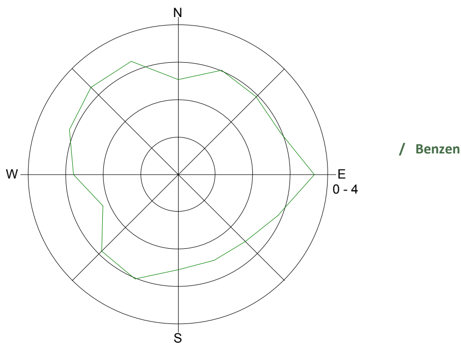
Slika 6: Roža onesnaženosti – benzen, november 2015.
