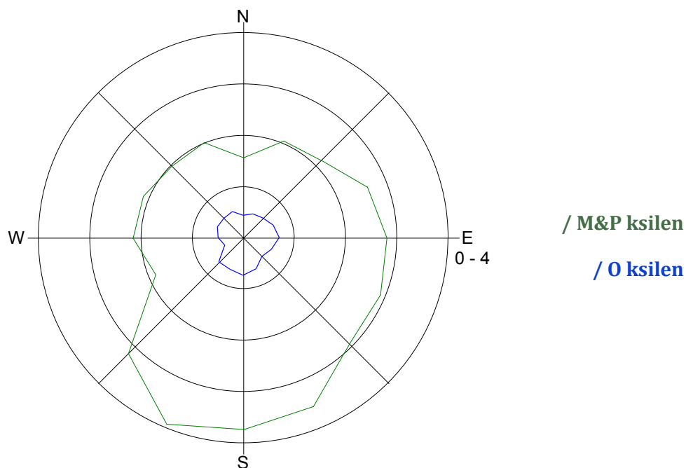
Slika 15: Roža onesnaženosti - M & P ksilen in O ksilen, november 2015.
