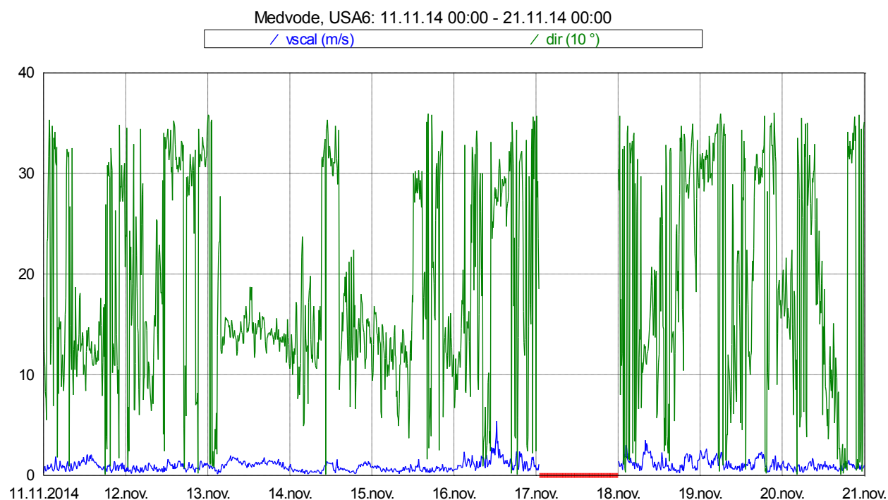
Slika 17: Smer in hitrost vetra med 11. 11. 2014 in 20. 11. 2014.
