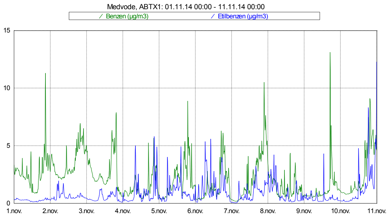
Slika 3: Imisijske koncentracije benzena in etilbenzena med vključno 1. 11. 2014 in 10. 11. 2014.
