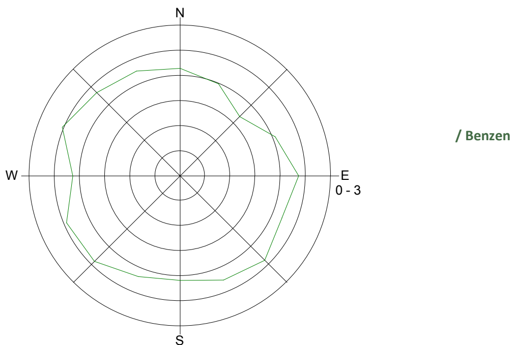
Slika 6: Roža onesnaženosti – benzen, november 2014.
