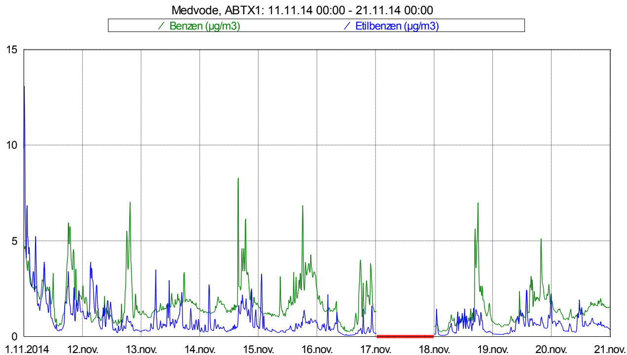
Slika 4: Imisijske koncentracije benzena in etilbenzena med 11. 11. 2014 in 20. 11. 2014.
