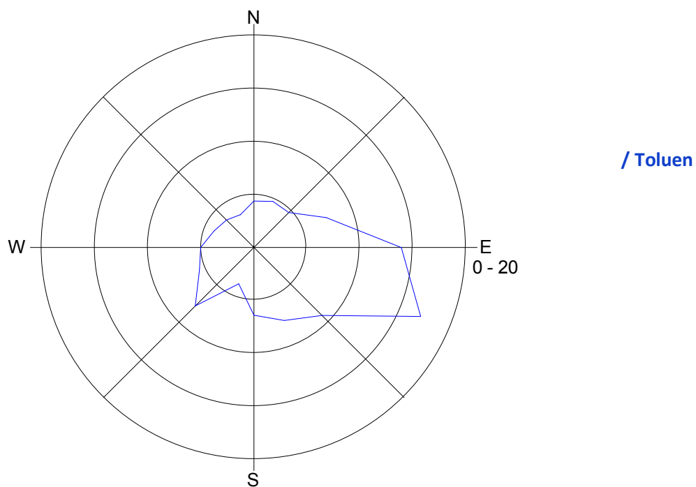
Slika 11: Roža onesnaženost - toluen, november 2014.
