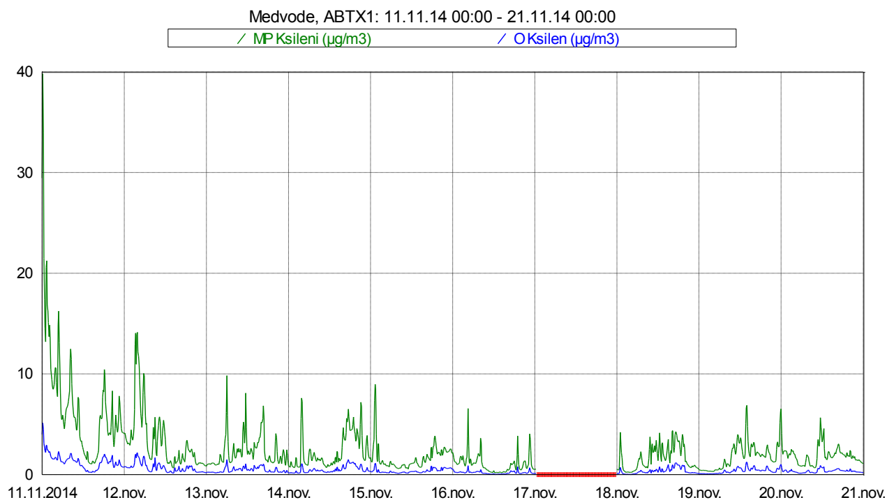
Slika 13: Imisijske koncentracije M&P in O ksilena med 11. 11. 2014 in 20. 11. 2014.
