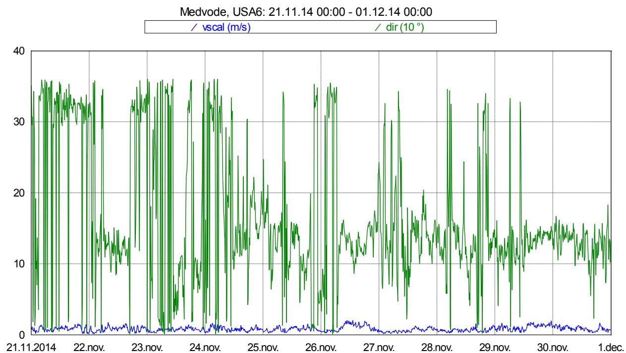
Slika 18: Smer in hitrost vetra med 21. 11. 2014 in 31. 11. 2014.
