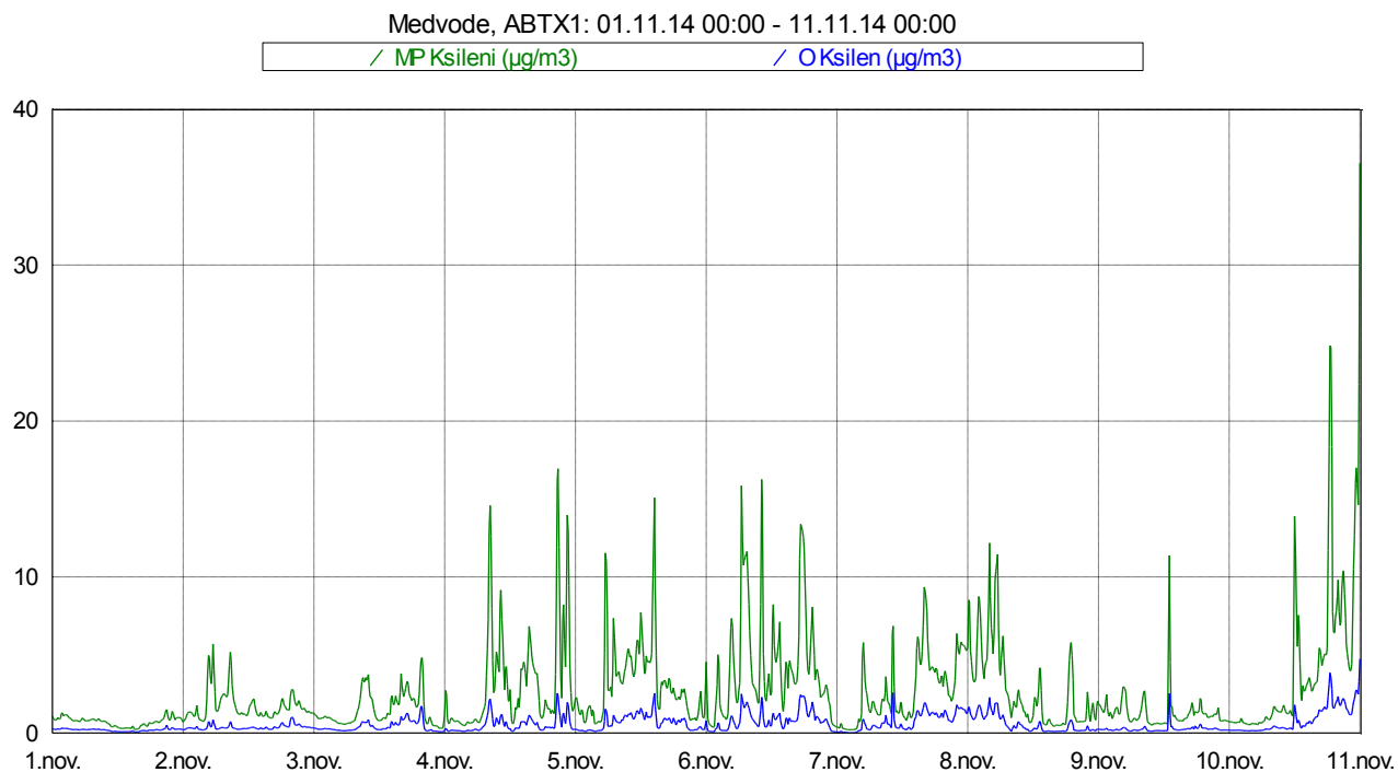
Slika 12: Imisijske koncentracije M&P in O ksilena med vključno 1. 11. 2014 in 10. 11. 2014.
