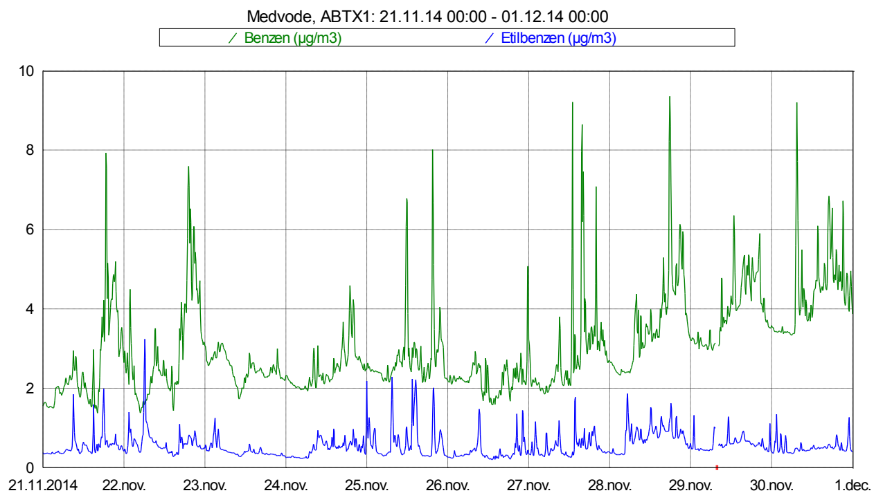
Slika 5: Imisijske koncentracije benzena in etilbenzena med 21. 11. 2014 in 31. 11. 2014.
