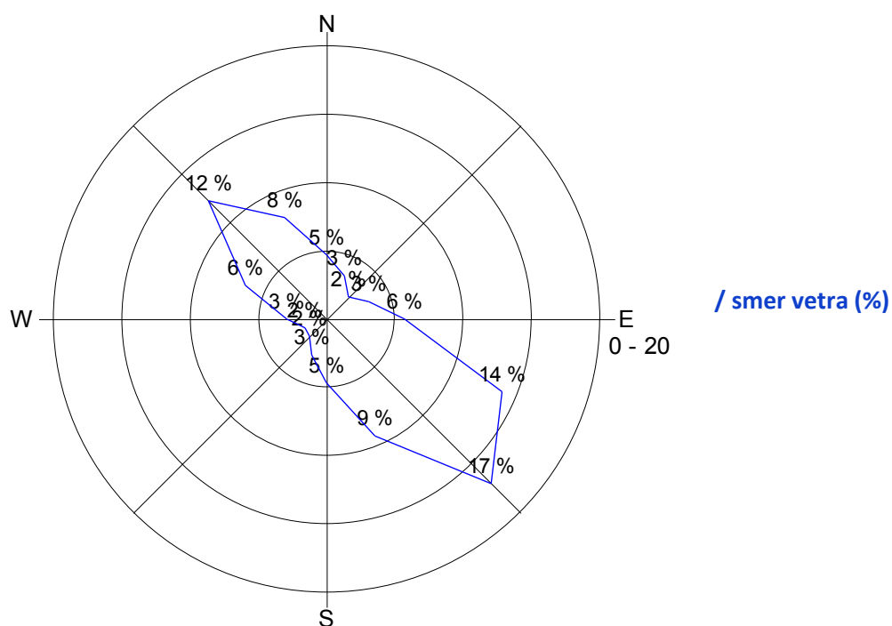
Slika 18: Smer in hitrost vetra med 21. 11. 2014 in 31. 11. 2014.
