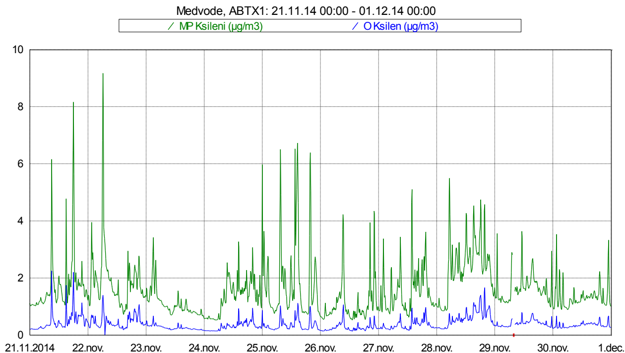
Slika 14: Imisijske koncentracije M&P in O ksilena med 21. 11. 2014 in 30. 11. 2014.
