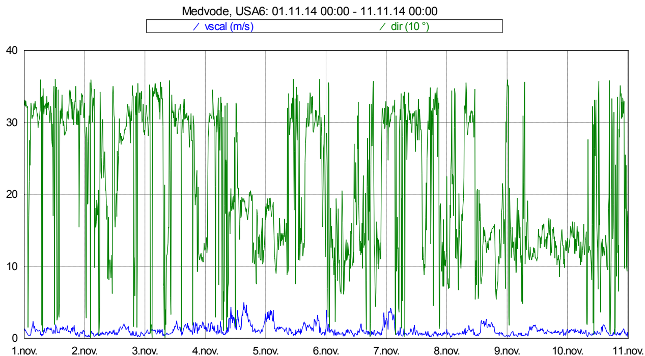
Slika 16: Smer in hitrost vetra med 1. 11. 2014 in 10. 11. 2014.
