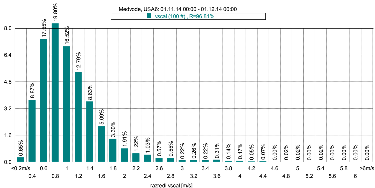
Slika 20: Frekvenčna porazdelitev po hitrosti vetra, november 2014.
