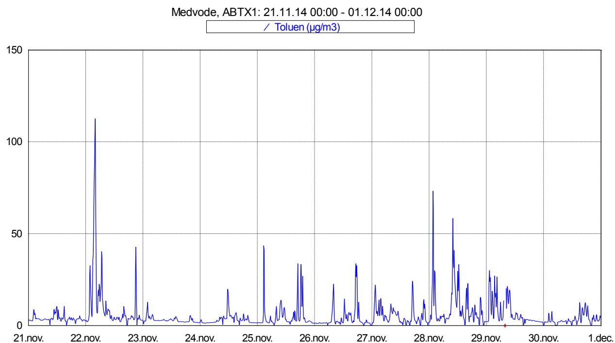
Slika 10: Imisijske koncentracije tolueuna med 21. 11. 2014 in 30. 11. 2014.
