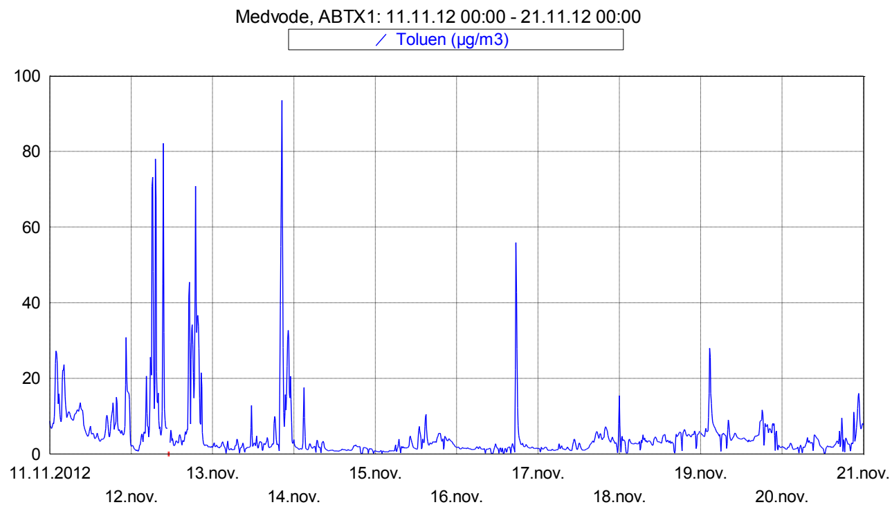
Slika 8: Imisijske koncentracije toluena med 11. 11. 2012 in 20. 11. 2012.
