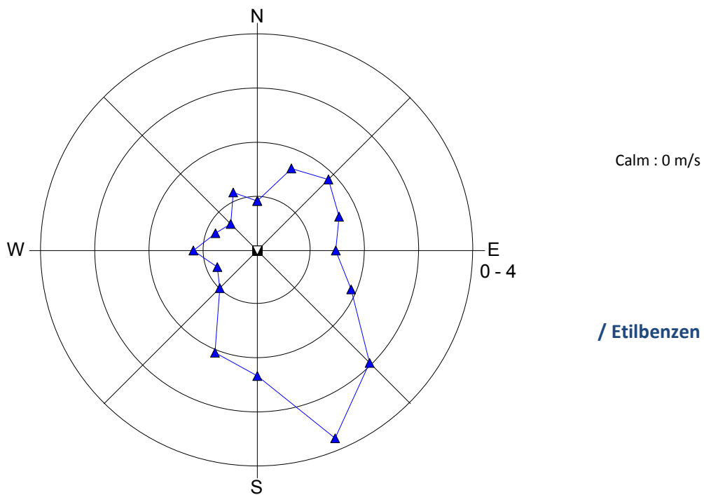
Slika 6: Roža onesnaženosti – benzen (zgoraj) in etilbenzen (spodaj), november 2012.
