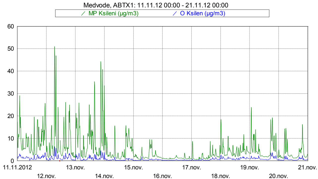
Slika 12: Imisijske koncentracije M&P in O ksilena med 11. 11. 2012 in 20. 11. 2012.
