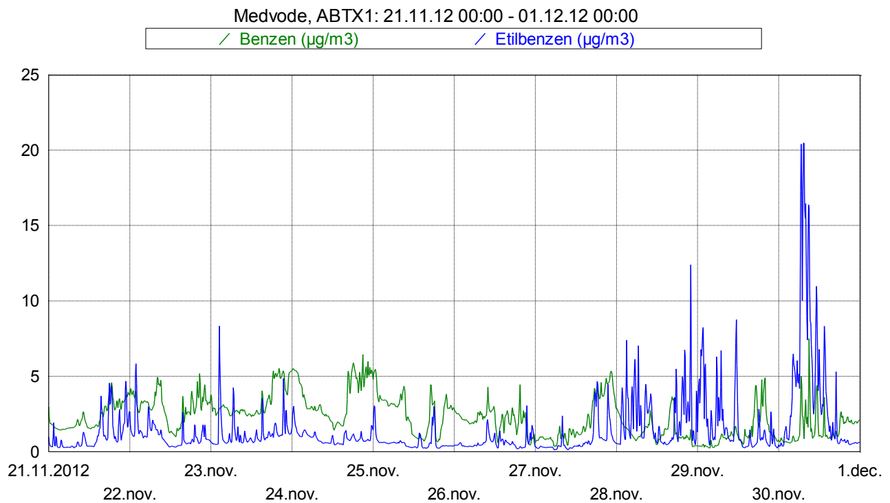
Slika 5: Imisijske koncentracije benzena in etilbenzena med 21. 11. 2012 in 30. 11. 2012.
