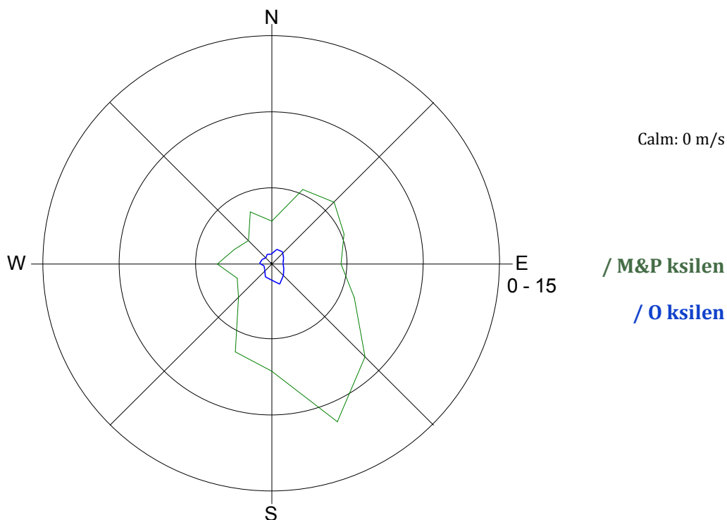
Slika 14: Roža onesnaženosti - M & P ksilen in O ksilen, november 2012.
