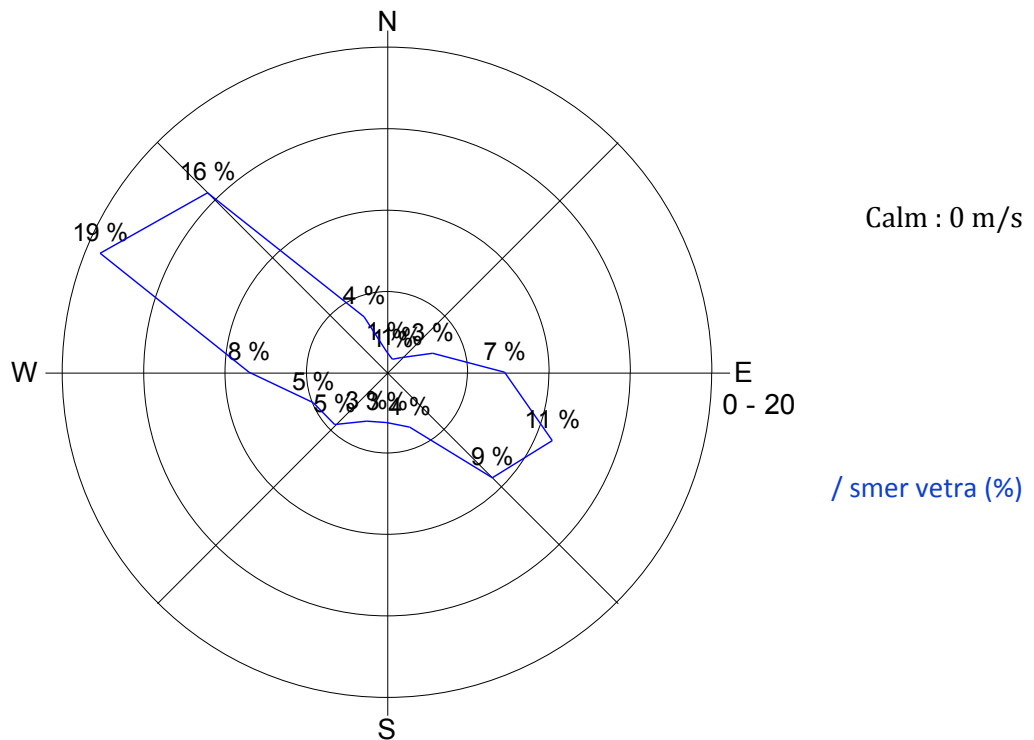
Slika 17: Smer in hitrost vetra med 21. 11. 2012 in 30. 11. 2012.
