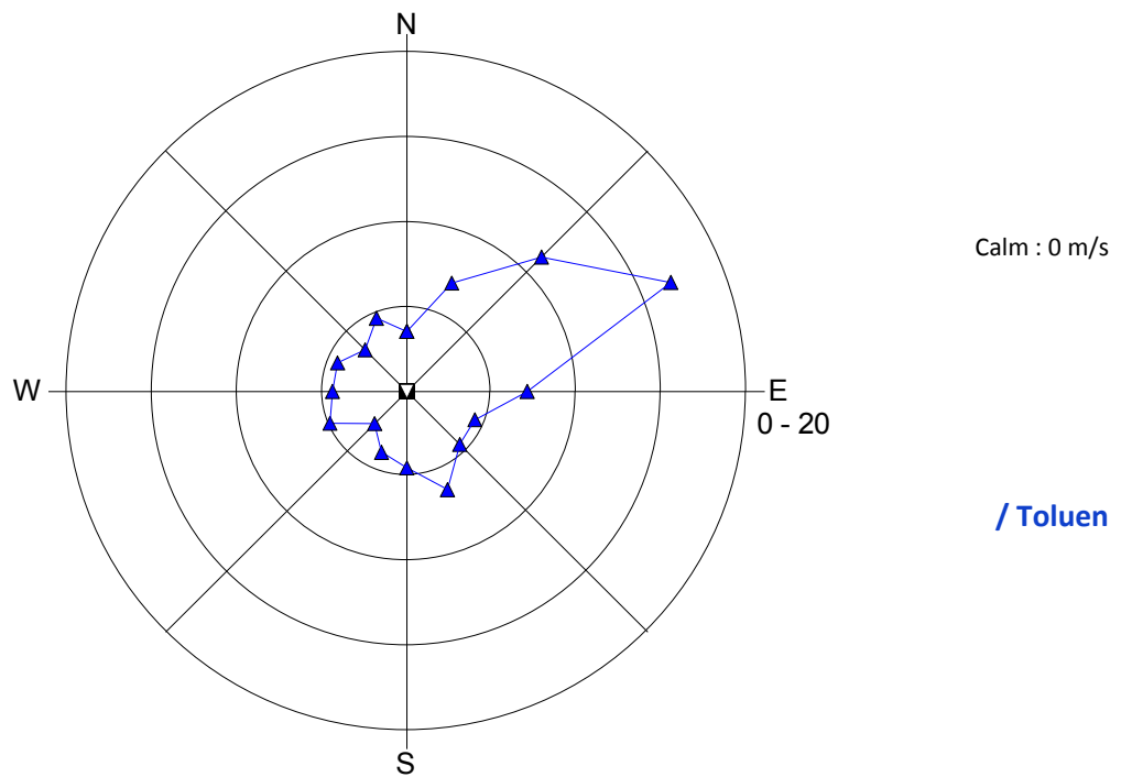
Slika 10: Roža onesnaženost - toluen, november 2012.
