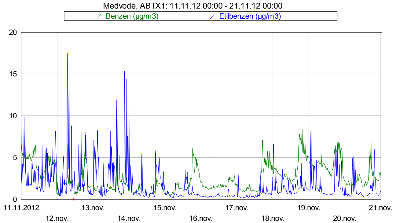
Slika 4: Imisijske koncentracije benzena in etilbenzena med 11. 11. 2012 in 20. 11. 2012.
