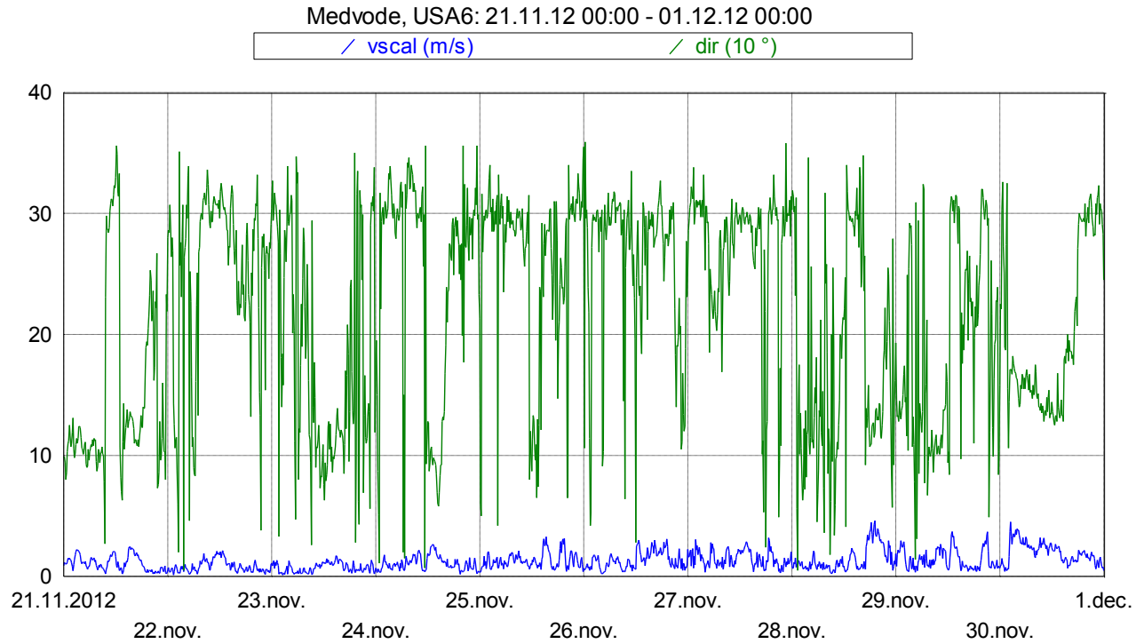
Slika 17: Smer in hitrost vetra med 21. 11. 2012 in 30. 11. 2012.
