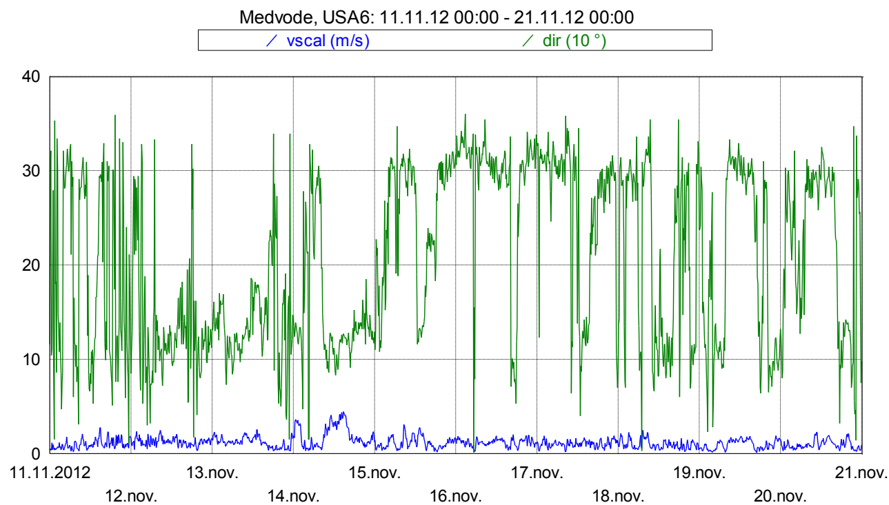
Slika 16: Smer in hitrost vetra med 11. 11. 2012 in 20. 11. 2012.
