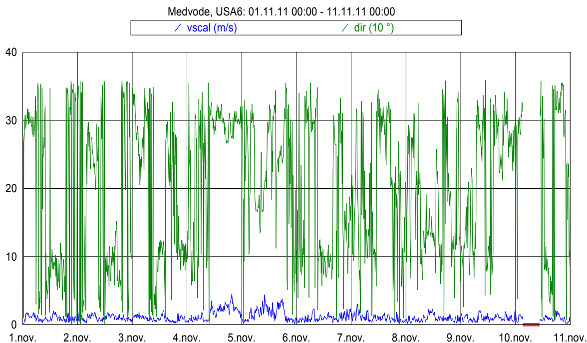
Slika 15: Smer in hitrost vetra med 1. 11. 2011 in 10. 11. 2011.
