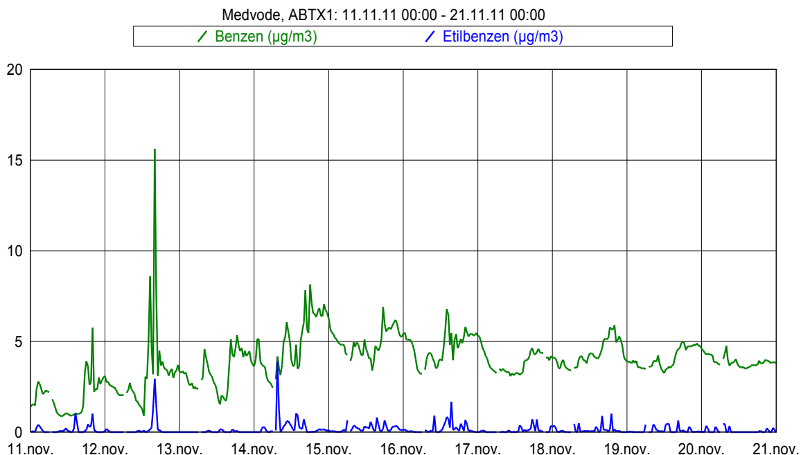
Slika 4: Imisijske koncentracije benzena in etilbenzena med 11. 11. 2011 in 20. 11. 2011.
