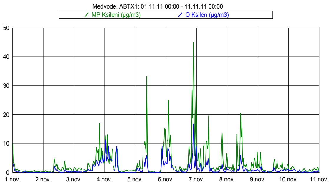
Slika 11: Imisijske koncentracije M&P in O ksilena med 1. 11. 2011 in 10. 11. 2011.
