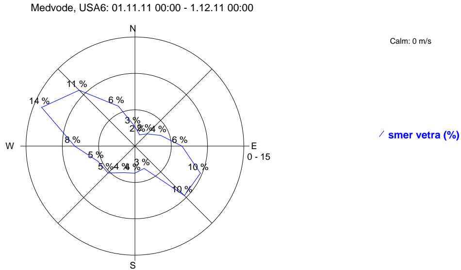
Slika 18: Roža vetrov, november 2011.
