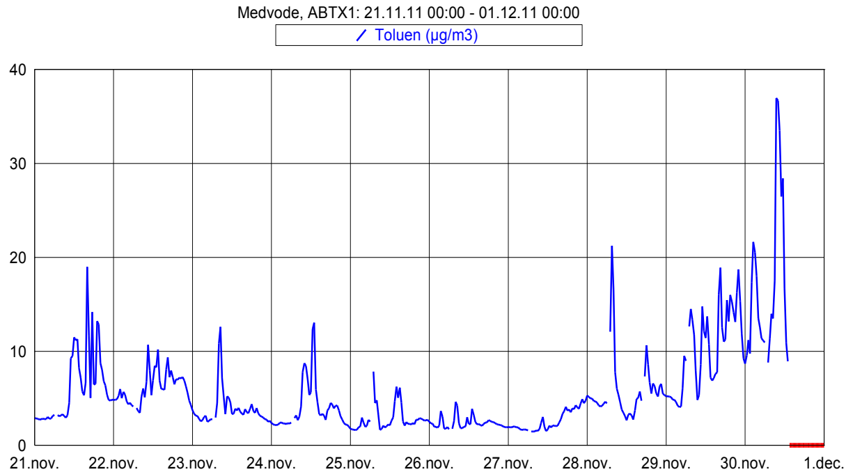
Slika 9: Imisijske koncentracije toluena med 21. 11. 2011 in 30. 11. 2011.
