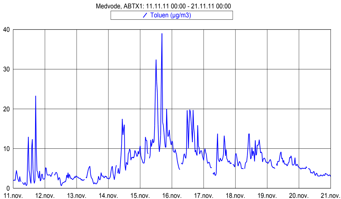
Slika 8: Imisijske koncentracije toluena med 11. 11. 2011 in 20. 11. 2011.
