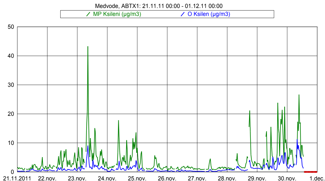
Slika 13: Imisijske koncentracije M&P in O ksilena med 21. 11. 2011 in 30. 11. 2011.
