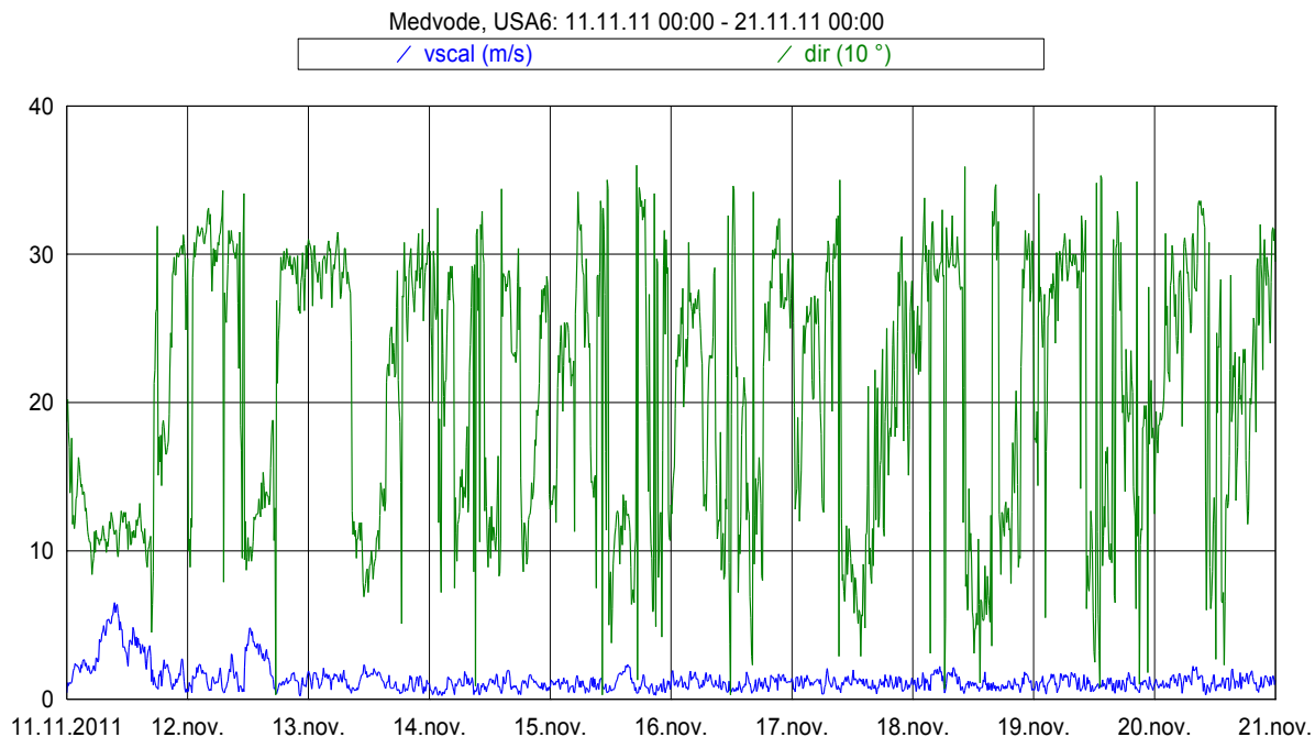
Slika 16: Smer in hitrost vetra med 11. 11. 2011 in 20. 11. 2011.
