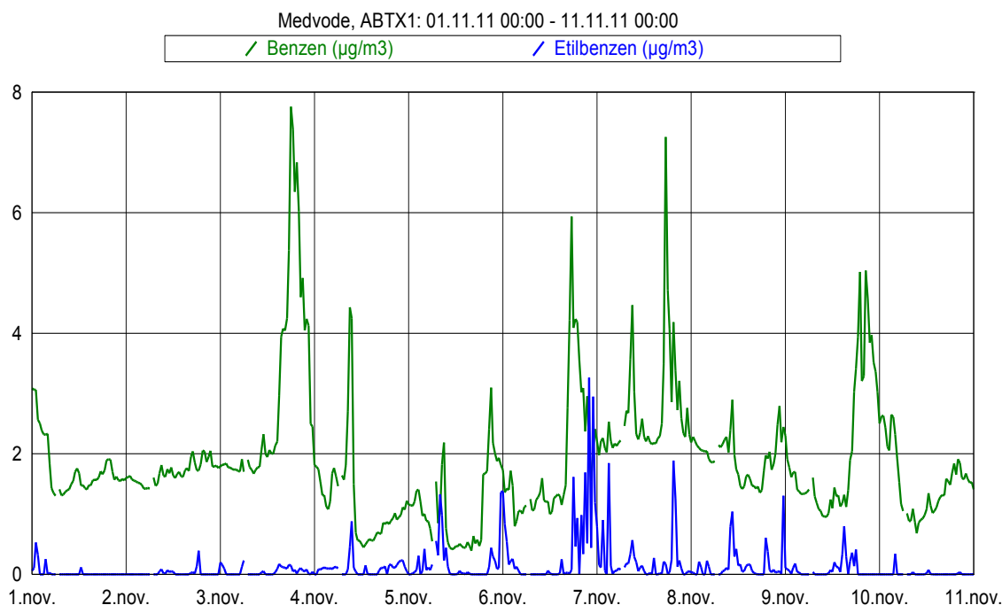
Slika 3: Imisijske koncentracije benzena in etilbenzena med vključno 1. 11. 2011 in 10. 11. 2011.
