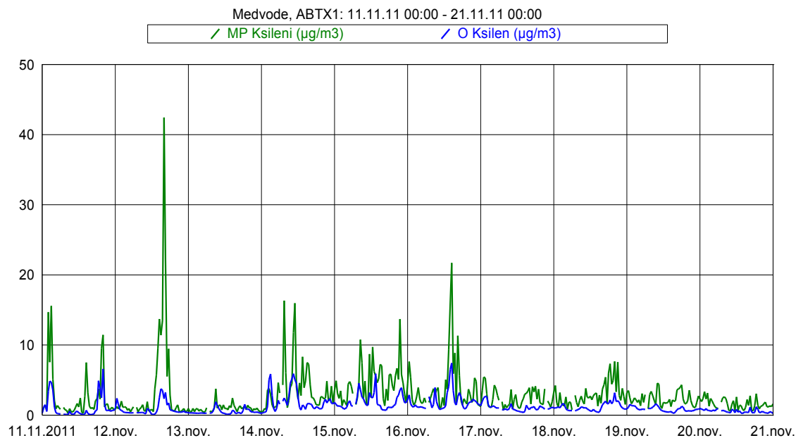
Slika 12: Imisijske koncentracije M&P in O ksilena med 11. 11. 2011 in 20. 11. 2011.
