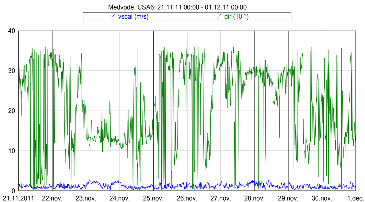
Slika 17: Smer in hitrost vetra med 21. 11. 2011 in 30. 11. 2011.
