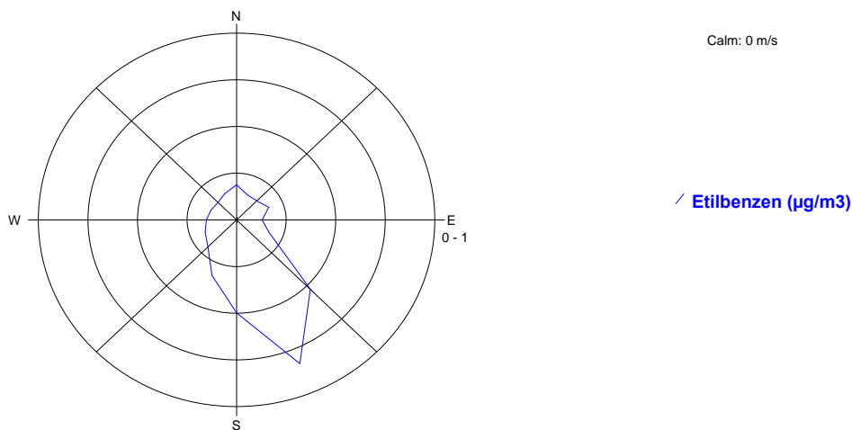
Slika 6: Roža onesnaženosti – benzen (zgoraj) in etilbenzen (spodaj), november 2011.
