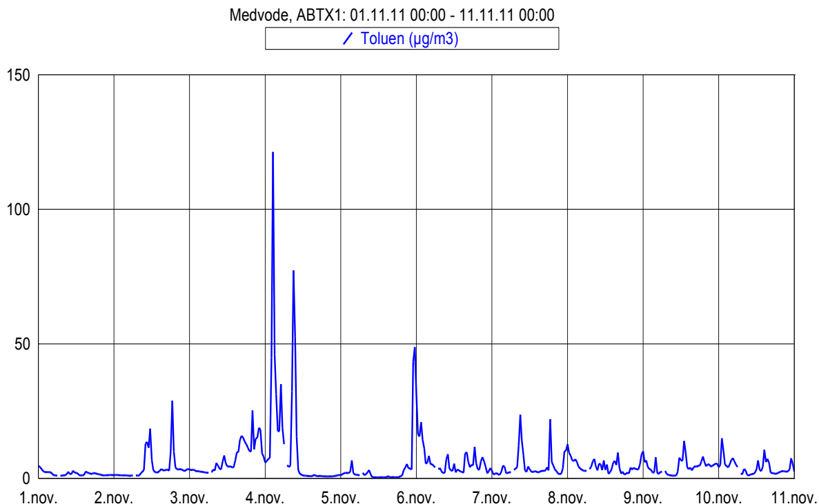
Slika 7: Imisijske koncentracije toluena med 1. 11. 2011 in 10. 11. 2011.
