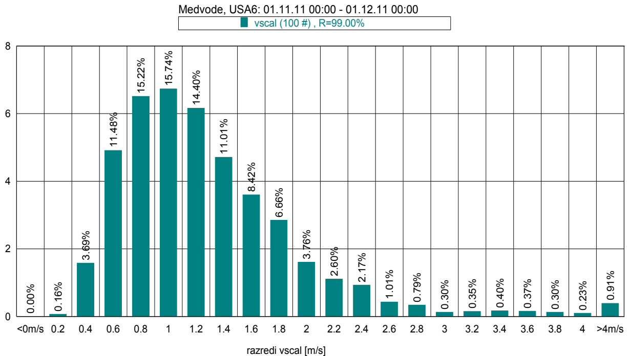
Slika 19: Frekvenčna porazdelitev po hitrosti vetra, november 2011.
