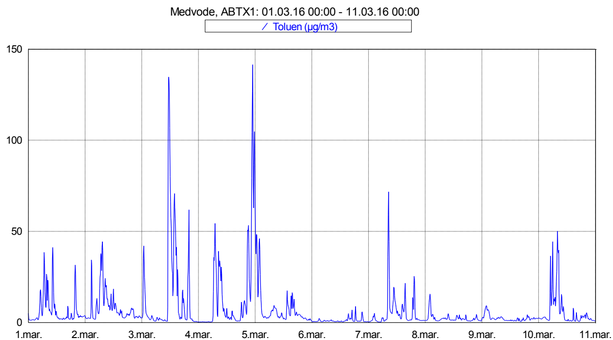
Slika 8: Imisijske koncentracije toluena med vključno 1. 3. 2016 in 10. 3. 2016.
