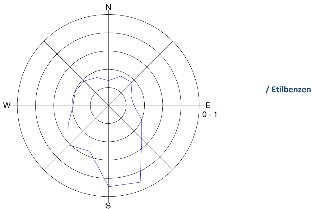
Slika 7: Roža onesnaženosti – etilbenzen, marec 2016.
