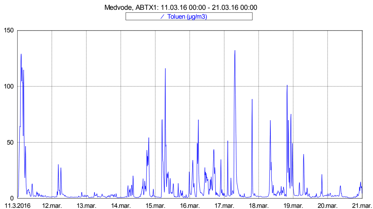
Slika 9: Imisijske koncentracije toluena med 11. 3. 2016 in 20. 3. 2016.
