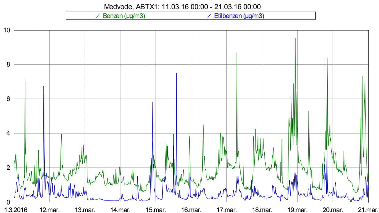
Slika 4: Imisijske koncentracije benzena in etilbenzena med 11. 3. 2016 in 20. 3. 2016.
