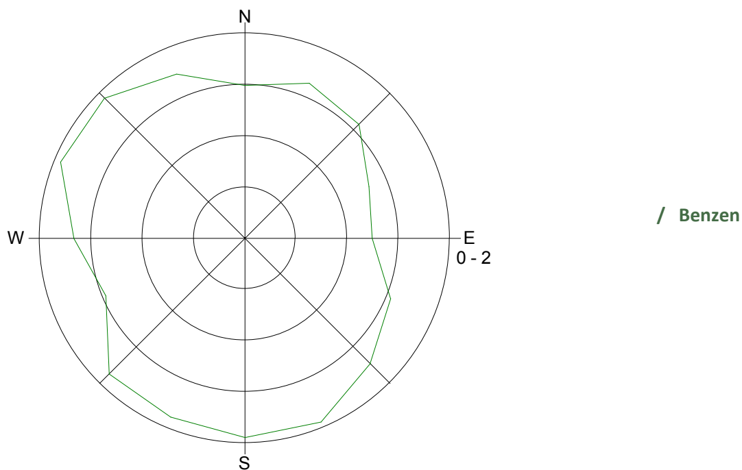
Slika 6: Roža onesnaženosti – benzen, marec 2016.
