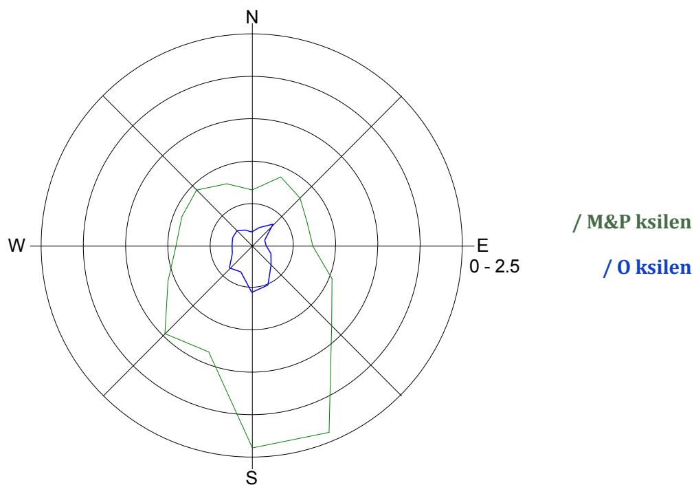
Slika 15: Roža onesnaženosti - M & P ksilen in O ksilen, marec 2016.
