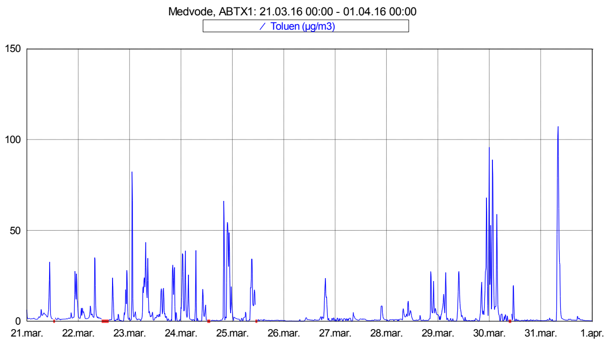
Slika 10: Imisijske koncentracije toluenta med 21. 3. 2016 in 31. 3. 2016.
