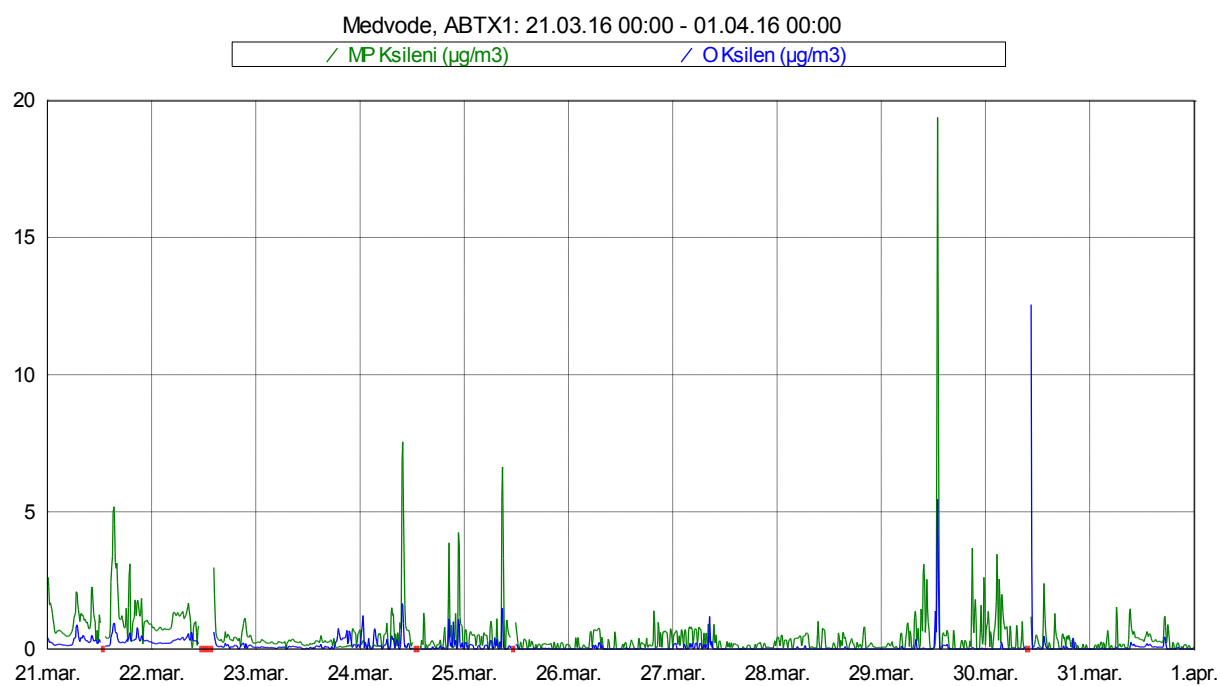
Slika 14: Imisijske koncentracije M&P in O ksilena med 21. 3. 2016 in 31. 3. 2016.
