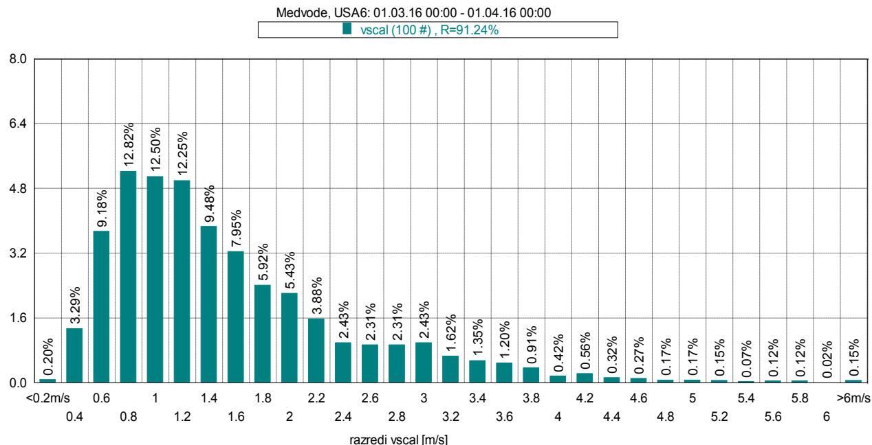
Slika 20: Frekvenčna porazdelitev po hitrosti vetra, marec 2016.
