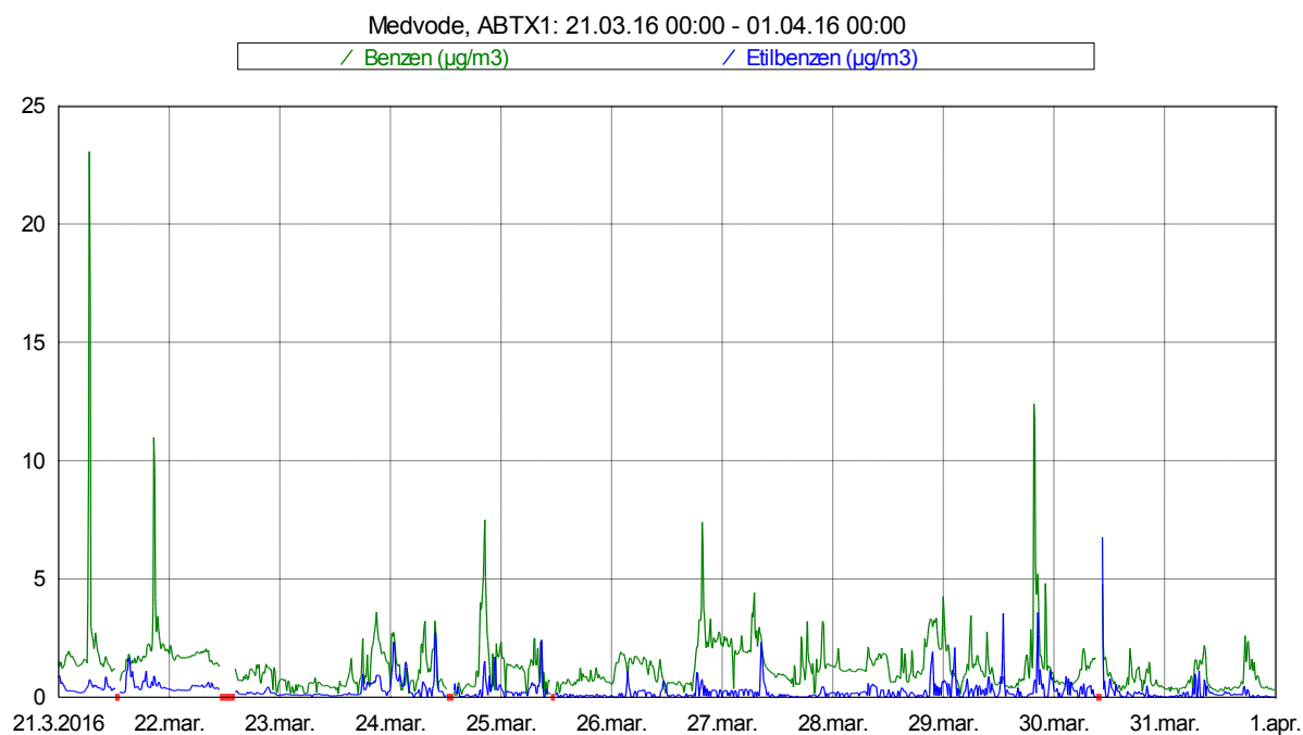
Slika 5: Imisijske koncentracije benzena in etilbenzena med 21. 3. 2016 in 31. 3. 2016.
