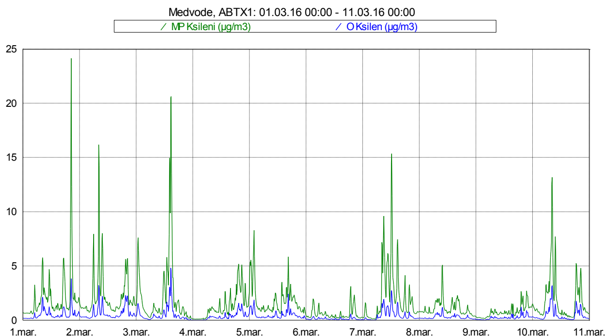
Slika 12: Imisijske koncentracije M&P in O ksilena med vključno 1. 3. 2016 in 10. 3. 2016.
