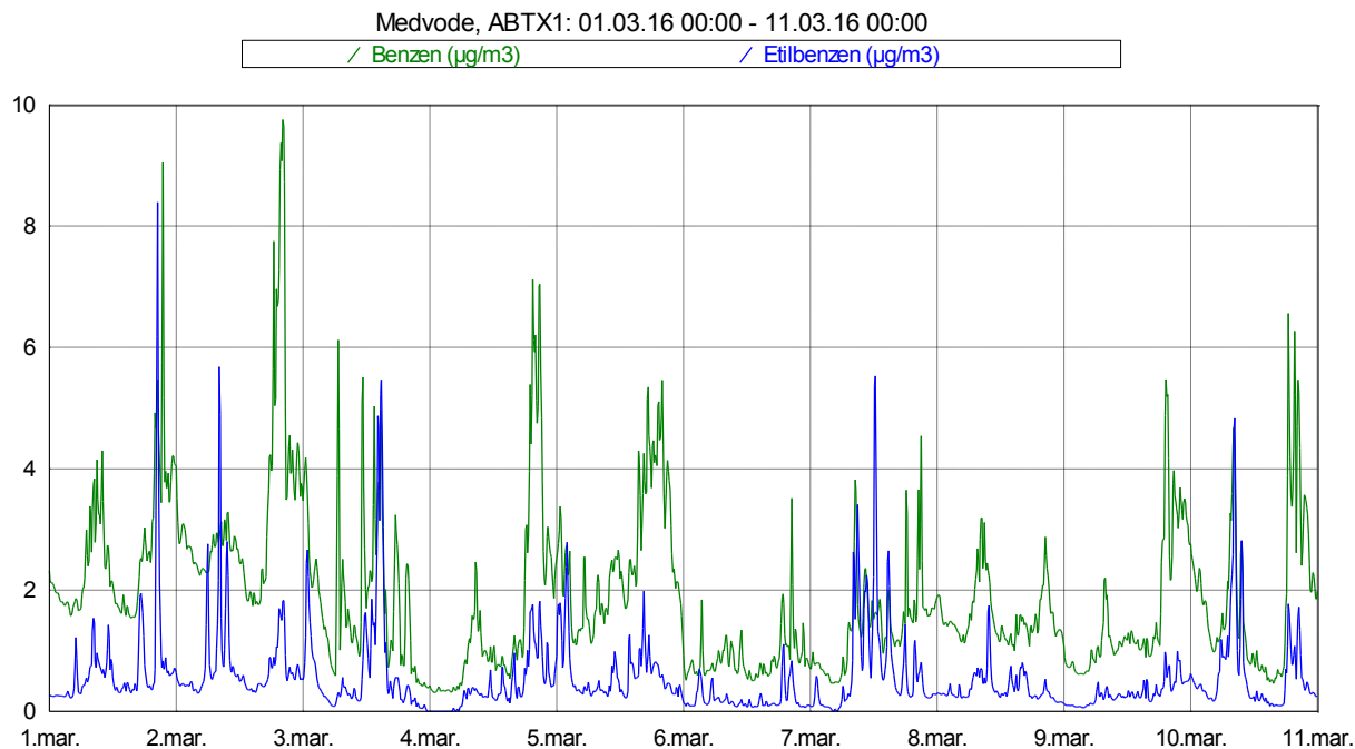
Slika 3: Imisijske koncentracije benzena in etilbenzena med vključno 1. 3. 2016 in 10. 3. 2016.
