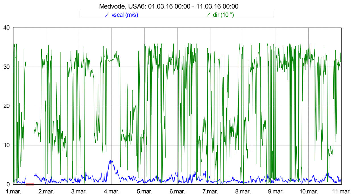
Slika 16: Smer in hitrost vetra med 1. 3. 2016 in 10. 3. 2016.
