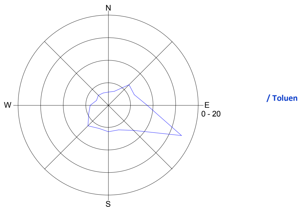
Slika 11: Roža onesnaženost - toluen, marec 2016.
