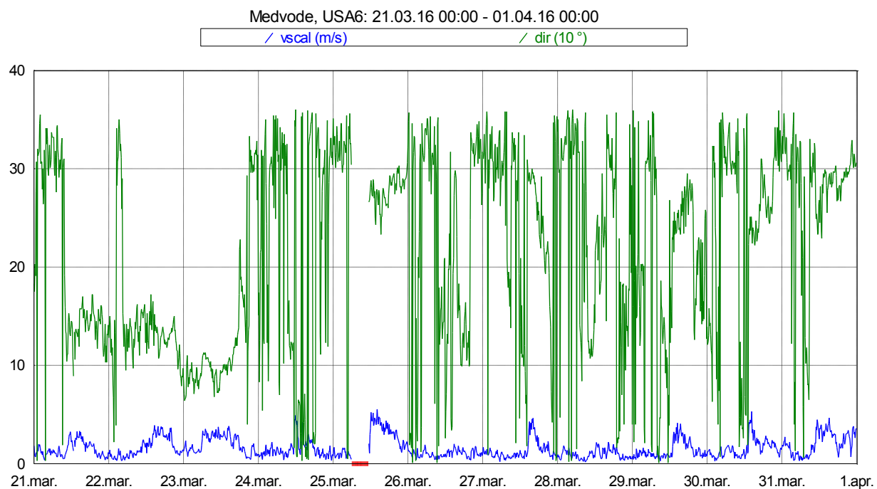
Slika 18: Smer in hitrost vetra med 21. 3. 2016 in 31. 3. 2016.
