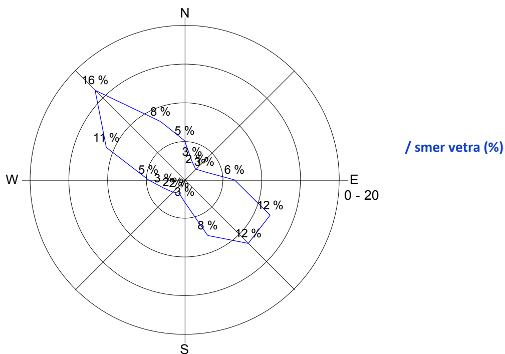
Slika 19: Roža vetrov, marec 2016.
