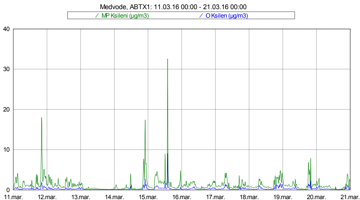
Slika 13: Imisijske koncentracije M&P in O ksilena med 11. 3. 2016 in 20. 3. 2016.
