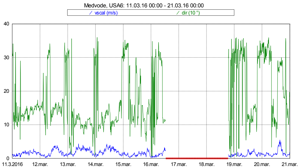
Slika 17: Smer in hitrost vetra med 11. 3. 2016 in 20. 3. 2016.
