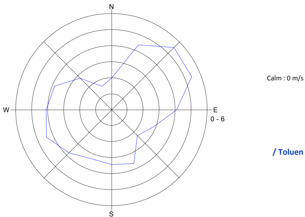
Slika 10: Roža onesnaženost - toluen, marec 2013.
