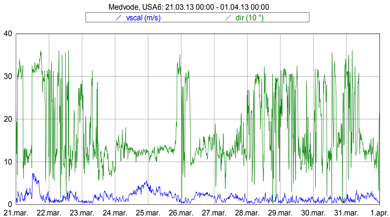
Slika 17: Smer in hitrost vetra med 21. 3. 2013 in 31. 3. 2013.
