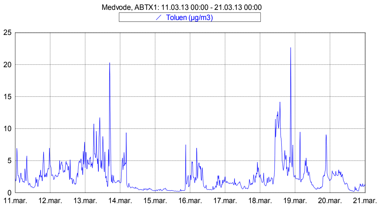
Slika 8: Imisijske koncentracije toluena med 11. 3. 2013 in 21. 3. 2013.
