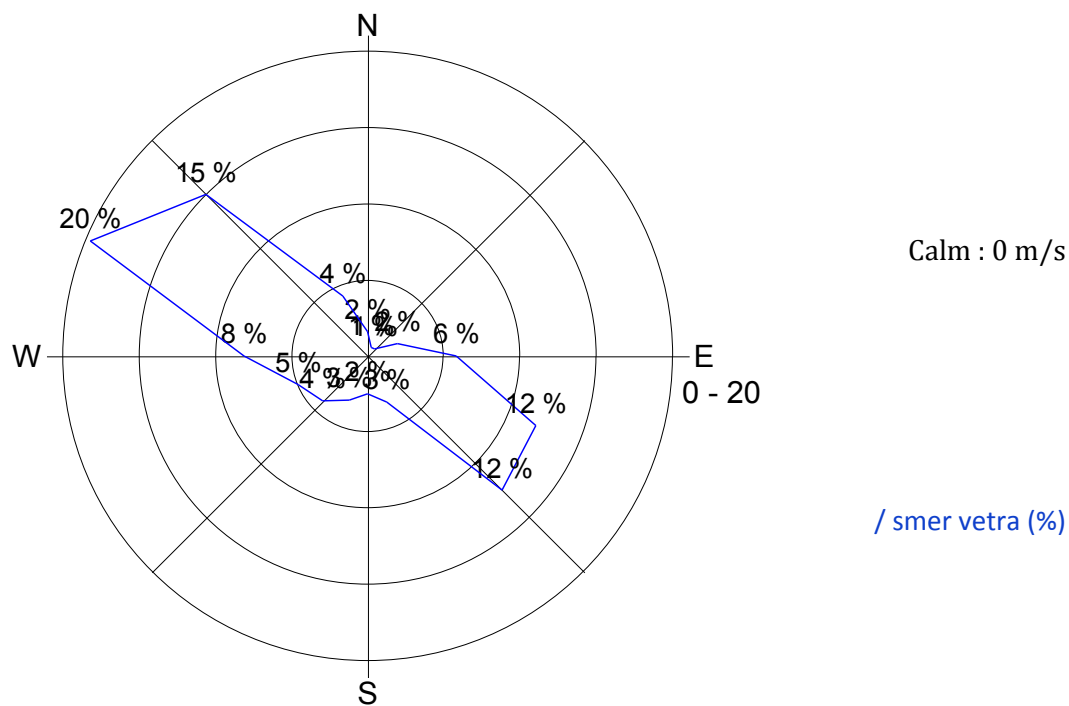
Slika 18: Roža vetrov, marec 2013.
