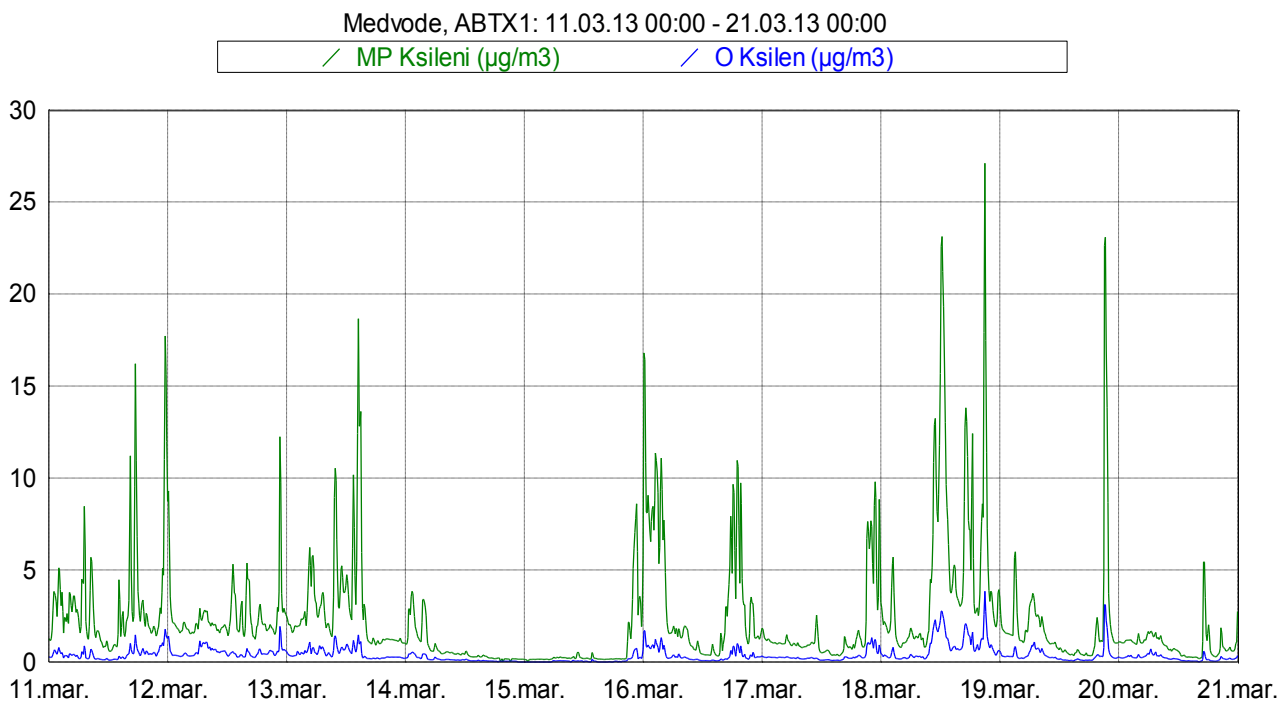
Slika 12: Imisijske koncentracije M&P in O ksilena med 11. 3. 2013 in 21. 3. 2013.
