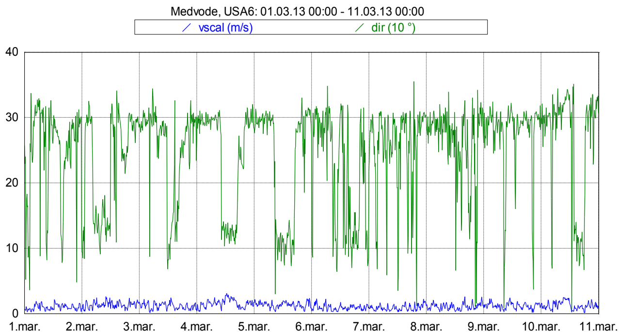
Slika 15: Smer in hitrost vetra med 1. 3. 2013 in 11. 3. 2013.
