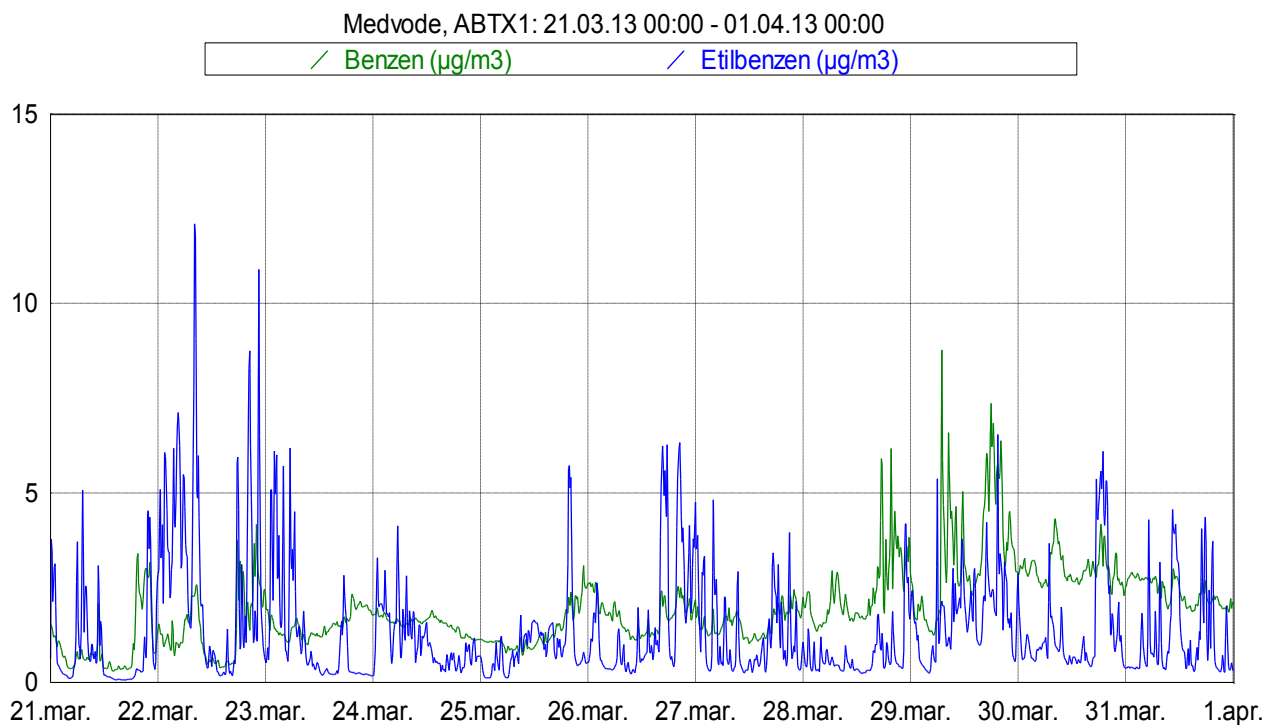
Slika 5: Imisijske koncentracije benzena in etilbenzena med 21. 3. 2013 in 31. 3. 2013.
