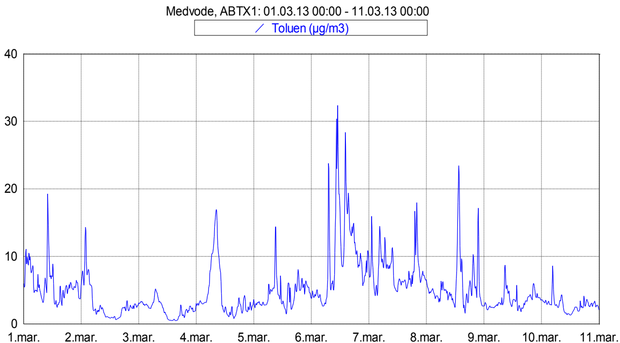
Slika 7: Imisijske koncentracije toluena med vključno 1. 3. 2013 in 11. 3. 2013.
