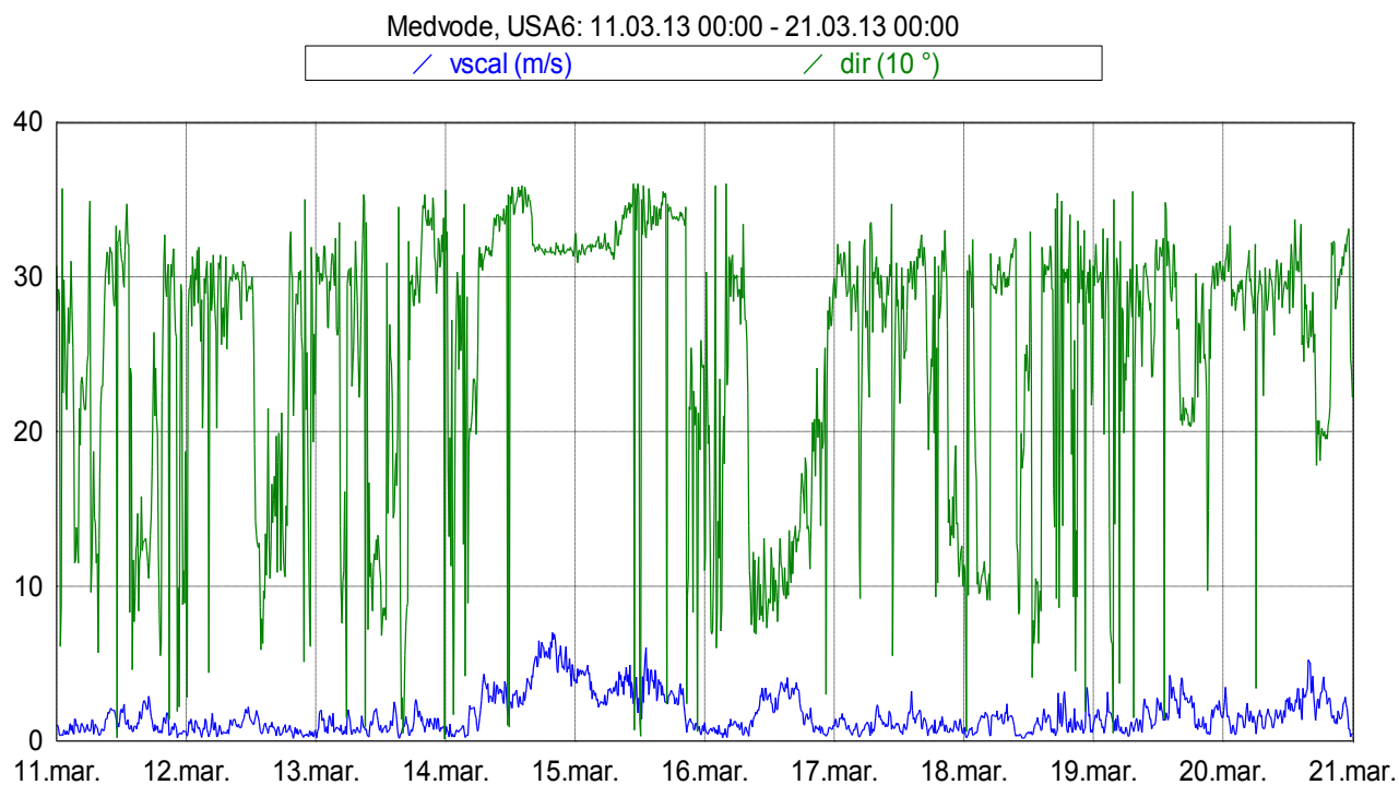
Slika 16: Smer in hitrost vetra med 11. 3. 2013 in 21. 3. 2013.
