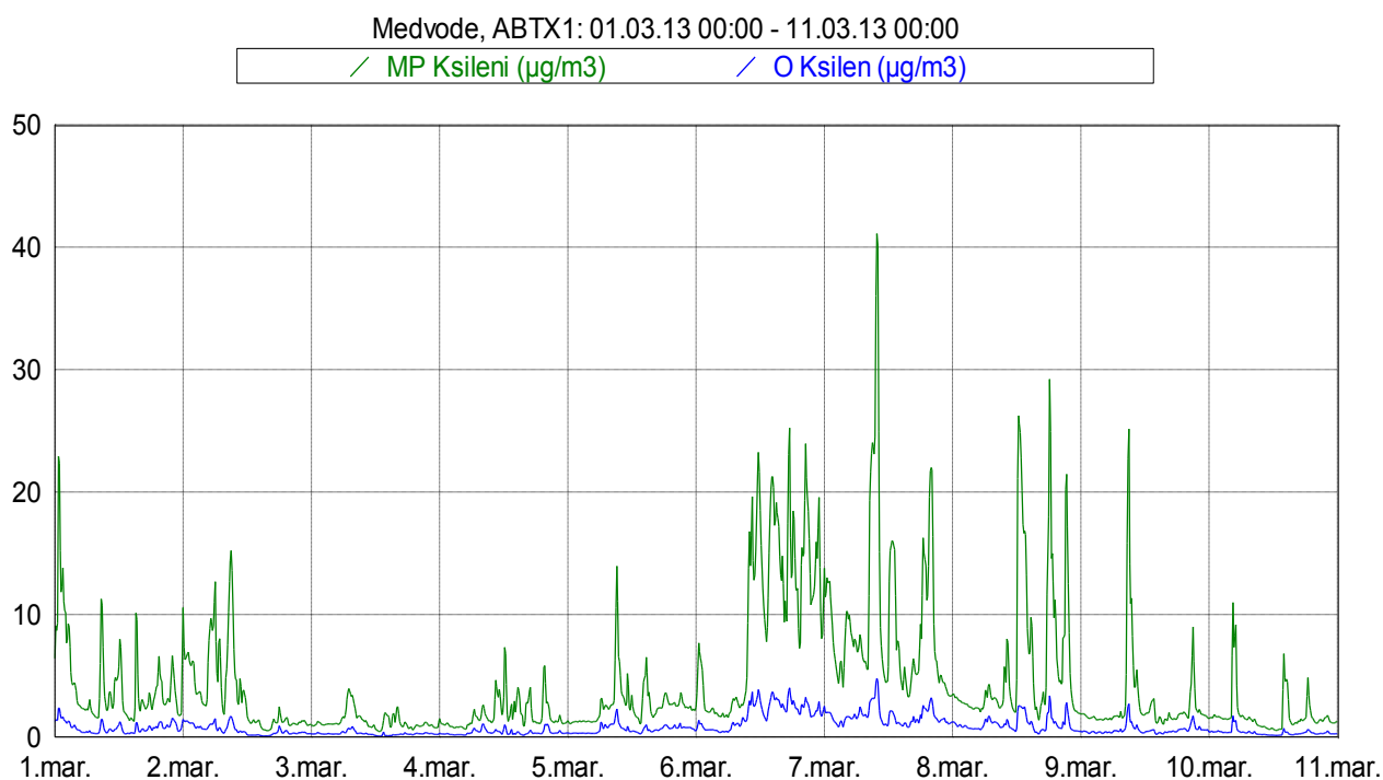
Slika 11: Imisijske koncentracije M&P in O ksilena med vključno 1. 3. 2013 in 11. 3. 2013.
