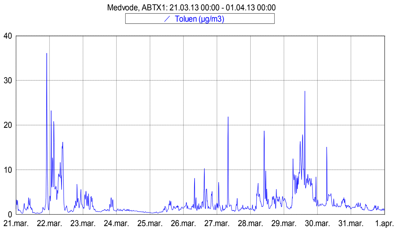
Slika 9: Imisijske koncentracije toluea med 21. 3. 2013 in 31. 3. 2013.
