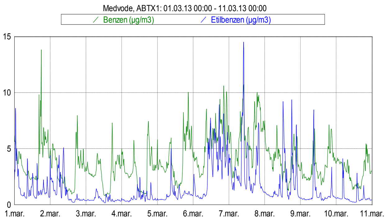
Slika 3: Imisijske koncentracije benzena in etilbenzena med vključno 1. 3. 2013 in 11. 3. 2013.
