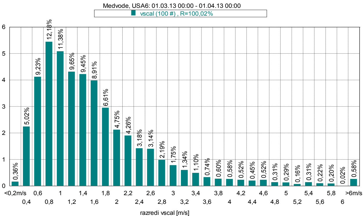
Slika 19: Frekvenčna porazdelitev po hitrosti vetra, marec 2013.
