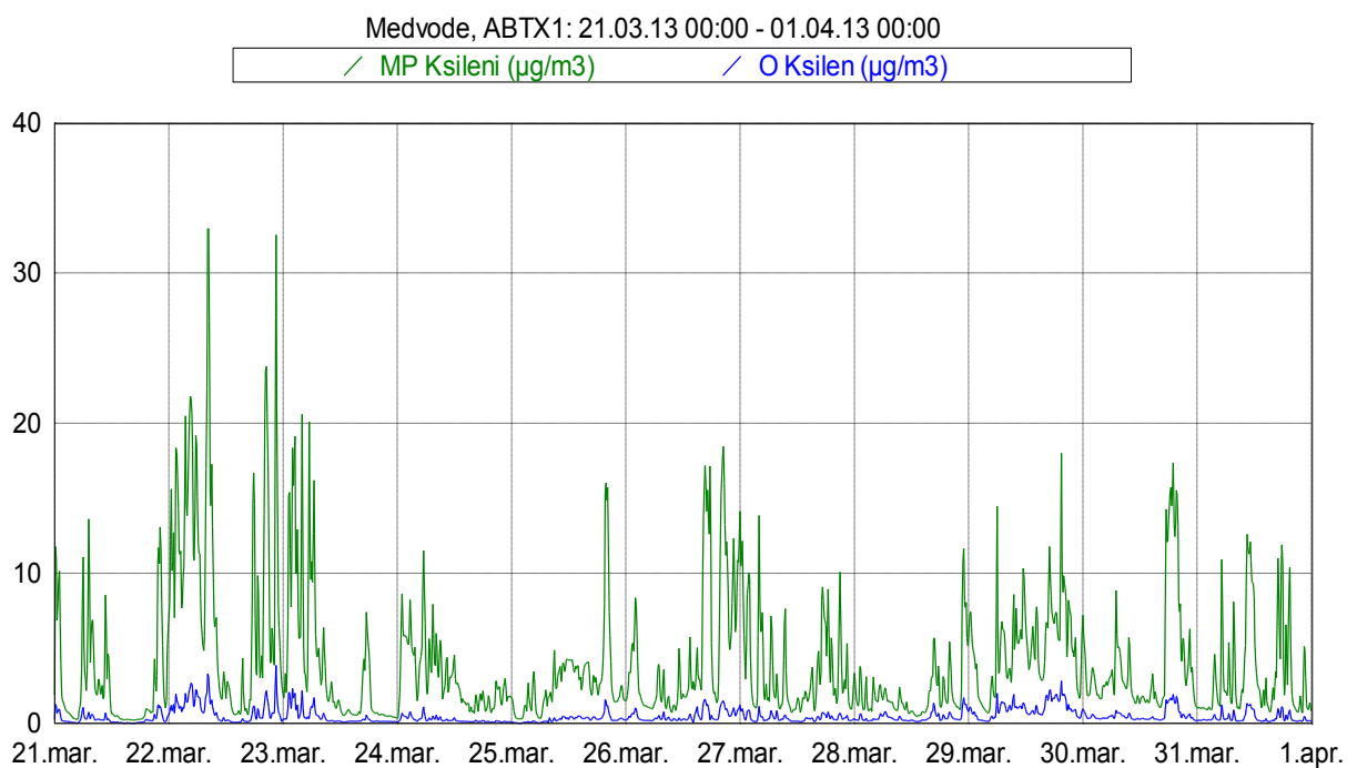
Slika 13: Imisijske koncentracije M&P in O ksilena med 21. 3. 2013 in 31. 3. 2013.
