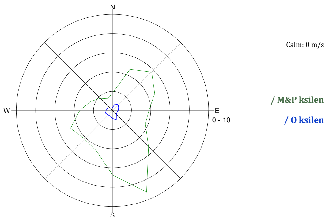
Slika 14: Roža onesnaženosti - M & P ksilen in O ksilen, marec 2013.
