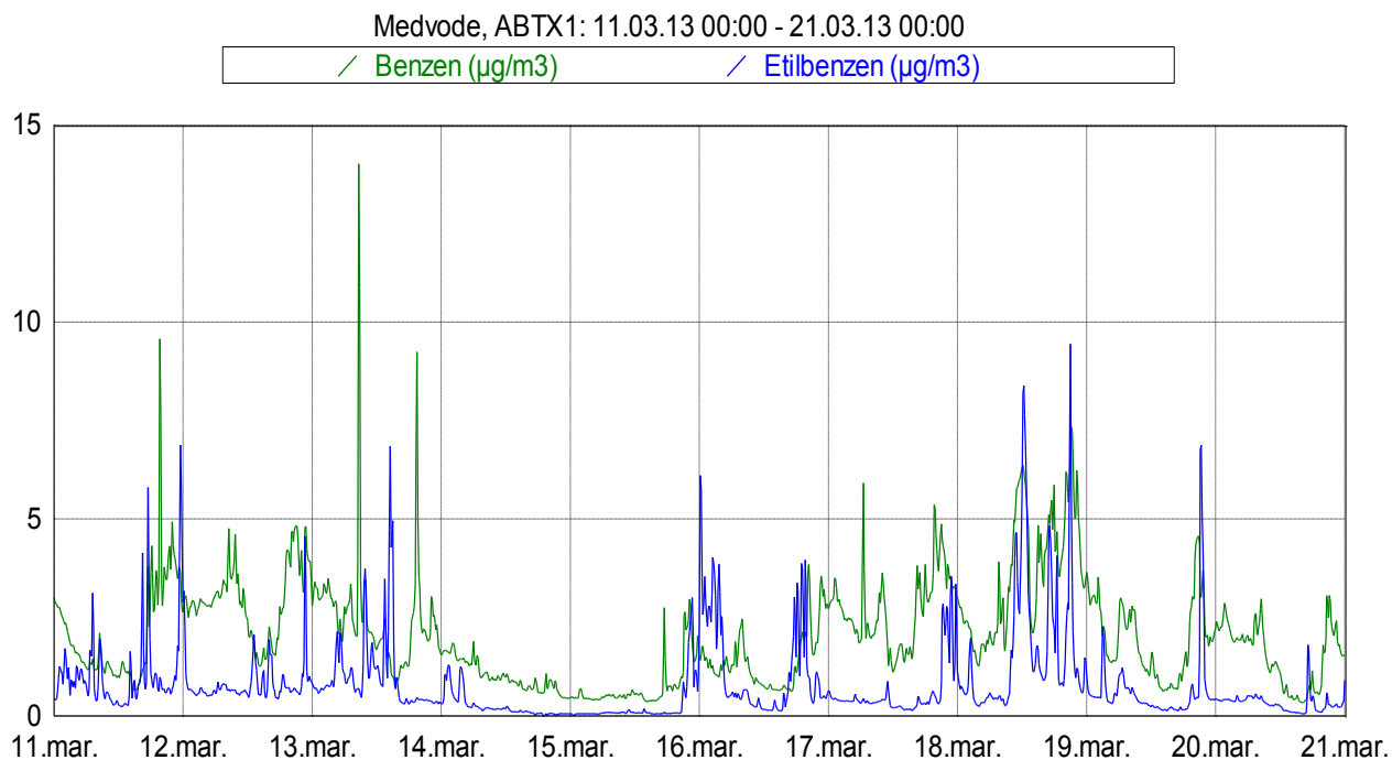
Slika 4: Imisijske koncentracije benzena in etilbenzena med 11. 3. 2013 in 21. 3. 2013.
