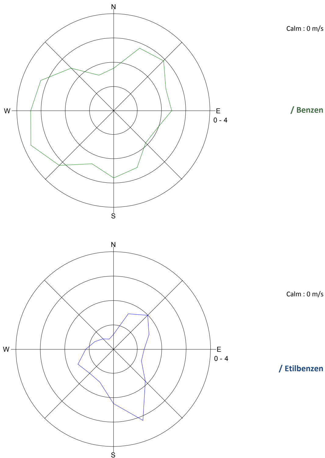
Slika 6: Roža onesnaženosti – benzen (zgoraj) in etilbenzen (spodaj), marec 2013.
