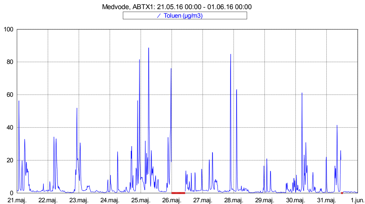
Slika 10: Imisijske koncentracije toluena med 21. 5. 2016 in 31. 5. 2016.
