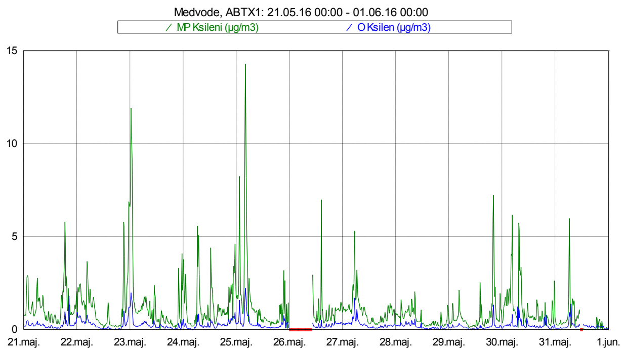
Slika 14: Imisijske koncentracije M&P in O ksilena med 21. 5. 2016 in 31. 5. 2016.
