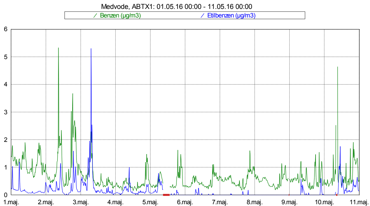
Slika 3: Imisijske koncentracije benzena in etilbenzena med vključno 1. 5. 2016 in 10. 5. 2016.
