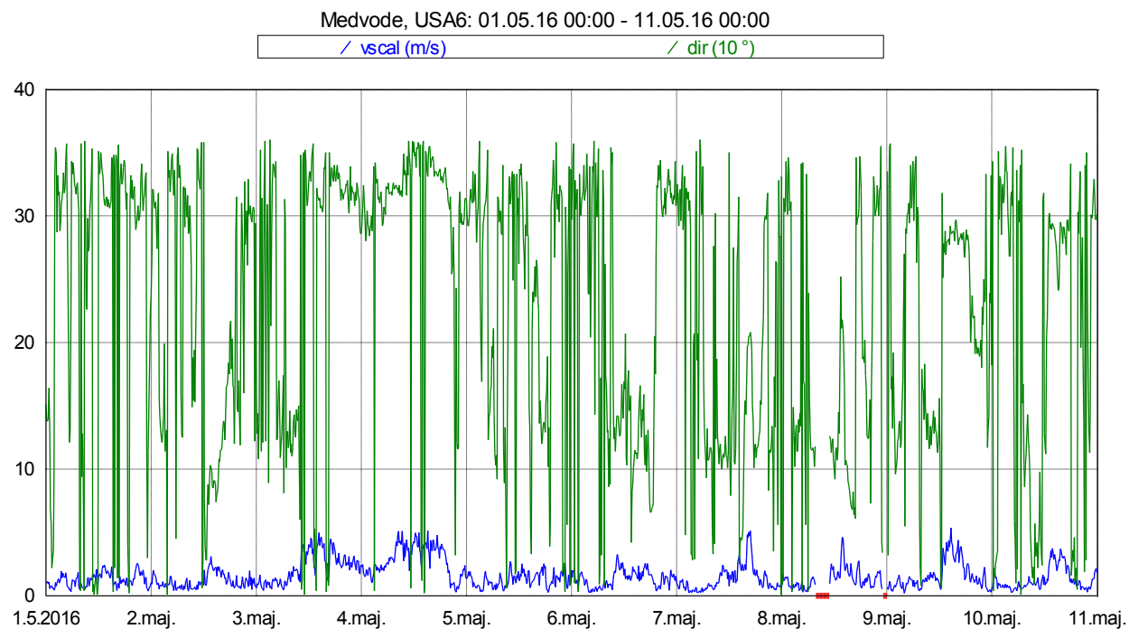
Slika 16: Smer in hitrost vetra med 1. 5. 2016 in 10. 5. 2016.
