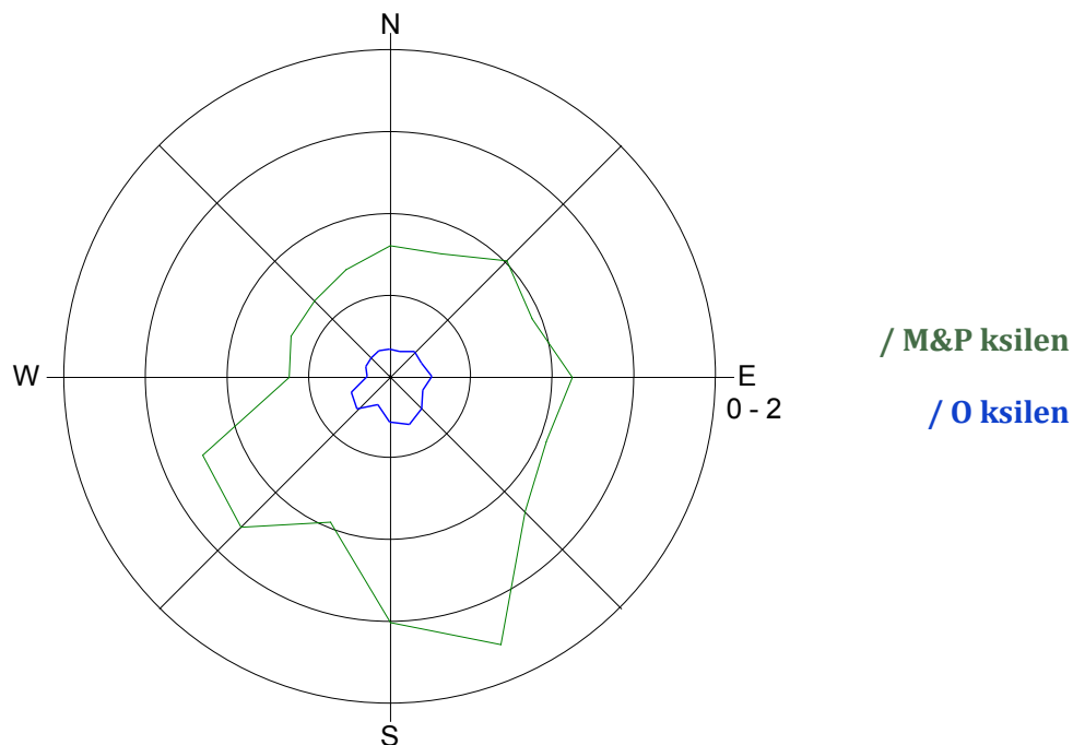
Slika 15: Roža onesnaženosti - M & P ksilen in O ksilen, maj 2016.
