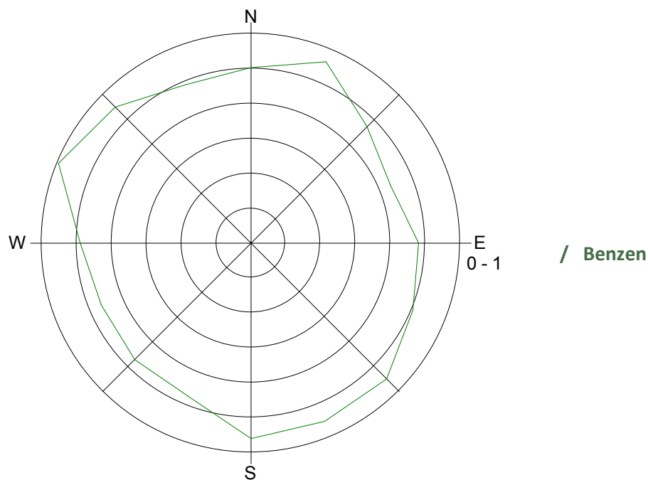
Slika 5: Imisijske koncentracije benzena in etilbenzena med 21. 5. 2016 in 31. 5. 2016.
