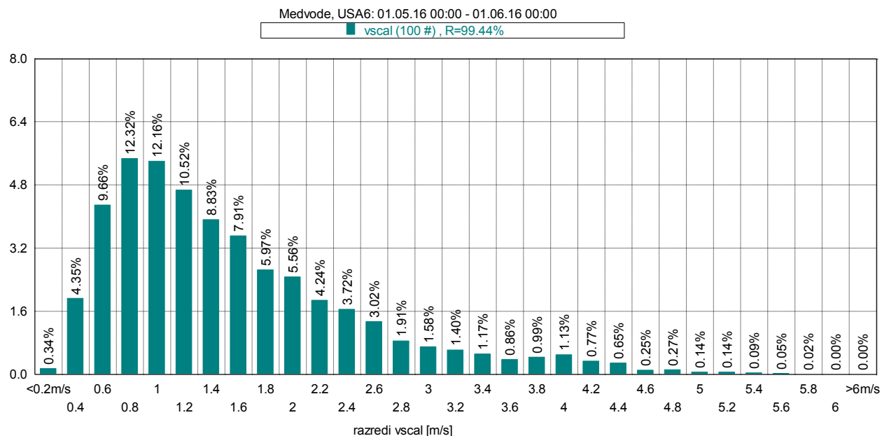
Slika 20: Frekvenčna porazdelitev po hitrosti vetra, maj 2016.
