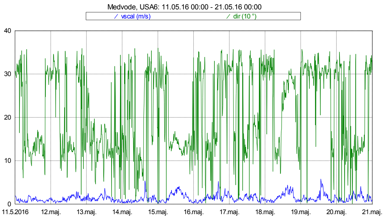
Slika 17: Smer in hitrost vetra med 11. 5. 2016 in 20. 5. 2016.
