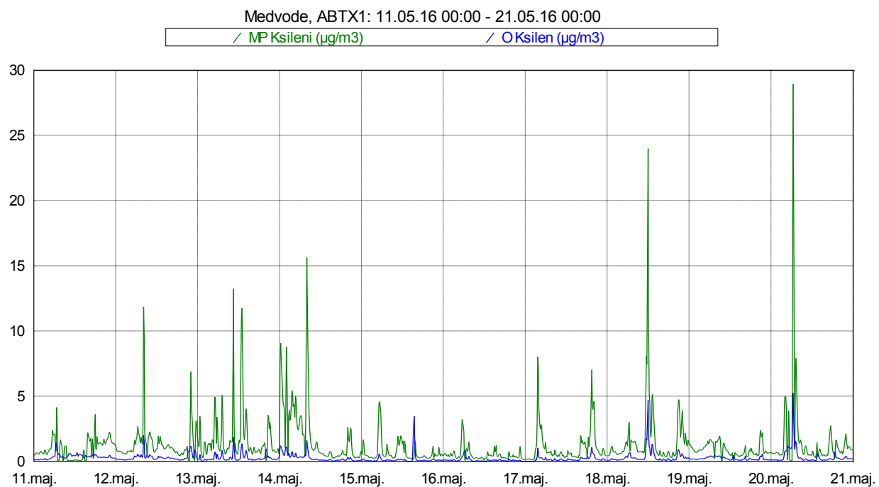
Slika 13: Imisijske koncentracije M&P in O ksilena med 11. 5. 2016 in 20. 5. 2016.
