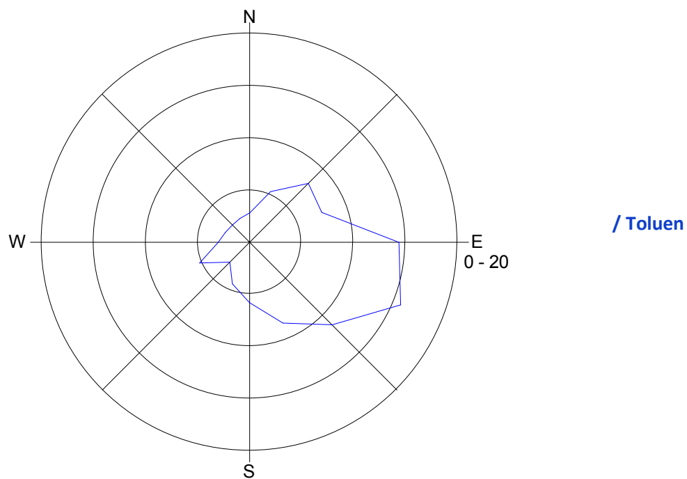
Slika 11: Roža onesnaženost - toluen, maj 2016.
