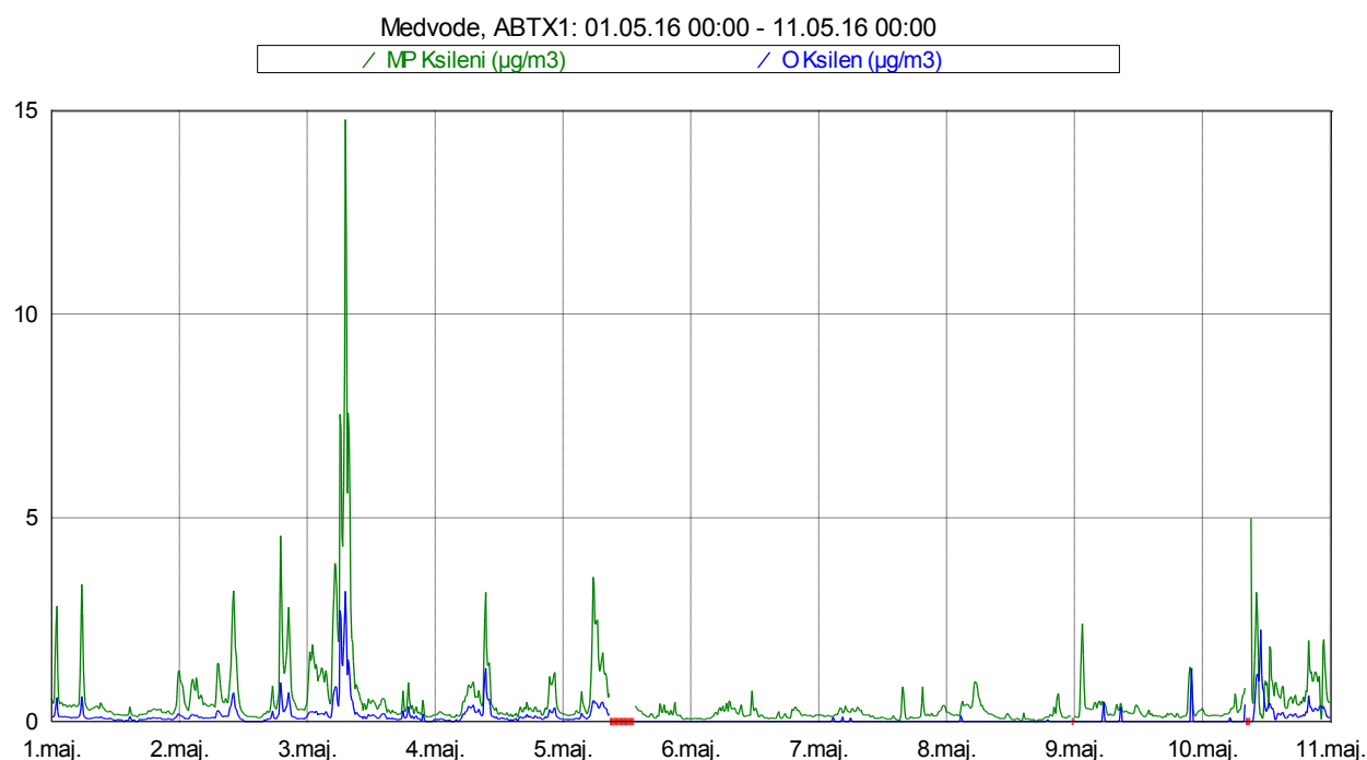
Slika 12: Imisijske koncentracije M&P in O ksilena med vključno 1. 5. 2016 in 10. 5. 2016.
