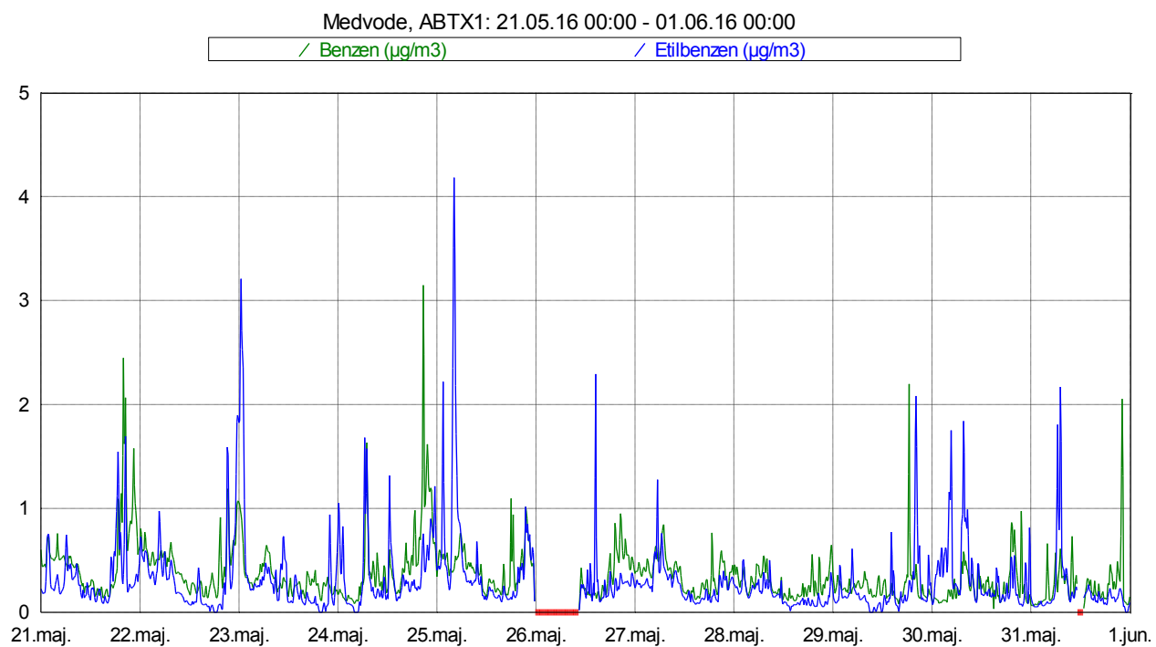
Slika 5: Imisijske koncentracije benzena in etilbenzena med 21. 5. 2016 in 31. 5. 2016.
