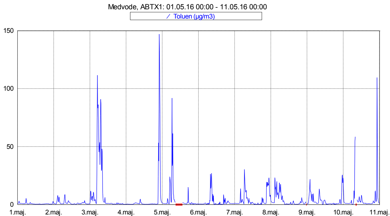
Slika 8: Imisijske koncentracije toluena med vključno 1. 5. 2016 in 10. 5. 2016.
