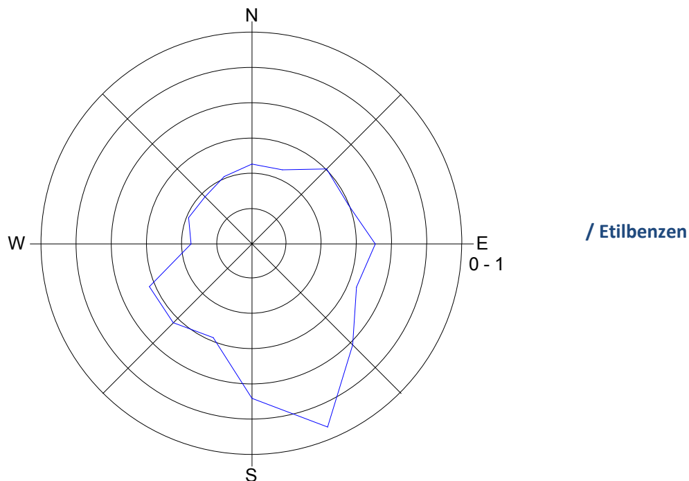
Slika 7: Roža onesnaženosti – etilbenzen, maj 2016.
