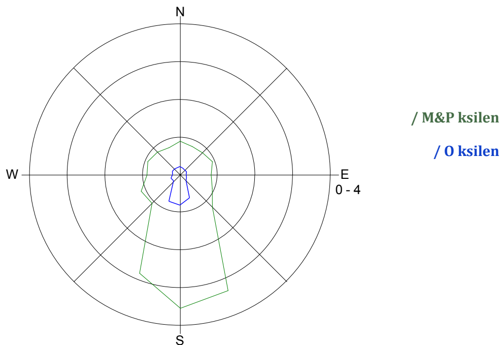
Slika 15: Roža onesnaženosti - M & P ksilen in O ksilen, maj 2015.
