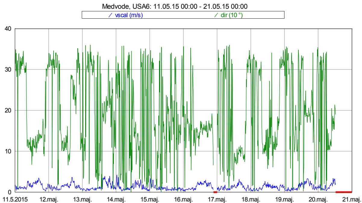
Slika 17: Smer in hitrost vetra med 11. 5. 2015 in 20. 5. 2015.
