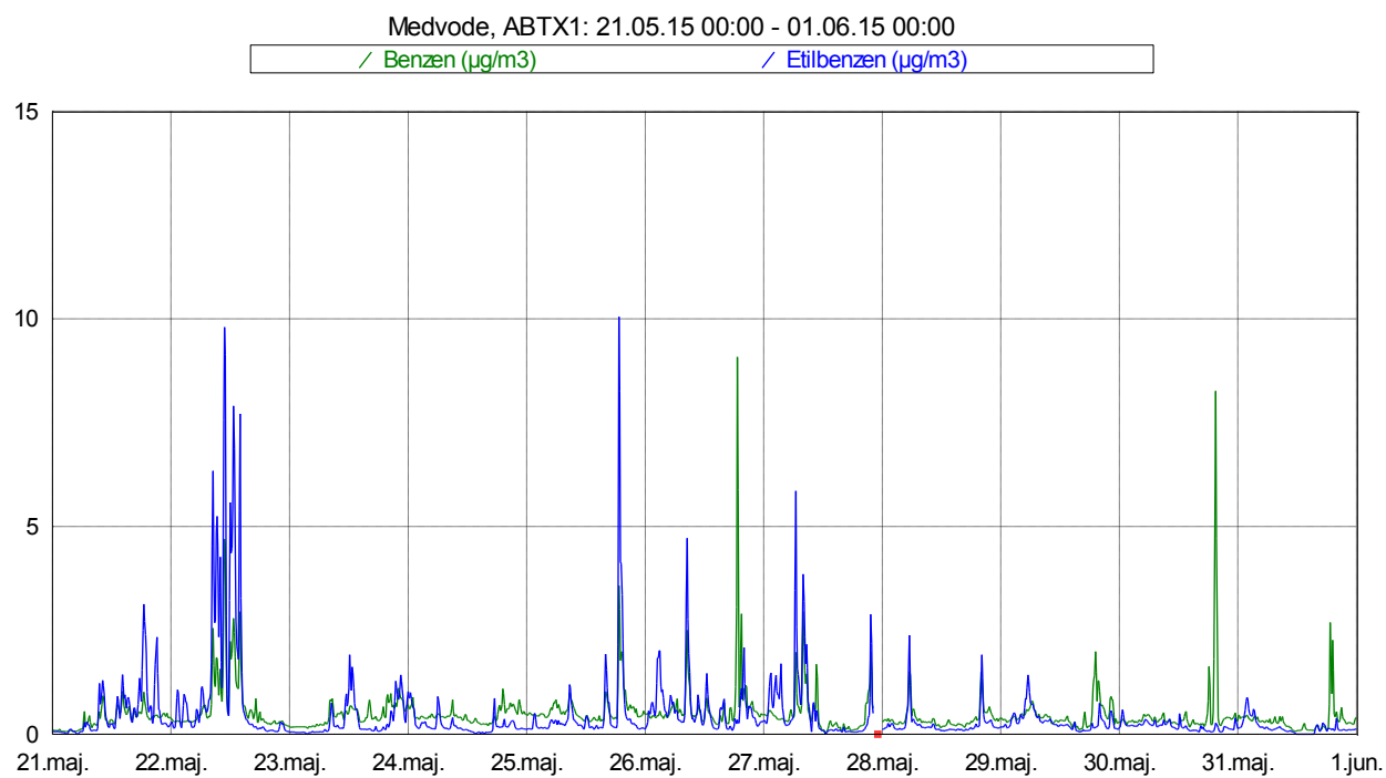
Slika 5: Imisijske koncentracije benzena in etilbenzena med 21. 5. 2015 in 31. 5. 2015.
