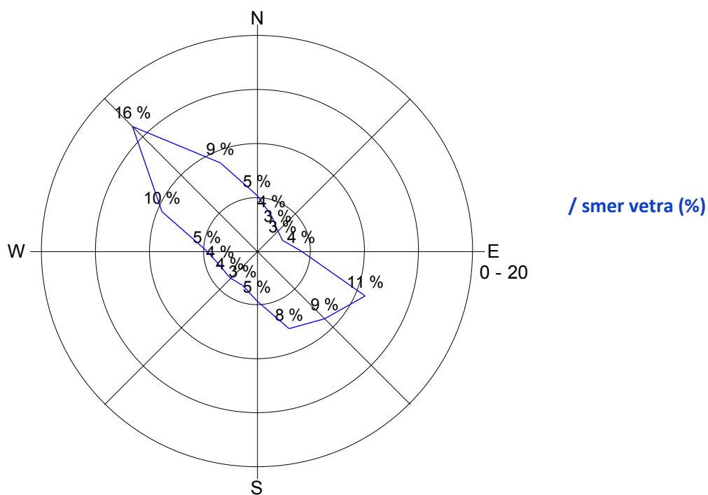
Slika 19: Roža vetrov, maj 2015.
