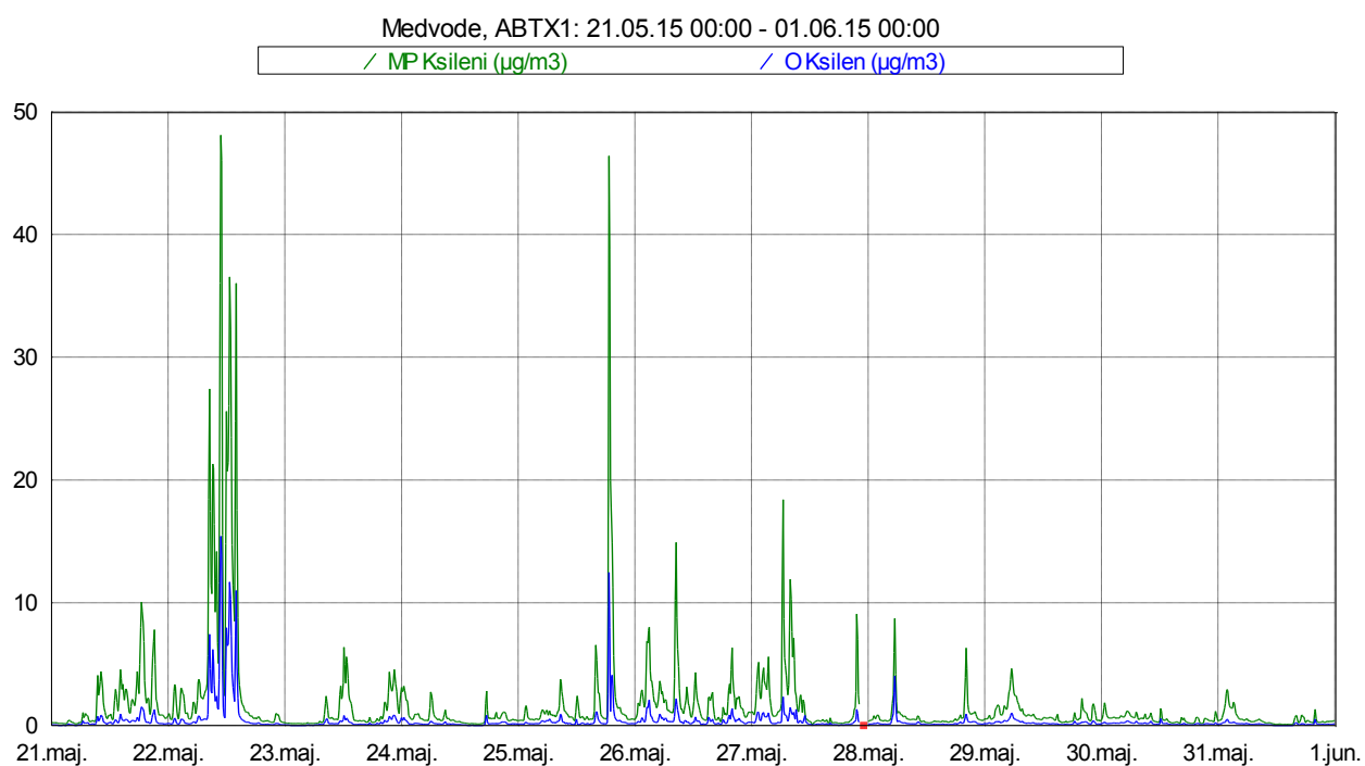
Slika 14: Imisijske koncentracije M&P in O ksilena med 21. 5. 2015 in 31. 5. 2015.
