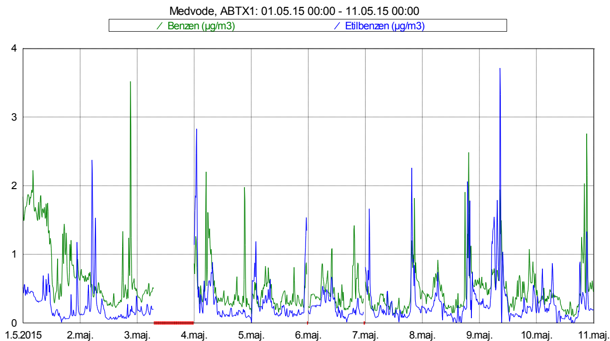
Slika 3: Imisijske koncentracije benzena in etilbenzena med vključno 1. 5. 2015 in 10. 5. 2015.
