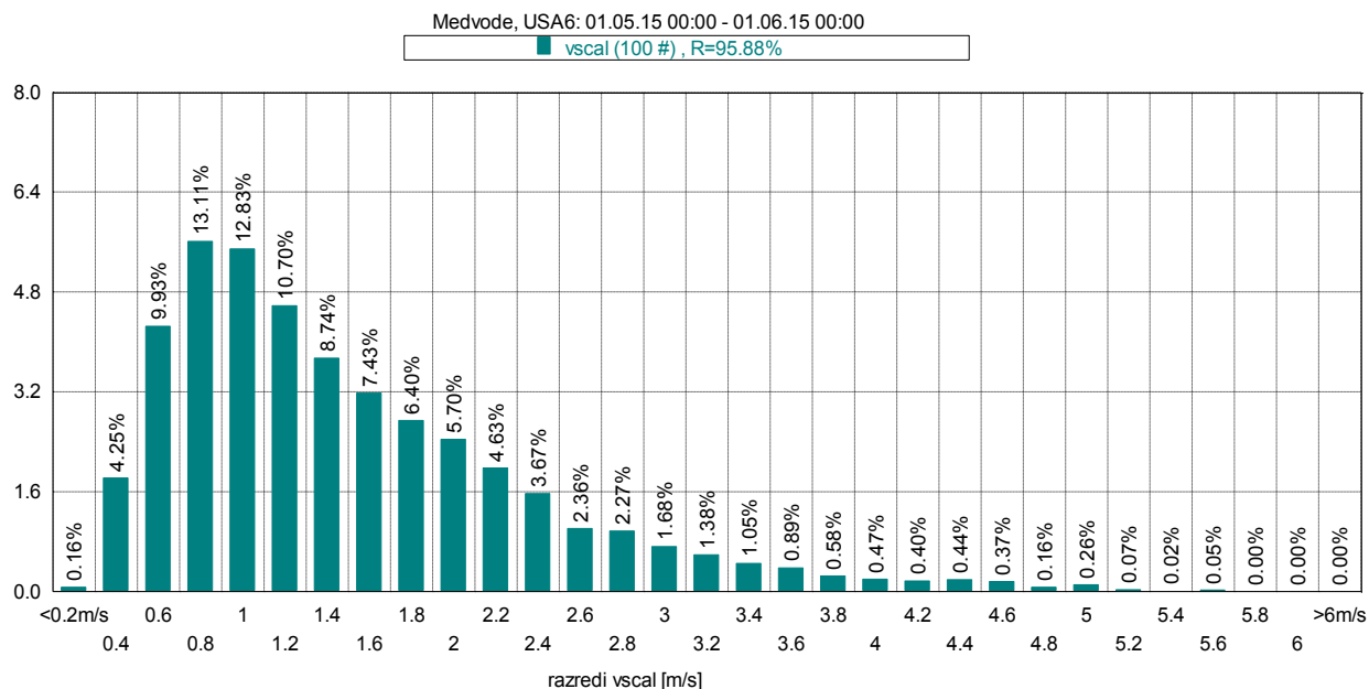
Slika 20: Frekvenčna porazdelitev po hitrosti vetra, maj 2015.
