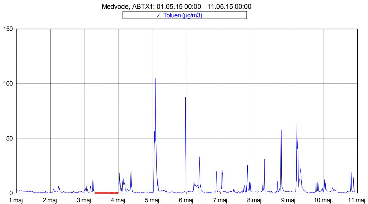
Slika 8: Imisijske koncentracije toluena med vključno 1. 5. 2015 in 10. 5. 2015.
