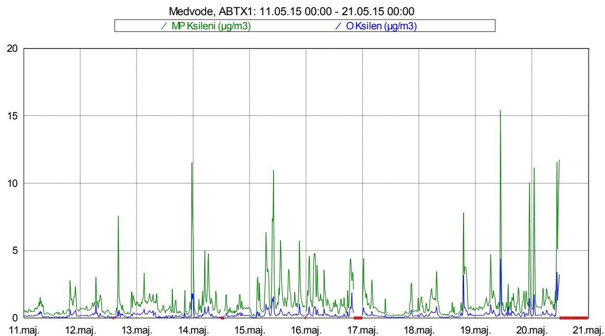
Slika 13: Imisijske koncentracije M&P in O ksilena med 11. 5. 2015 in 20. 5. 2015.
