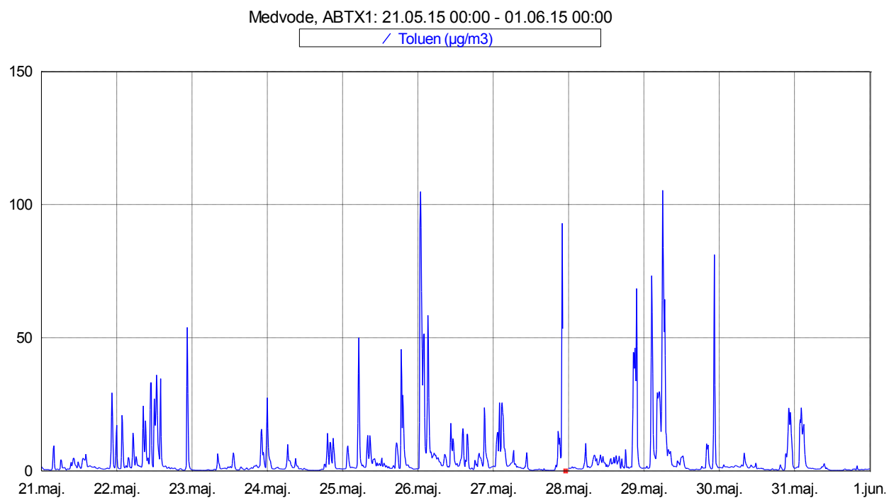
Slika 10: Imisijske koncentracije toluenta med 21. 5. 2015 in 31. 5. 2015.
