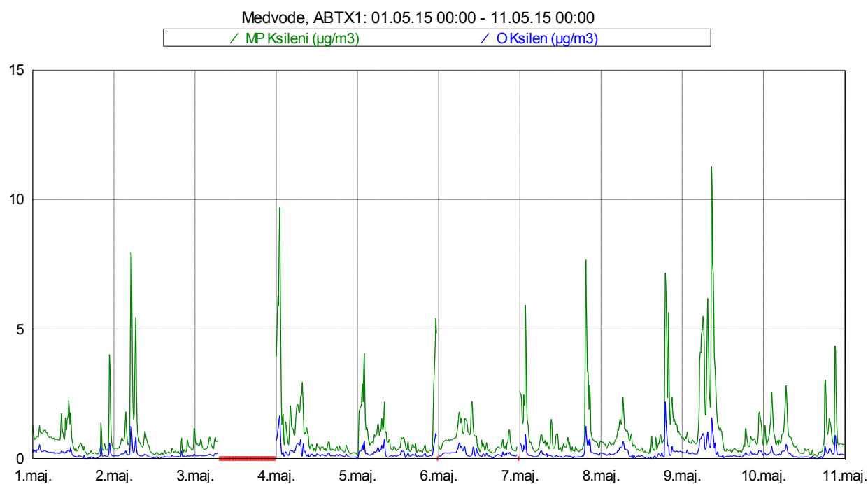
Slika 12: Imisijske koncentracije M&P in O ksilena med vključno 1. 5. 2015 in 10. 5. 2015.
