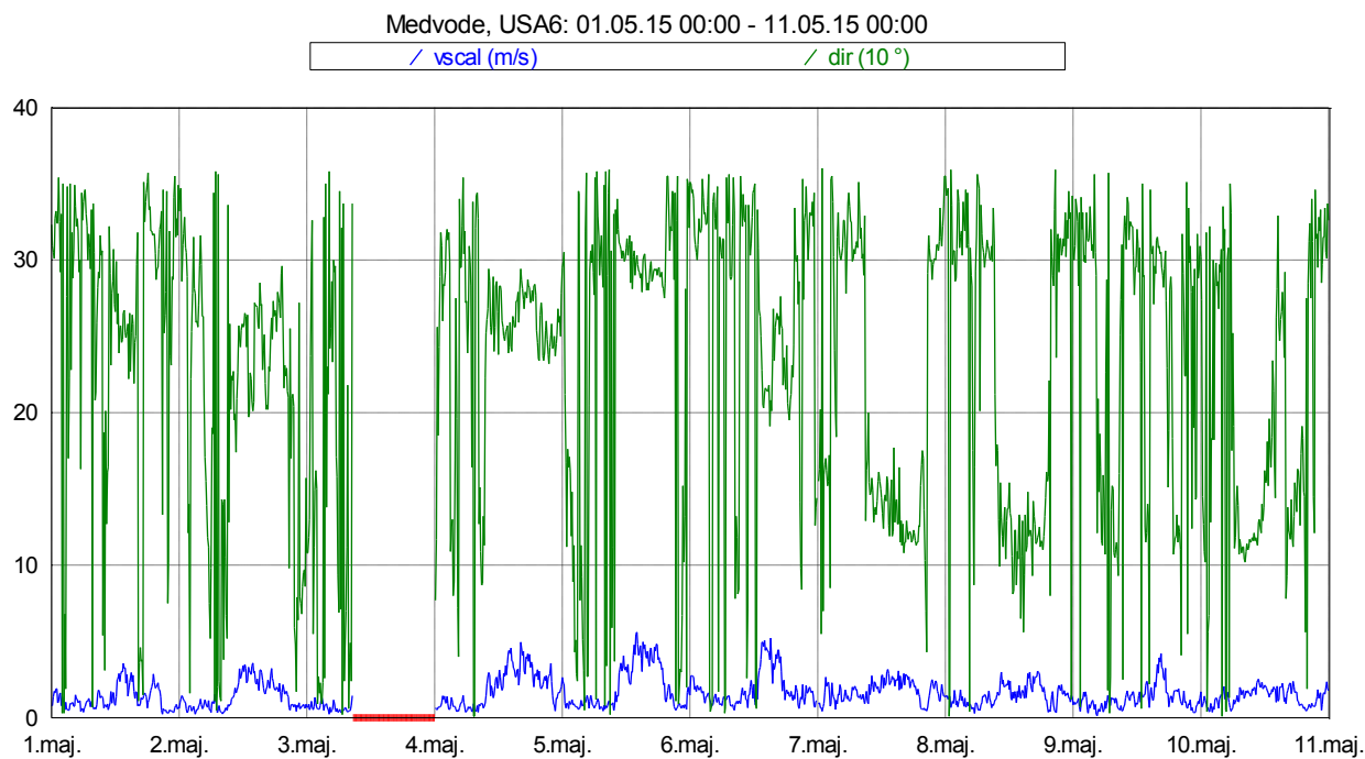
Slika 16: Smer in hitrost vetra med 1. 5. 2015 in 10. 5. 2015.
