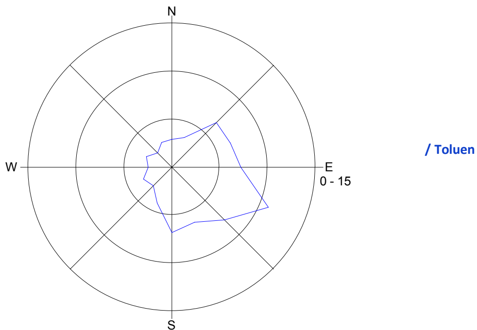
Slika 11: Roža onesnaženost - toluen, maj 2015.
