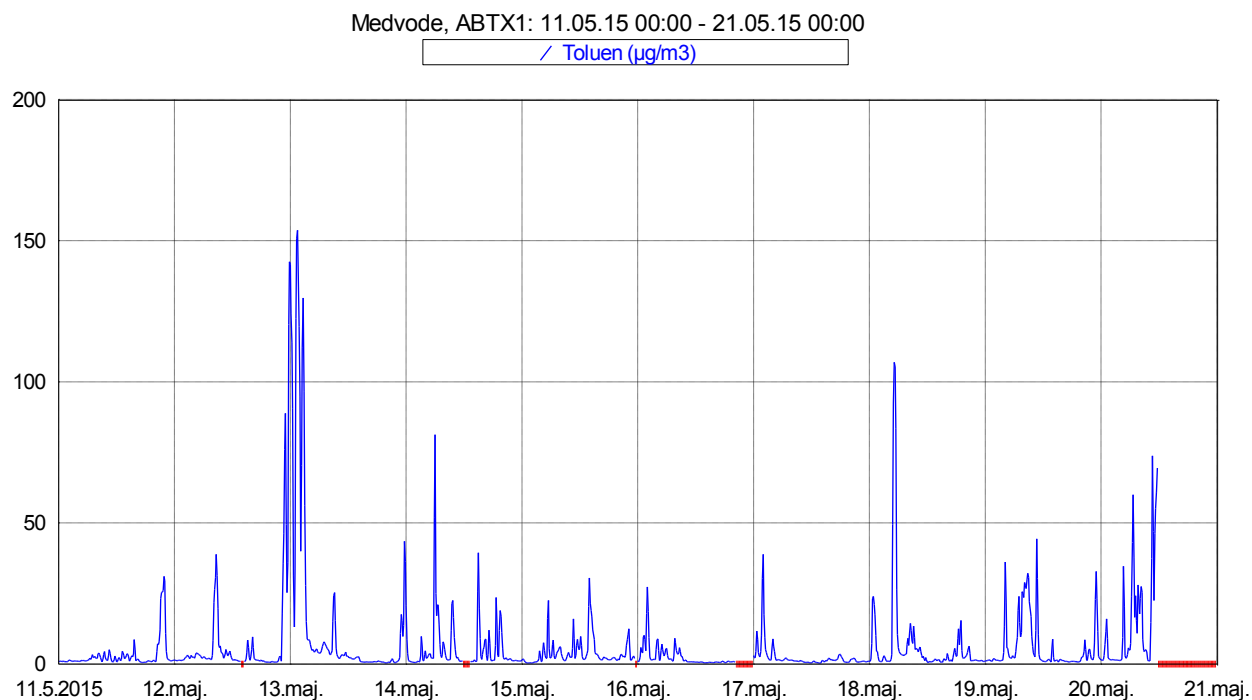
Slika 9: Imisijske koncentracije toluena med 11. 5. 2015 in 20. 5. 2015.
