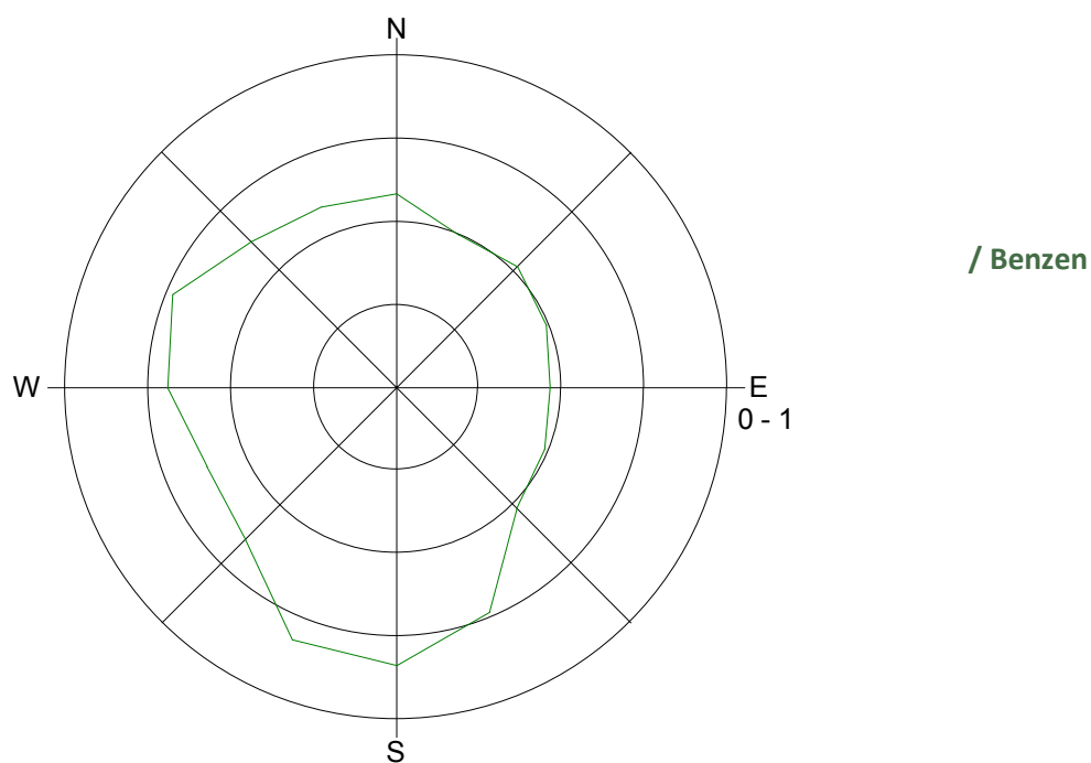
Slika 6: Roža onesnaženosti – benzen, maj 2015.
