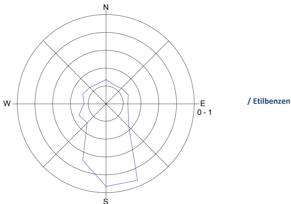
Slika 7: Roža onesnaženosti – etilbenzen, maj 2015.
