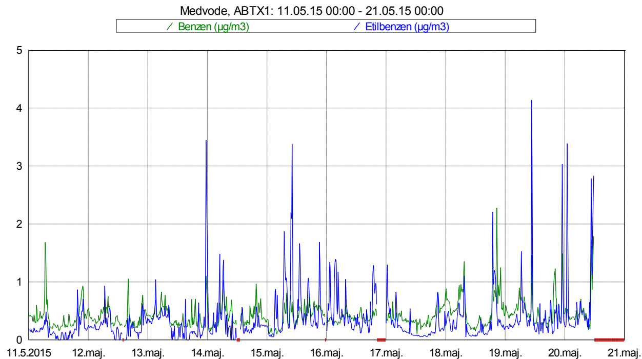
Slika 4: Imisijske koncentracije benzena in etilbenzena med 11. 5. 2015 in 20. 5. 2015.
