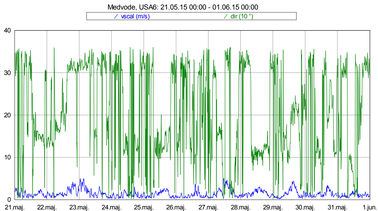
Slika 18: Smer in hitrost vetra med 21. 5. 2015 in 31. 5. 2015.
