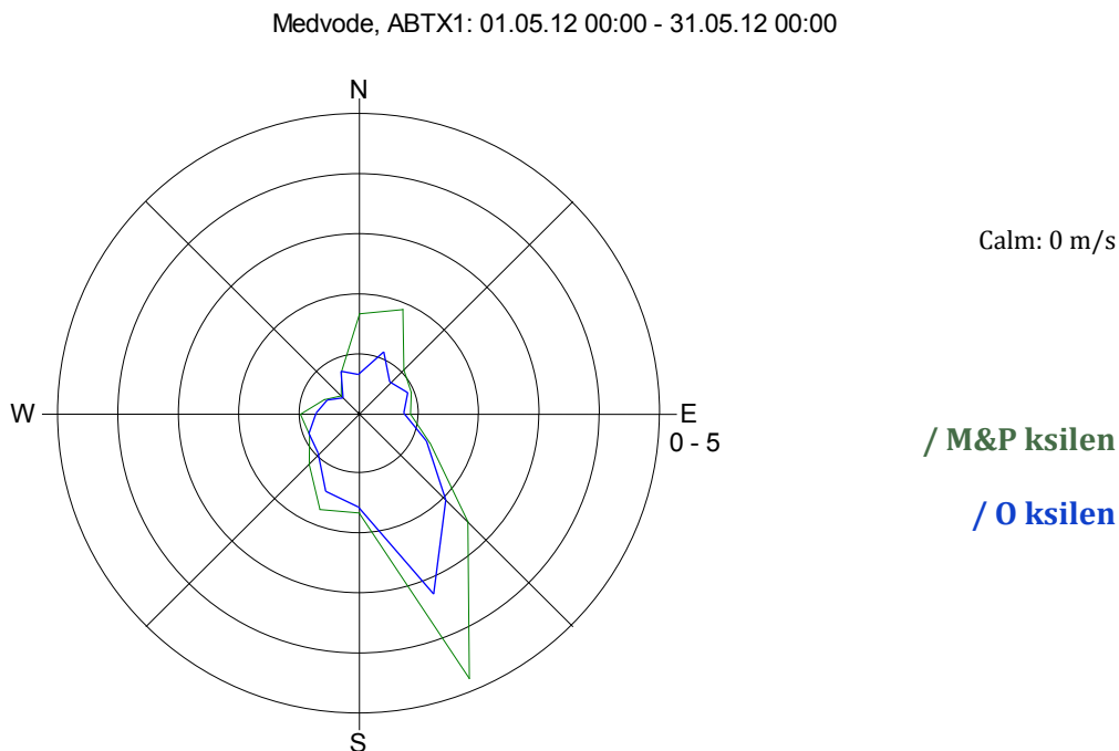
Slika 14: Roža onesnaženosti - M & P ksilen in O ksilen, maj 2012.
