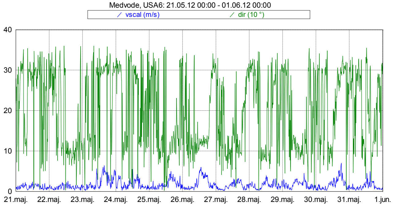
Slika 17: Smer in hitrost vetra med 21. 5. 2012 in 31. 5. 2012.
