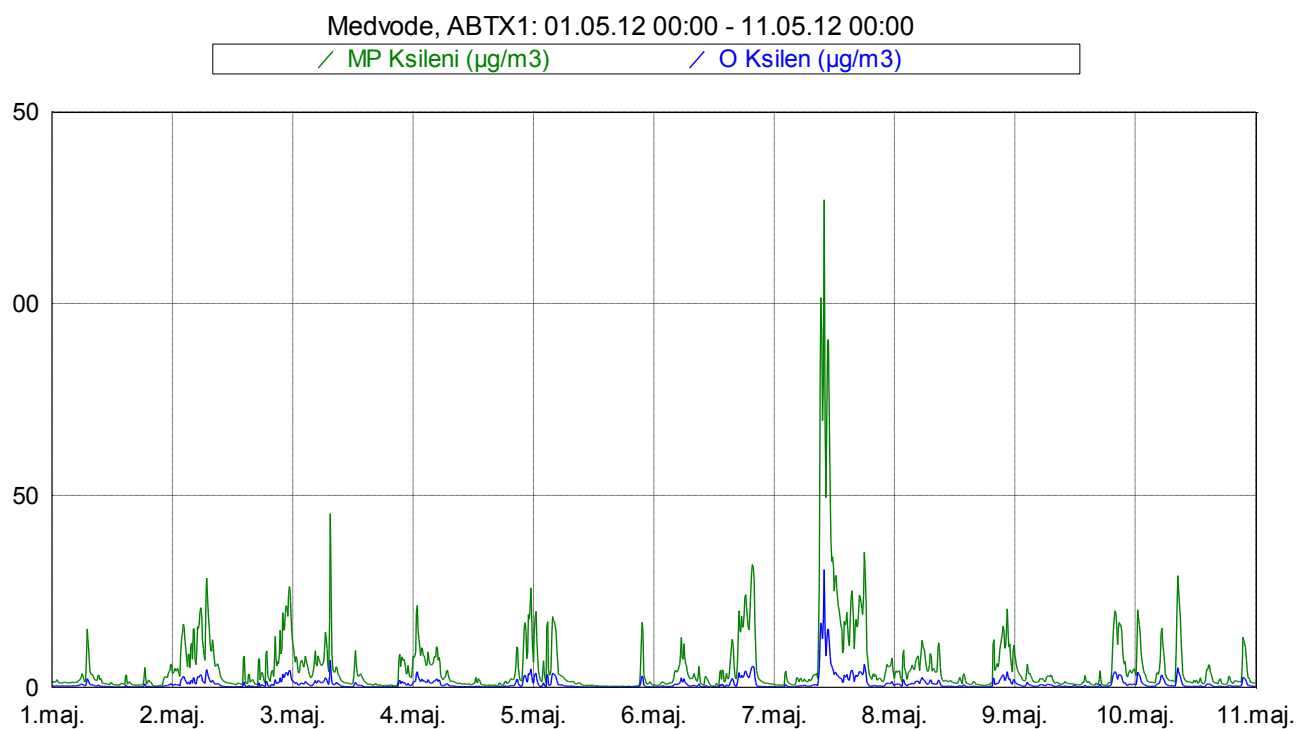
Slika 11: Imisijske koncentracije M&P in O ksilena med 1. 5. 2012 in 10. 5. 2012.
