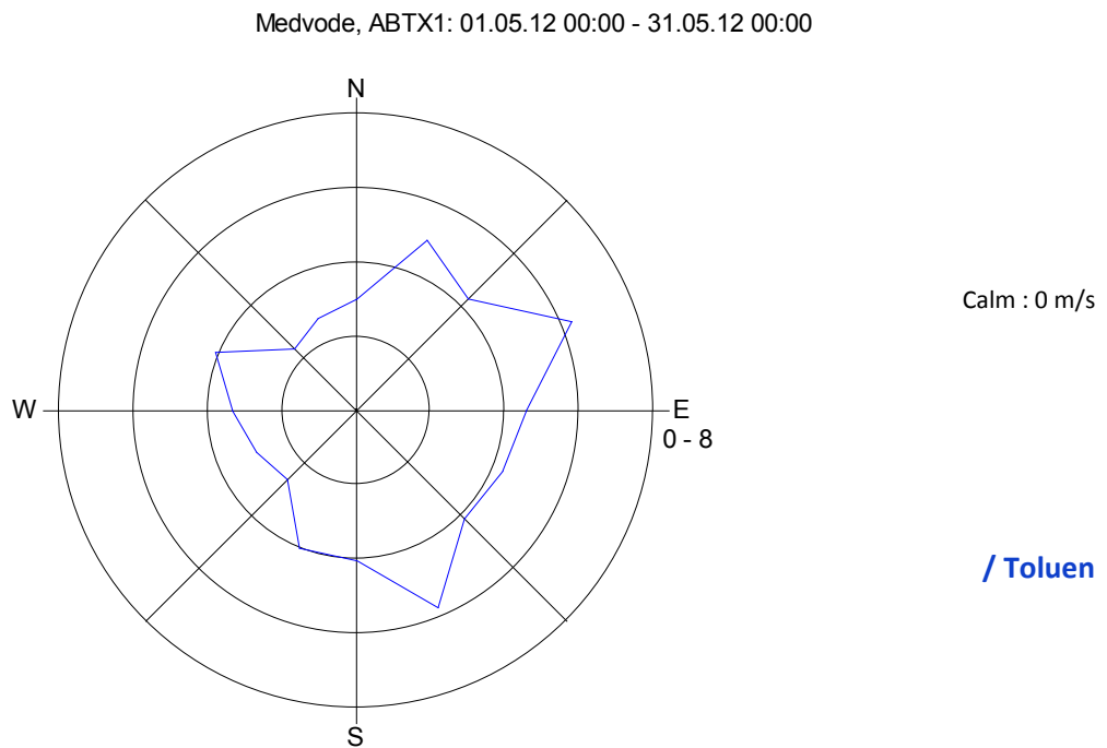
Slika 10: Roža onesnaženost - toluen, maj 2012.
