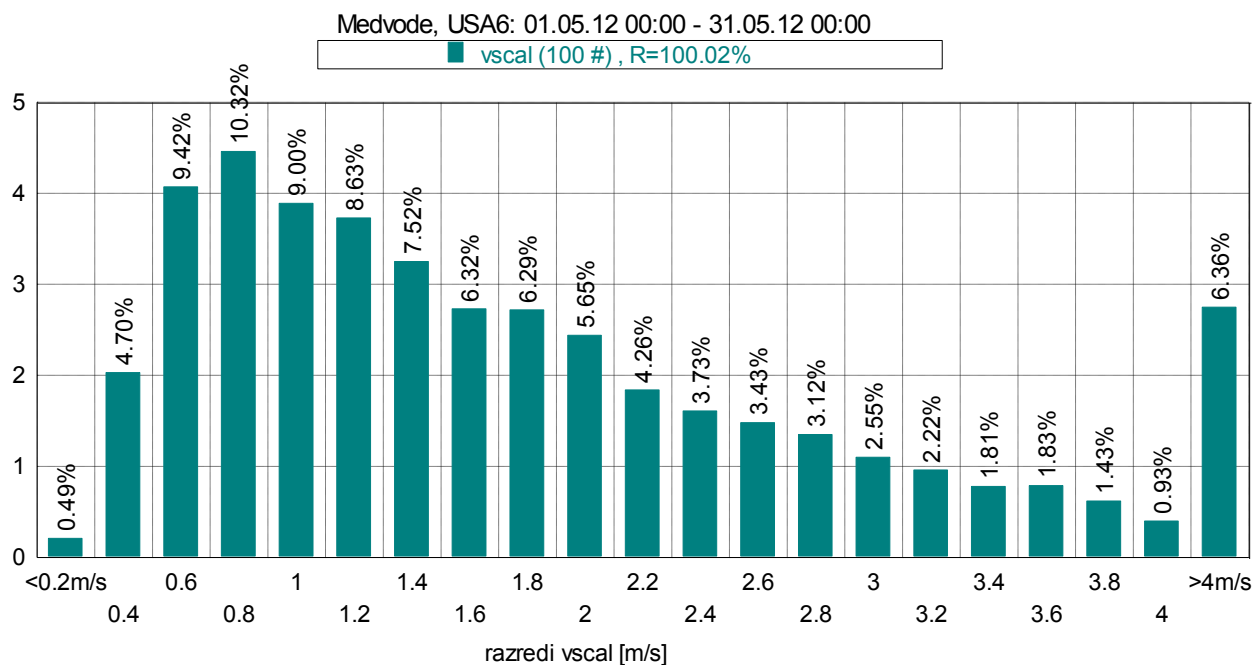
Slika 19: Frekvenčna porazdelitev po hitrosti vetra, maj 2012.
