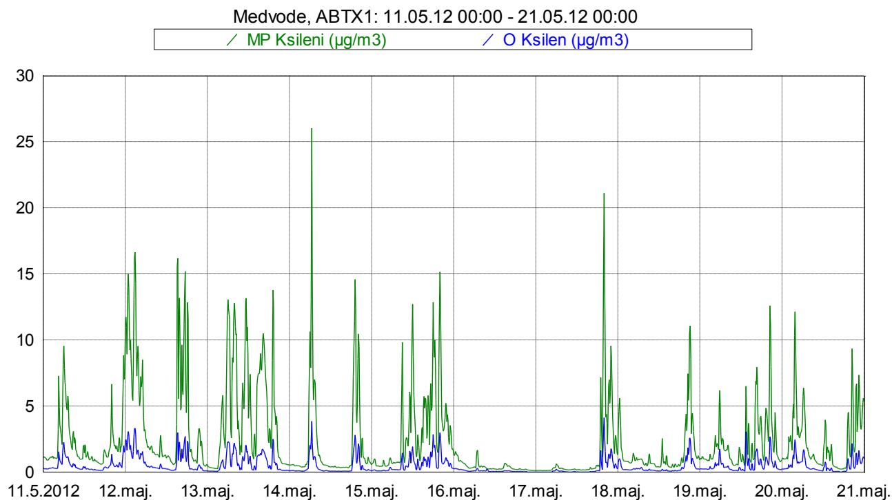
Slika 12: Imisijske koncentracije M&P in O ksilena med 11. 5. 2012 in 20. 5. 2012.
