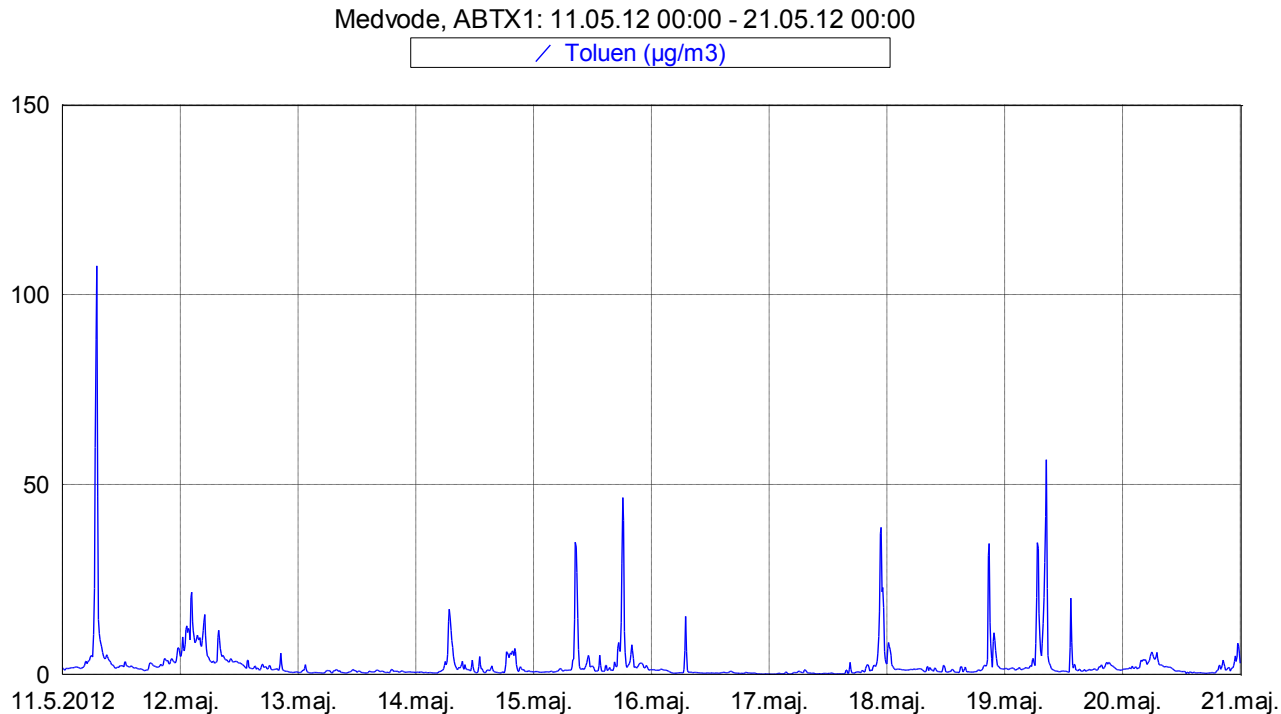
Slika 8: Imisijske koncentracije toluena med 11. 5. 2012 in 20. 5. 2012.
