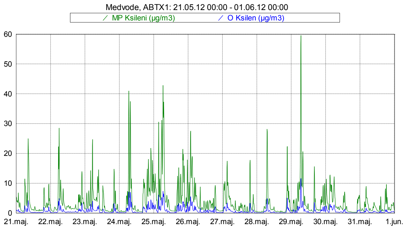
Slika 13: Imisijske koncentracije M&P in O ksilena med 21. 5. 2012 in 31. 5. 2012.
