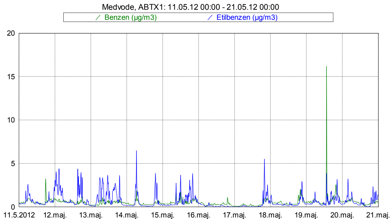
Slika 4: Imisijske koncentracije benzena in etilbenzena med 11. 5. 2012 in 20. 5. 2012.
