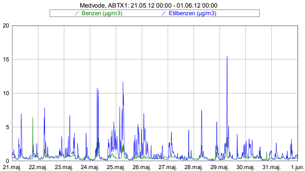
Slika 5: Imisijske koncentracije benzena in etilbenzena med 21. 5. 2012 in 31. 5. 2012.
