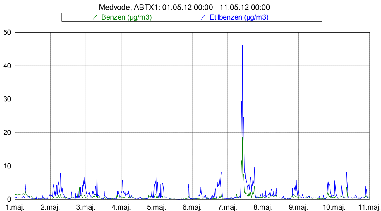
Slika 3: Imisijske koncentracije benzena in etilbenzena med vključno 1. 5. 2012 in 10. 5. 2012.
