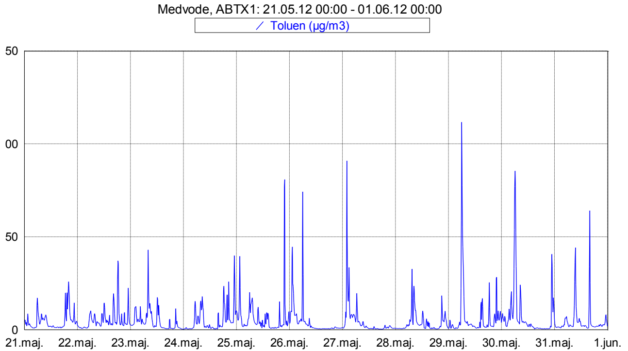
Slika 9: Imisijske koncentracije toluena med 21. 5. 2012 in 31. 5. 2012.
