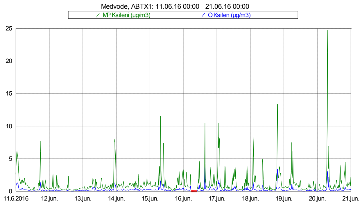
Slika 13: Imisijske koncentracije M&P in O ksilena med 11. 6. 2016 in 20. 6. 2016.
