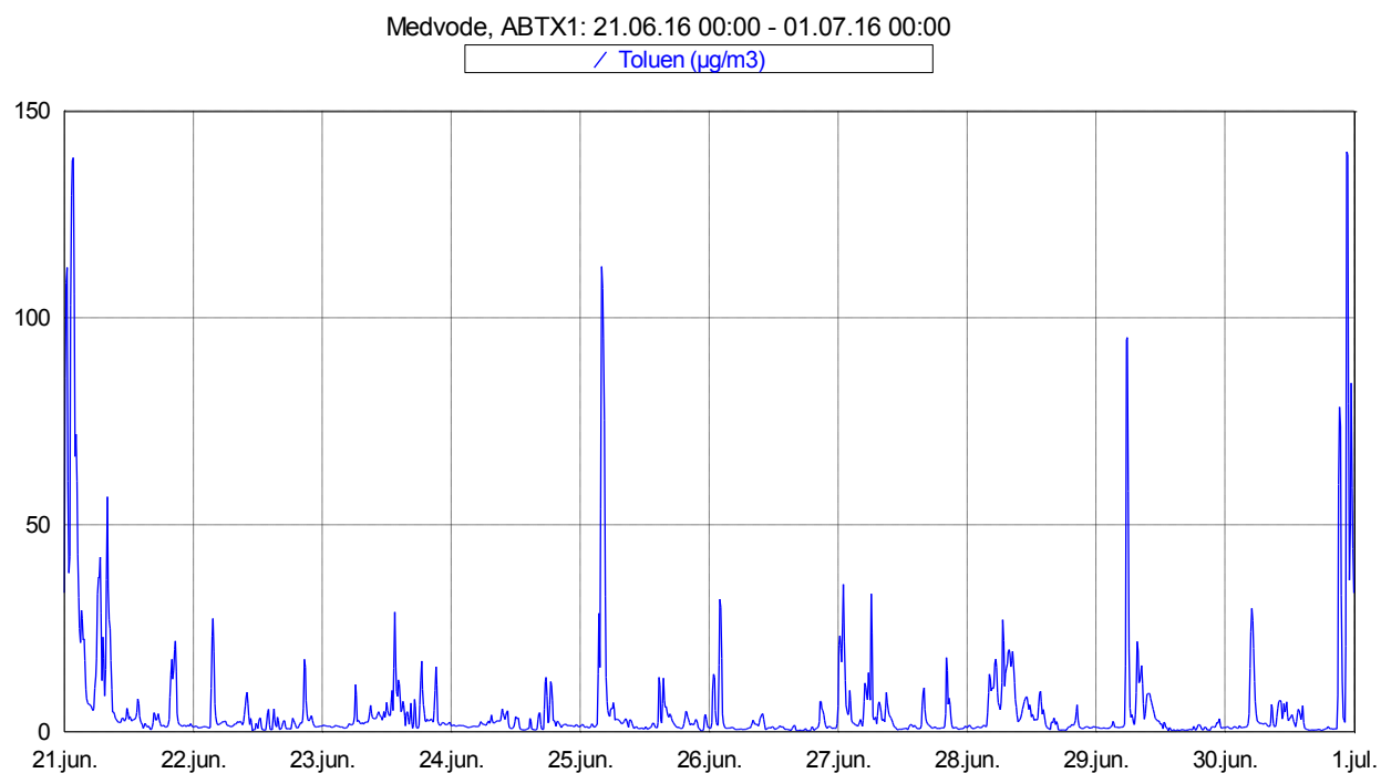
Slika 10: Imisijske koncentracije toluenta med 21. 6. 2016 in 30. 6. 2016.
