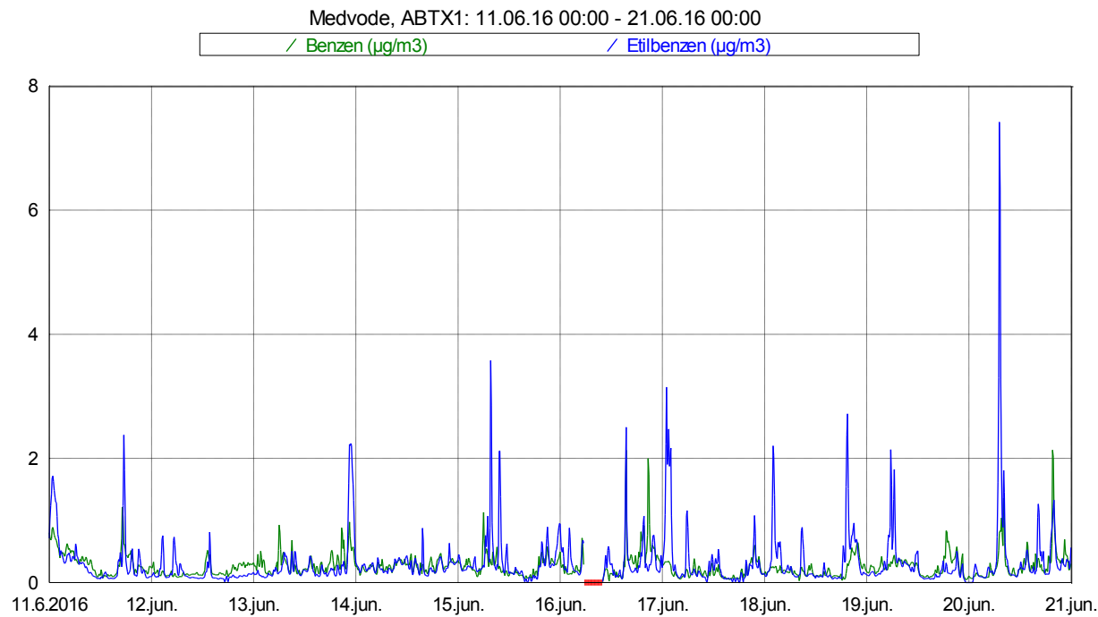
Slika 4: Imisijske koncentracije benzena in etilbenzena med 11. 6. 2016 in 20. 6. 2016.
