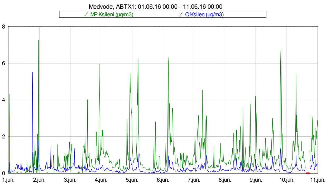
Slika 12: Imisijske koncentracije M&P in O ksilena med vključno 1. 6. 2016 in 10. 6. 2016.
