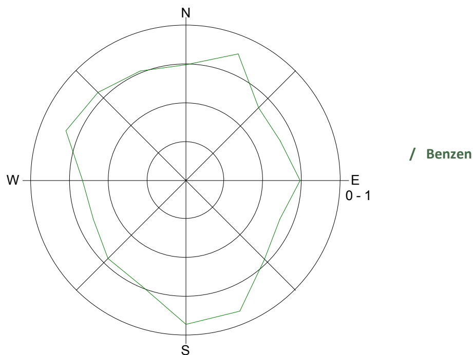
Slika 6: Roža onesnaženosti – benzen, junij 2016.
