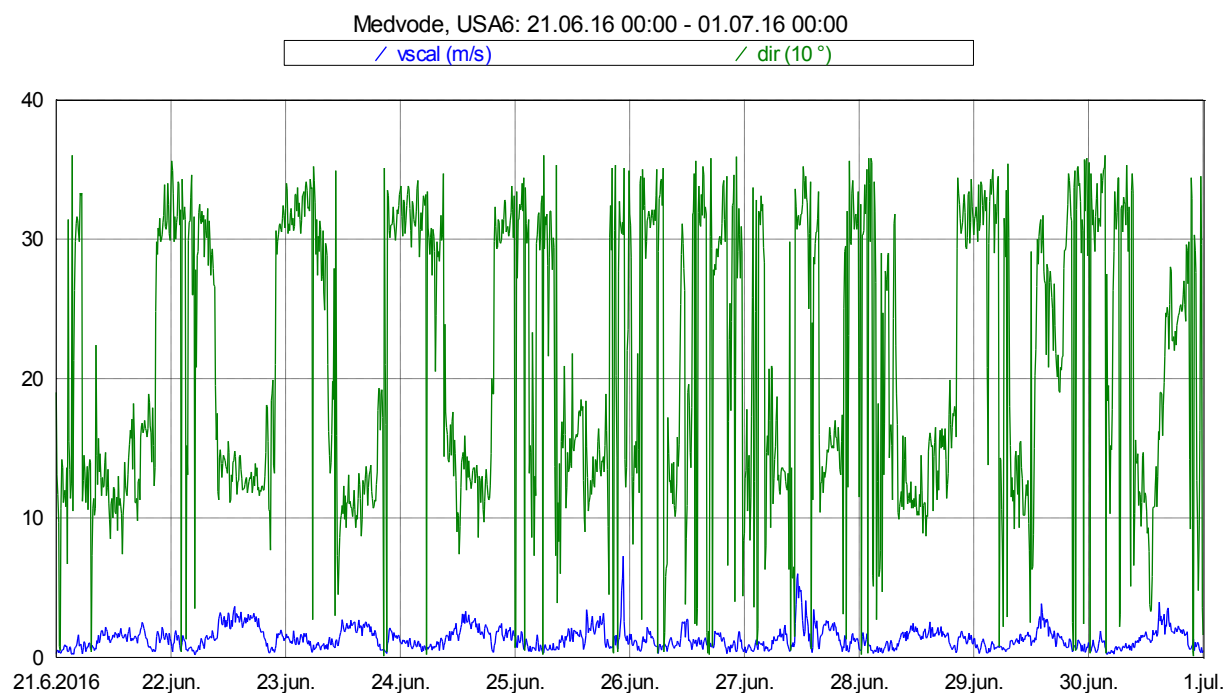
Slika 18: Smer in hitrost vetra med 21. 6. 2016 in 30. 6. 2016.
