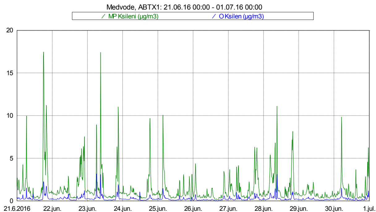
Slika 14: Imisijske koncentracije M&P in O ksilena med 21. 6. 2016 in 30. 6. 2016.
