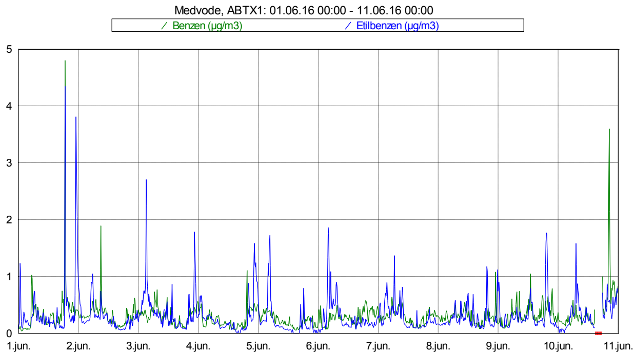
Slika 3: Imisijske koncentracije benzena in etilbenzena med vključno 1. 6. 2016 in 10. 6. 2016.
