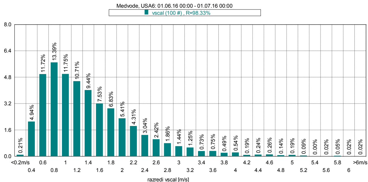
Slika 20: Frekvenčna porazdelitev po hitrosti vetra, junij 2016.
