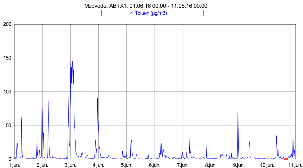
Slika 8: Imisijske koncentracije toluena med vključno 1. 6. 2016 in 10. 6. 2016.
