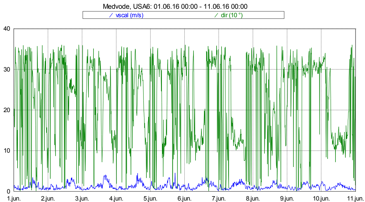
Slika 16: Smer in hitrost vetra med 1. 6. 2016 in 10. 6. 2016.
