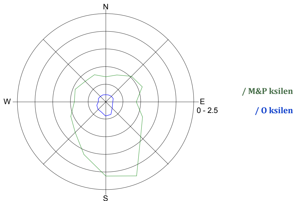
Slika 15: Roža onesnaženosti - M & P ksilen in O ksilen, junij 2016.
