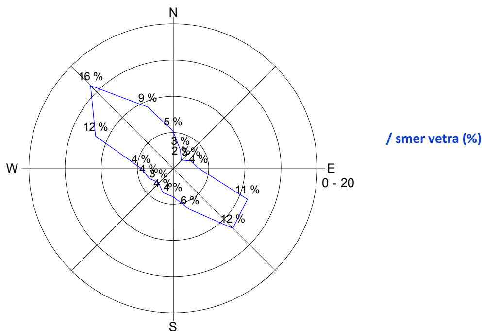
Slika 19: Roža vetrov, junij 2016.
