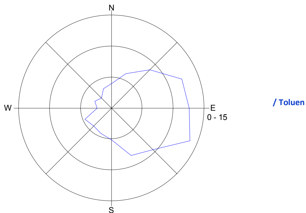
Slika 11: Roža onesnaženost - toluen, junij 2016.
