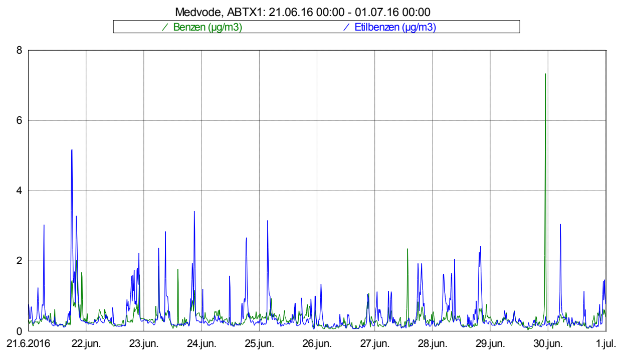
Slika 5: Imisijske koncentracije benzena in etilbenzena med 21. 6. 2016 in 31. 6. 2016.
