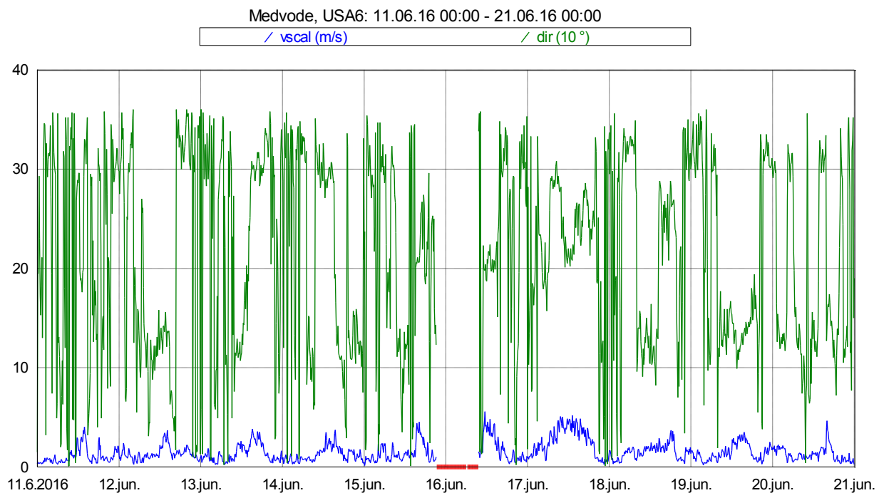
Slika 17: Smer in hitrost vetra med 11. 6. 2016 in 20. 6. 2016.
