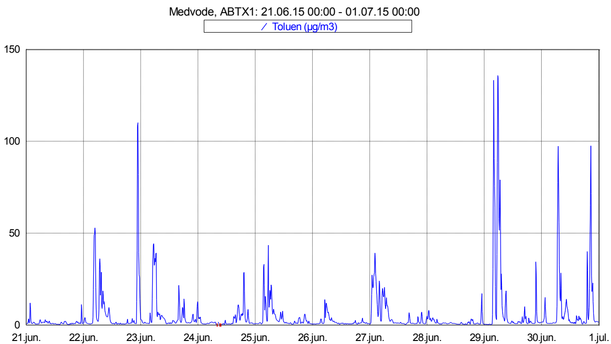
Slika 10: Imisijske koncentracije toluenta med 21. 6. 2015 in 30. 6. 2015.
