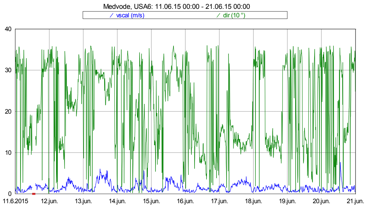
Slika 17: Smer in hitrost vetra med 11. 6. 2015 in 20. 6. 2015.
