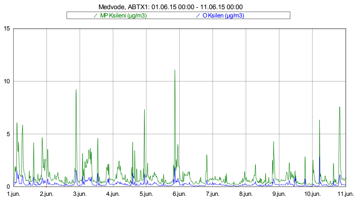
Slika 12: Imisijske koncentracije M&P in O ksilena med vključno 1. 6. 2015 in 10. 6. 2015.
