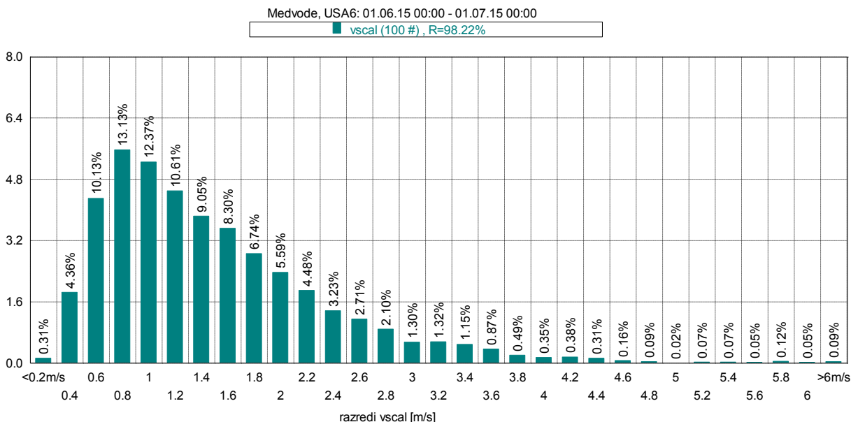
Slika 20: Frekvenčna porazdelitev po hitrosti vetra, junij 2015.
