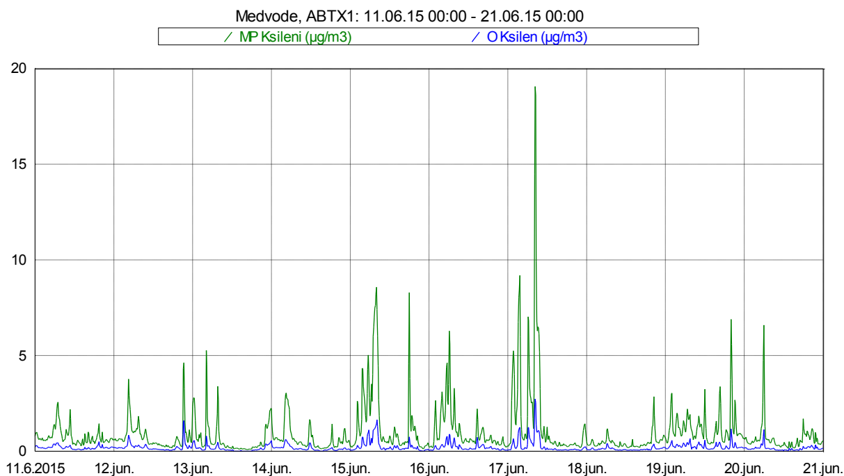
Slika 13: Imisijske koncentracije M&P in O ksilena med 11. 6. 2015 in 20. 6. 2015.
