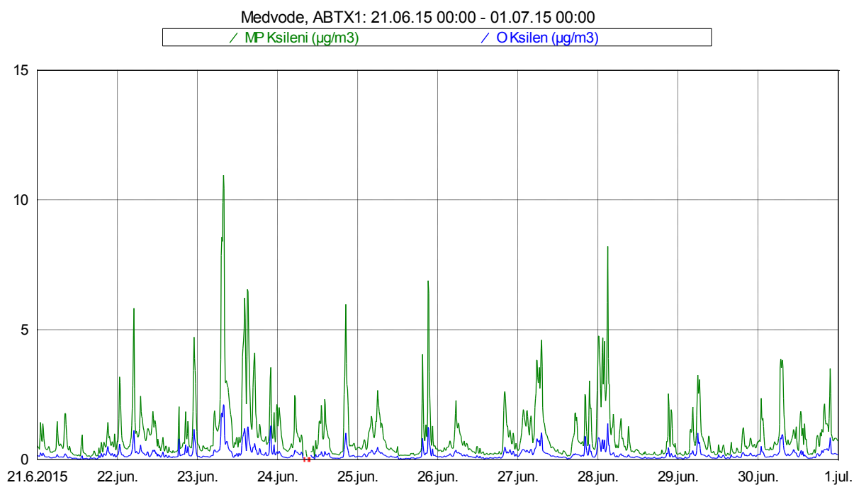
Slika 14: Imisijske koncentracije M&P in O ksilena med 21. 6. 2015 in 30. 6. 2015.
