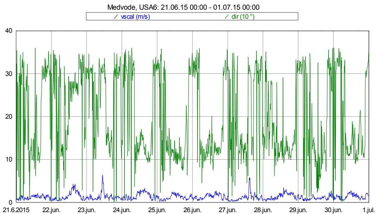
Slika 18: Smer in hitrost vetra med 21. 6. 2015 in 30. 6. 2015.
