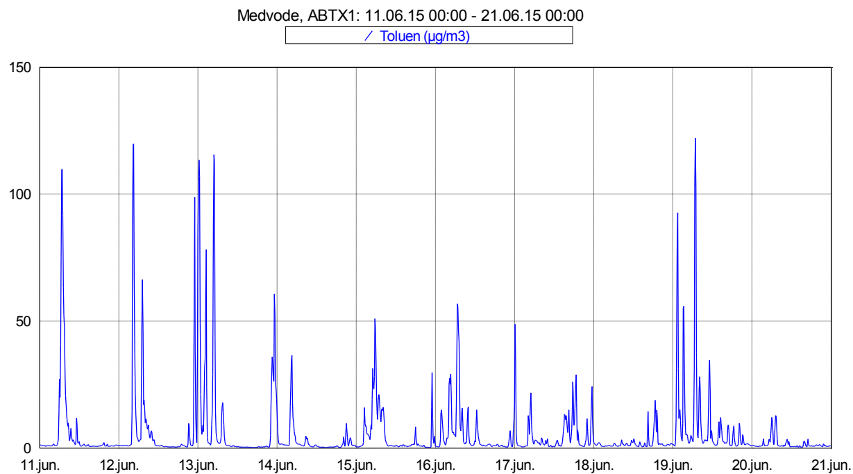
Slika 9: Imisijske koncentracije toluena med 11. 6. 2015 in 20. 6. 2015.
