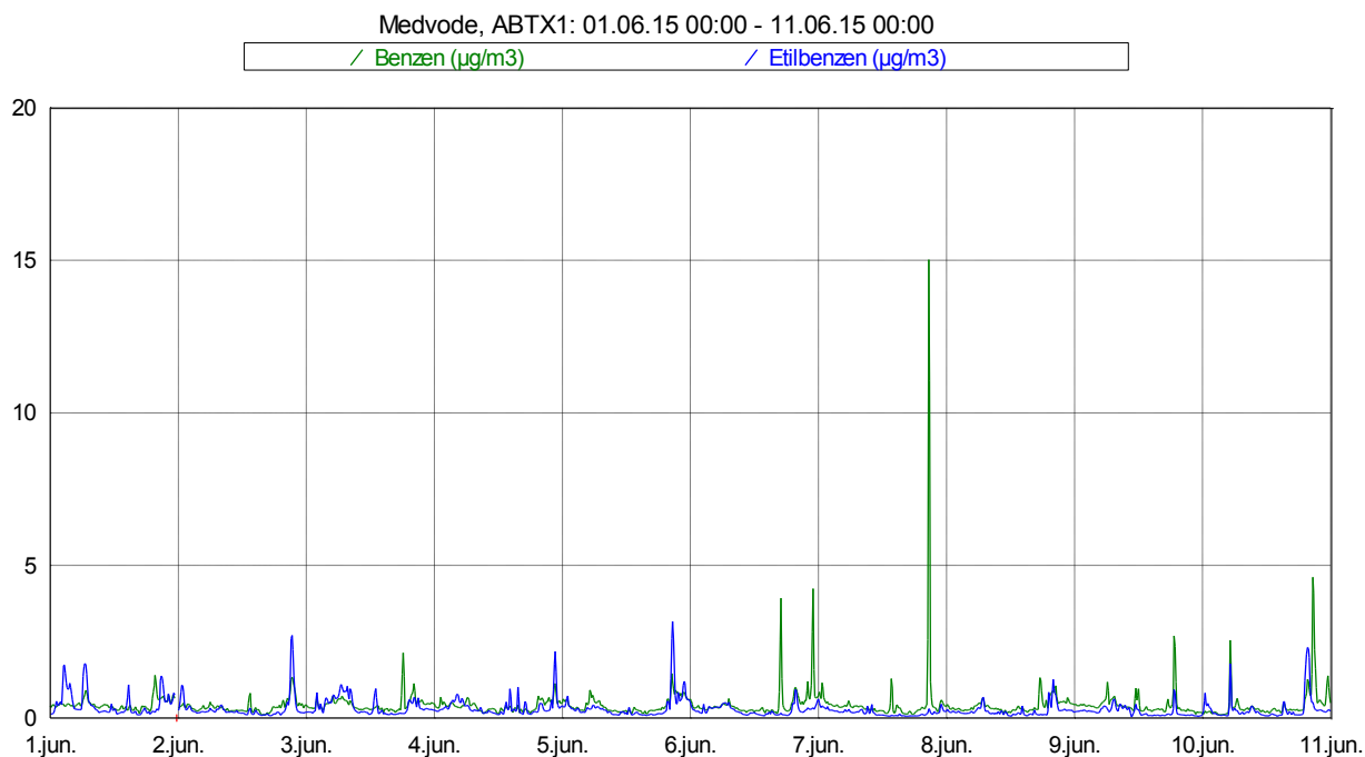
Slika 3: Imisijske koncentracije benzena in etilbenzena med vključno 1. 6. 2015 in 10. 6. 2015.
