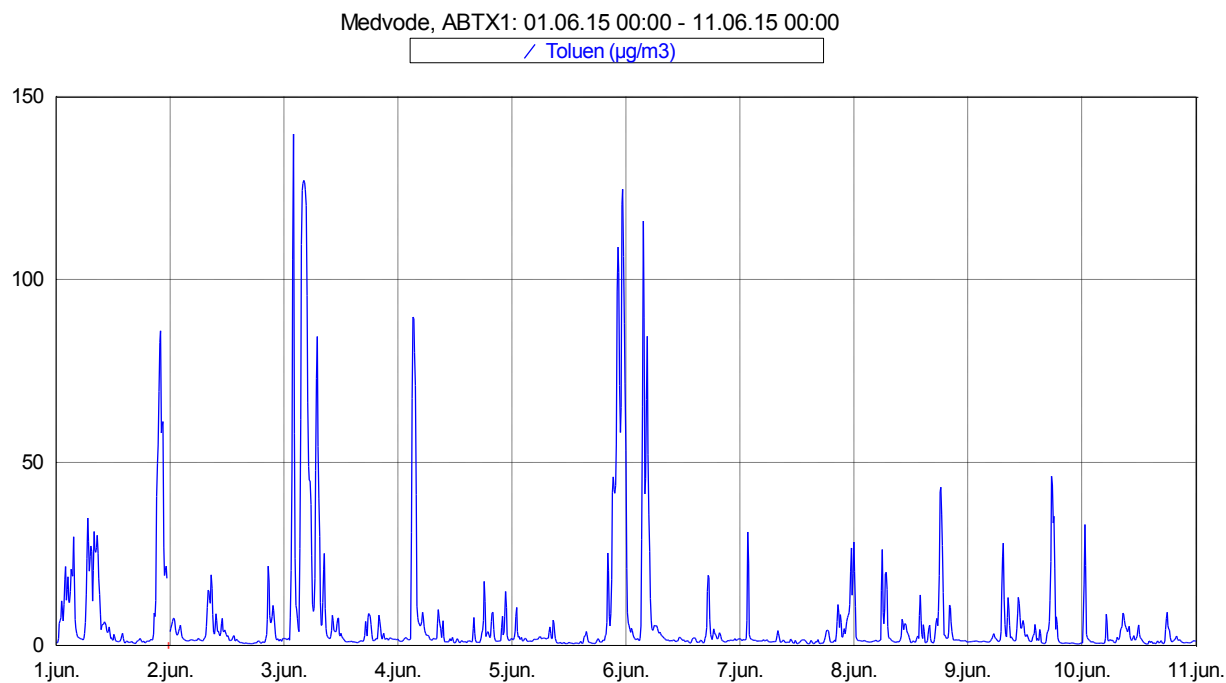
Slika 8: Imisijske koncentracije toluena med vključno 1. 6. 2015 in 10. 6. 2015.
