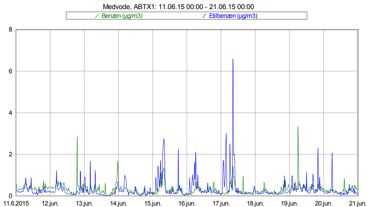
Slika 4: Imisijske koncentracije benzena in etilbenzena med 11. 6. 2015 in 20. 6. 2015.
