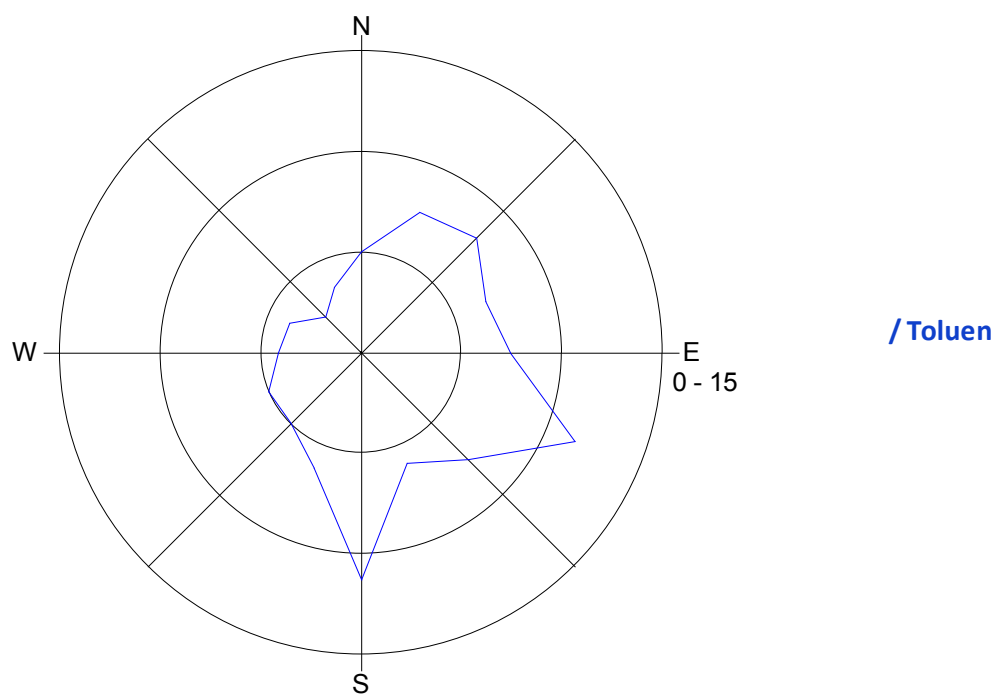
Slika 11: Roža onesnaženost - toluen, junij 2015.
