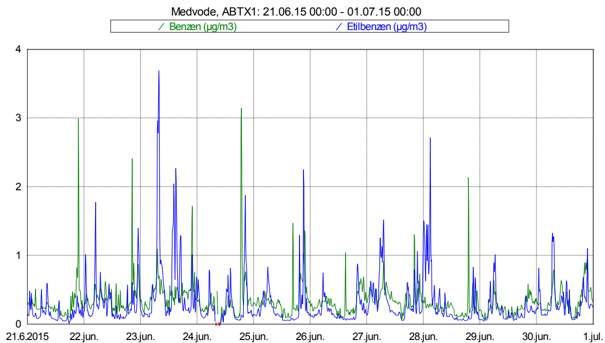
Slika 5: Imisijske koncentracije benzena in etilbenzena med 21. 6. 2015 in 30. 6. 2015.
