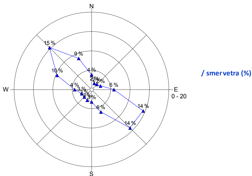
Slika 19: Roža vetrov, junij 2015.
