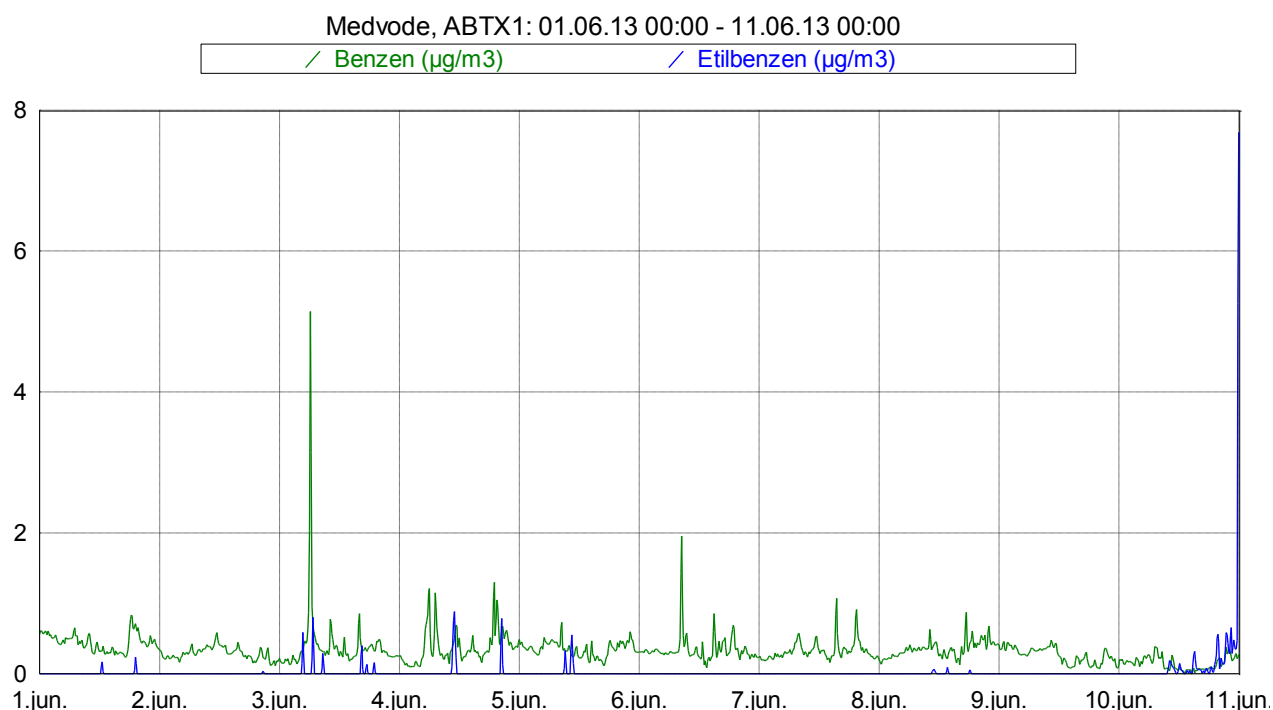
Slika 3: Imisijske koncentracije benzena in etilbenzena med vključno 1. 6. 2013 in 10. 6. 2013.
