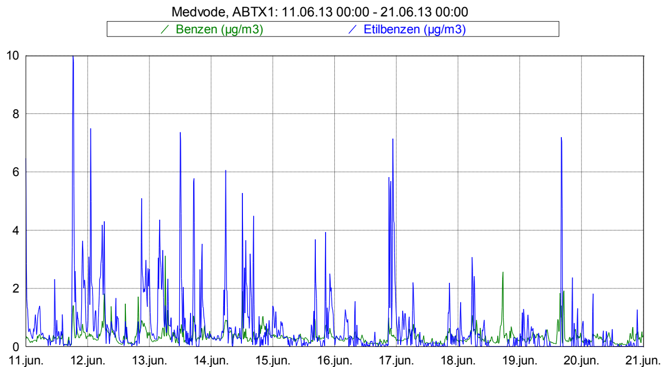
Slika 4: Imisijske koncentracije benzena in etilbenzena med 11. 6. 2013 in 20. 6. 2013.
