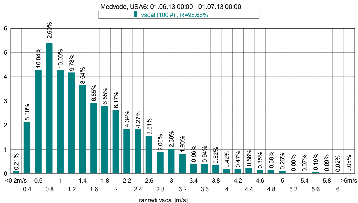
Slika 19: Frekvenčna porazdelitev po hitrosti vetra, junij 2013.
