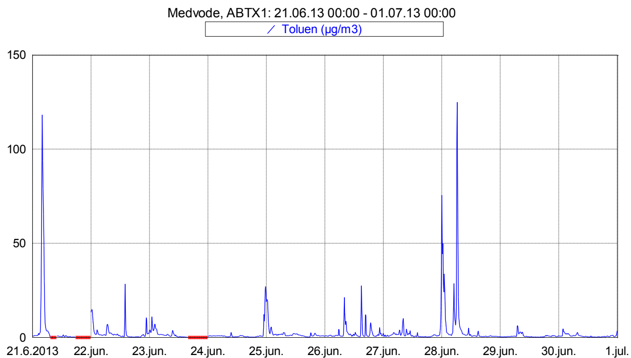
Slika 9: Imisijske koncentracije toluenta med 21. 6. 2013 in 30. 6. 2013.
