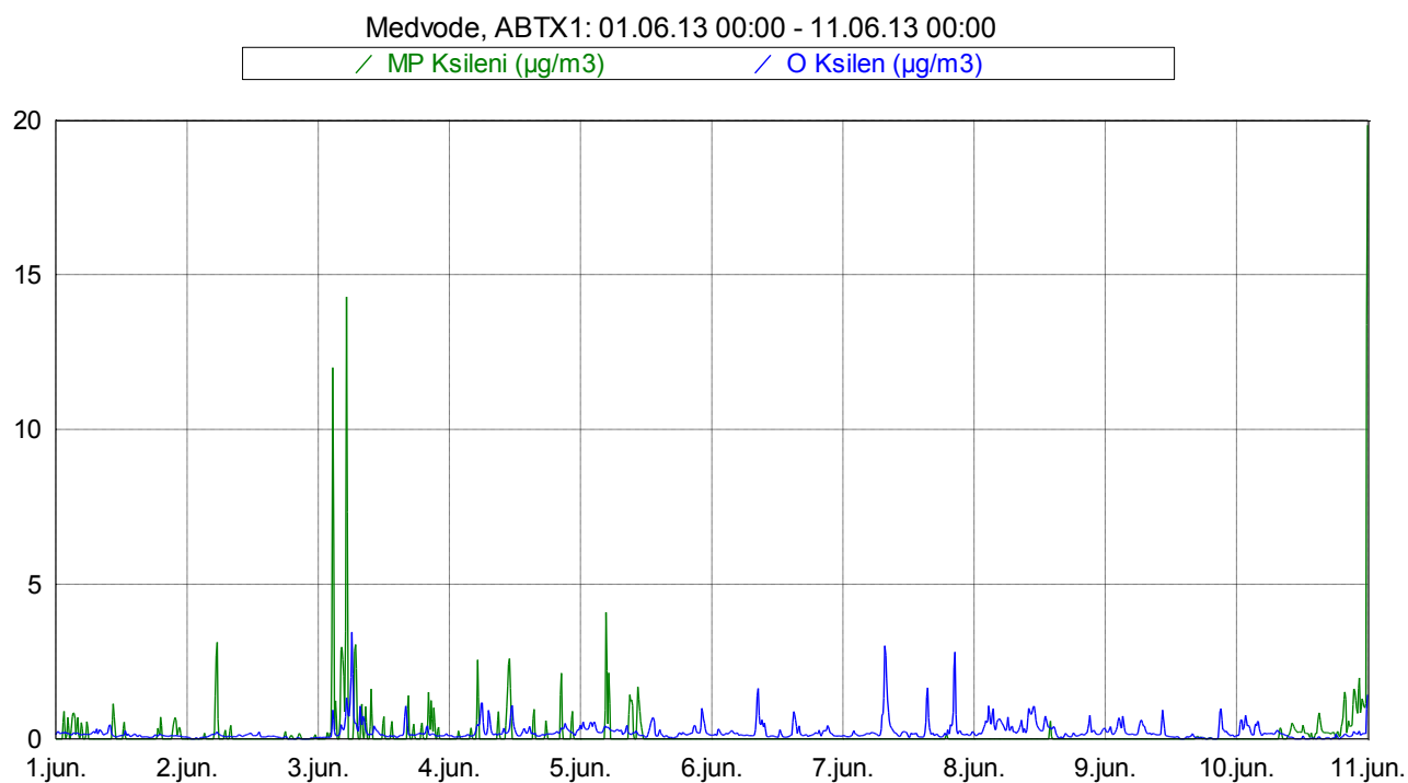
Slika 11: Imisijske koncentracije M&P in O ksilena med vključno 1. 6. 2013 in 10. 6. 2013.
