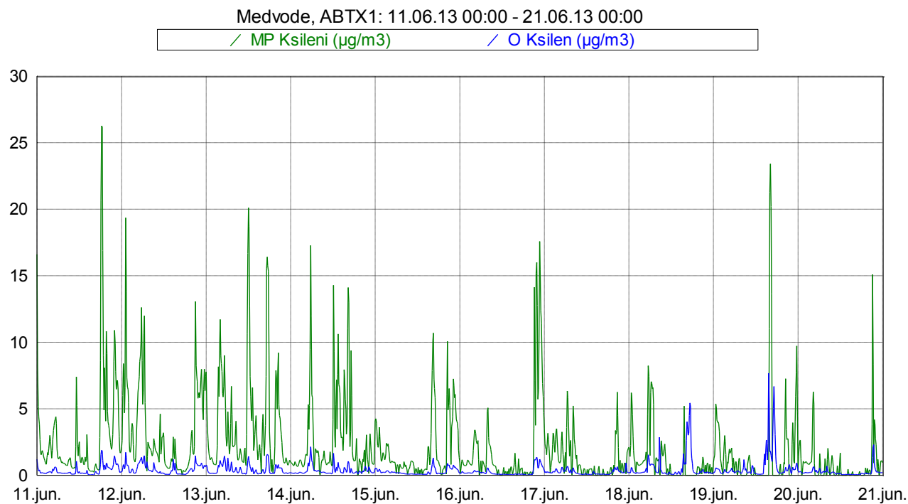
Slika 12: Imisijske koncentracije M&P in O ksilena med 11. 6. 2013 in 20. 6. 2013.
