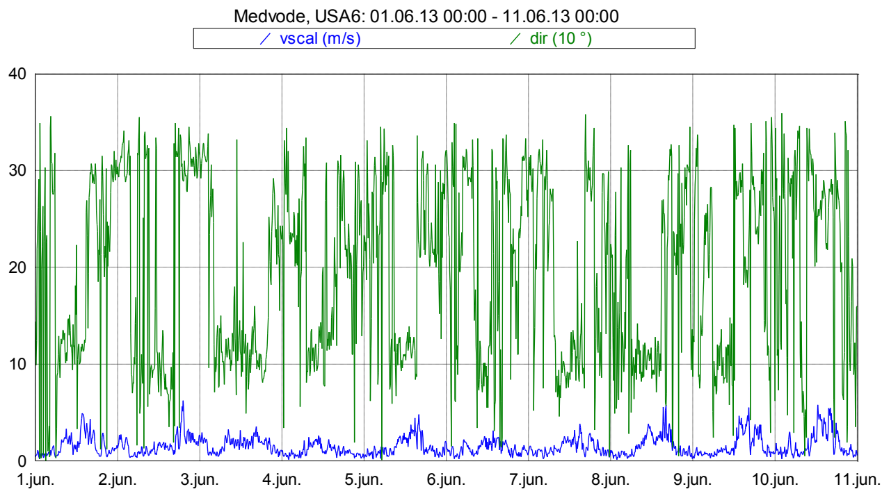
Slika 15: Smer in hitrost vetra med 1. 6. 2013 in 10. 6. 2013.
