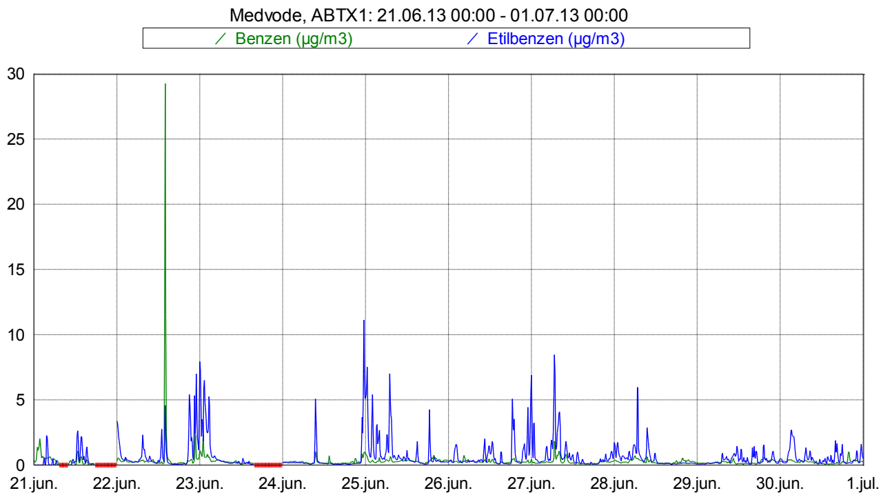
Slika 5: Imisijske koncentracije benzena in etilbenzena med 21. 6. 2013 in 30. 6. 2013.
