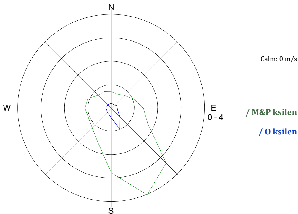
Slika 14: Roža onesnaženosti - M & P ksilen in O ksilen, junij 2013.
