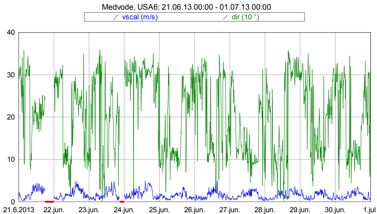
Slika 17: Smer in hitrost vetra med 21. 6. 2013 in 30. 6. 2013.
