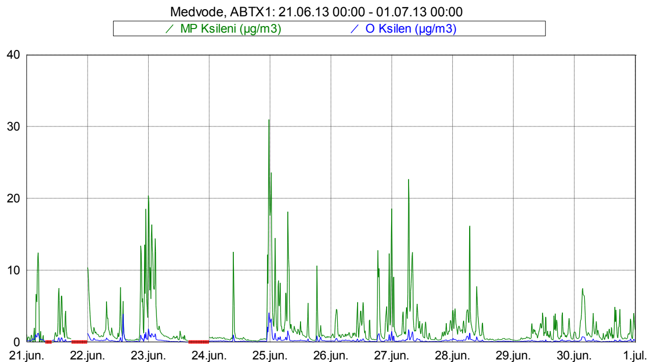
Slika 13: Imisijske koncentracije M&P in O ksilena med 21. 6. 2013 in 30. 6. 2013.
