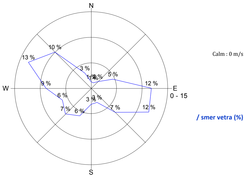
Slika 18: Roža vetrov, junij 2013.
