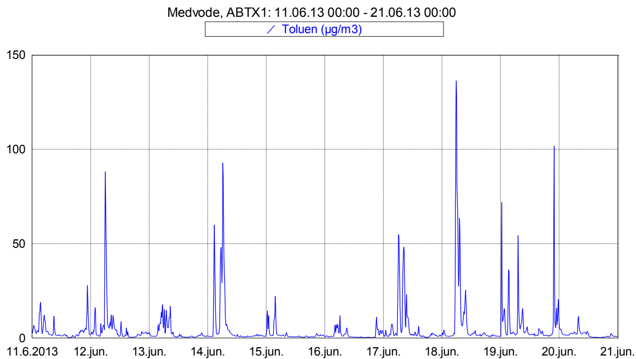
Slika 8: Imisijske koncentracije toluena med 11. 6. 2013 in 20. 6. 2013.
