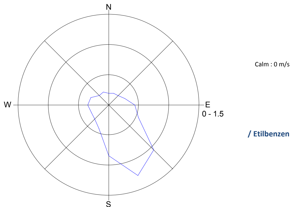
Slika 6: Roža onesnaženosti – benzen (zgoraj) in etilbenzen (spodaj), junij 2013.
