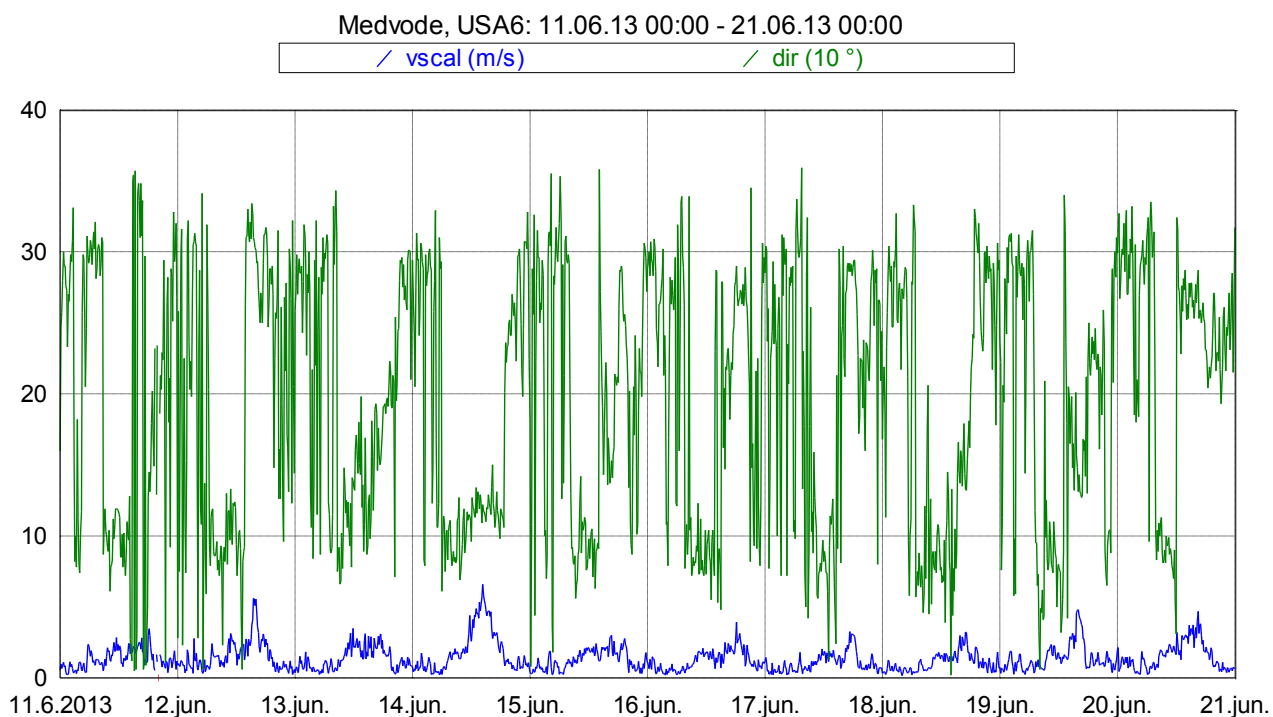
Slika 16: Smer in hitrost vetra med 11. 6. 2013 in 20. 6. 2013.
