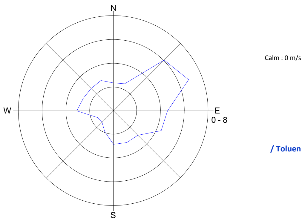
Slika 10: Roža onesnaženost - toluen, junij 2013.
