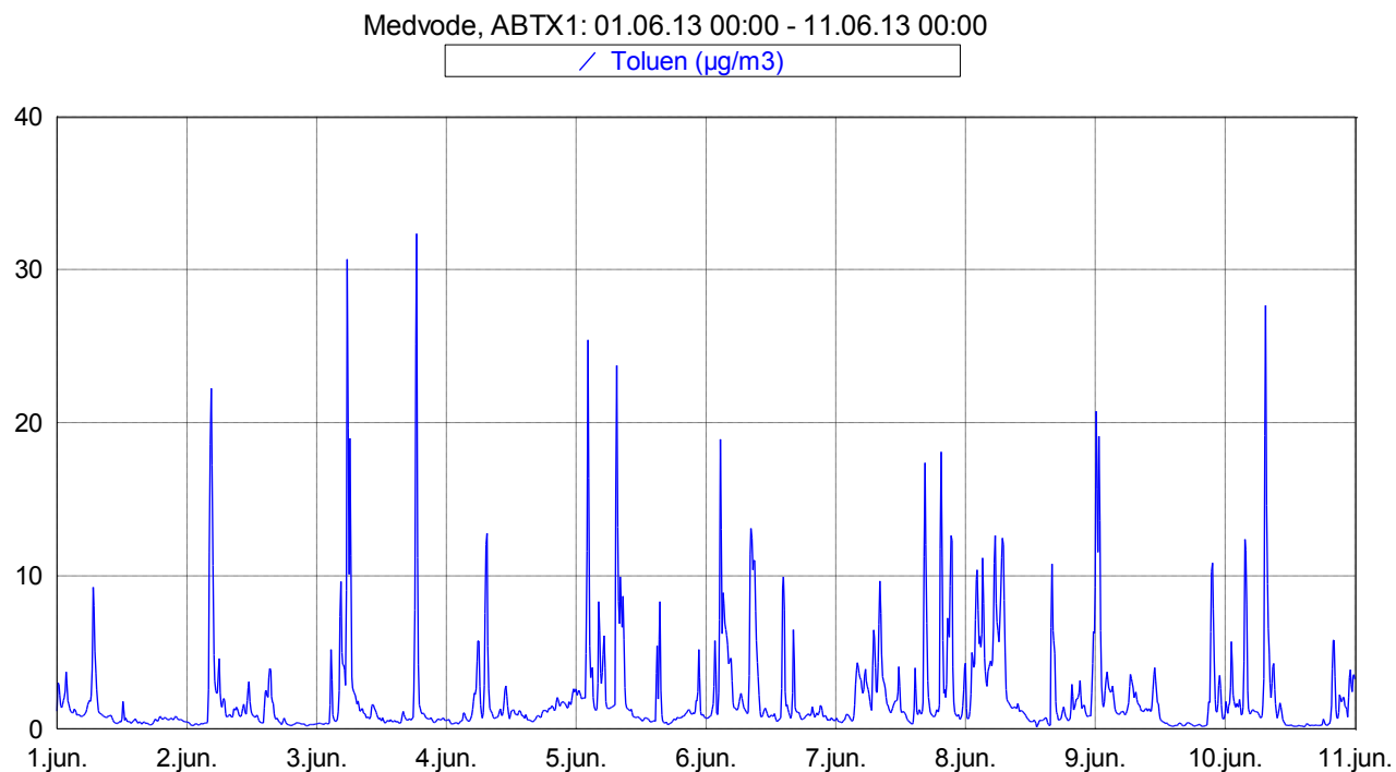
Slika 7: Imisijske koncentracije toluena med vključno 1. 6. 2013 in 10. 6. 2013.
