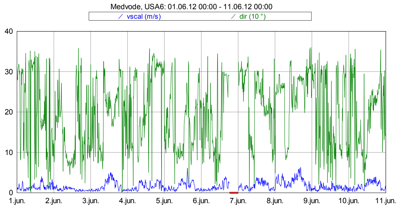
Slika 15: Smer in hitrost vetra med 1. 6. 2012 in 10. 6. 2012.
