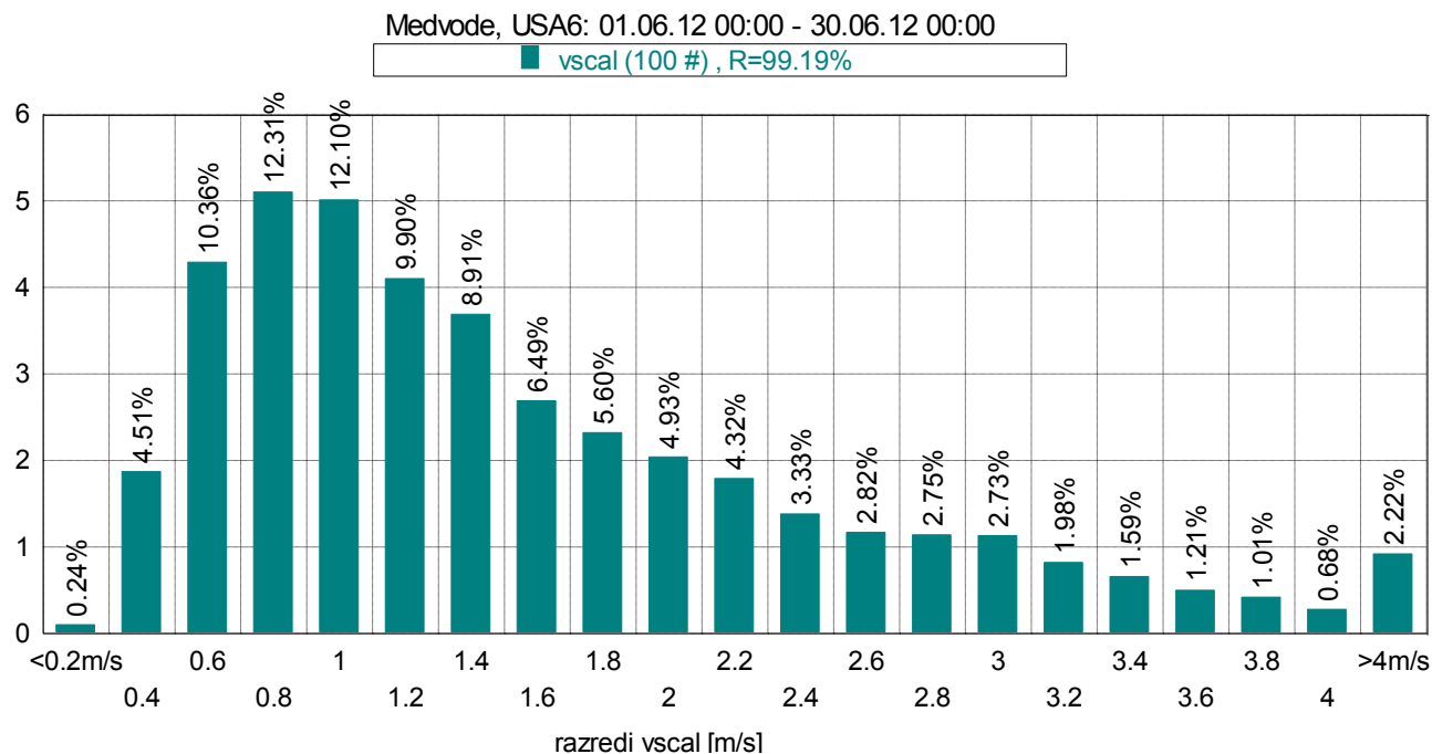
Slika 19: Frekvenčna porazdelitev po hitrosti vetra, junij 2012.
