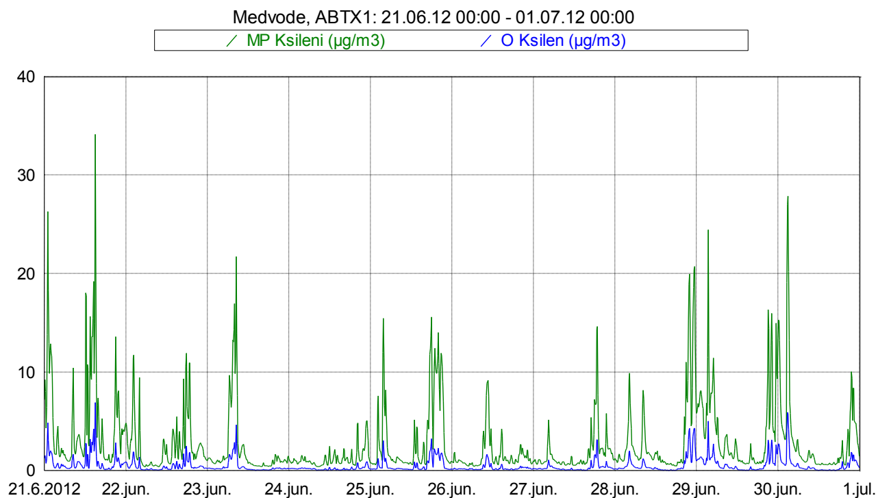
Slika 13: Imisijske koncentracije M&P in O ksilena med 21. 6. 2012 in 30. 6. 2012.
