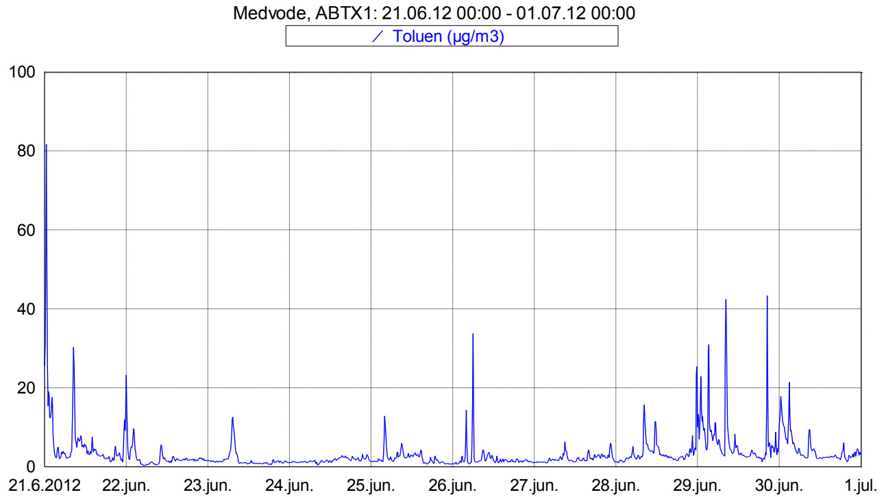
Slika 9: Imisijske koncentracije toluena med 21. 6. 2012 in 30. 6. 2012.
