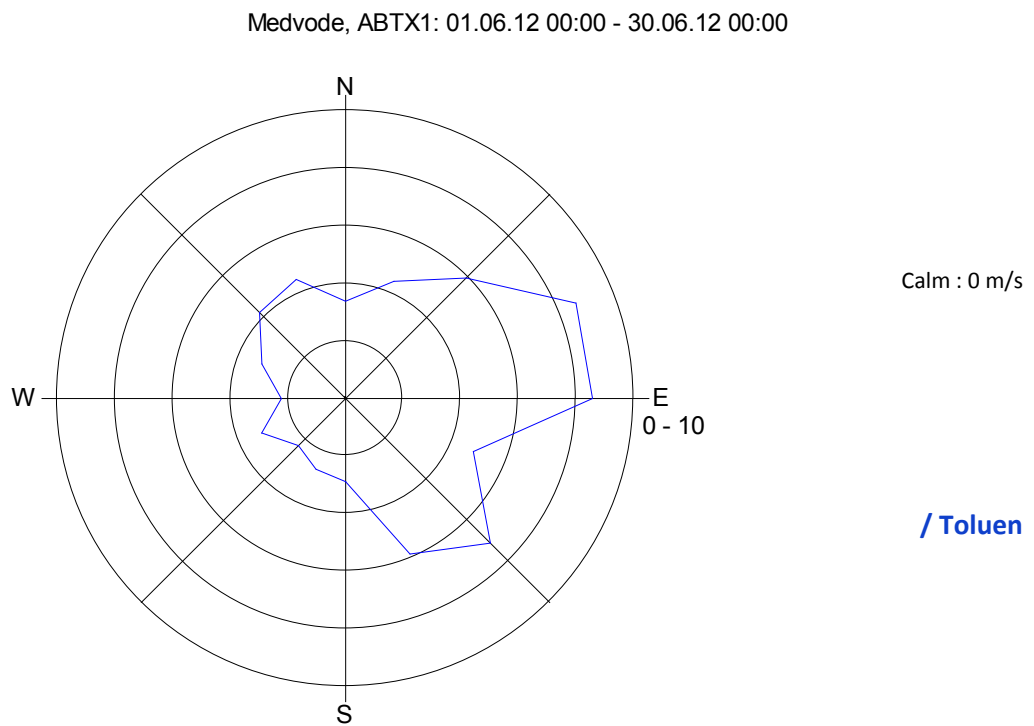
Slika 10: Roža onesnaženost - toluen, junij 2012.
