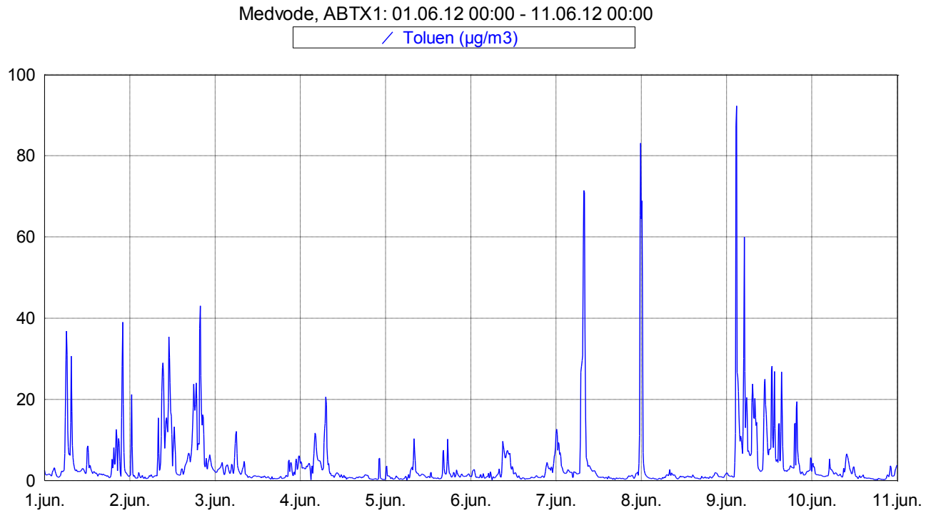
Slika 7: Imisijske koncentracije toluena med 1. 6. 2012 in 10. 6. 2012.
