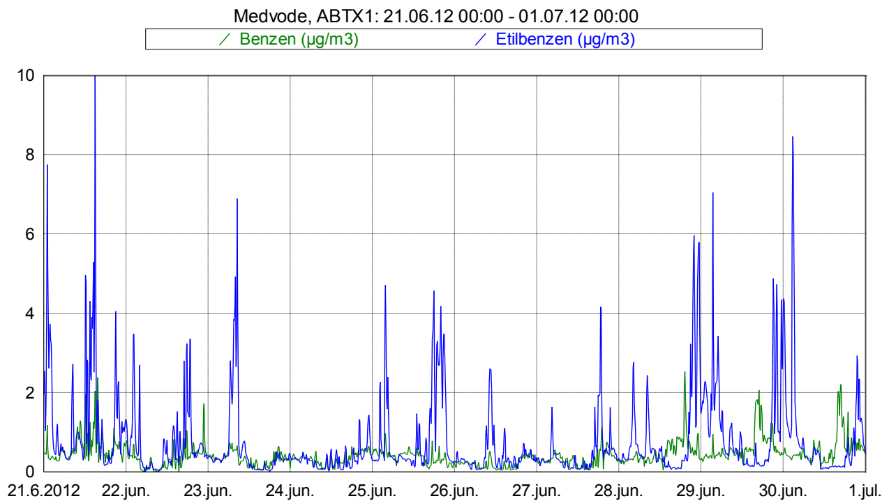
Slika 5: Imisijske koncentracije benzena in etilbenzena med 21. 6. 2012 in 30. 6. 2012.
