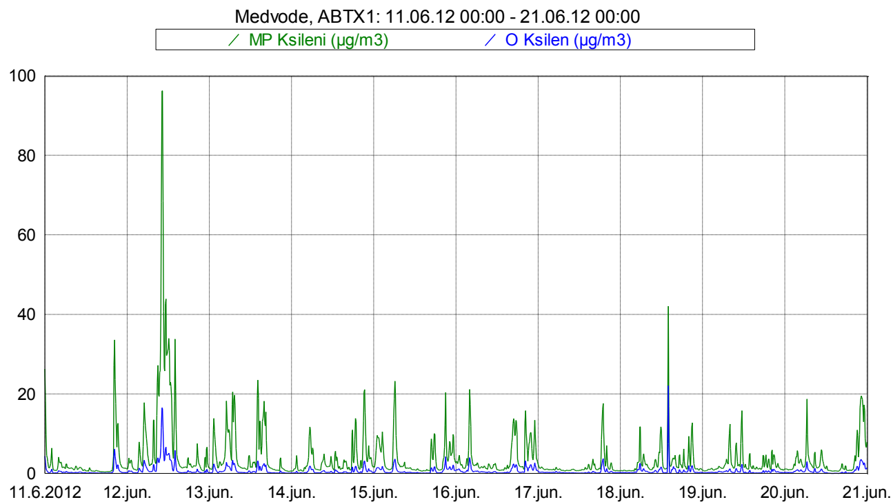
Slika 12: Imisijske koncentracije M&P in O ksilena med 11. 6. 2012 in 20. 6. 2012.
