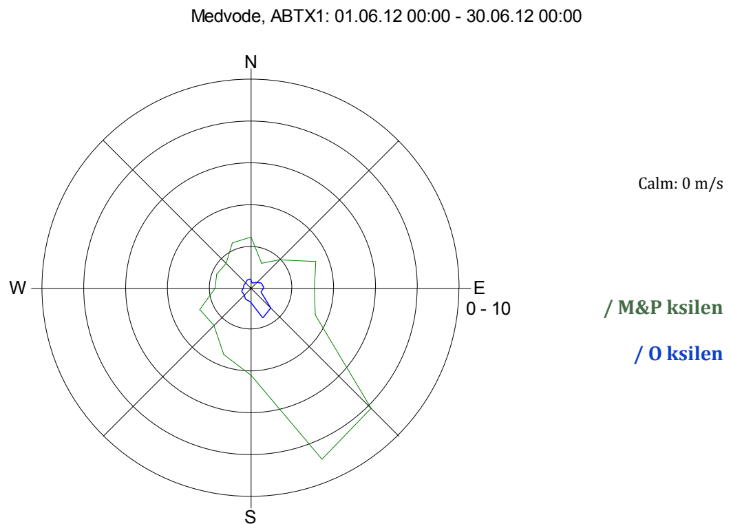
Slika 14: Roža onesnaženosti - M & P ksilen in O ksilen, junij 2012.
