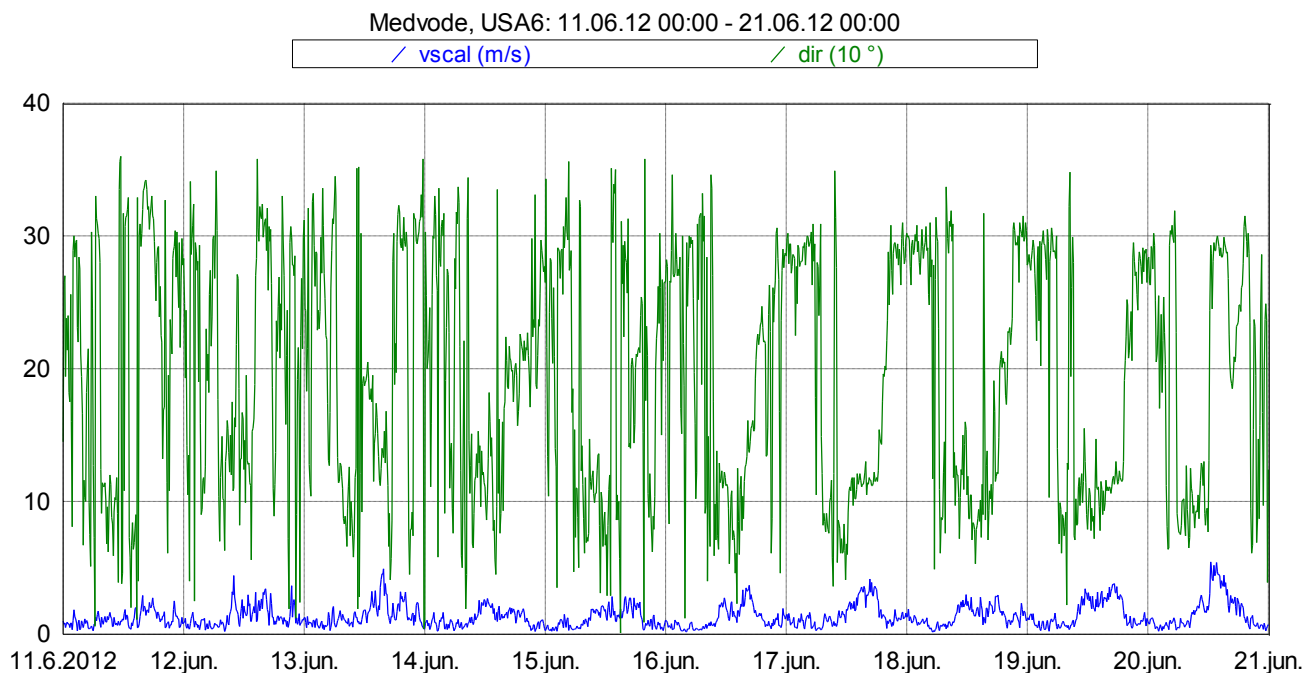
Slika 16: Smer in hitrost vetra med 11. 6. 2012 in 20. 6. 2012.
