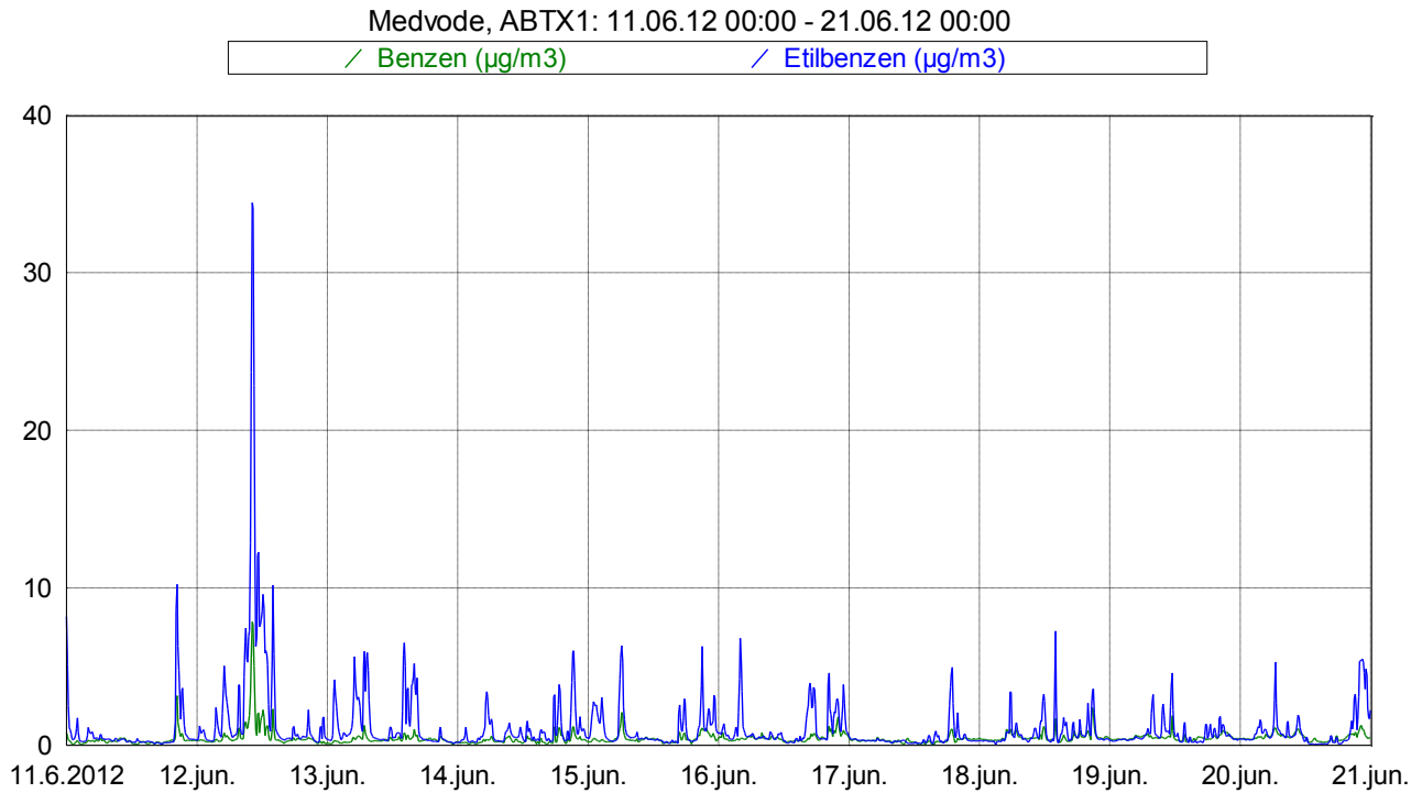
Slika 4: Imisijske koncentracije benzena in etilbenzena med 11. 6. 2012 in 20. 6. 2012.
