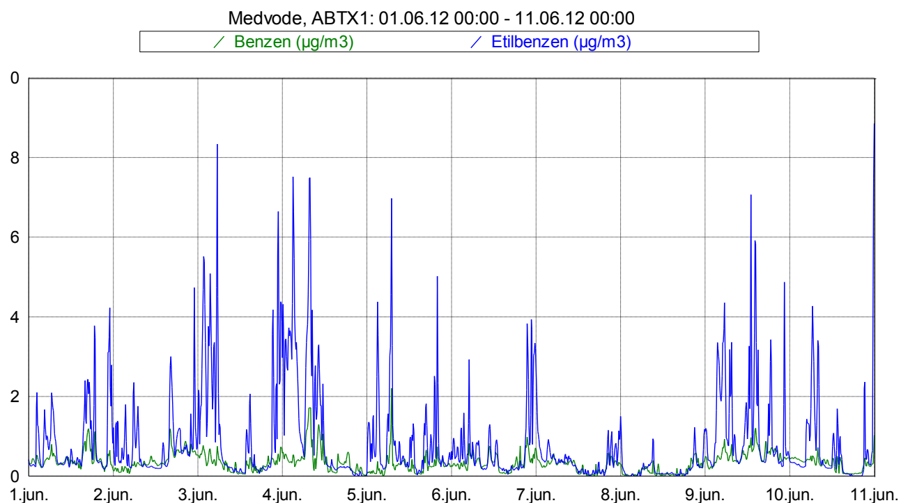
Slika 3: Imisijske koncentracije benzena in etilbenzena med vključno 1. 6. 2012 in 10. 6. 2012.
