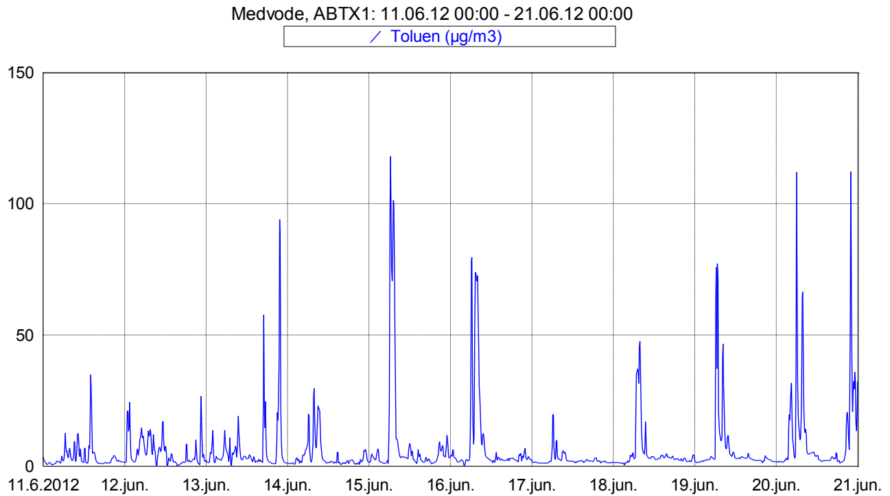
Slika 8: Imisijske koncentracije toluena med 11. 6. 2012 in 20. 6. 2012.
