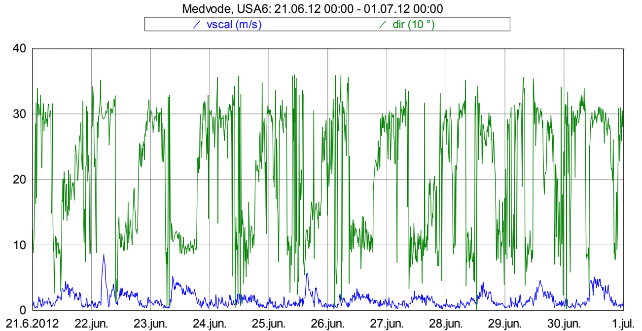
Slika 17: Smer in hitrost vetra med 21. 6. 2012 in 30. 6. 2012.
