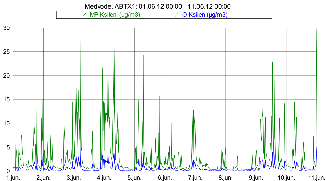
Slika 11: Imisijske koncentracije M&P in O ksilena med 1. 6. 2012 in 10. 6. 2012.
