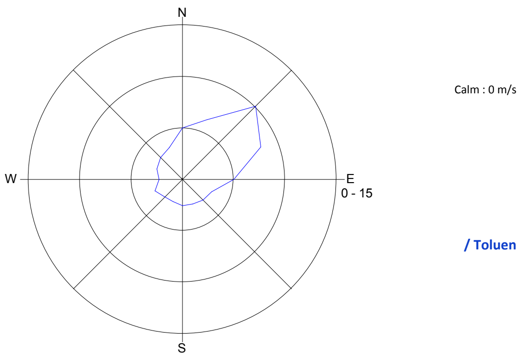
Slika 10: Roža onesnaženost - toluen, julij 2013.
