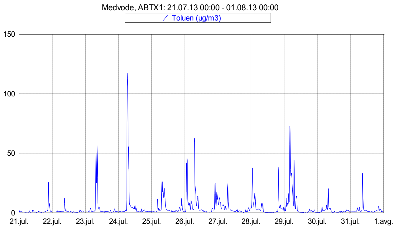
Slika 9: Imisijske koncentracije toluea med 21. 7. 2013 in 31. 7. 2013.
