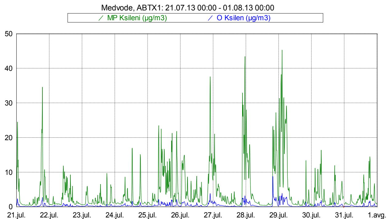
Slika 13: Imisijske koncentracije M&amp;P in O ksilena med 21. 7. 2013 in 31. 7. 2013.
