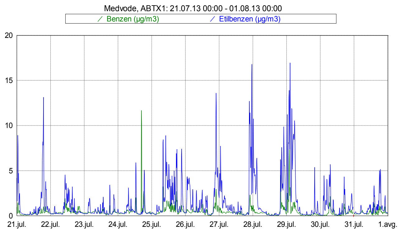
Slika 5: Imisijske koncentracije benzena in etilbenzena med 21. 7. 2013 in 31. 7. 2013.
