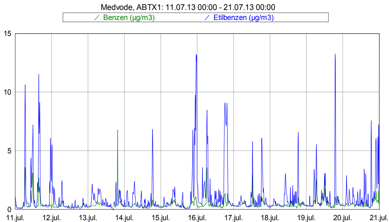
Slika 4: Imisijske koncentracije benzena in etilbenzena med 11. 7. 2013 in 20. 7. 2013.
