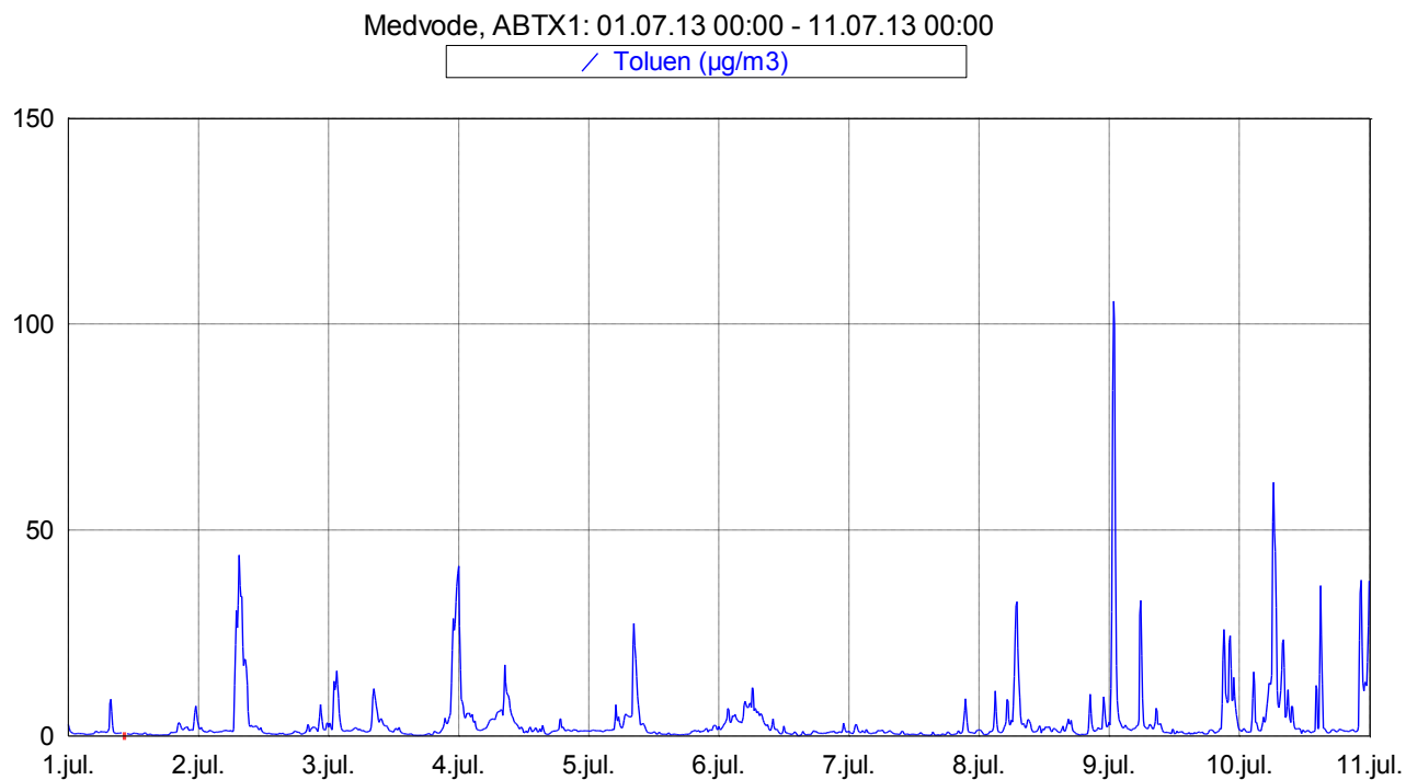
Slika 7: Imisijske koncentracije toluena med vključno 1. 7. 2013 in 10. 7. 2013.
