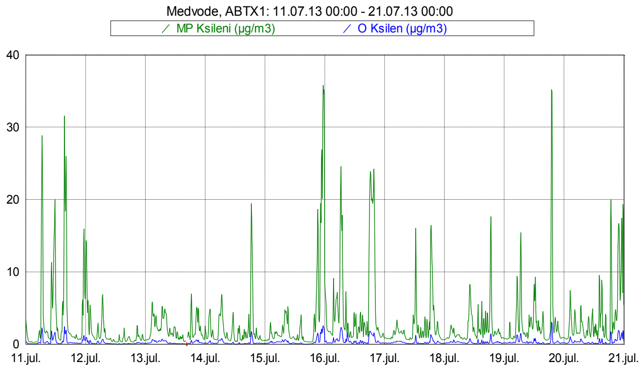
Slika 12: Imisijske koncentracije M&amp;P in O ksilena med 11. 7. 2013 in 20. 7. 2013.
