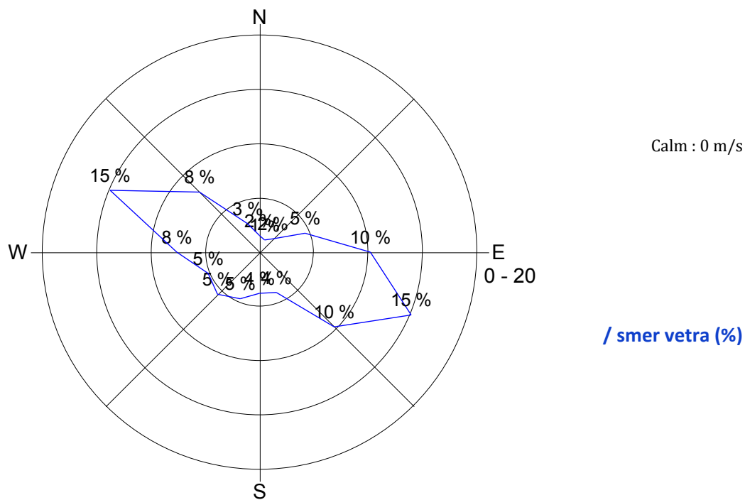
Slika 18: Roža vetrov, julij 2013.
