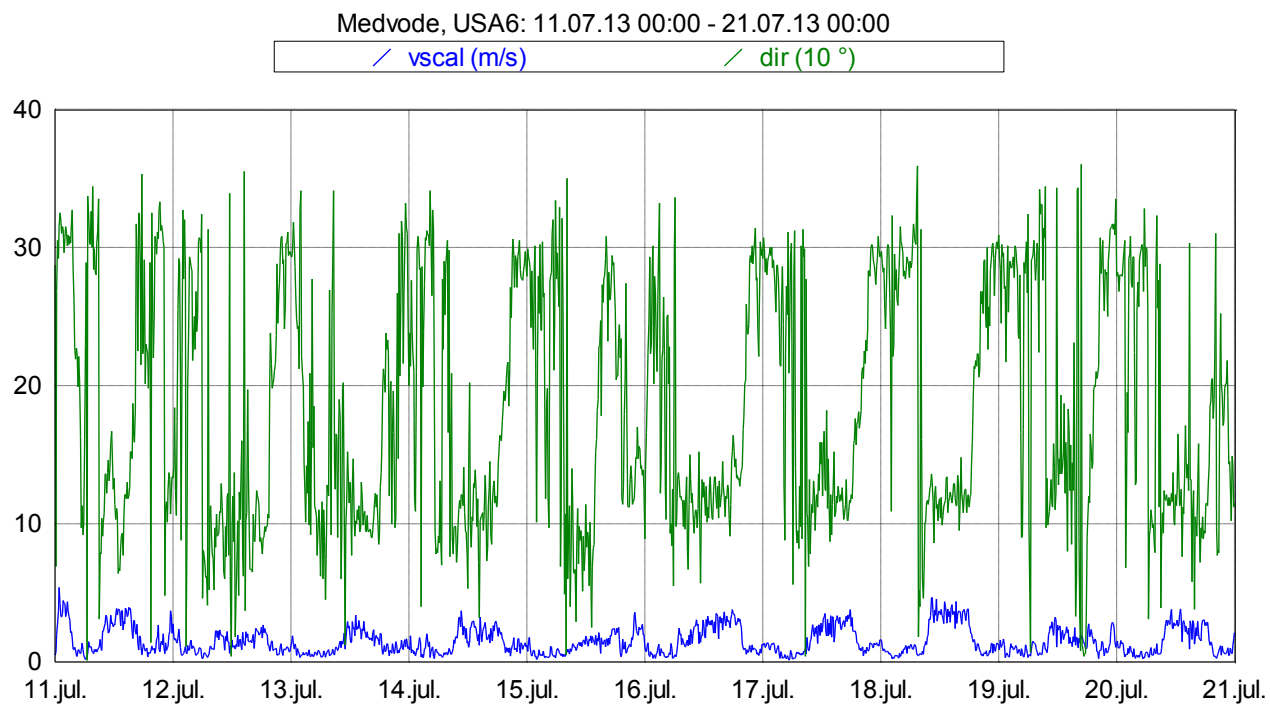
Slika 16: Smer in hitrost vetra med 11. 7. 2013 in 20. 7. 2013.
