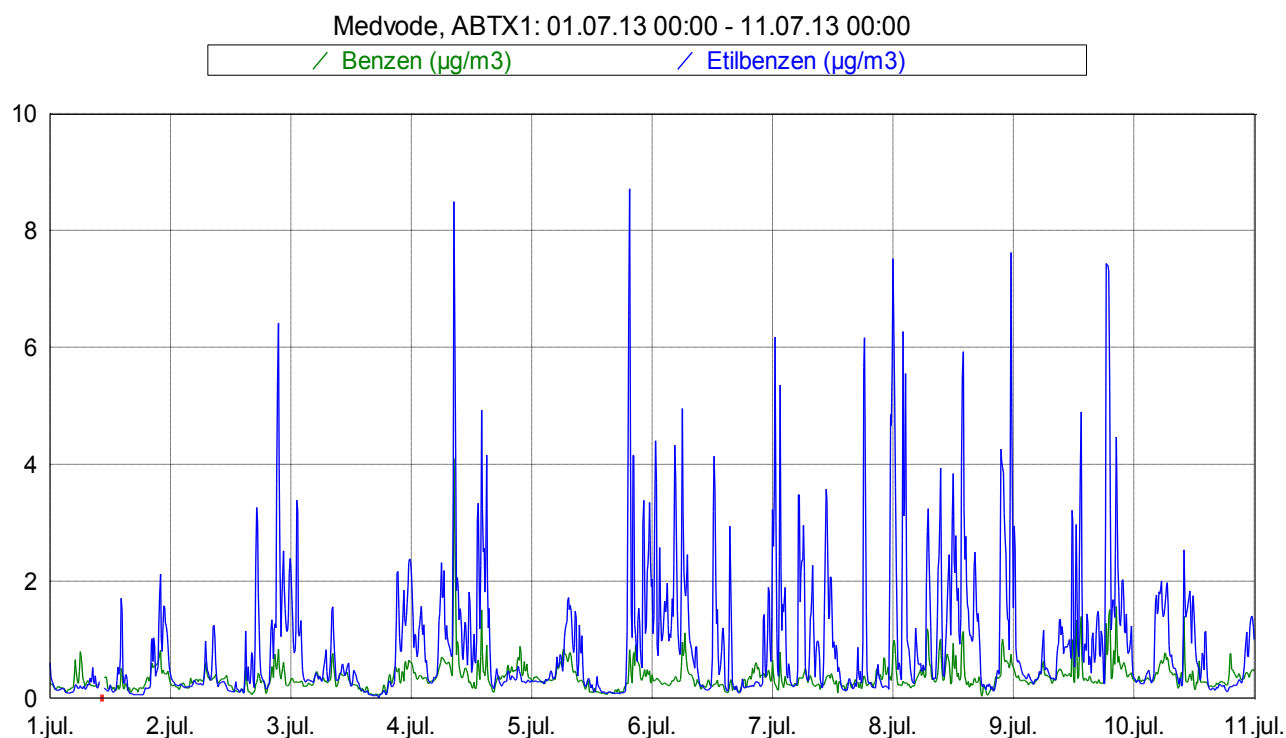
Slika 3: Imisijske koncentracije benzena in etilbenzena med vključno 1. 7. 2013 in 10. 7. 2013.
