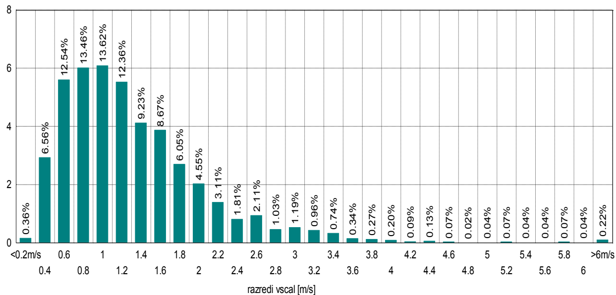
Slika 19: Frekvenčna porazdelitev po hitrosti vetra, julij 2013.
