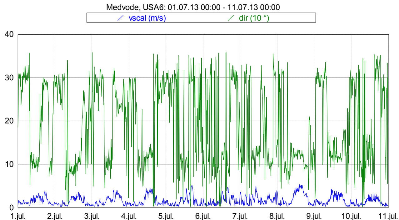
Slika 15: Smer in hitrost vetra med 1. 7. 2013 in 10. 7. 2013.
