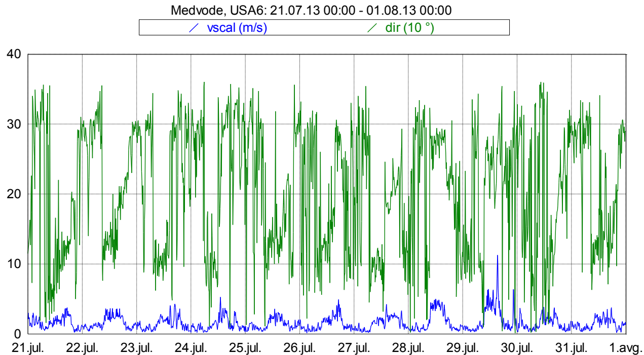
Slika 17: Smer in hitrost vetra med 21. 7. 2013 in 31. 7. 2013.
