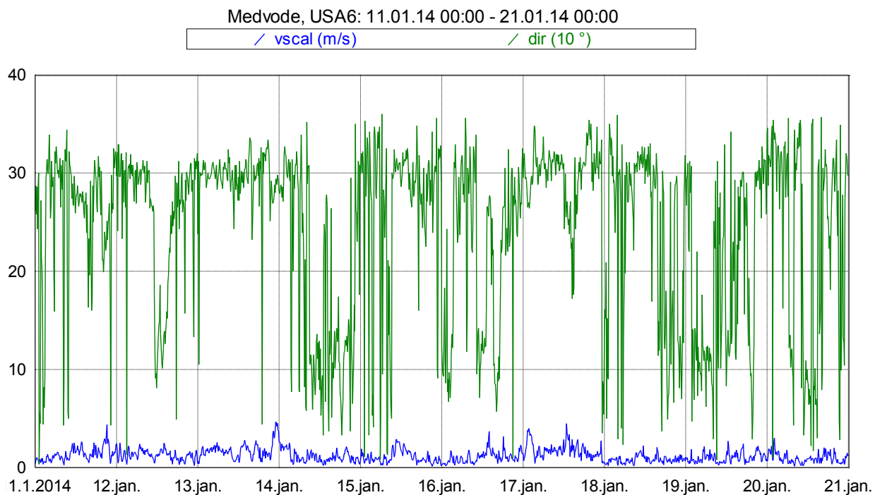
Slika 17: Smer in hitrost vetra med 11. 1. 2014 in 20. 1. 2014.
