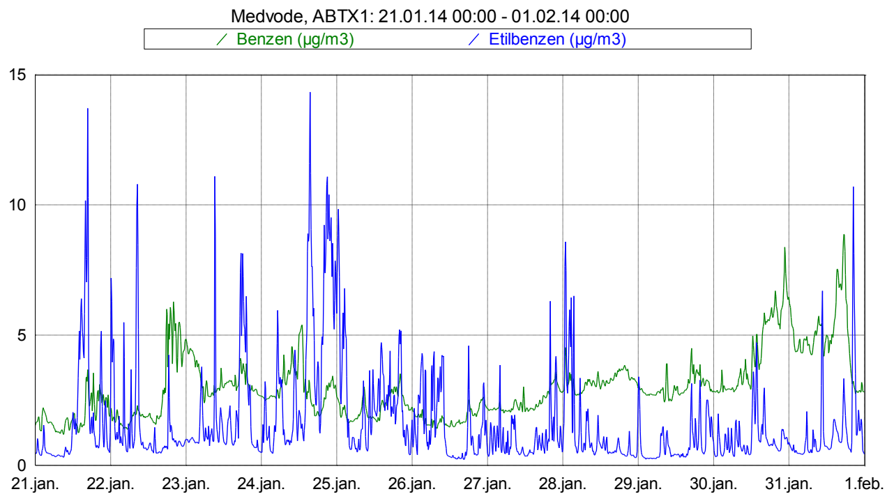
Slika 5: Imisijske koncentracije benzena in etilbenzena med 21. 1. 2014 in 31. 1. 2014.
