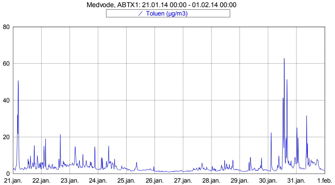
Slika 10: Imisijske koncentracije toluena med 21. 1. 2014 in 31. 1. 2014.
