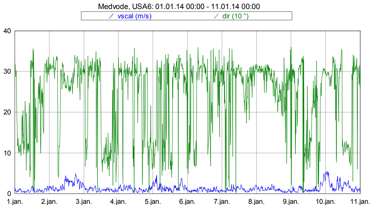
Slika 16: Smer in hitrost vetra med 1. 1. 2014 in 10. 1. 2014.
