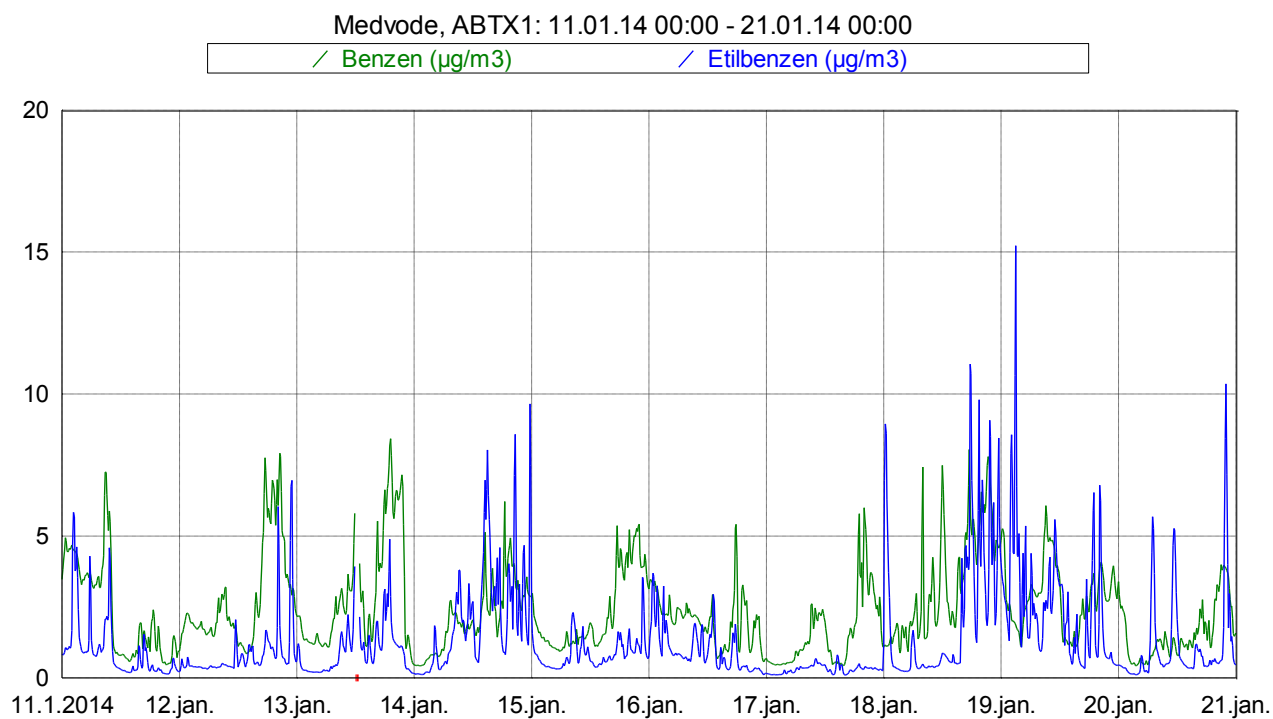
Slika 4: Imisijske koncentracije benzena in etilbenzena med 11. 1. 2014 in 20. 1. 2014.
