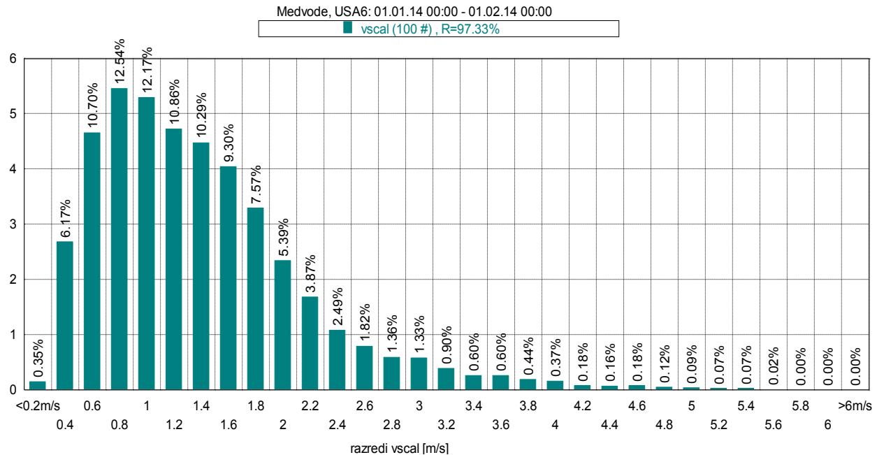
Slika 20: Frekvenčna porazdelitev po hitrosti vetra, januar 2014.
