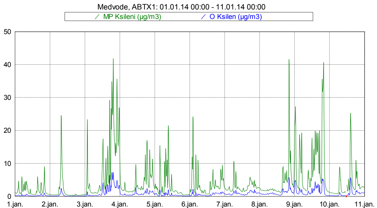
Slika 12: Imisijske koncentracije M&P in O ksilena med vključno 1. 1. 2014 in 10. 1. 2014.
