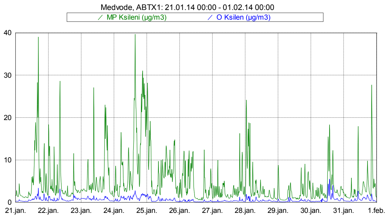
Slika 14: Imisijske koncentracije M&P in O ksilena med 21. 1. 2014 in 31. 1. 2014.
