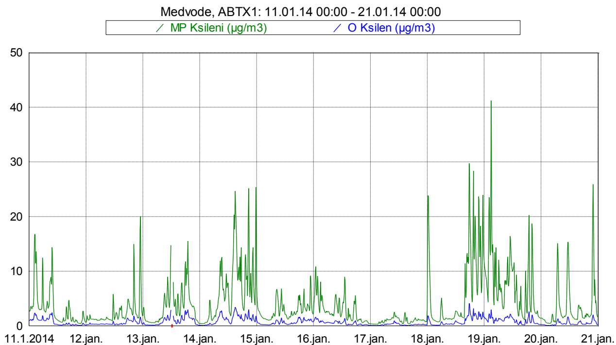
Slika 13: Imisijske koncentracije M&P in O ksilena med 11. 1. 2014 in 20. 1. 2014.
