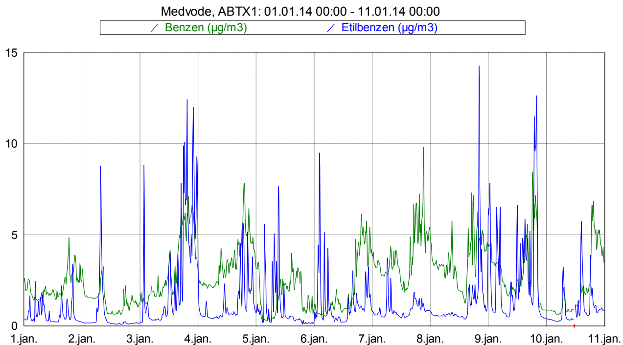
Slika 3: Imisijske koncentracije benzena in etilbenzena med vključno 1. 1. 2014 in 10. 1. 2014.
