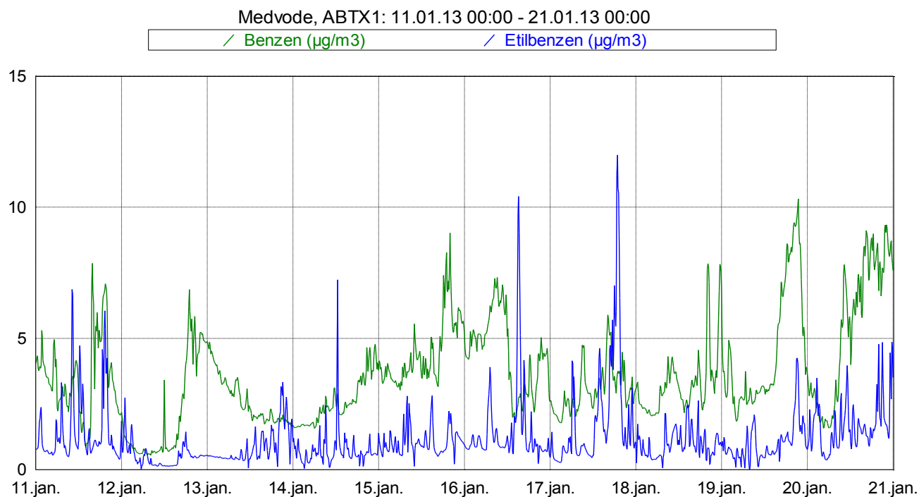
Slika 4: Imisijske koncentracije benzena in etilbenzena med 11. 1. 2013 in 21. 1. 2013.
