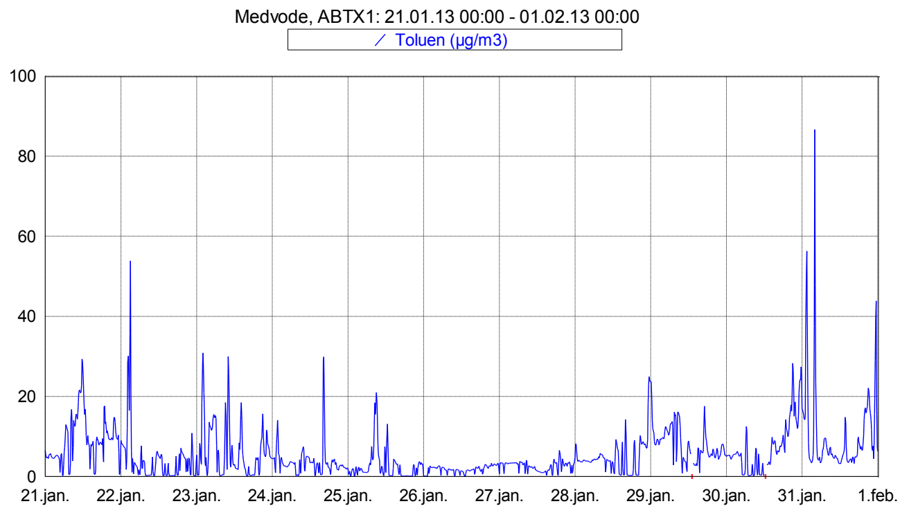
Slika 9: Imisijske koncentracije tolueuna med 21. 1. 2013 in 31. 1. 2013.
