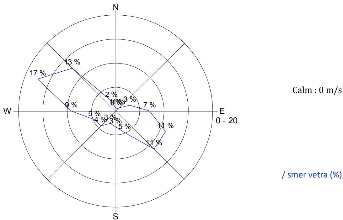
Slika 17: Smer in hitrost vetra med 21. 1. 2013 in 31. 1. 2013.
