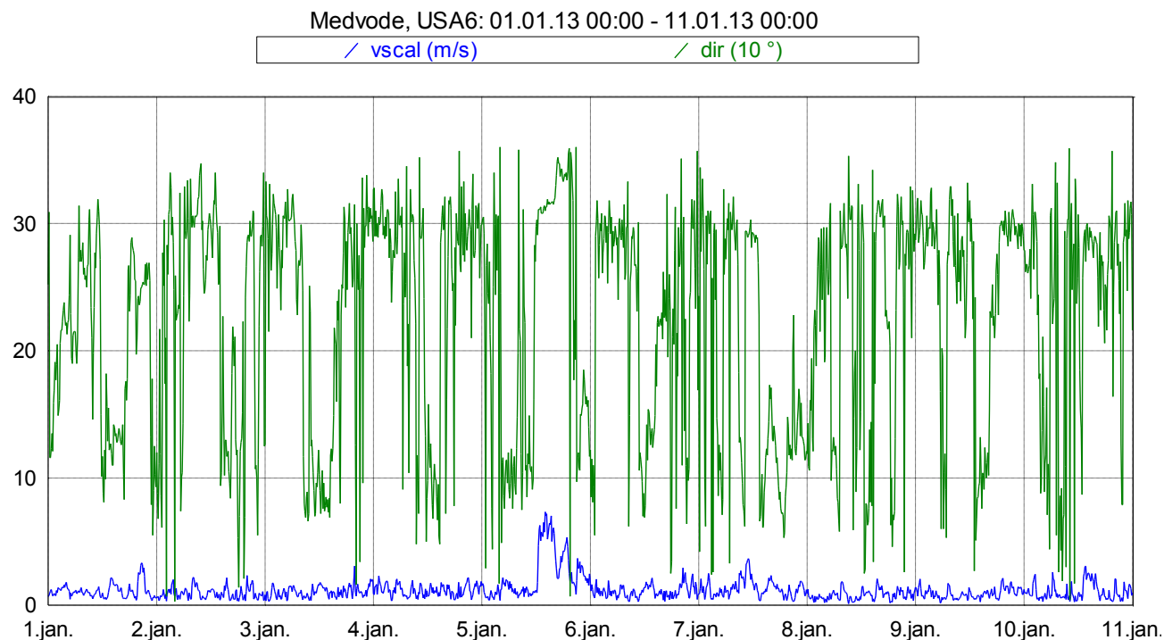
Slika 15: Smer in hitrost vetra med 1. 1. 2013 in 11. 1. 2013.
