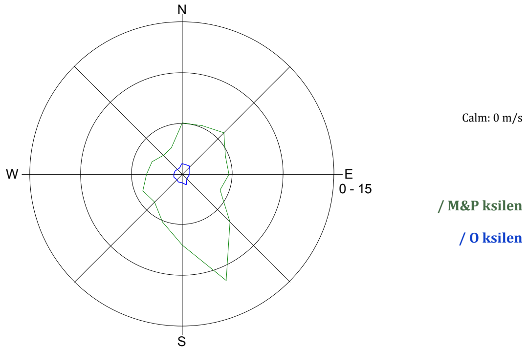
Slika 14: Roža onesnaženosti - M & P ksilen in O ksilen, januar 2013.
