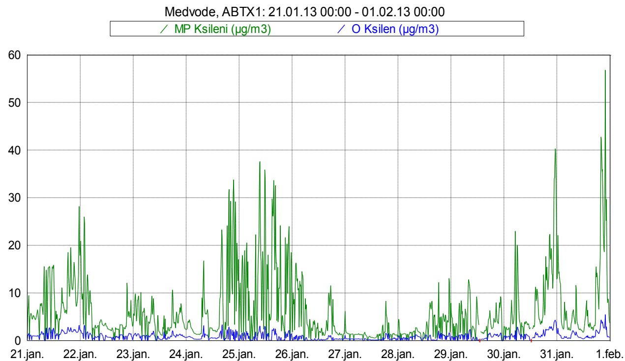
Slika 13: Imisijske koncentracije M&P in O ksilena med 21. 1. 2013 in 31. 1. 2013.
