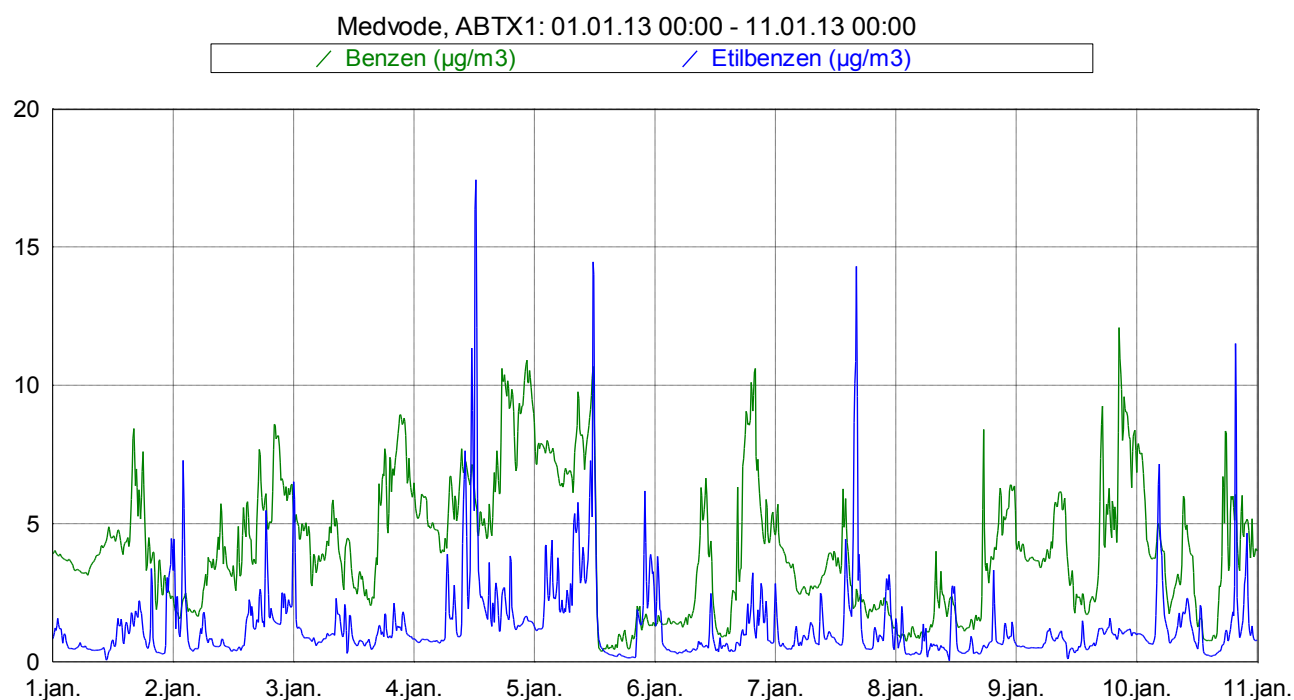
Slika 3: Imisijske koncentracije benzena in etilbenzena med vključno 1. 1. 2013 in 11. 1. 2013.
