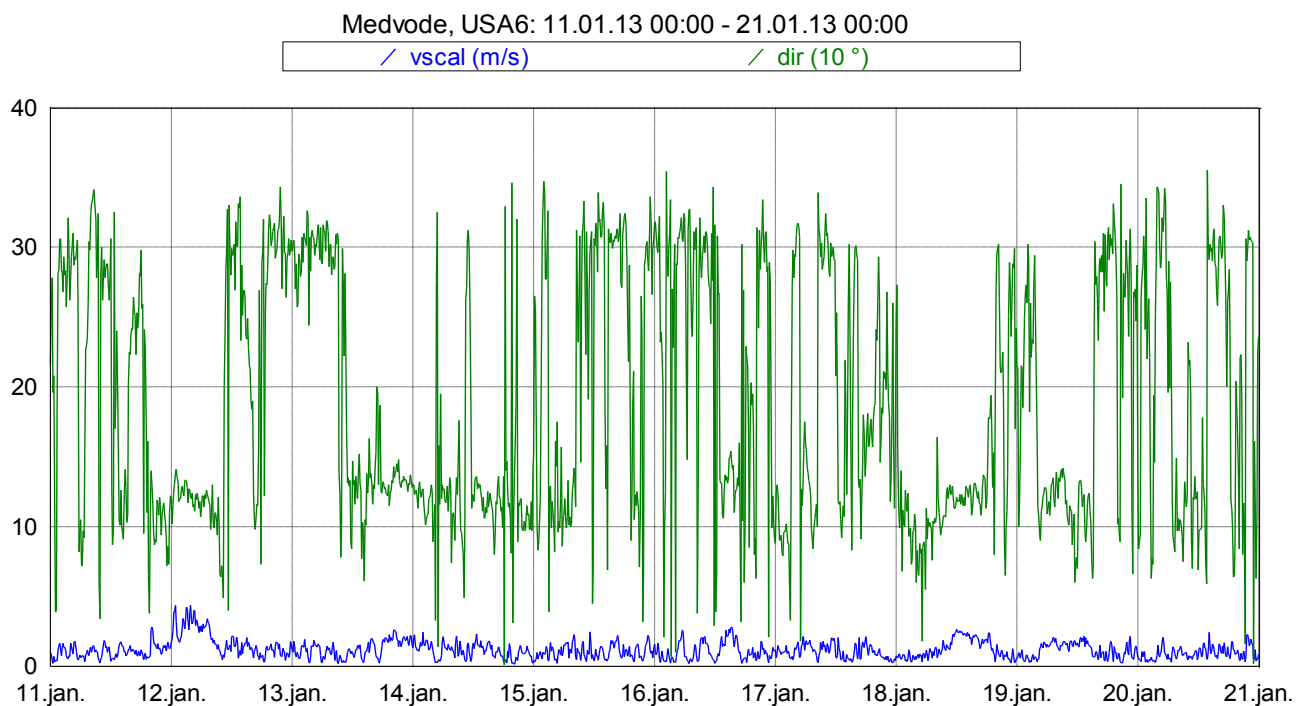
Slika 16: Smer in hitrost vetra med 11. 1. 2013 in 21. 1. 2013.
