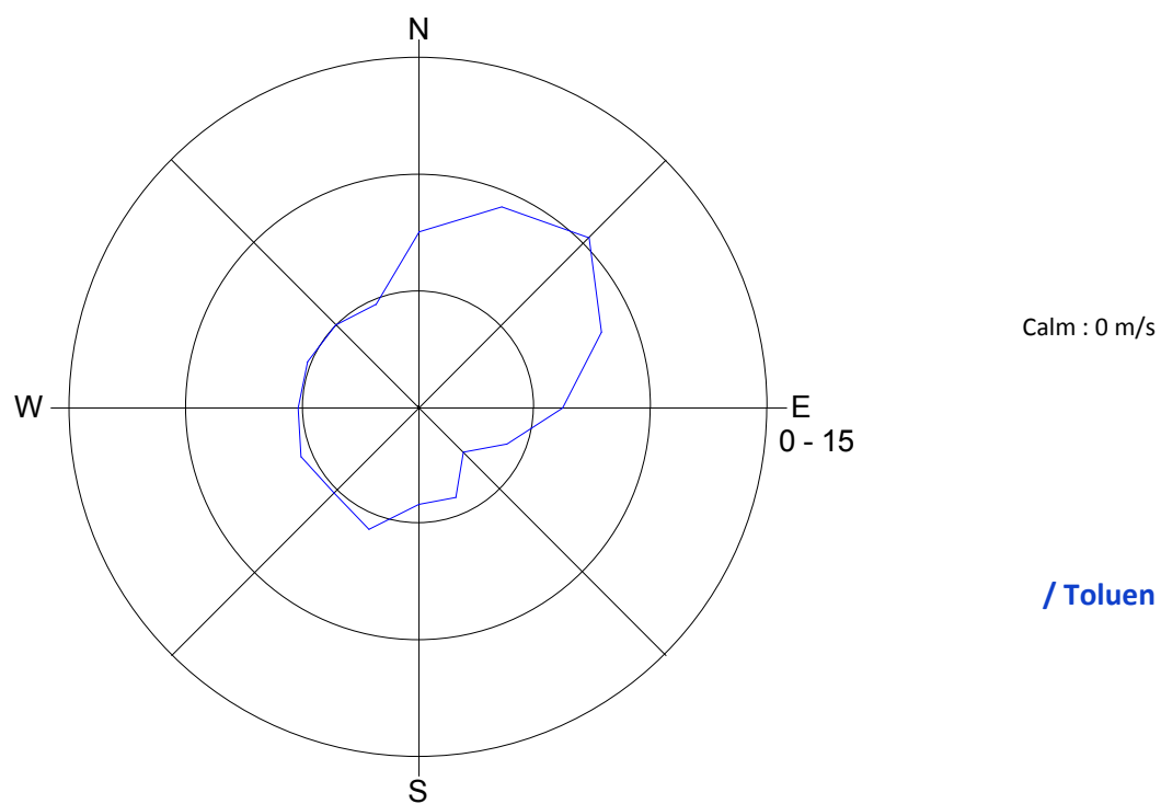
Slika 10: Roža onesnaženost - toluen, januar 2013.
