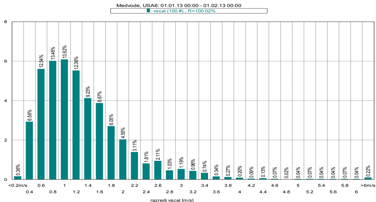
Slika 19: Frekvenčna porazdelitev po hitrosti vetra, januar 2013.
