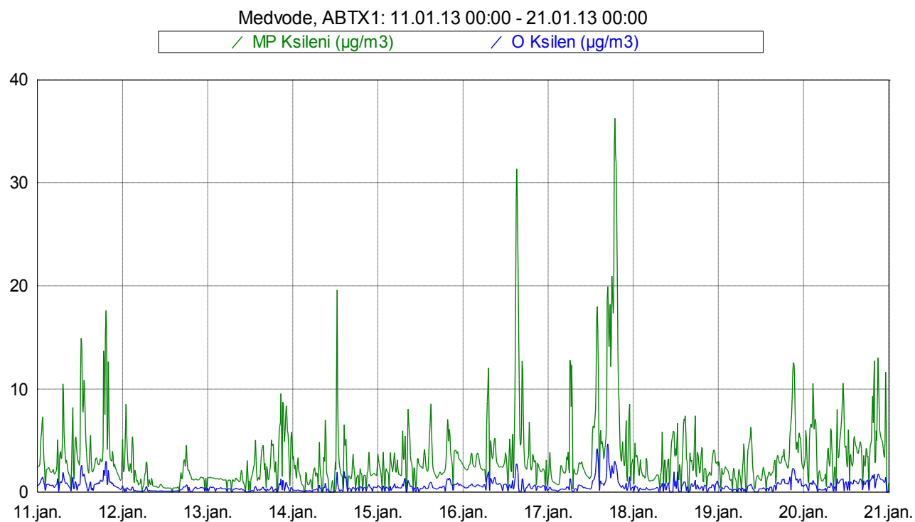
Slika 12: Imisijske koncentracije M&P in O ksilena med 11. 1. 2013 in 21. 1. 2013.
