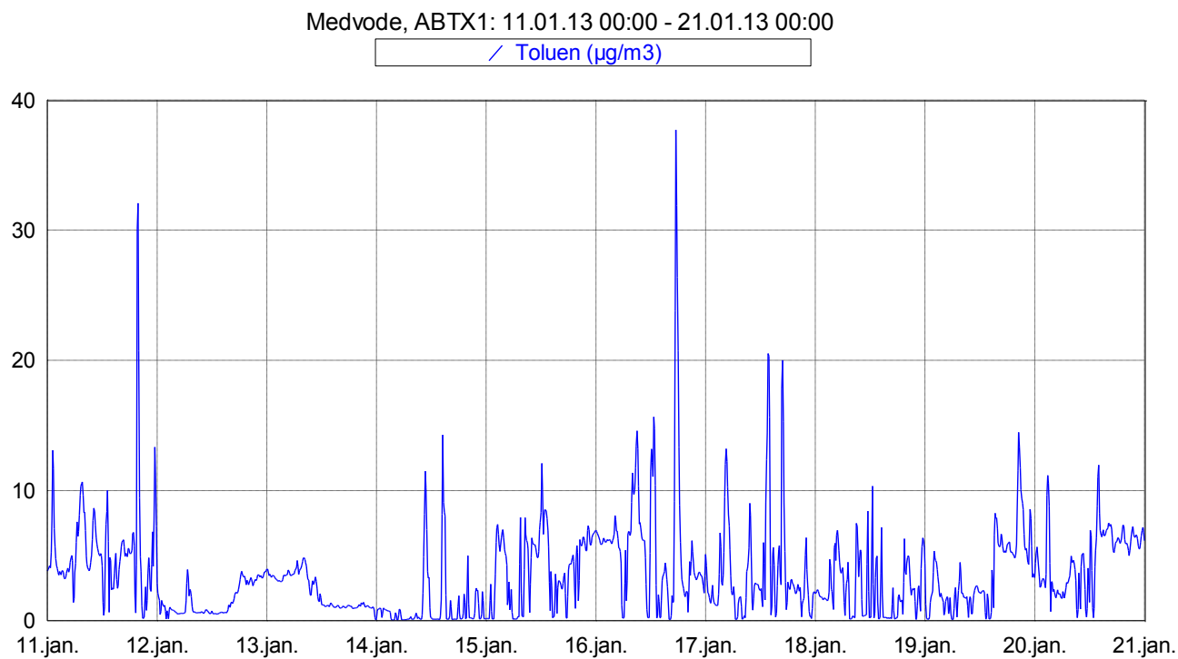
Slika 8: Imisijske koncentracije toluena med 11. 1. 2013 in 21. 1. 2013.
