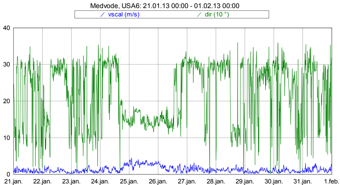
Slika 17: Smer in hitrost vetra med 21. 1. 2013 in 31. 1. 2013.
