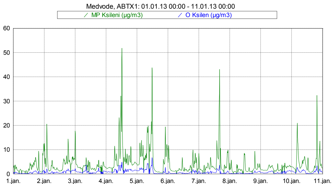
Slika 11: Imisijske koncentracije M&P in O ksilena med vključno 1. 1. 2013 in 11. 1. 2013.
