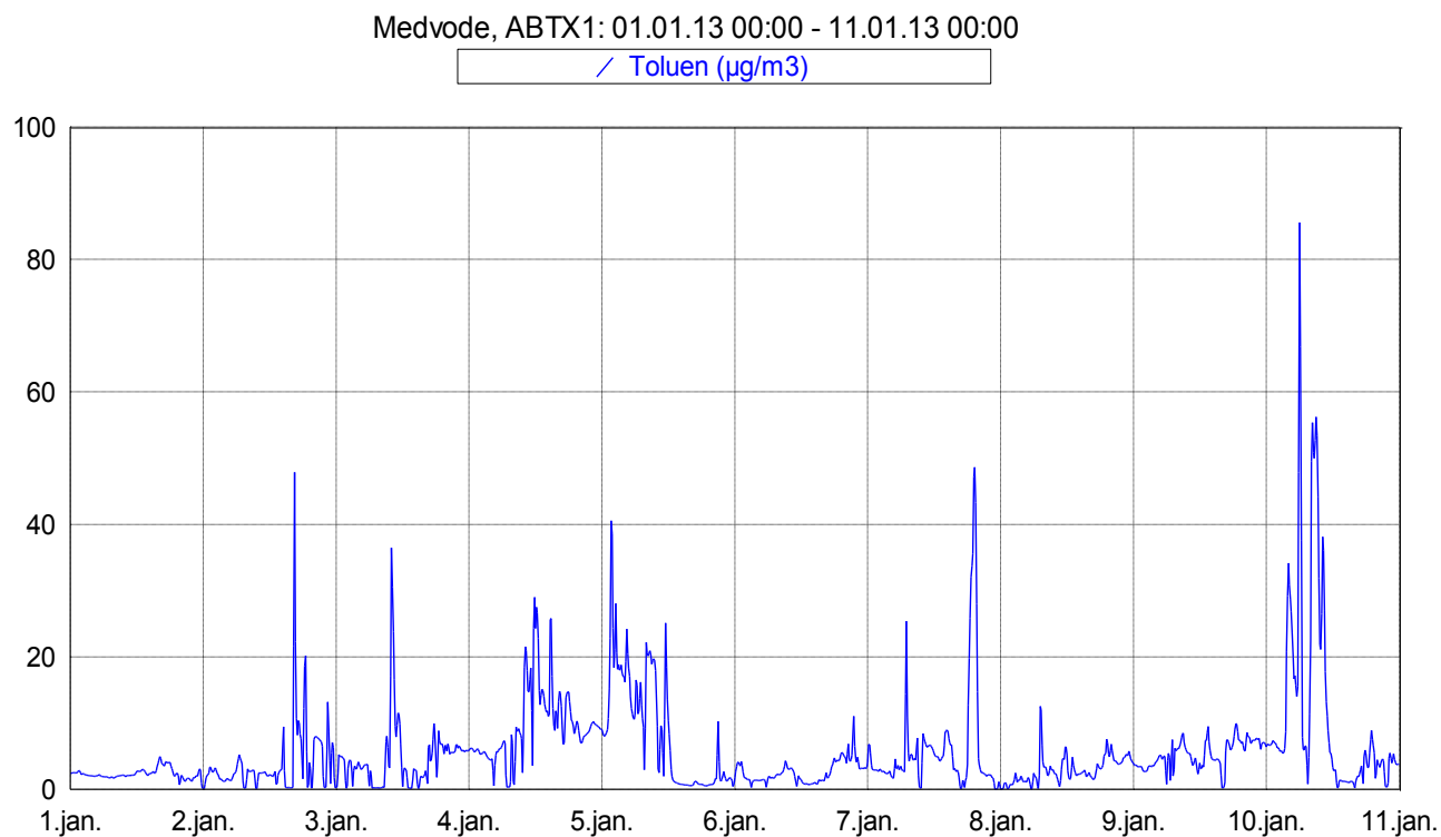
Slika 7: Imisijske koncentracije toluena med vključno 1. 1. 2013 in 11. 1. 2013.
