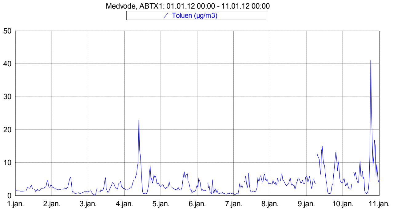
Slika 7: Imisijske koncentracije toluena med 1. 1. 2012 in 11. 1. 2012.
