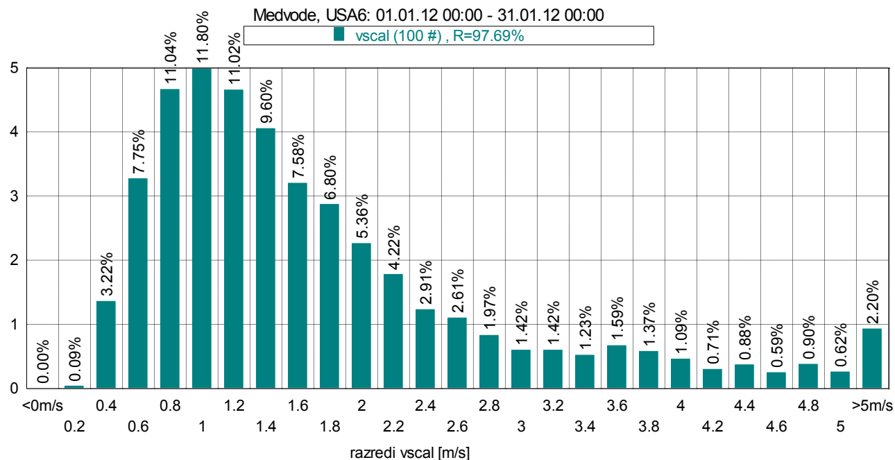
Slika 19: Frekvenčna porazdelitev po hitrosti vetra, januar 2012.
