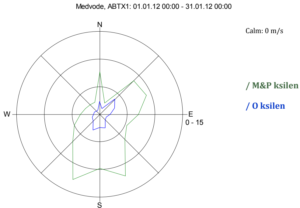
Slika 14: Roža onesnaženosti - M & P ksilen in O ksilen, januar 2012.
