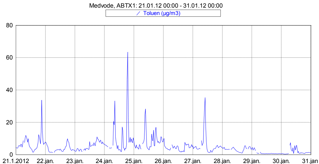
Slika 9: Imisijske koncentracije toluena med 21. 1. 2012 in 31. 1. 2012.
