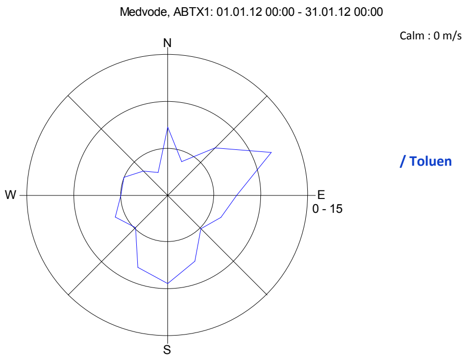
Slika 10: Roža onesnaženost - toluen, januar 2012.
