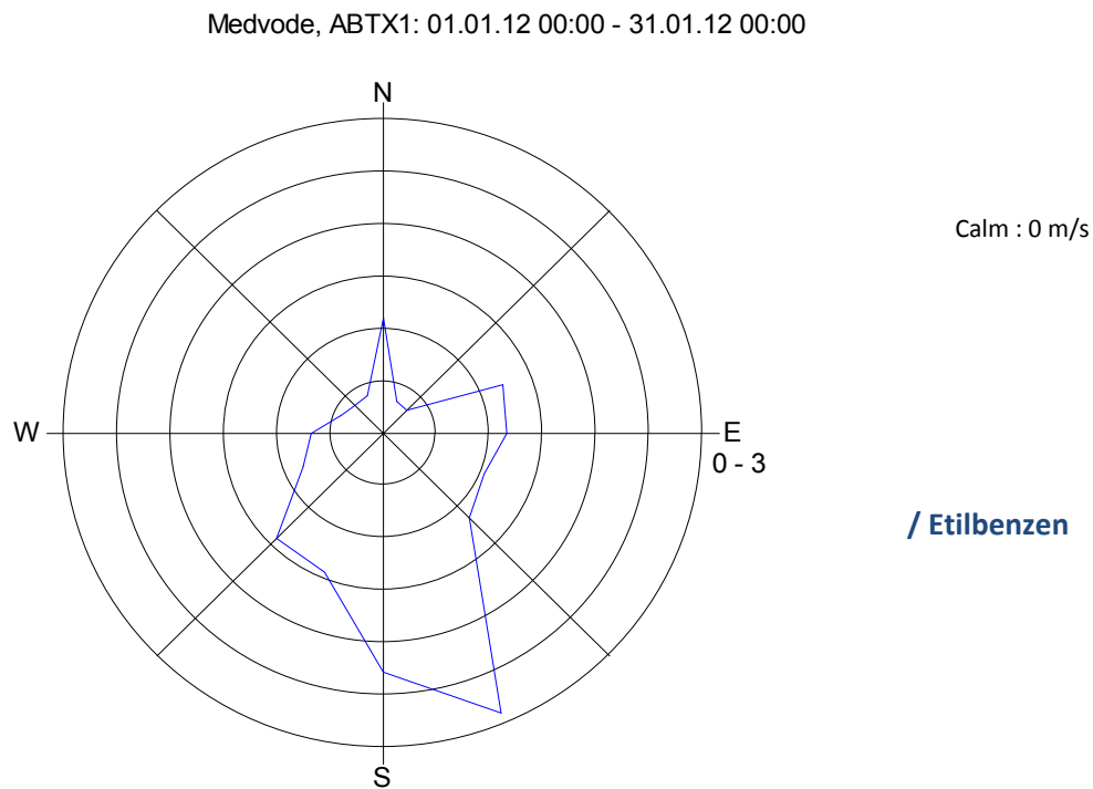
Slika 6: Roža onesnaženosti – benzen (zgoraj) in etilbenzen (spodaj), januar 2012.
