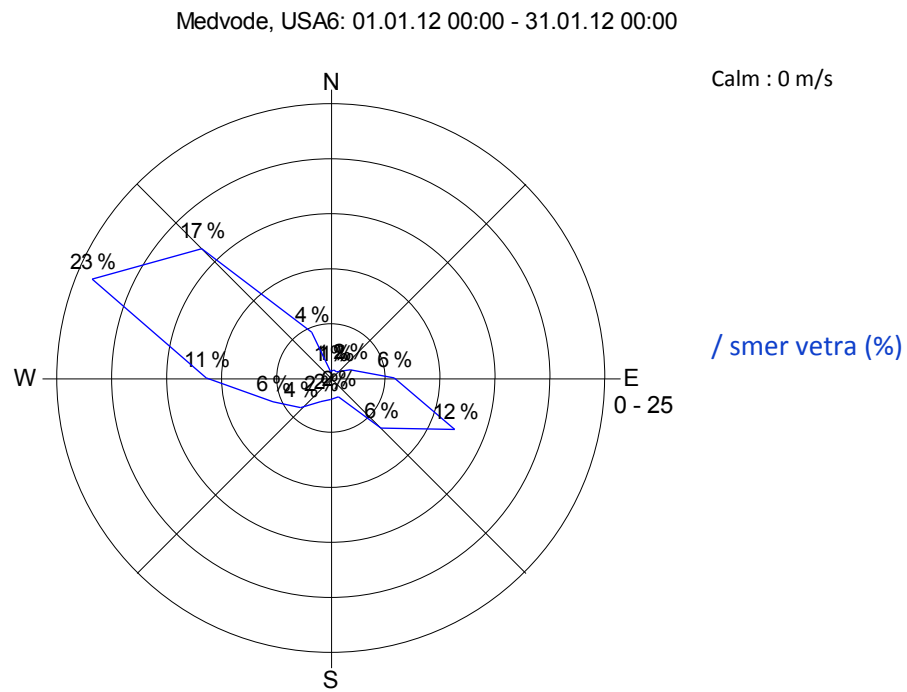
Slika 18: Roža Slika 18: Roža vetrov, januar 2012.
