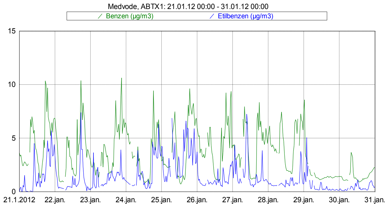
Slika 5: Imisijske koncentracije benzena in etilbenzena med 21. 1. 2012 in 31. 1. 2012.
