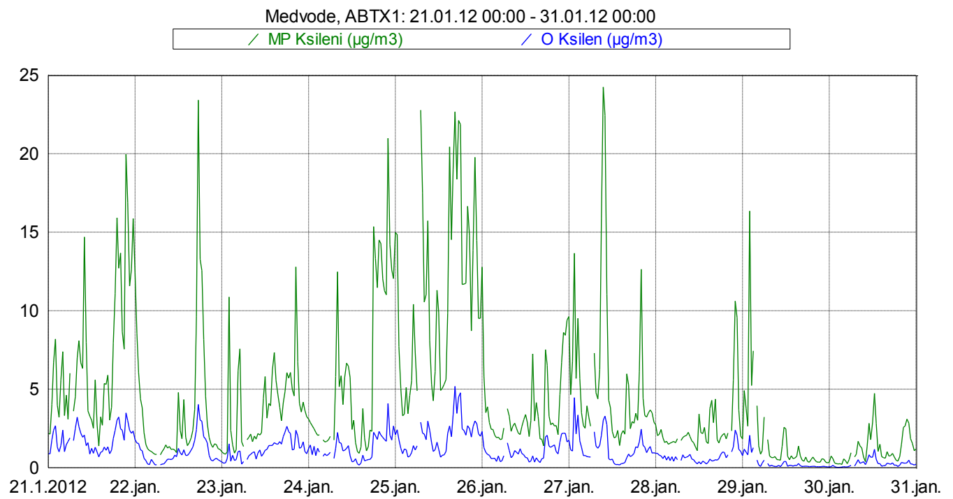
Slika 13: Imisijske koncentracije M&P in O ksilena med 21. 1. 2012 in 31. 1. 2012.
