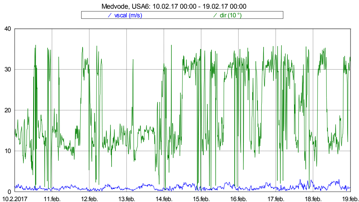
Slika 17: Smer in hitrost vetra med 10. 2. 2017 in 18. 2. 2017.
