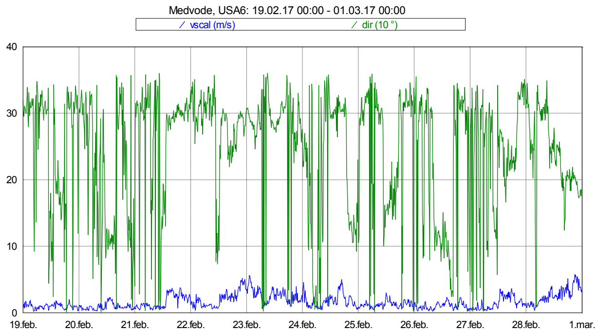
Slika 18: Smer in hitrost vetra med 19. 2. 2017 in 28. 2. 2017.
