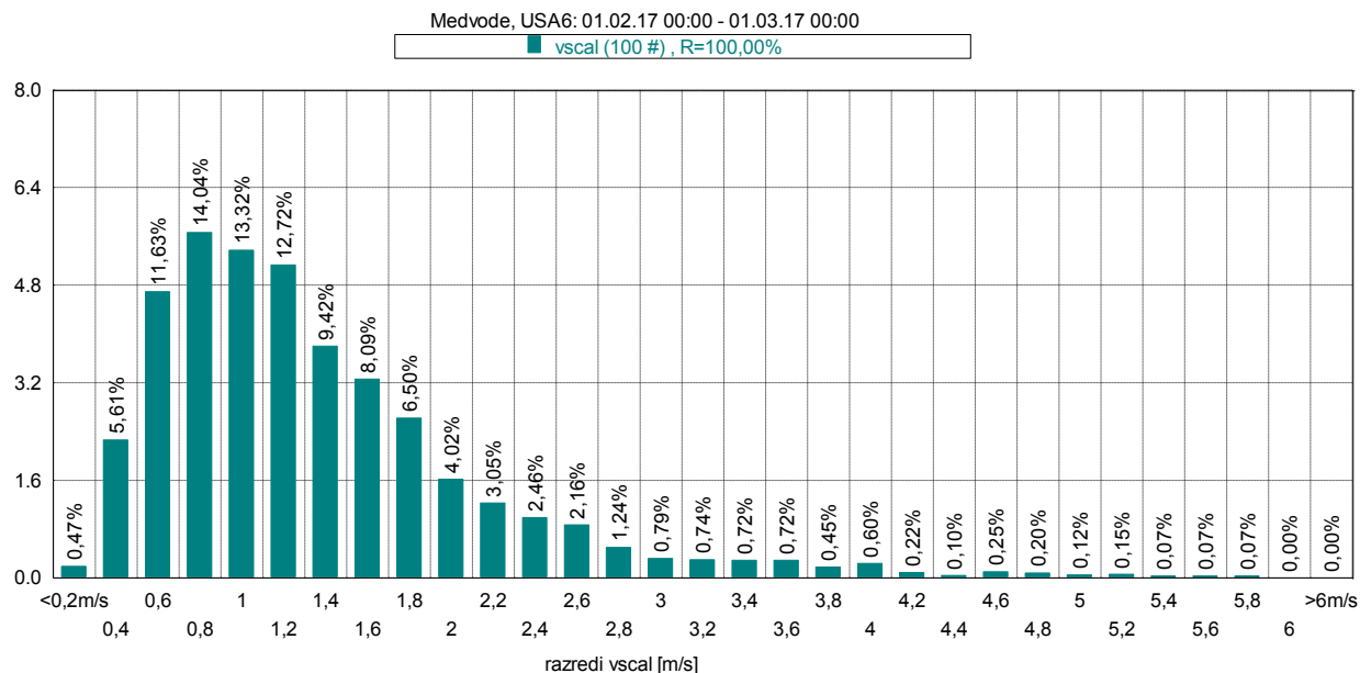
Slika 20: Frekvenčna porazdelitev po hitrosti vetra, februar 2017.
