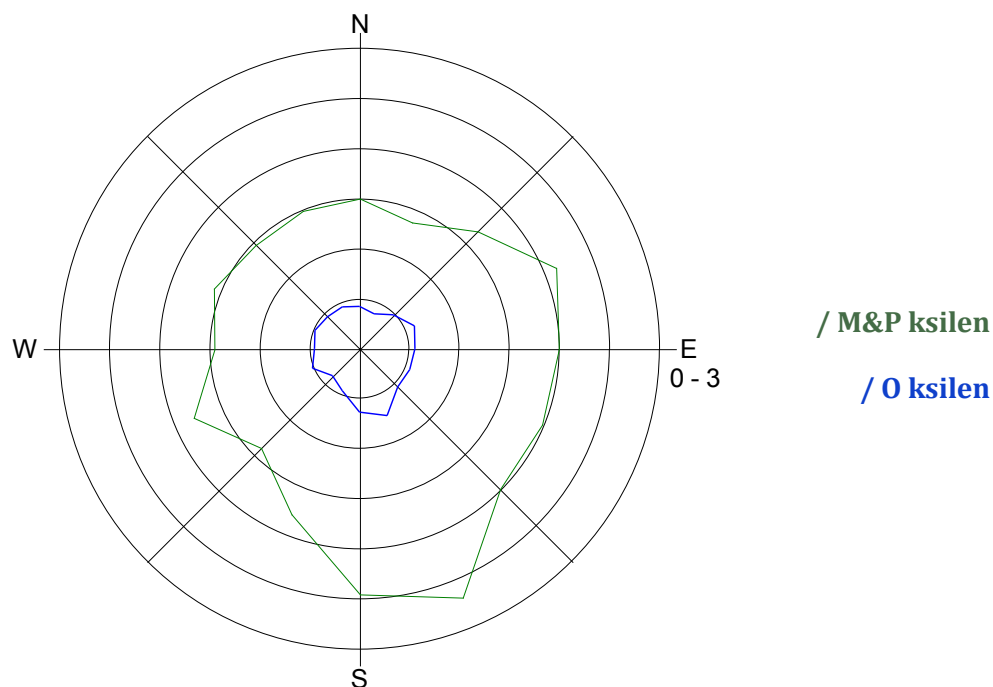
Slika 15: Roža onesnaženosti - M & P ksilen in O ksilen, februar 2016.
