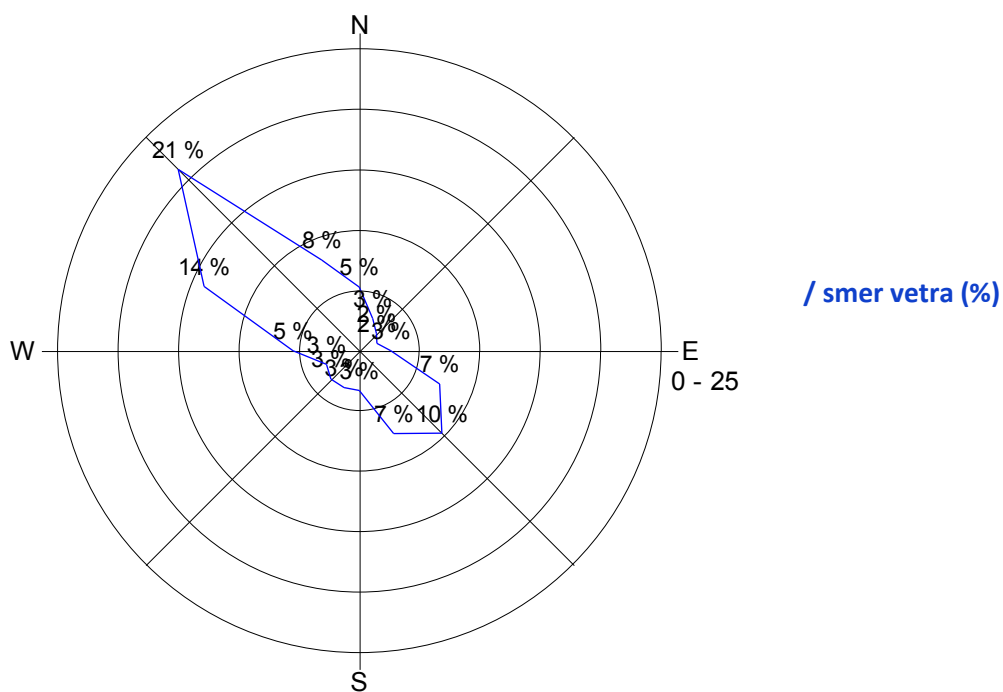
Slika 19: Roža vetrov, februar 2016.
