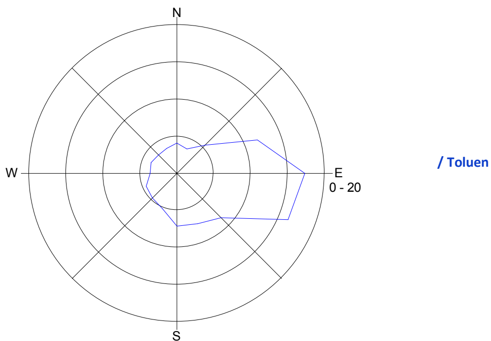
Slika 11: Roža onesnaženost - toluen, februar 2016.
