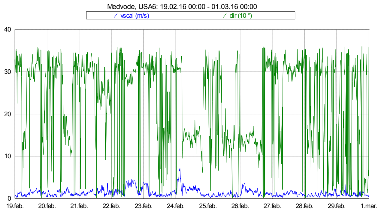
Slika 18: Smer in hitrost vetra med 19. 2. 2016 in 29. 2. 2016.
