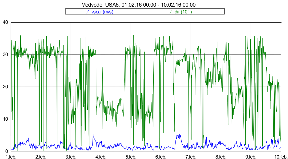
Slika 16: Smer in hitrost vetra med 1. 2. 2016 in 9. 2. 2016.
