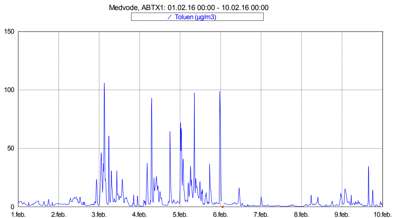
Slika 8: Imisijske koncentracije toluena med vključno 1. 2. 2016 in 9. 2. 2016.
