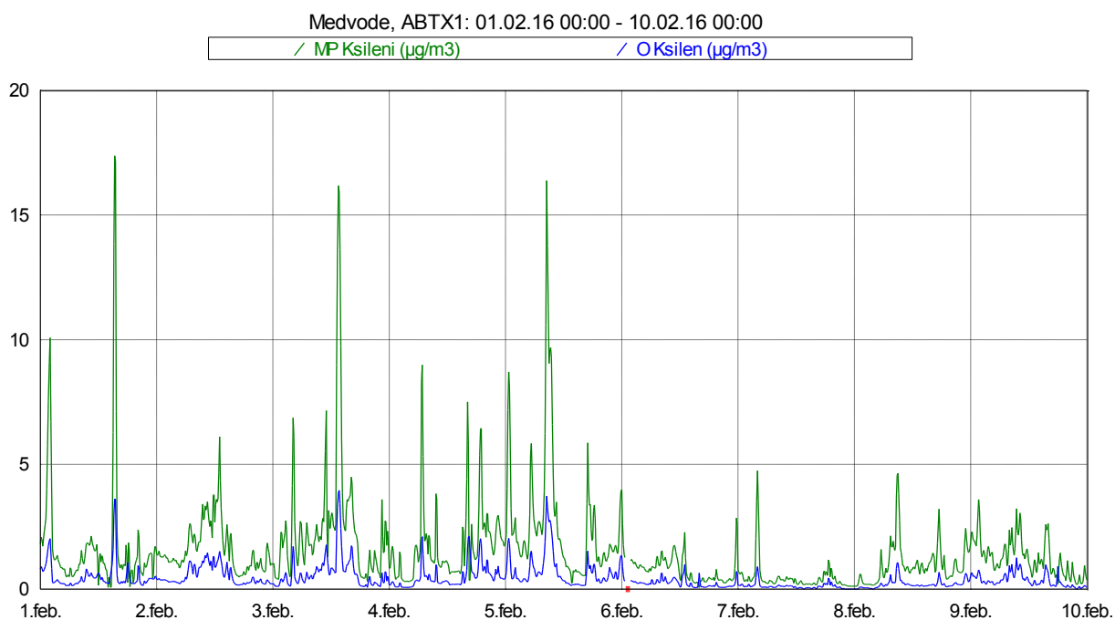
Slika 12: Imisijske koncentracije M&P in O ksilena med vključno 1. 2. 2016 in 9. 2. 2016.
