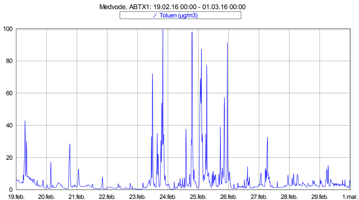
Slika 10: Imisijske koncentracije toluenta med 19. 2. 2016 in 29. 2. 2016.
