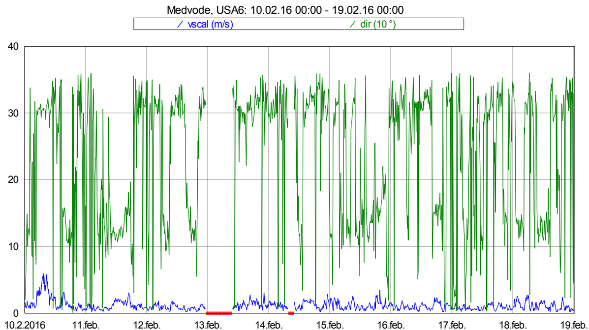
Slika 17: Smer in hitrost vetra med 10. 2. 2016 in 18. 2. 2016.
