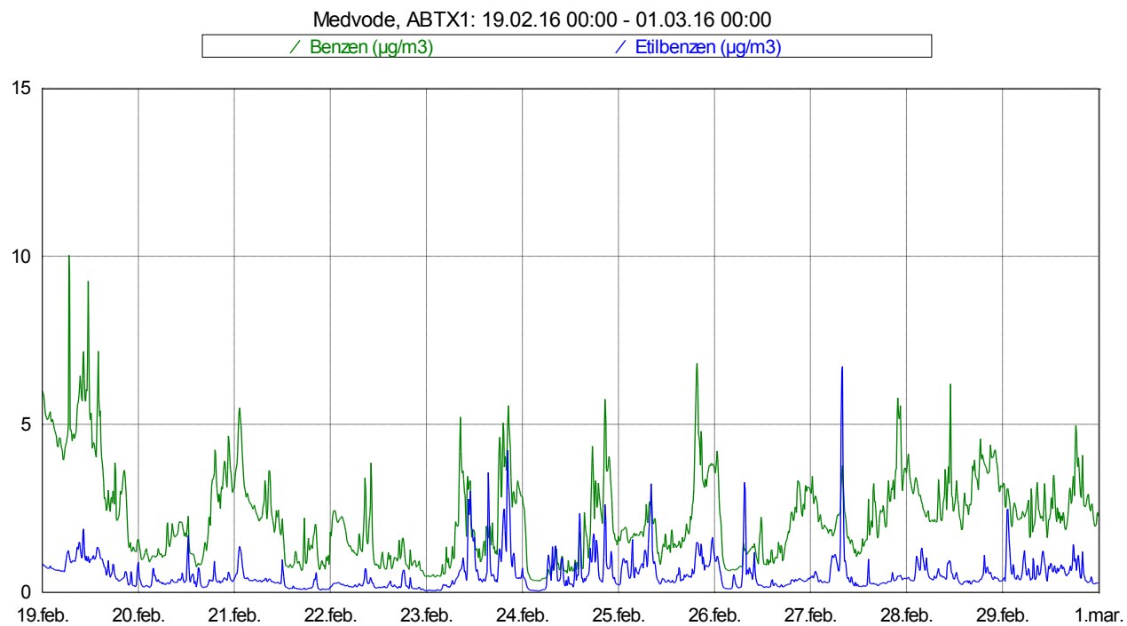
Slika 5: Imisijske koncentracije benzena in etilbenzena med 19. 2. 2016 in 29. 2. 2016.
