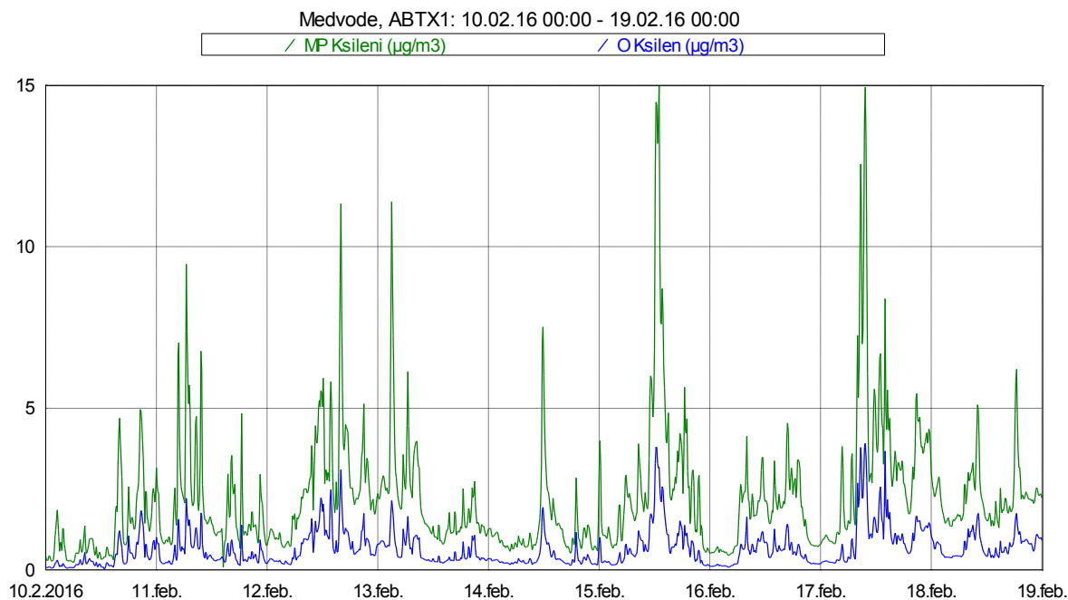
Slika 13: Imisijske koncentracije M&P in O ksilena med 10. 2. 2016 in 18. 2. 2016.
