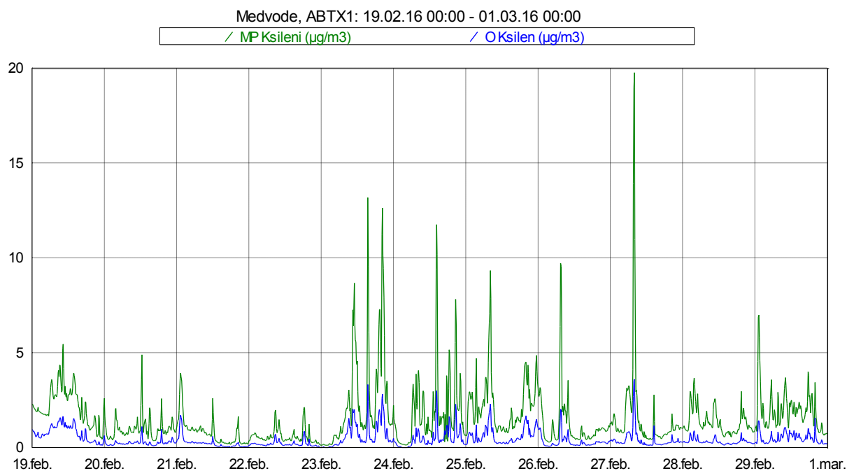
Slika 14: Imisijske koncentracije M&P in O ksilena med 19. 2. 2016 in 29. 2. 2016.
