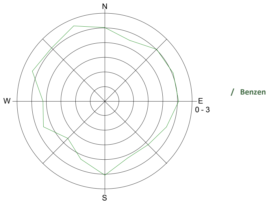
Slika 6: Roža onesnaženosti – benzen, februar 2016.
