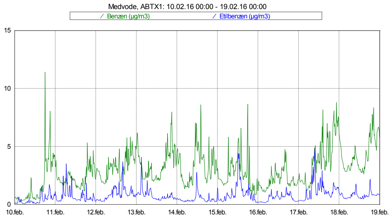
Slika 4: Imisijske koncentracije benzena in etilbenzena med 10. 2. 2016 in 18. 2. 2016.
