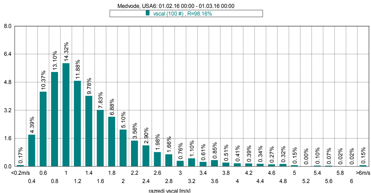
Slika 20: Frekvenčna porazdelitev po hitrosti vetra, februar 2016.
