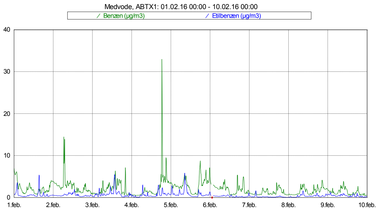
Slika 3: Imisijske koncentracije benzena in etilbenzena med vključno 1. 2. 2016 in 9. 2. 2016.
