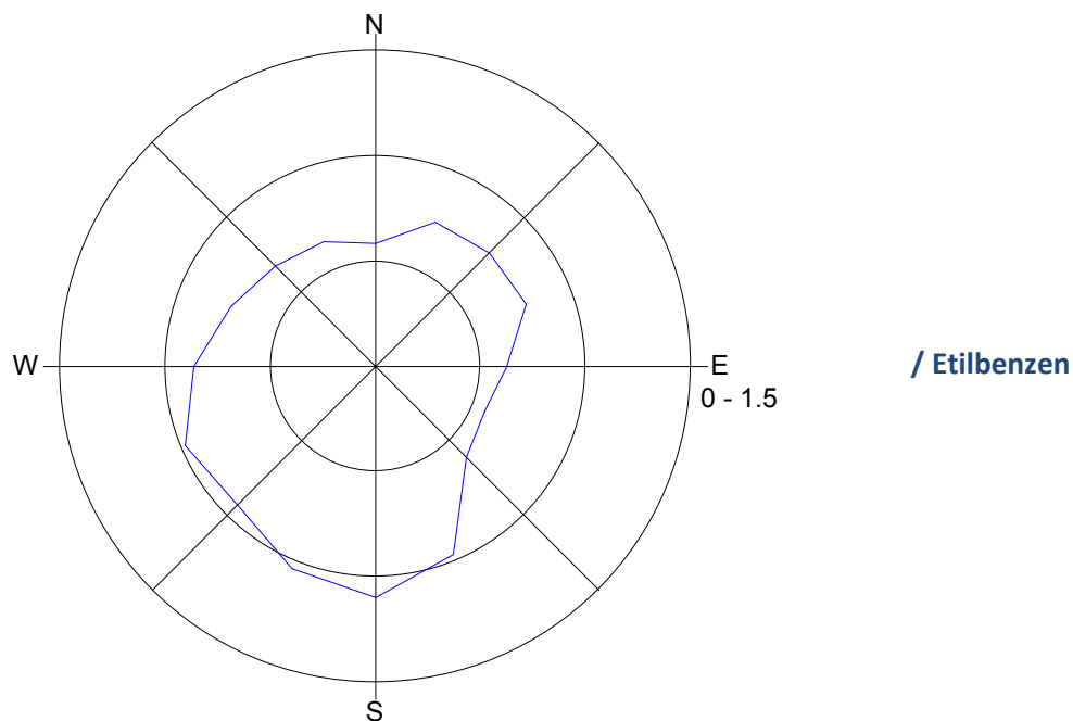
Slika 7: Roža onesnaženosti – etilbenzen, februar 2015.
