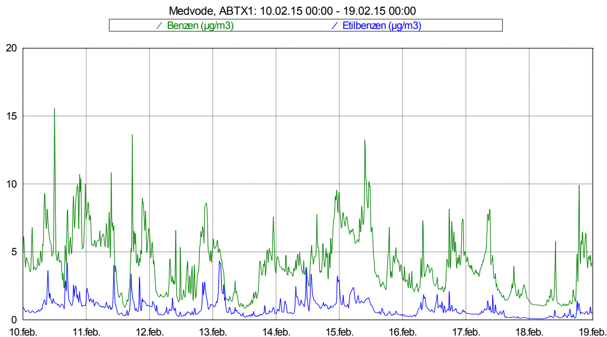
Slika 4: Imisijske koncentracije benzena in etilbenzena med 10. 2. 2015 in 18. 2. 2015.
