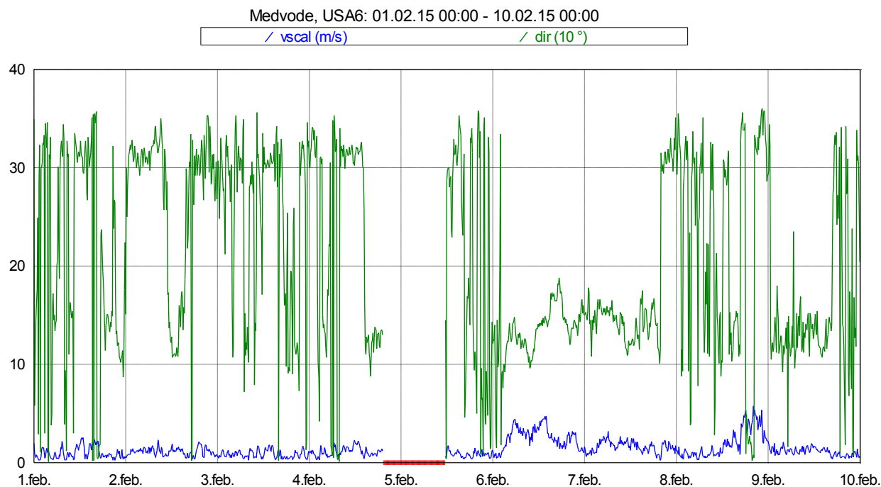
Slika 16: Smer in hitrost vetra med 1. 2. 2015 in 9. 2. 2015.
