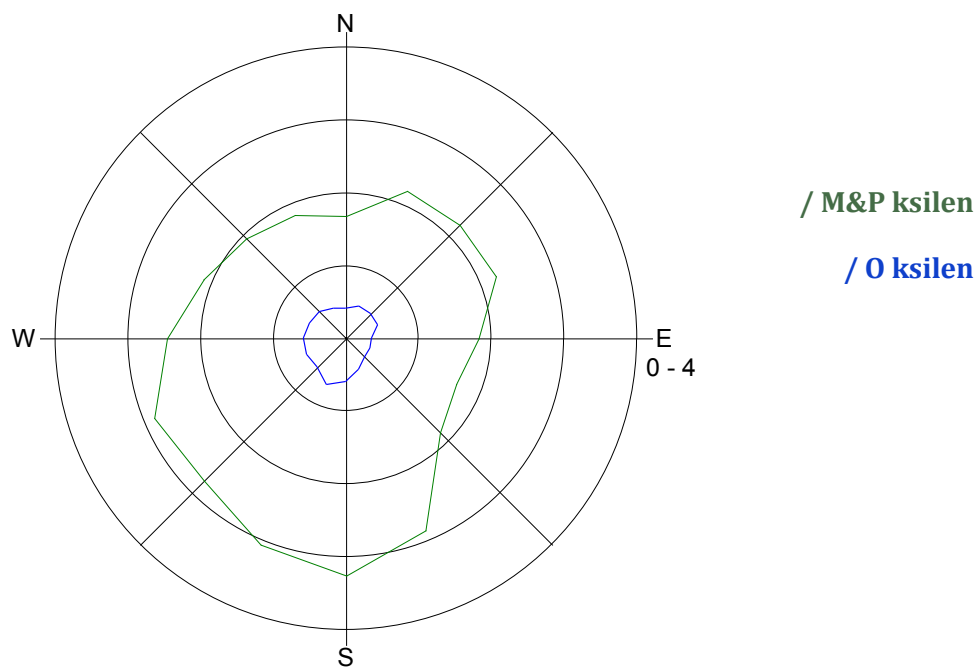
Slika 15: Roža onesnaženosti - M & P ksilen in O ksilen, februar 2015.
