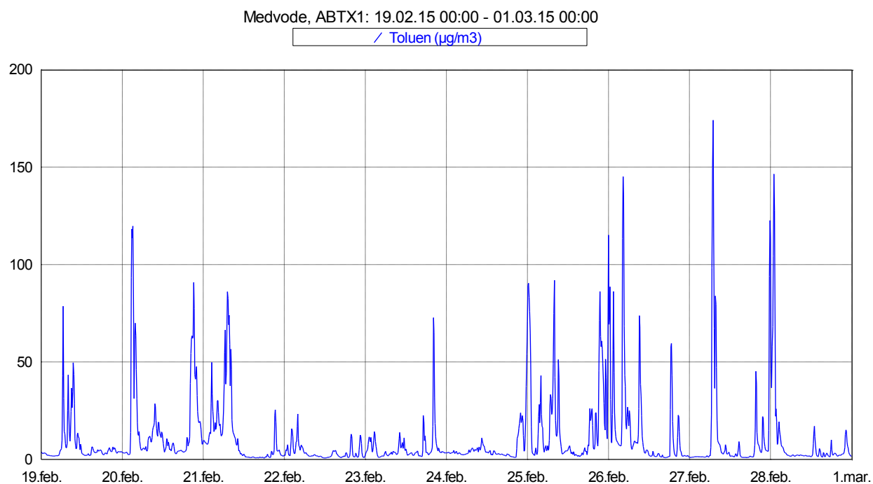
Slika 10: Imisijske koncentracije toluenta med 19. 2. 2015 in 28. 2. 2015.
