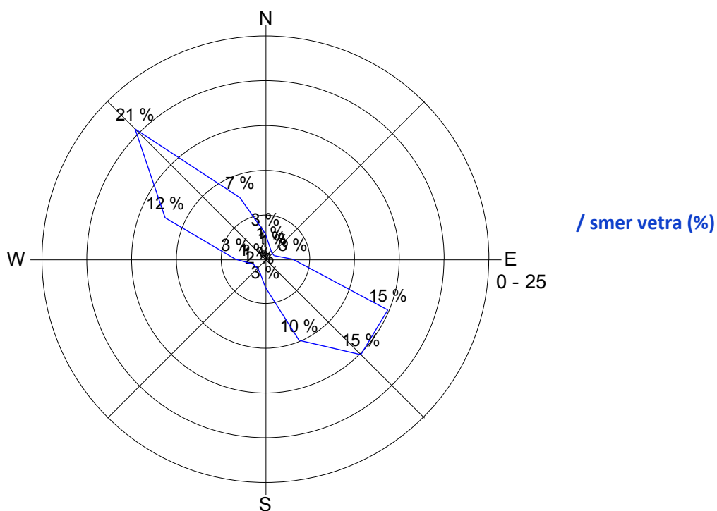
Slika 19: Roža vetrov, februar 2015.
