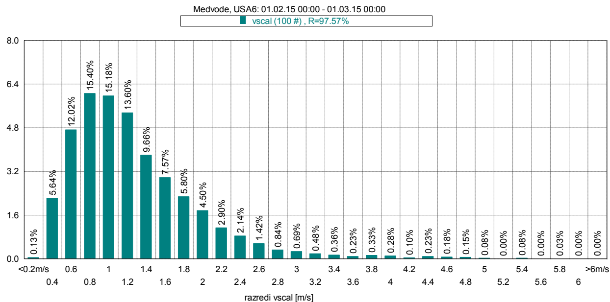
Slika 20: Frekvenčna porazdelitev po hitrosti vetra, februar 2015.
