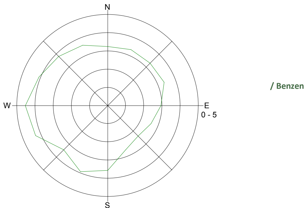
Slika 6: Roža onesnaženosti – benzen, februar 2015.
