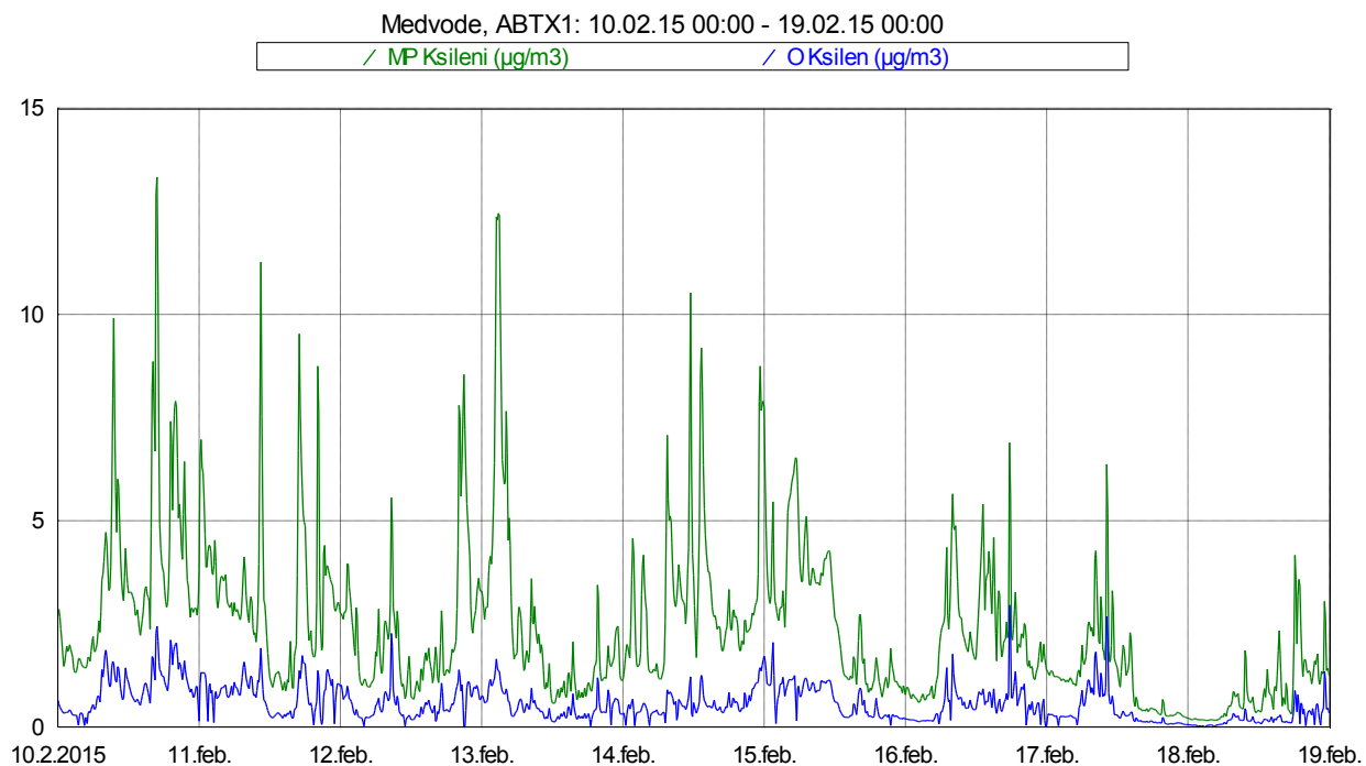
Slika 13: Imisijske koncentracije M&P in O ksilena med 10. 2. 2015 in 18. 2. 2015.
