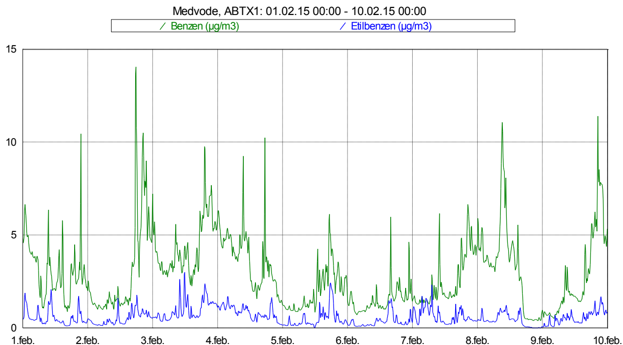
Slika 3: Imisijske koncentracije benzena in etilbenzena med vključno 1. 2. 2015 in 9. 2. 2015.
