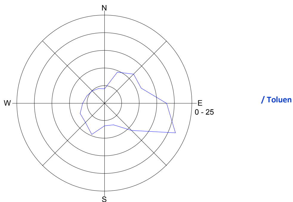
Slika 11: Roža onesnaženost - toluen, februar 2015.
