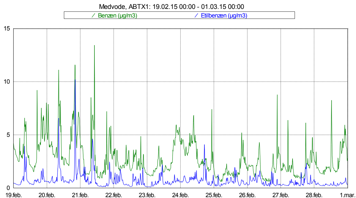
Slika 5: Imisijske koncentracije benzena in etilbenzena med 19. 2. 2015 in 28. 2. 2015.
