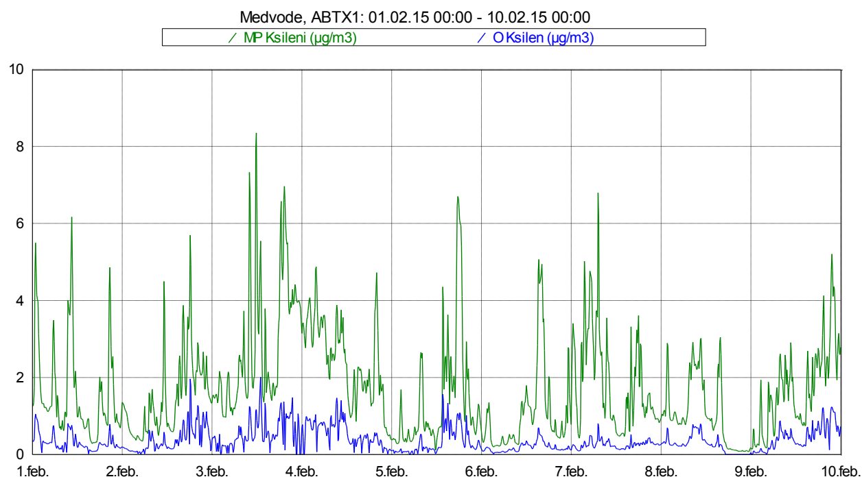
Slika 12: Imisijske koncentracije M&P in O ksilena med vključno 1. 2. 2015 in 9. 2. 2015.
