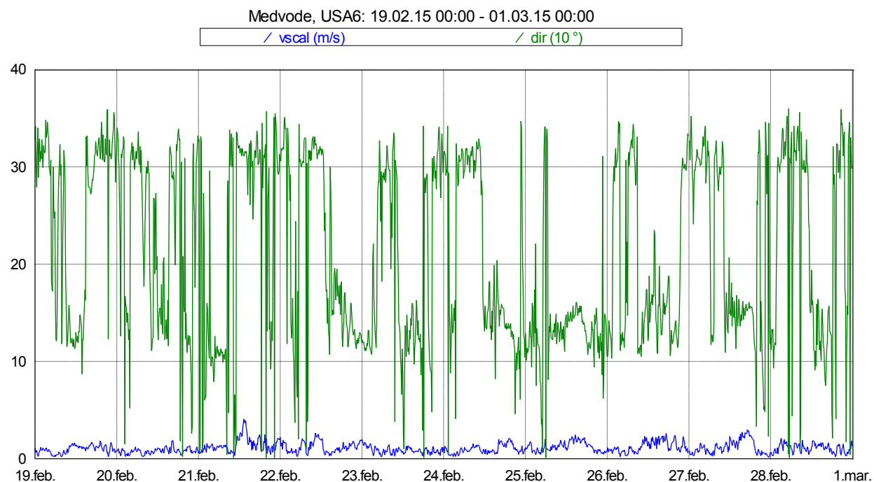
Slika 18: Smer in hitrost vetra med 19. 2. 2015 in 28. 2. 2015.
