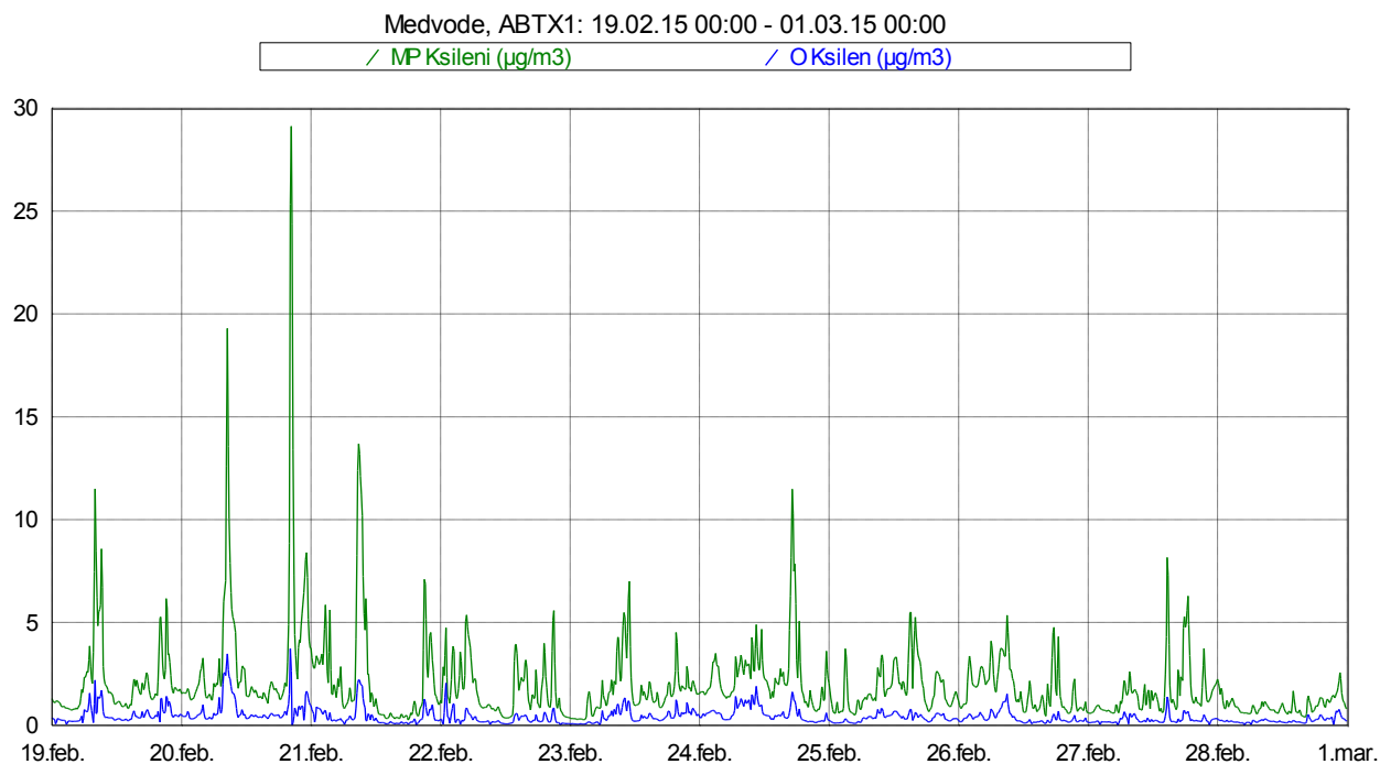
Slika 14: Imisijske koncentracije M&P in O ksilena med 19. 2. 2015 in 28. 2. 2015.
