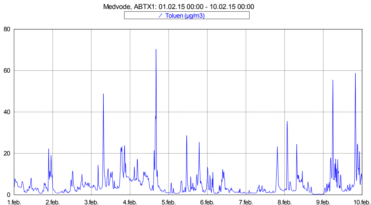
Slika 8: Imisijske koncentracije toluenta med vključno 1. 2. 2015 in 9. 2. 2015.
