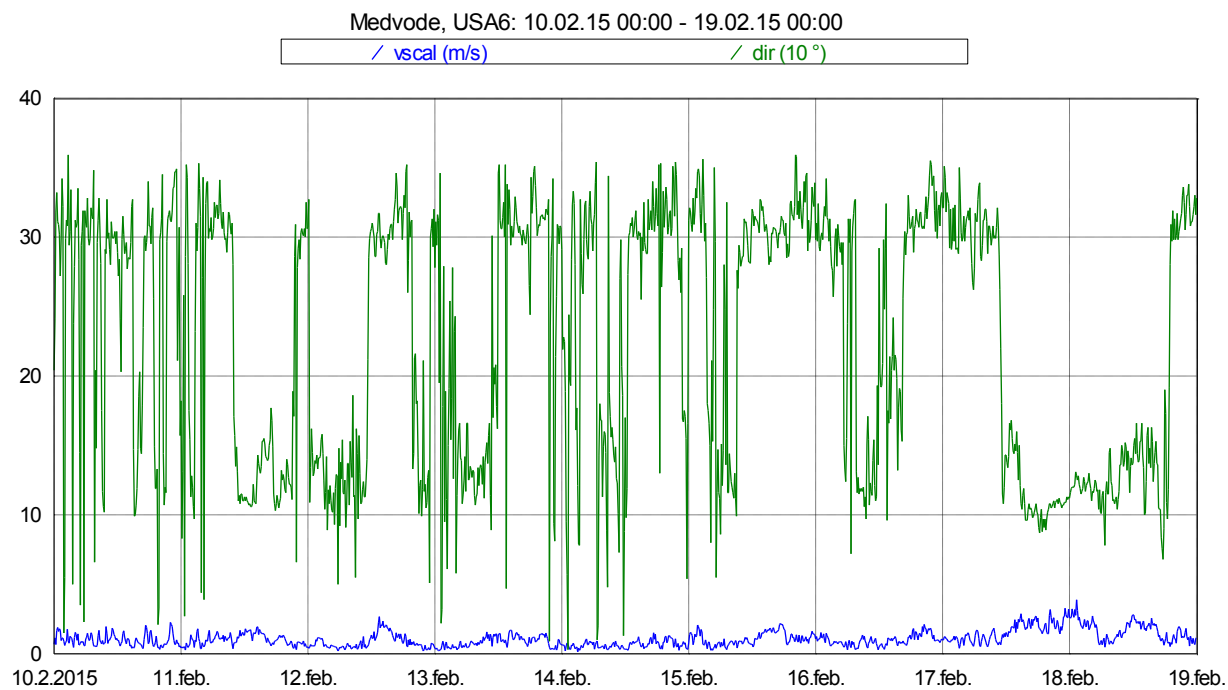
Slika 17: Smer in hitrost vetra med 10. 2. 2015 in 18. 2. 2015.
