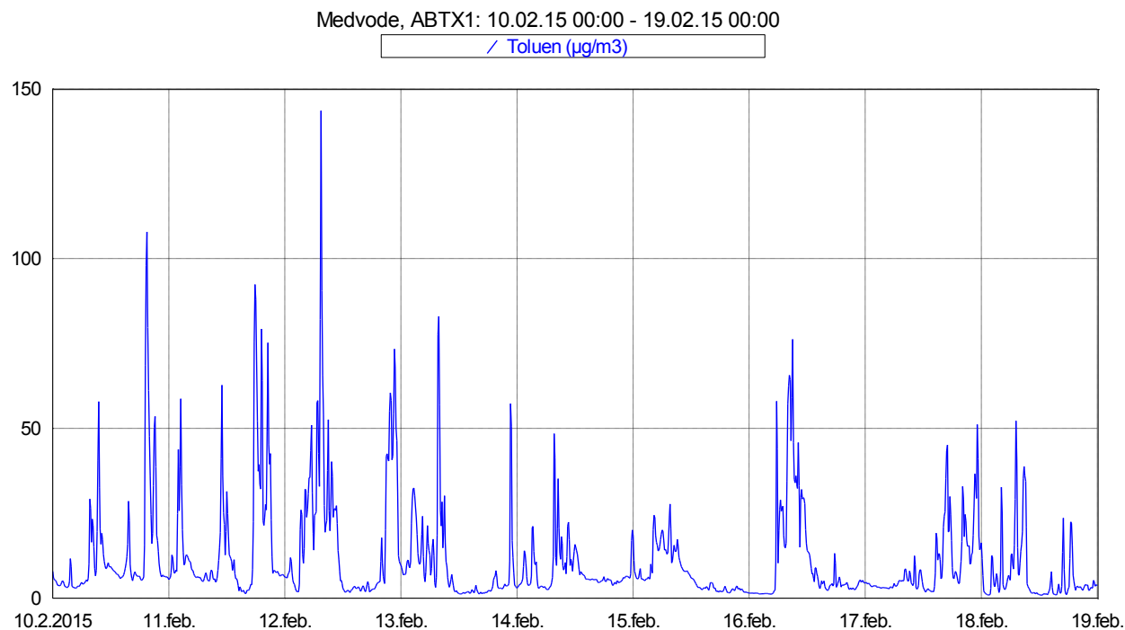
Slika 9: Imisijske koncentracije toluenta med 10. 2. 2015 in 18. 2. 2015.
