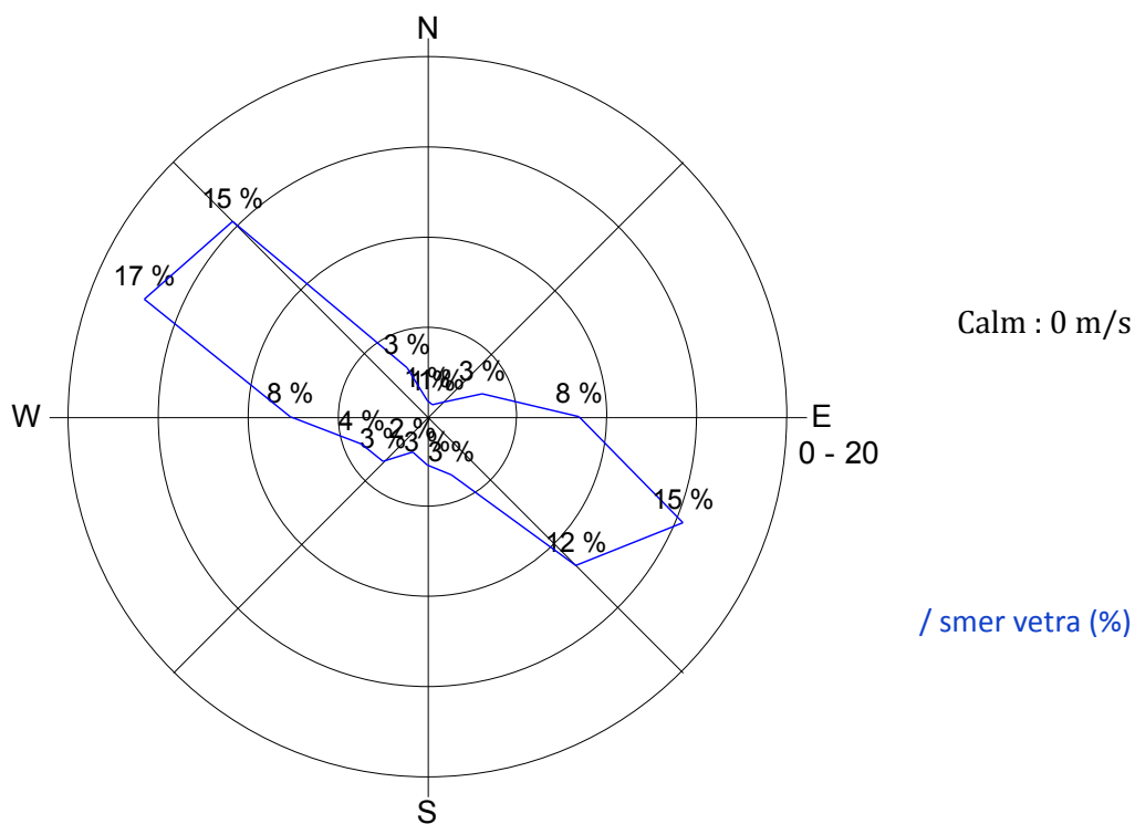
Slika 17: Smer in hitrost vetra med 21. 2. 2013 in 28. 2. 2013.
