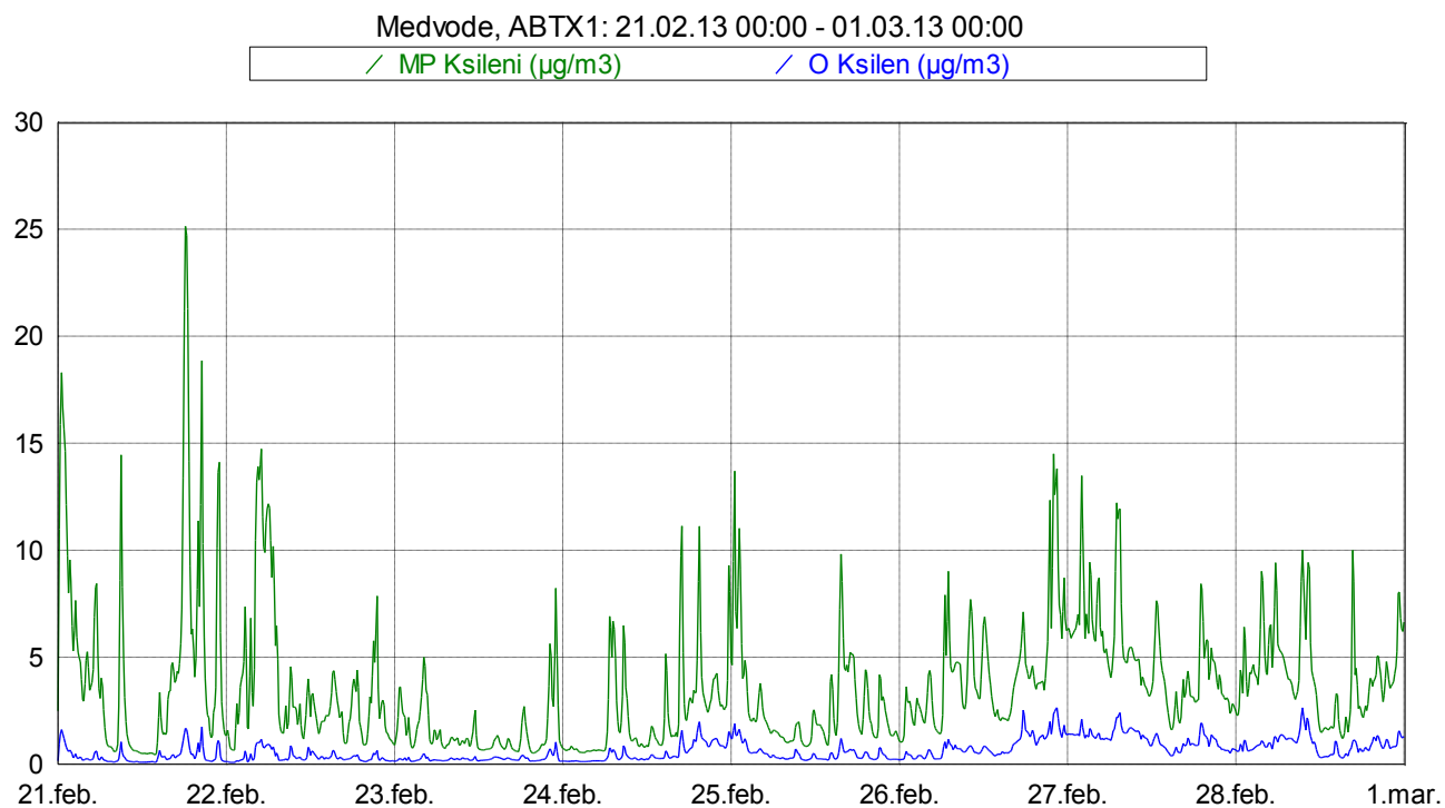
Slika 13: Imisijske koncentracije M&P in O ksilena med 21. 2. 2013 in 28. 2. 2013.
