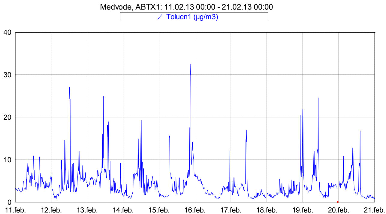
Slika 8: Imisijske koncentracije toluena med 11. 2. 2013 in 21. 2. 2013.
