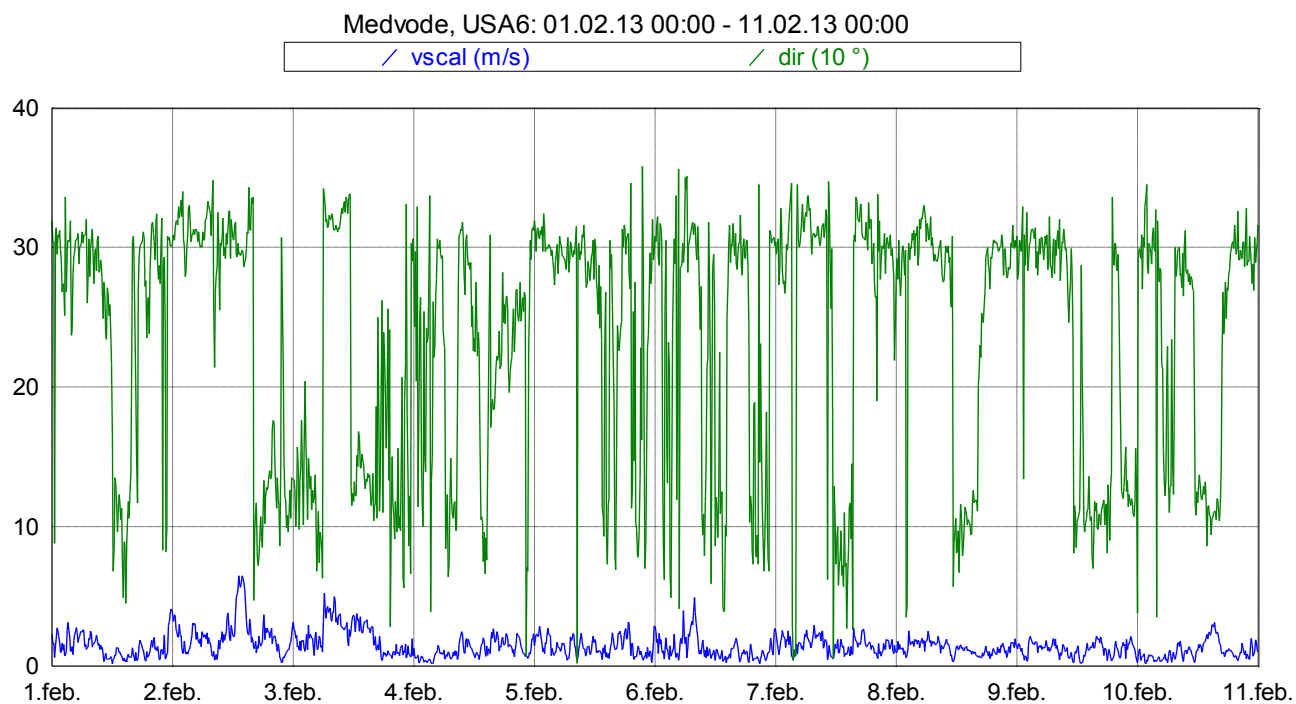
Slika 15: Smer in hitrost vetra med 1. 2. 2013 in 11. 2. 2013.
