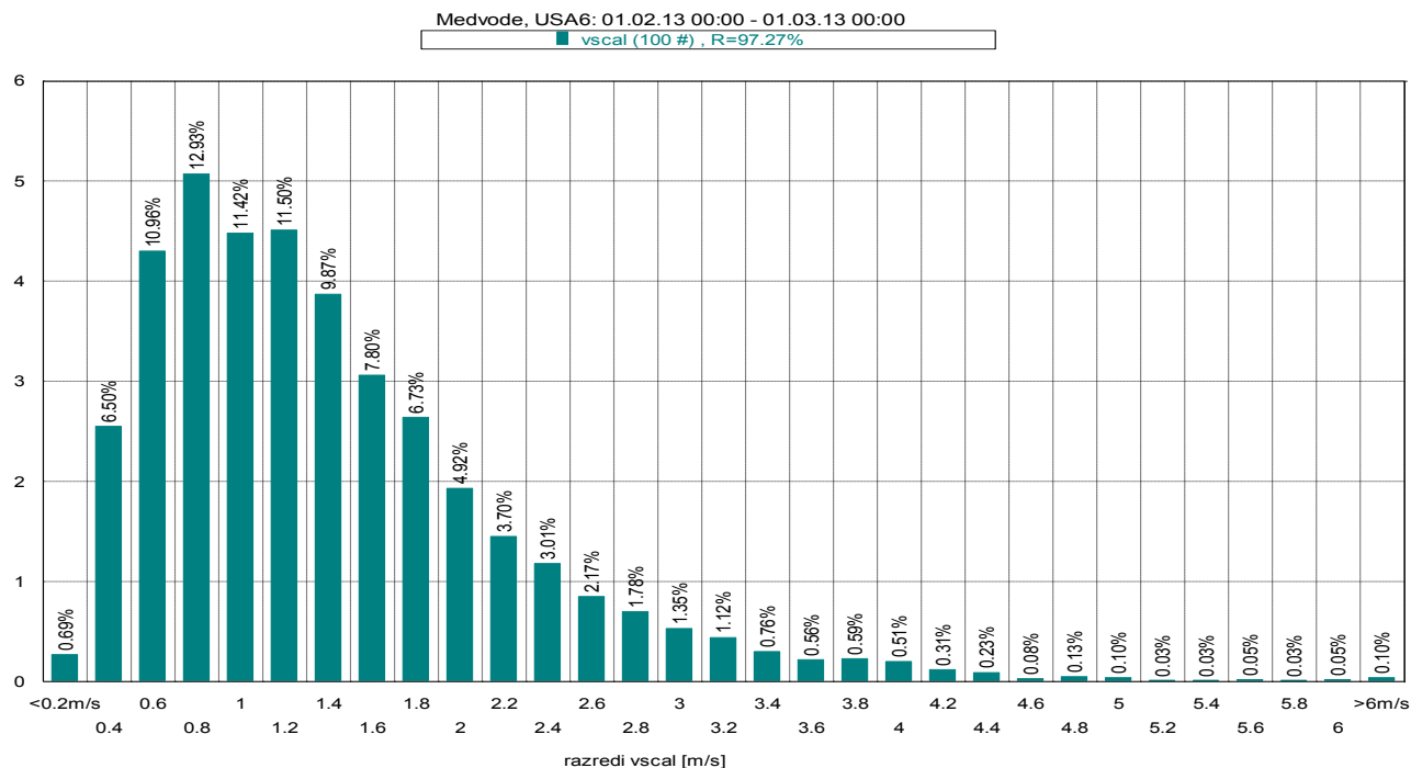
Slika 19: Frekvenčna porazdelitev po hitrosti vetra, februar 2013.
