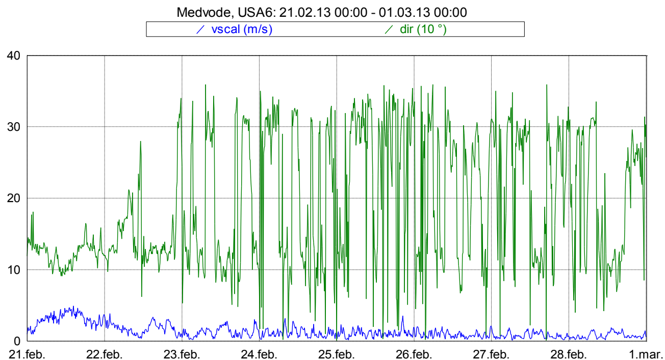
Slika 17: Smer in hitrost vetra med 21. 2. 2013 in 28. 2. 2013.
