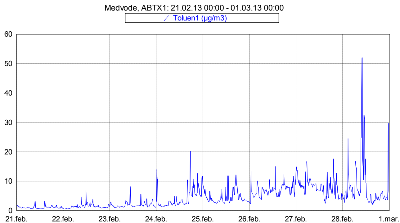
Slika 9: Imisijske koncentracije toluena med 21. 2. 2013 in 28. 2. 2013.
