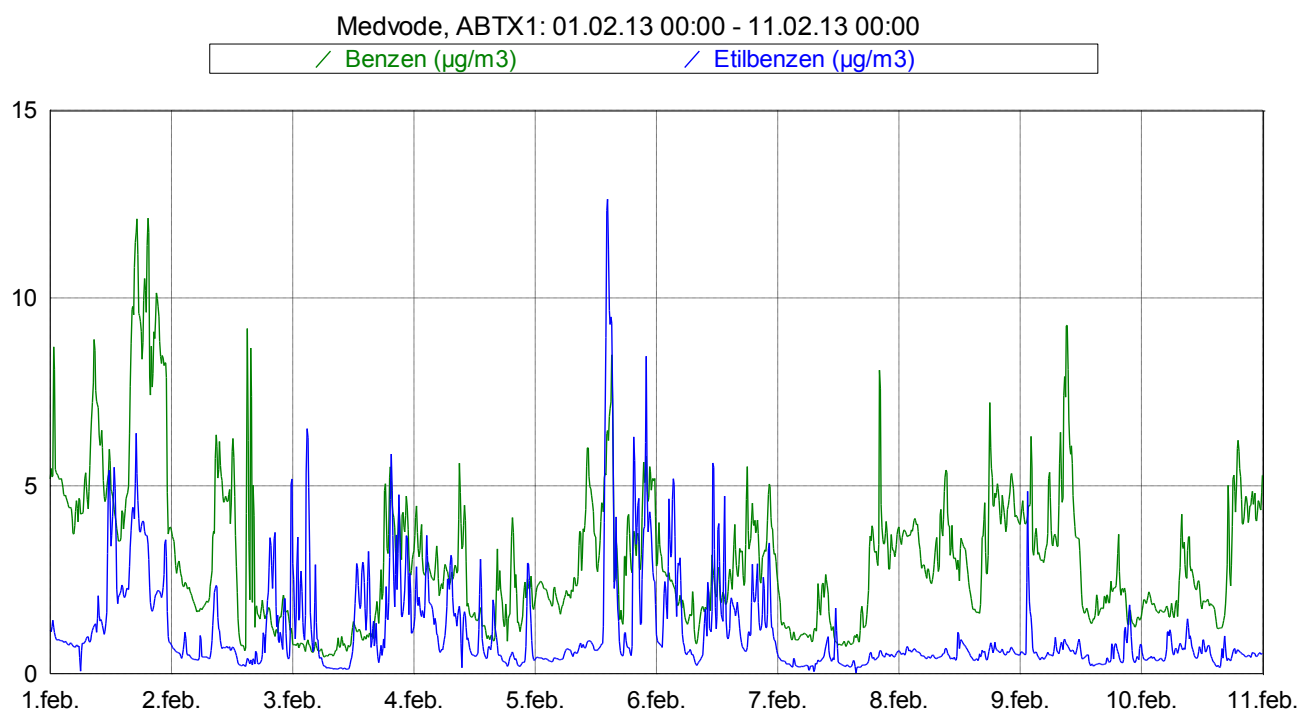
Slika 3: Imisijske koncentracije benzena in etilbenzena med vključno 1. 2. 2013 in 11. 2. 2013.
