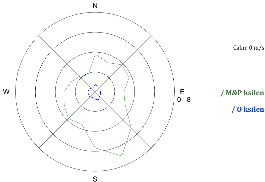
Slika 14: Roža onesnaženosti - M & P ksilen in O ksilen, februar 2013.
