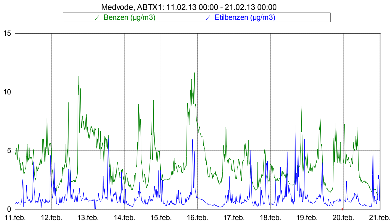
Slika 4: Imisijske koncentracije benzena in etilbenzena med 11. 2. 2013 in 21. 2. 2013.
