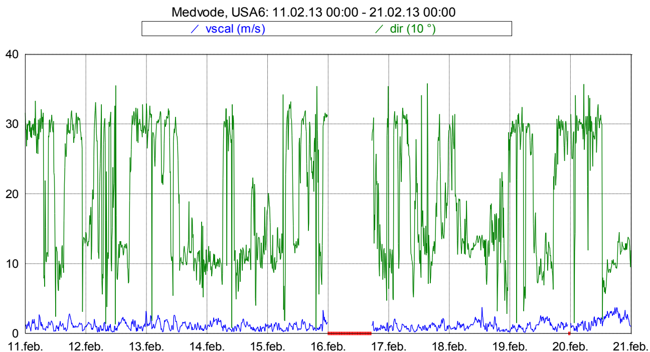
Slika 16: Smer in hitrost vetra med 11. 2. 2013 in 21. 2. 2013.
