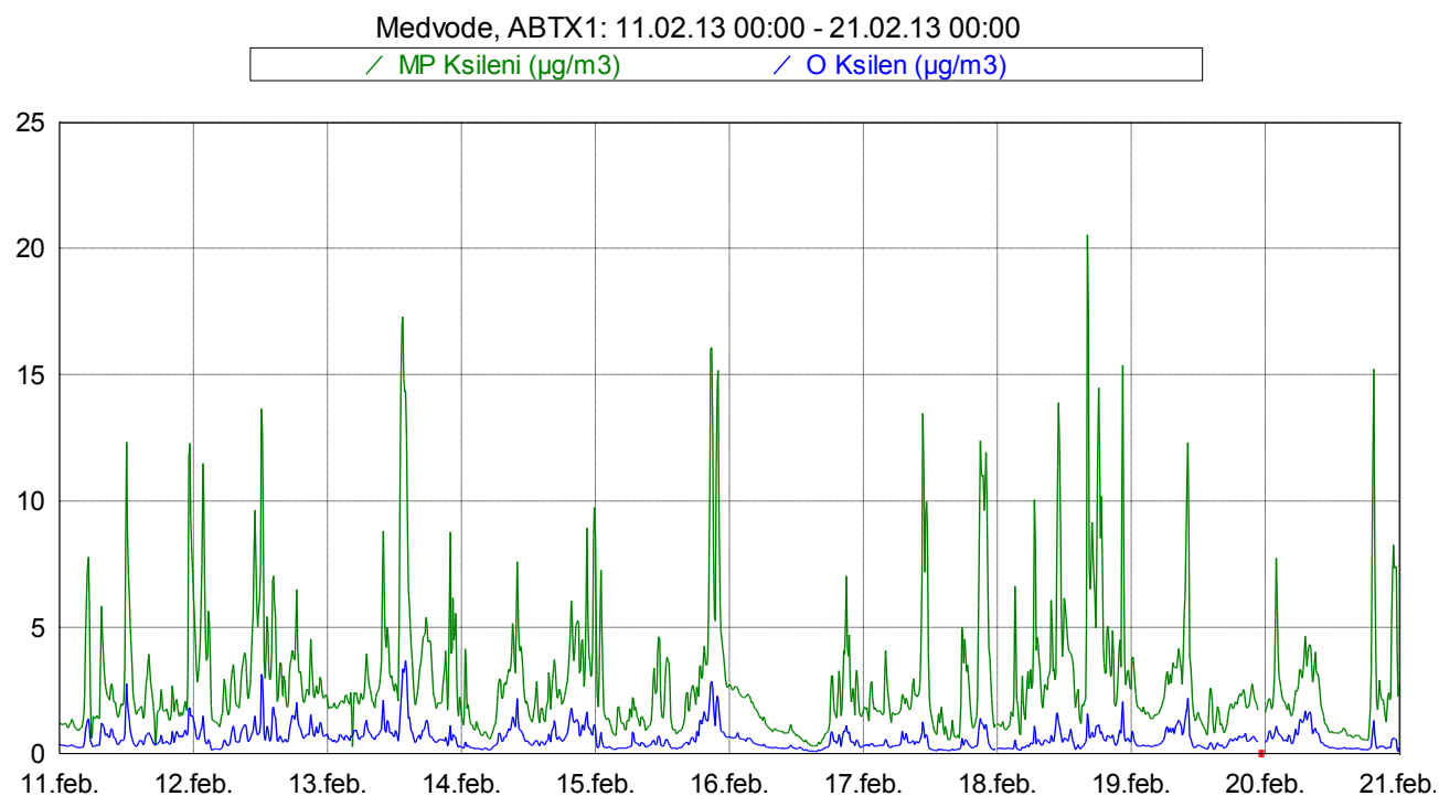
Slika 12: Imisijske koncentracije M&P in O ksilena med 11. 2. 2013 in 21. 2. 2013.
