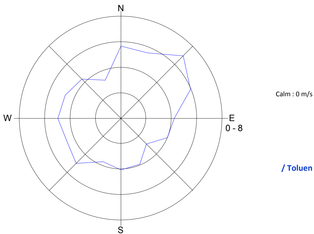
Slika 10: Roža onesnaženost - toluen, februar 2013.
