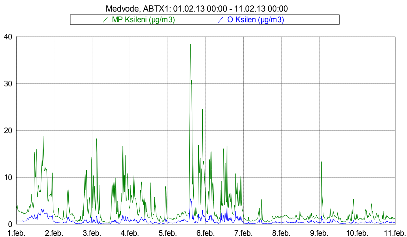
Slika 11: Imisijske koncentracije M&P in O ksilena med vključno 1. 2. 2013 in 11. 2. 2013.
