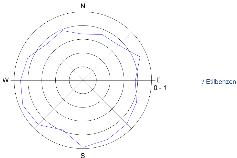
Slika 7: Roža onesnaženosti – etilbenzen, december 2017.
