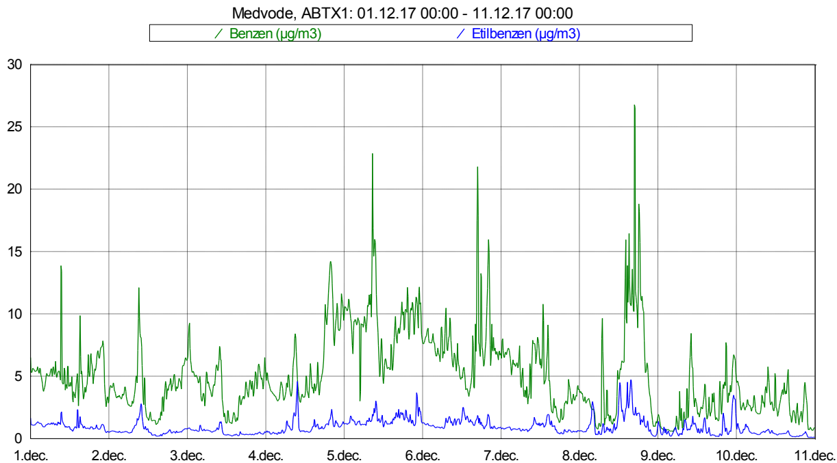
Slika 3: Imisijske koncentracije benzena in etilbenzena med vključno 1. 12. in 10. 12. 2017.
