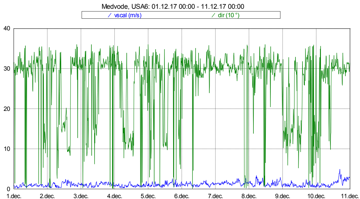
Slika 16: Smer in hitrost vetra med 1. 12. in 10. 12. 2017.
