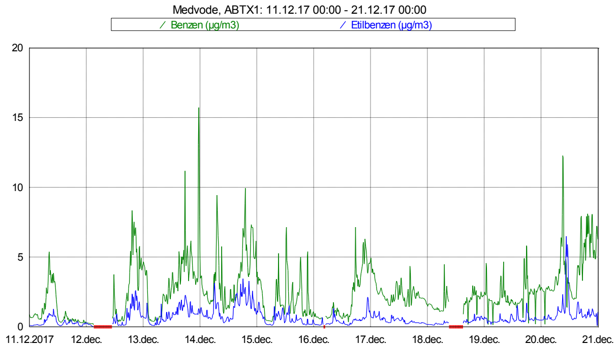
Slika 4: Imisijske koncentracije benzena in etilbenzena med vključno 11. 12. in 20. 12. 2017.
