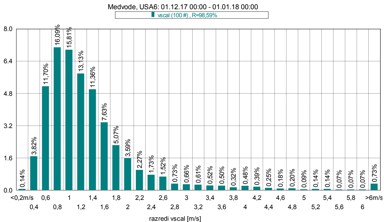
Slika 20: Frekvenčna porazdelitev po hitrosti vetra, december 2017.
