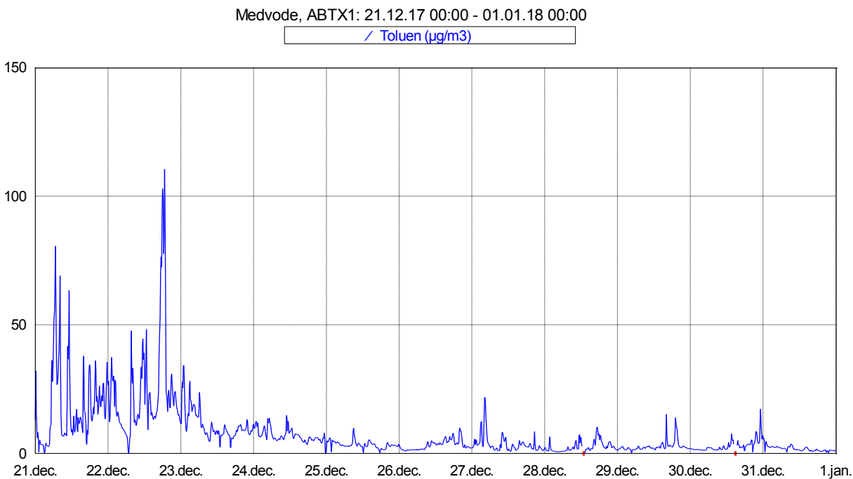
Slika 10: Imisijske koncentracije toluena med vključno 21. 12. in 31. 12. 2017.
