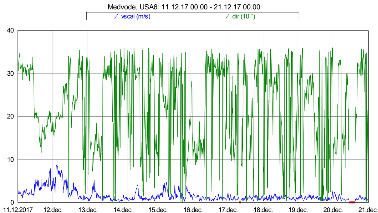
Slika 17: Smer in hitrost vetra med 11. 12. in 20. 12. 2017.
