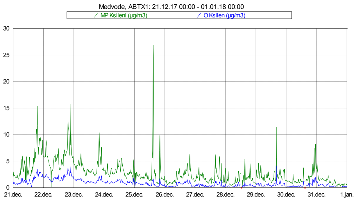
Slika 14: Imisijske koncentracije ksilenov med vključno 21. 12. in 31. 12. 2017.
