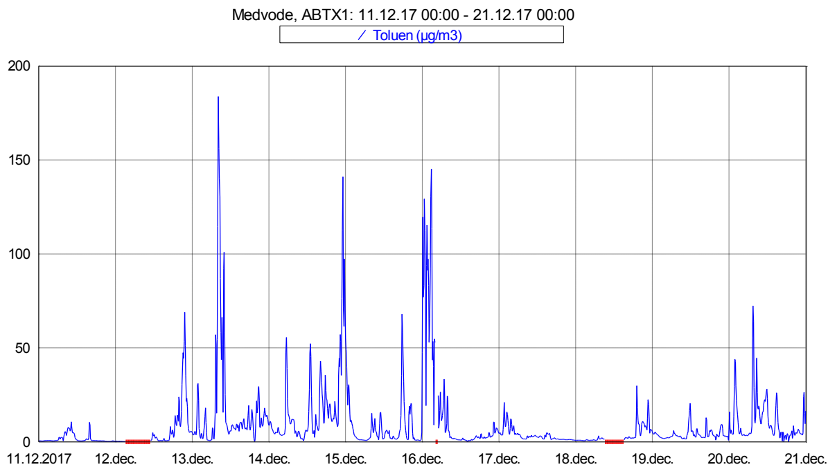
Slika 9: Imisijske koncentracije toluena med vključno 11. 12. in 20. 12. 2017.
