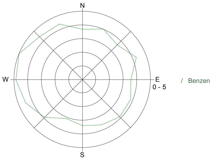
Slika 6: Roža onesnaženosti – benzen, december 2017.
