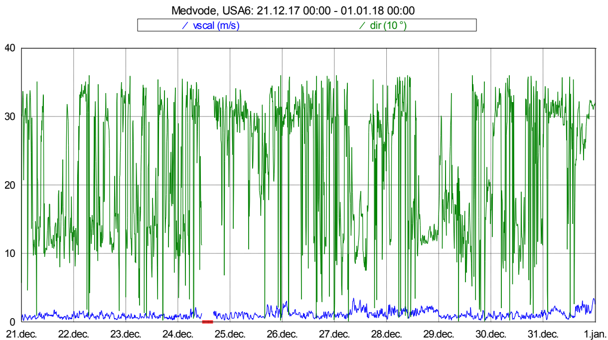
Slika 18: Smer in hitrost vetra med 21. 12. in 31. 12. 2017.
