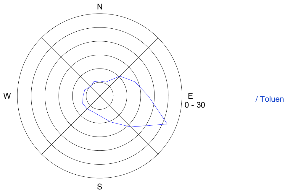
Slika 11: Roža onesnaženosti – toluen, december 2017.
