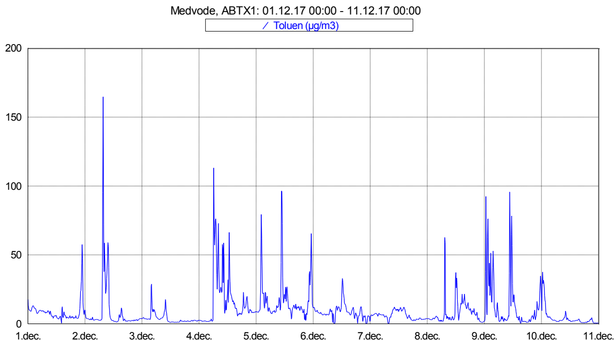
Slika 8: Imisijske koncentracije toluena med vključno 1. 12. in 10. 12. 2017.
