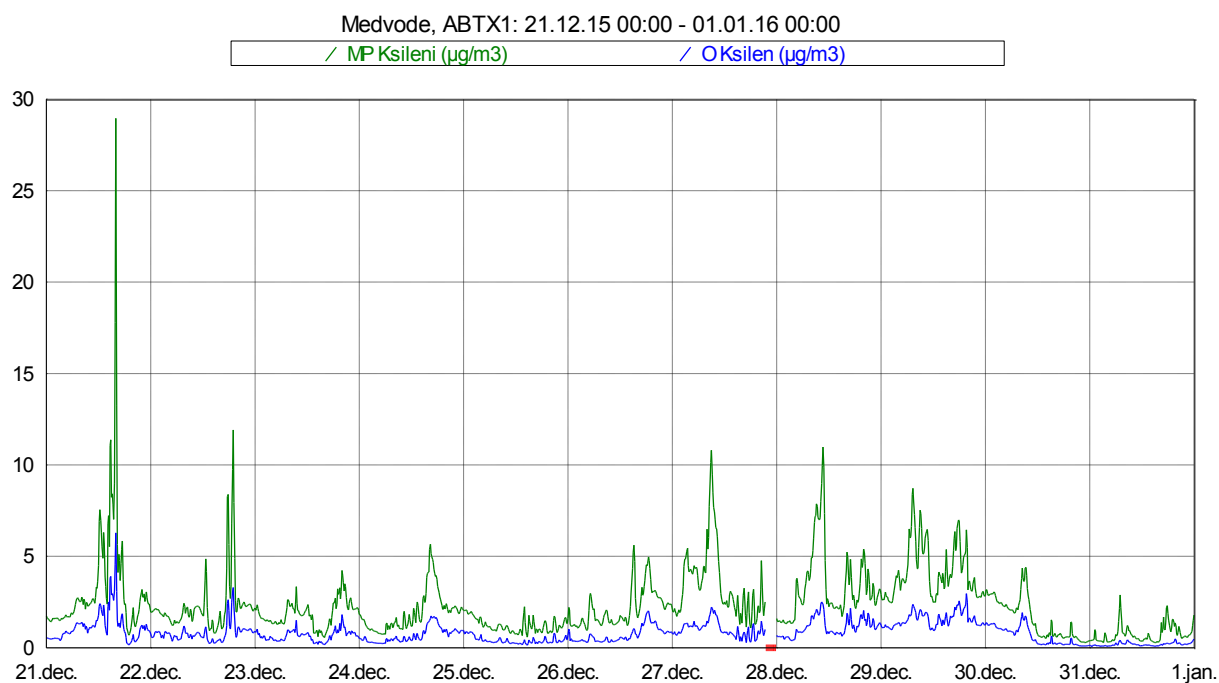
Slika 14: Imisijske koncentracije M&P in O ksilena med 21. 12. 2015 in 31. 12. 2015.
