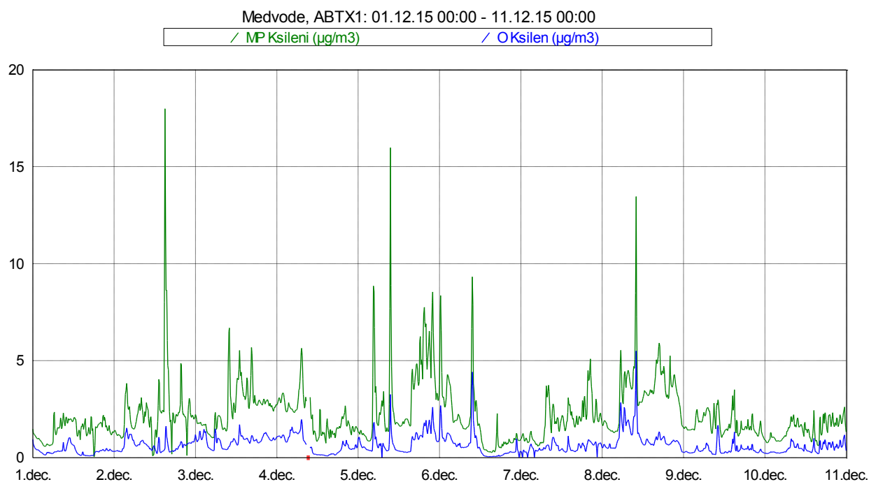
Slika 12: Imisijske koncentracije M&P in O ksilena med vključno 1. 12. 2015 in 10. 12. 2015.
