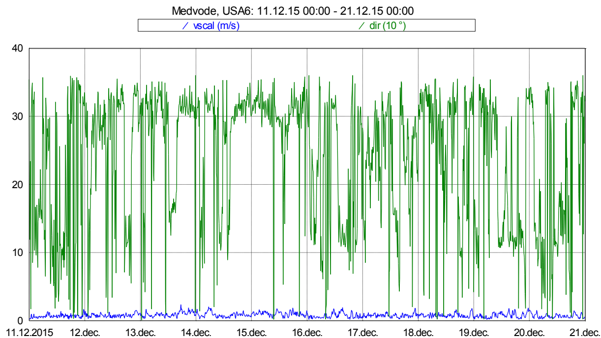
Slika 17: Smer in hitrost vetra med 11. 12. 2015 in 20. 12. 2015.
