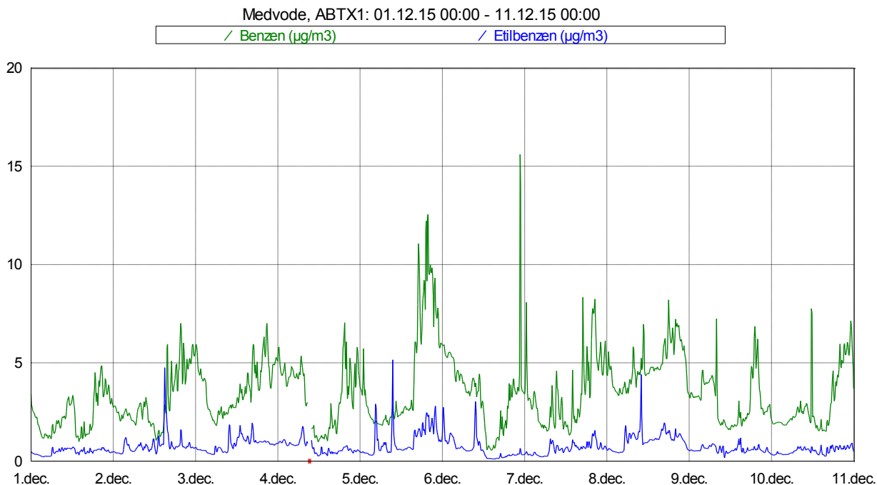
Slika 3: Imisijske koncentracije benzena in etilbenzena med vključno 1. 12. 2015 in 10. 12. 2015.
