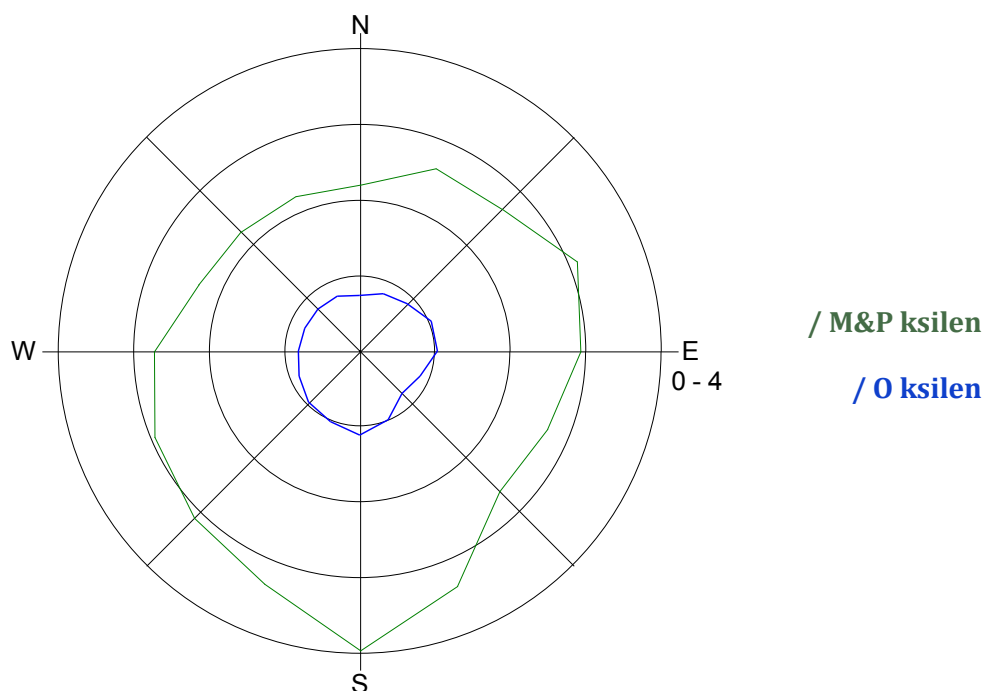
Slika 15: Roža onesnaženosti - M & P ksilen in O ksilen, december 2015.
