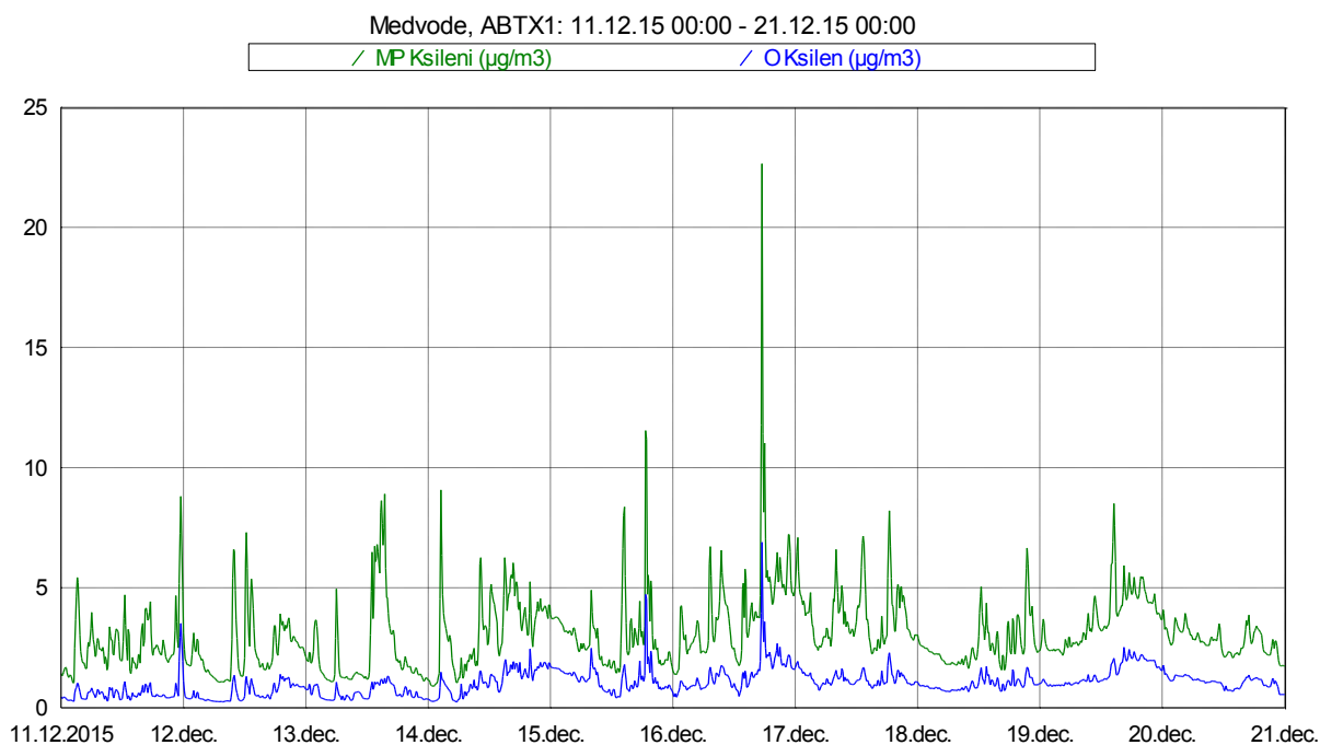
Slika 13: Imisijske koncentracije M&P in O ksilena med 11. 12. 2015 in 20. 12. 2015.
