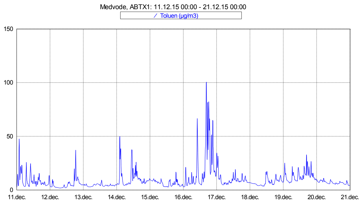
Slika 9: Imisijske koncentracije toluenta med 11. 12. 2015 in 20. 12. 2015.
