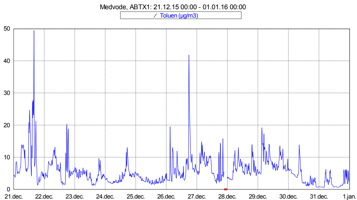
Slika 10: Imisijske koncentracije toluena med 21. 12. 2015 in 31. 12. 2015.
