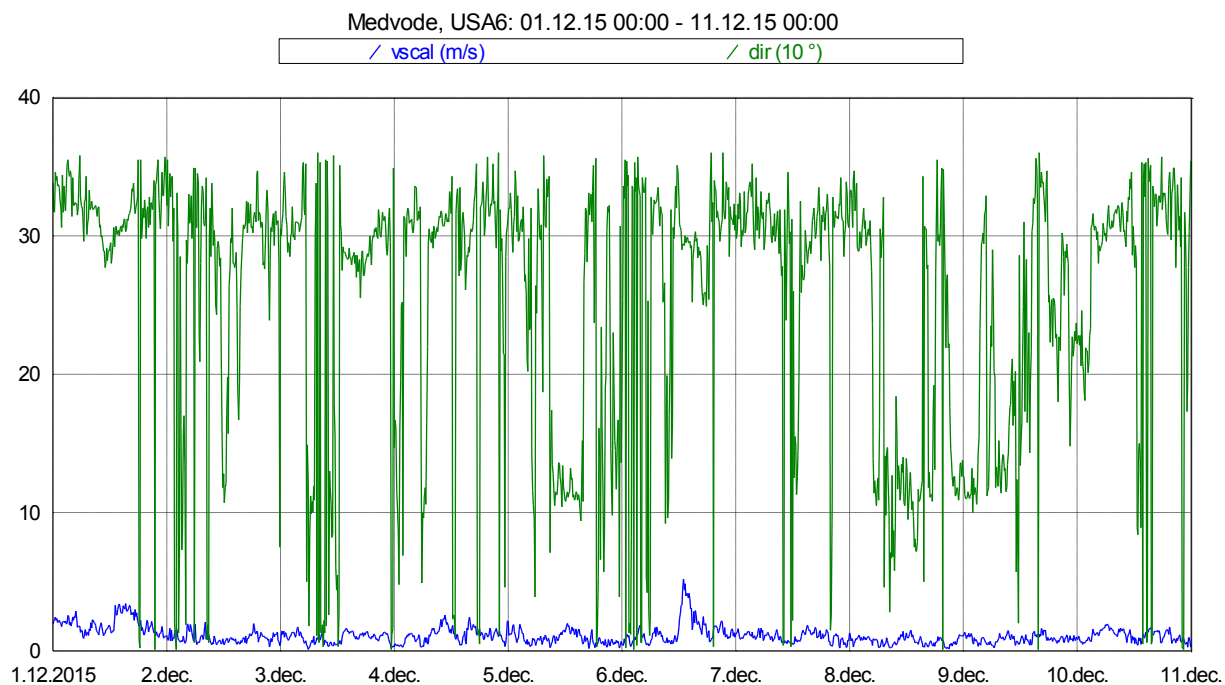
Slika 16: Smer in hitrost vetra med 1. 12. 2015 in 10. 12. 2015.
