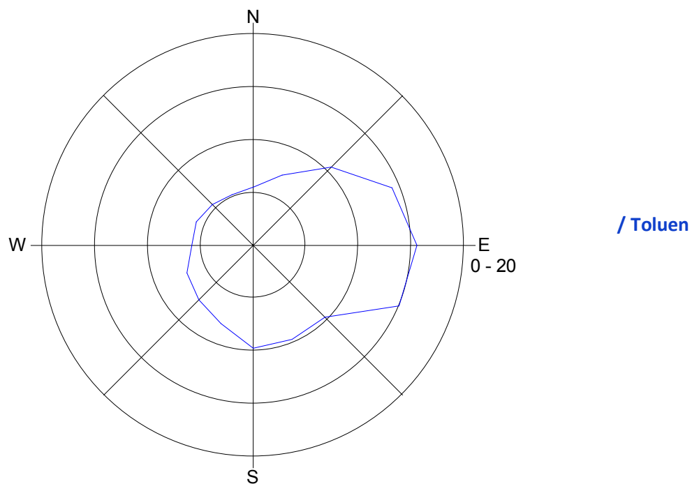
Slika 11: Roža onesnaženost - toluen, december 2015.
