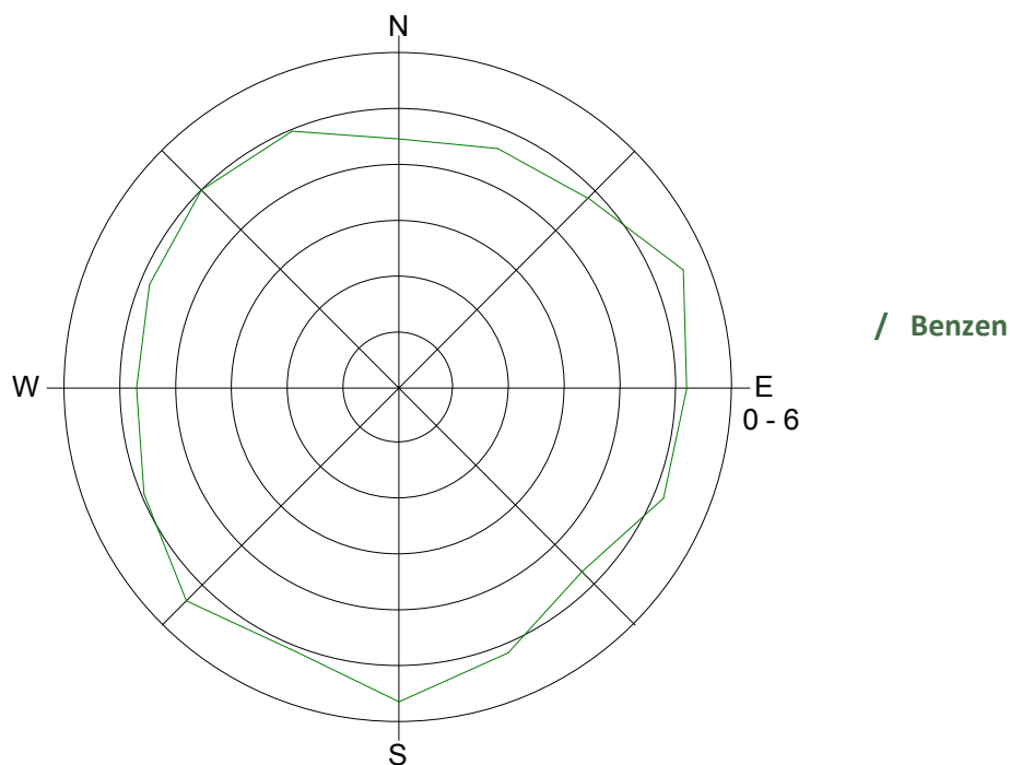
Slika 6: Roža onesnaženosti – benzen, december 2015.
