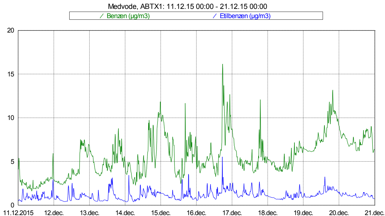
Slika 4: Imisijske koncentracije benzena in etilbenzena med 11. 12. 2015 in 20. 12. 2015.
