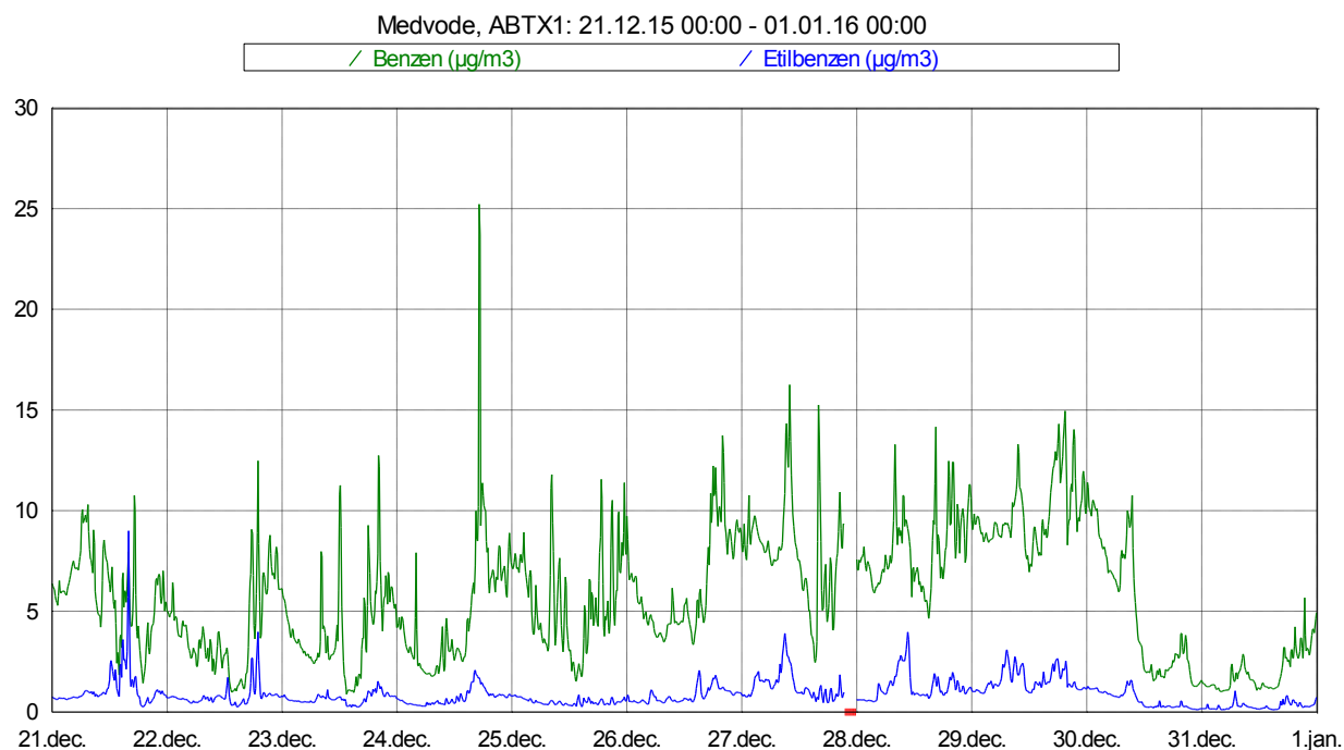
Slika 5: Imisijske koncentracije benzena in etilbenzena med 21. 12. 2015 in 31. 12. 2015.
