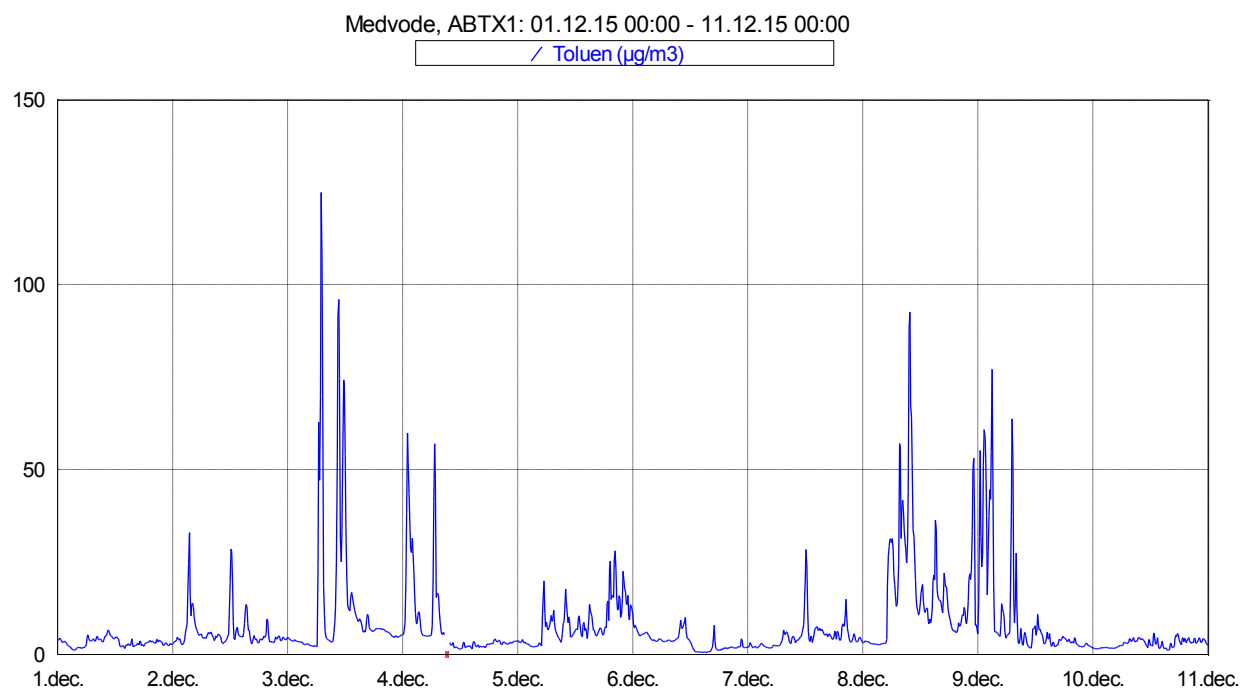
Slika 8: Imisijske koncentracije toluenta med vključno 1. 12. 2015 in 10. 12. 2015.
