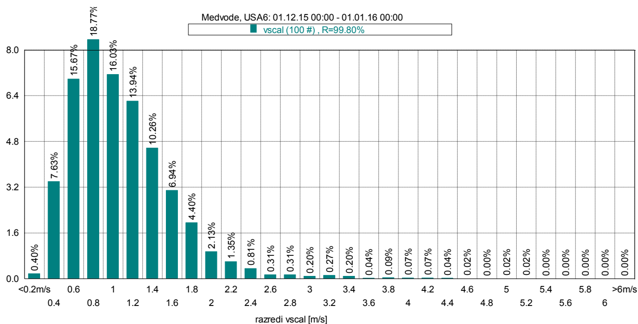
Slika 20: Frekvenčna porazdelitev po hitrosti vetra, december 2015.
