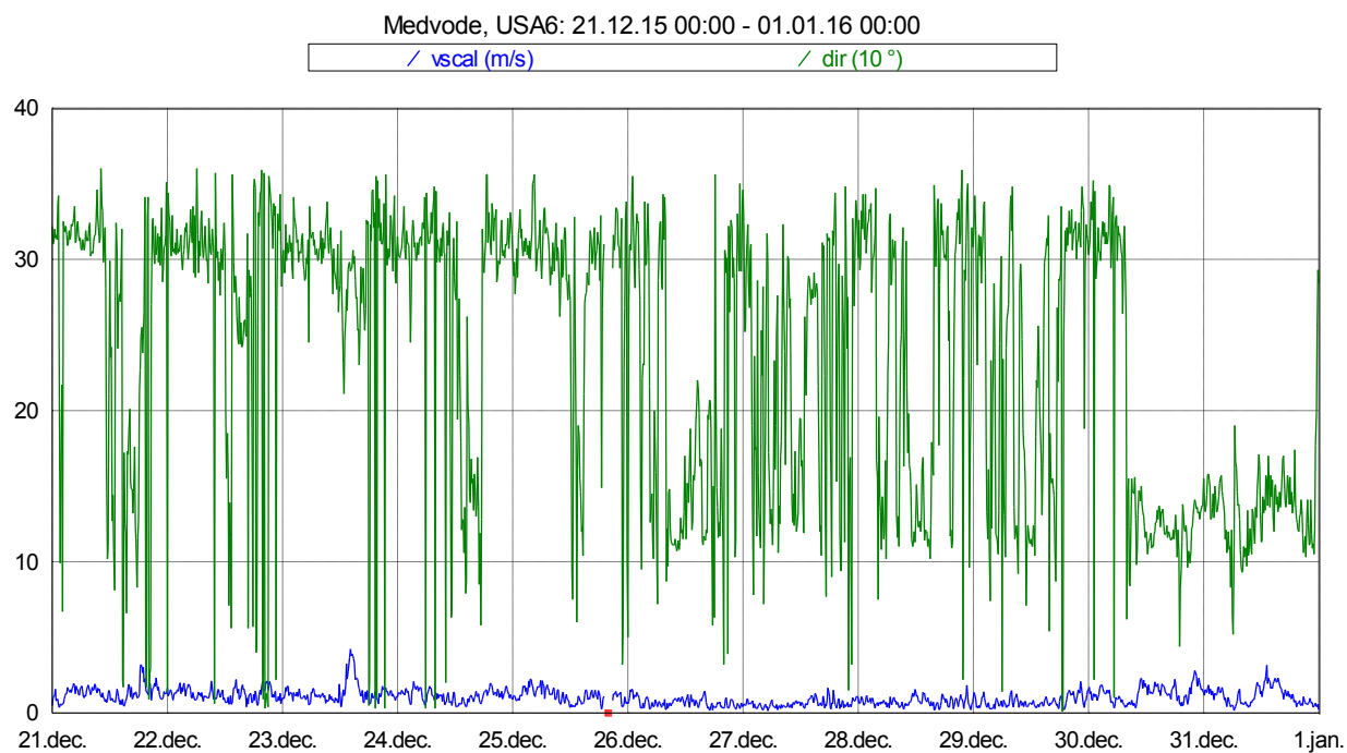
Slika 18: Smer in hitrost vetra med 21. 12. 2015 in 31. 12. 2015.
