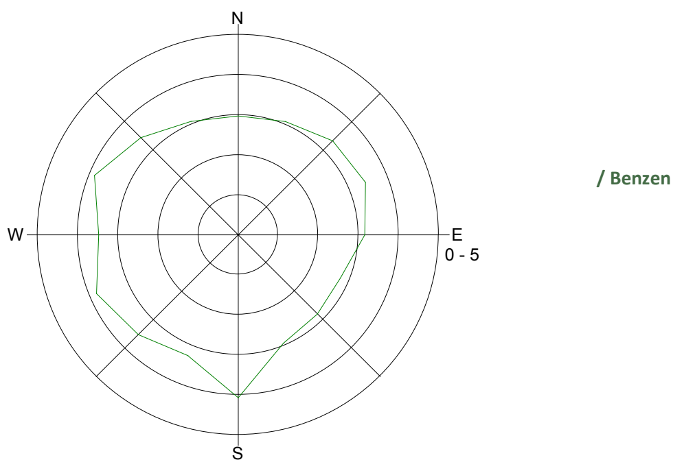
Slika 6: Roža onesnaženosti – benzen, december 2014.
