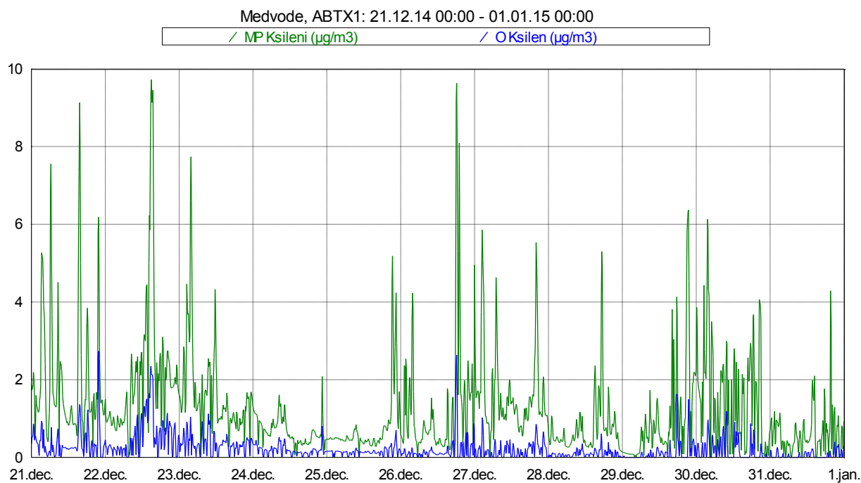
Slika 14: Imisijske koncentracije M&P in O ksilena med 21. 12. 2014 in 30. 12. 2014.
