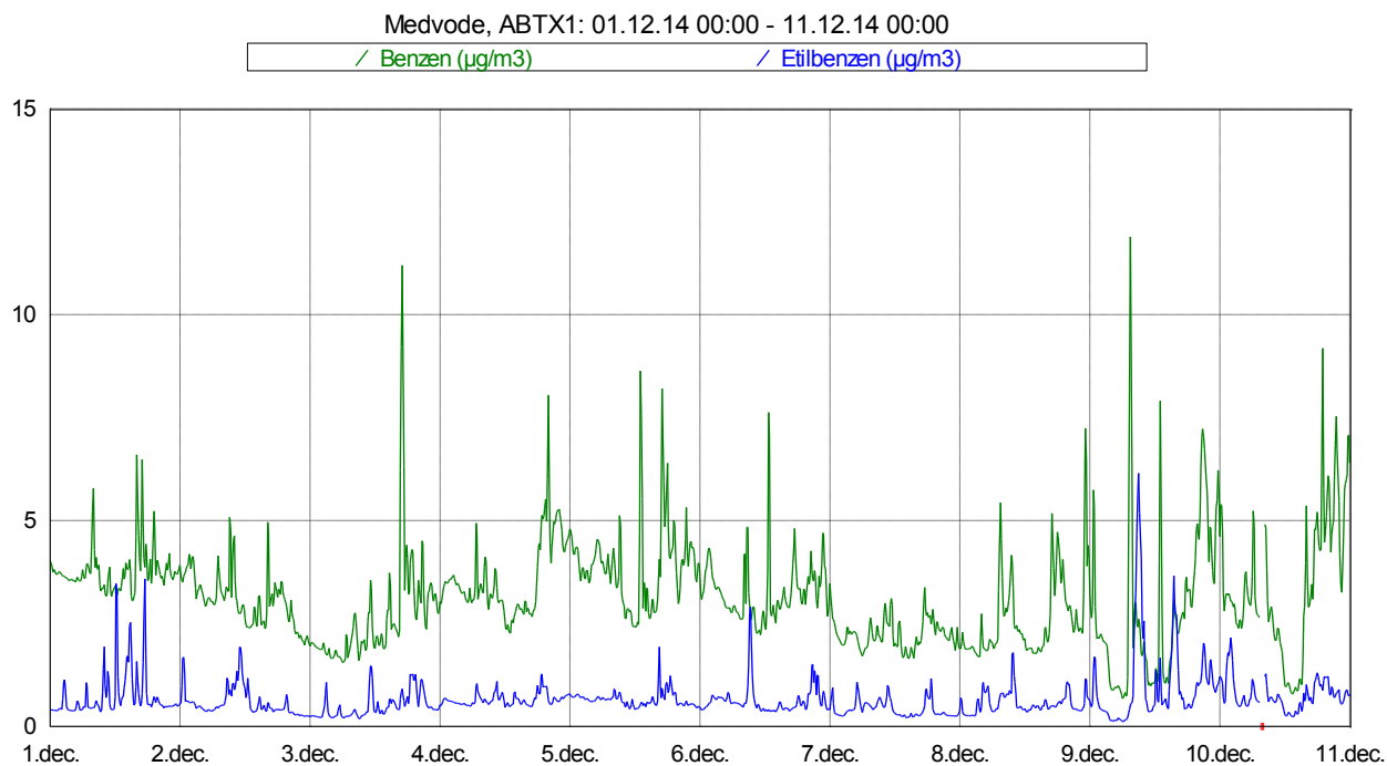
Slika 3: Imisijske koncentracije benzena in etilbenzena med vključno 1. 12. 2014 in 10. 12. 2014.
