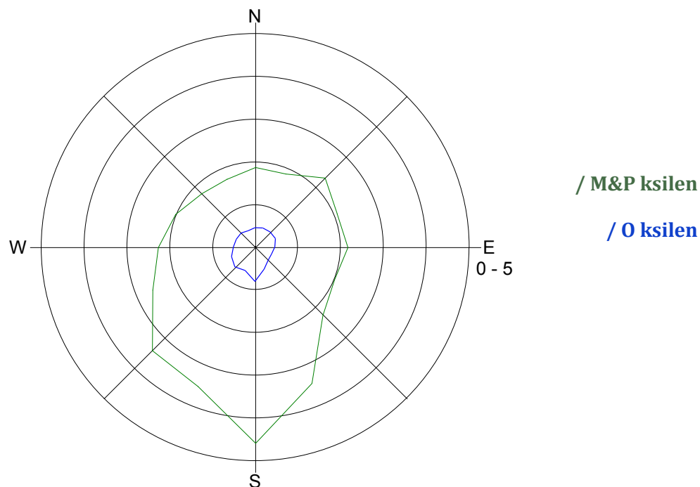
Slika 15: Roža onesnaženosti - M & P ksilen in O ksilen, december 2014.
