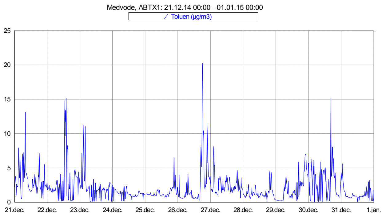
Slika 10: Imisijske koncentracije toluenta med 21. 12. 2014 in 31. 12. 2014.
