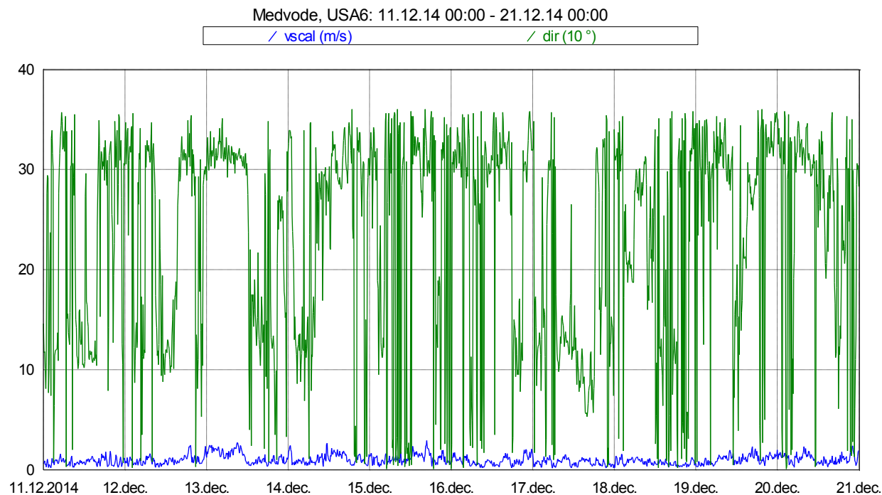
Slika 17: Smer in hitrost vetra med 11. 12. 2014 in 20. 12. 2014.
