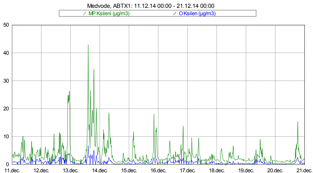
Slika 13: Imisijske koncentracije M&P in O ksilena med 11. 12. 2014 in 20. 12. 2014.
