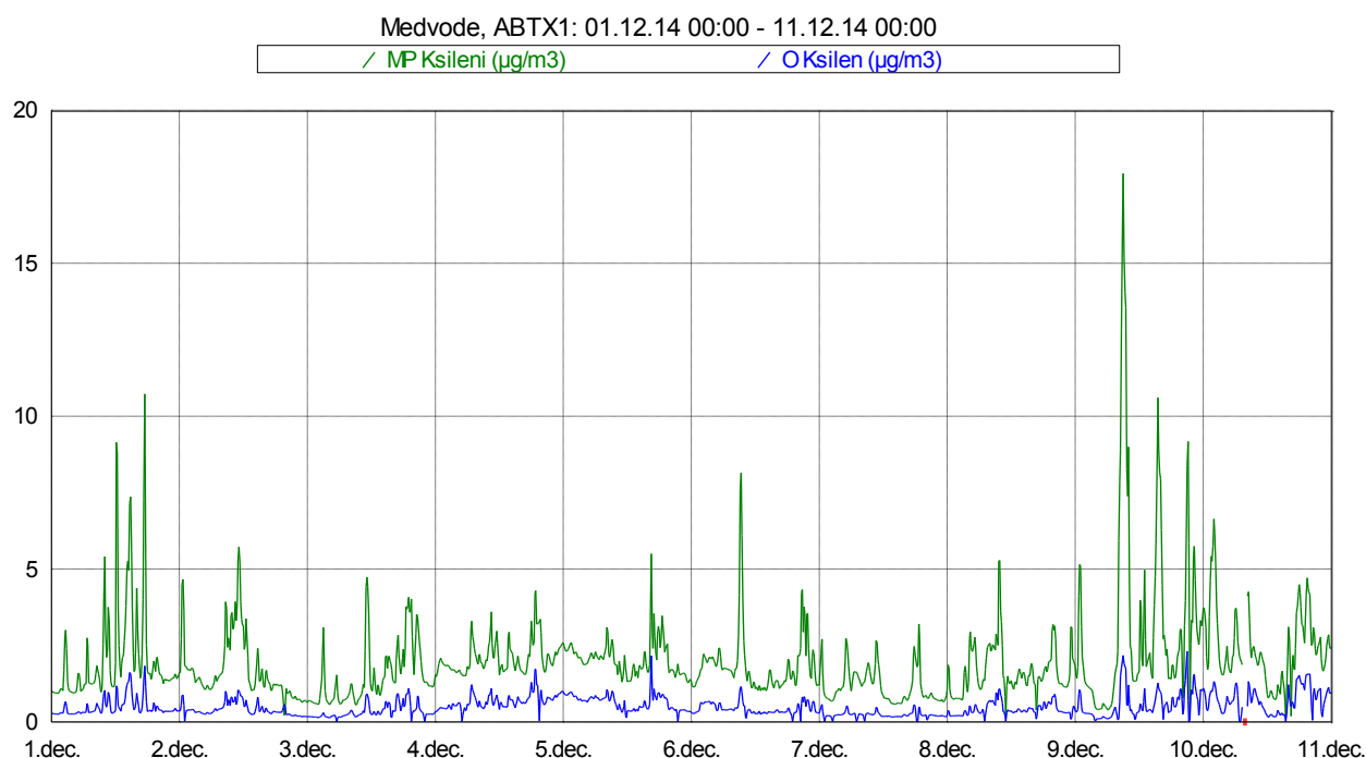
Slika 12: Imisijske koncentracije M&P in O ksilena med vključno 1. 12. 2014 in 10. 12. 2014.
