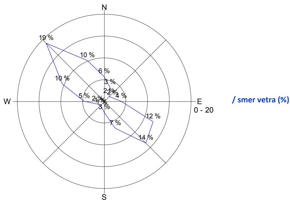
Slika 18: Smer in hitrost vetra med 21. 12. 2014 in 31. 12. 2014.
