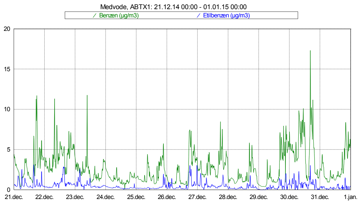
Slika 5: Imisijske koncentracije benzena in etilbenzena med 21. 12. 2014 in 31. 12. 2014.
