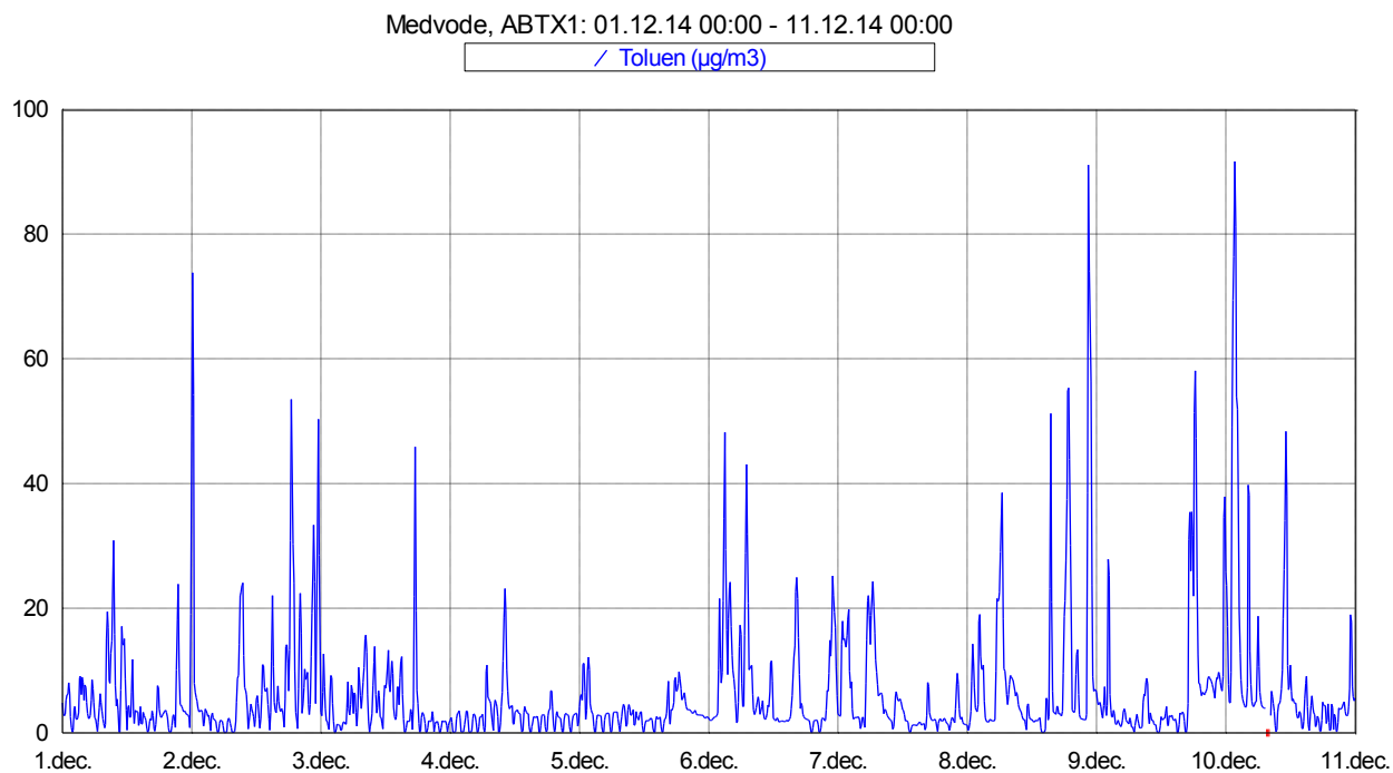
Slika 8: Imisijske koncentracije toluena med vključno 1. 12. 2014 in 10. 12. 2014.
