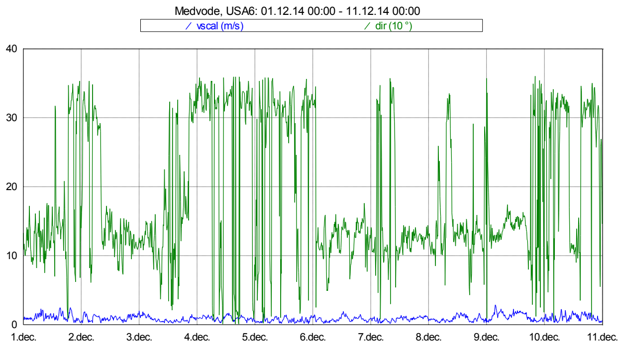
Slika 16: Smer in hitrost vetra med 1. 12. 2014 in 10. 12. 2014.
