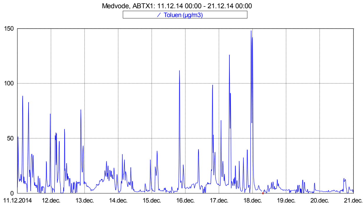
Slika 9: Imisijske koncentracije toluena med 11. 12. 2014 in 20. 12. 2014.
