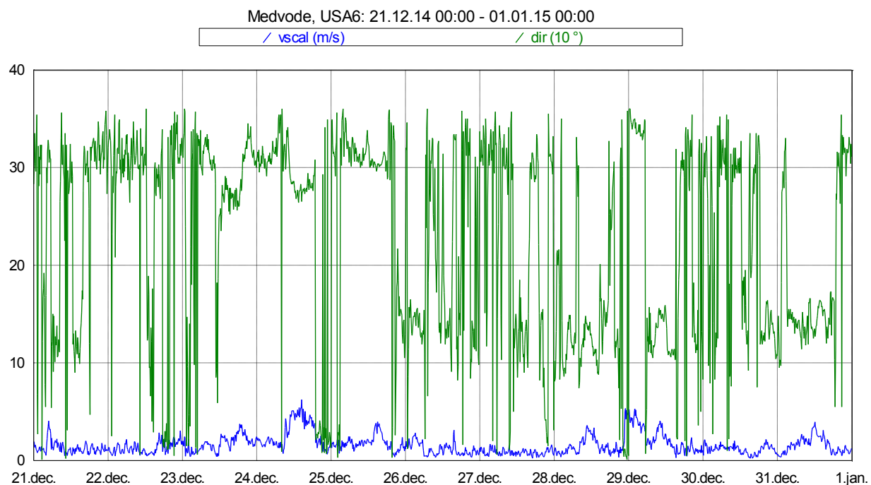
Slika 18: Smer in hitrost vetra med 21. 12. 2014 in 31. 12. 2014.
