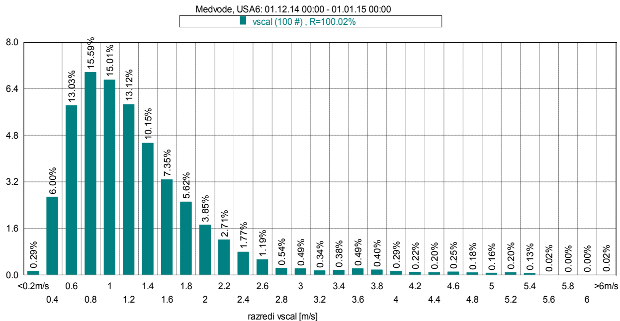
Slika 20: Frekvenčna porazdelitev po hitrosti vetra, december 2014.
