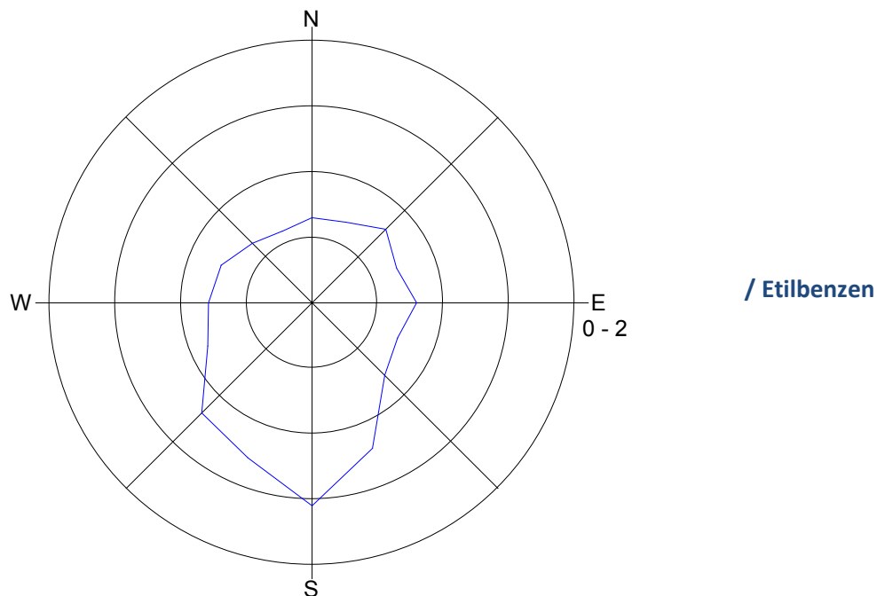
Slika 7: Roža onesnaženosti – etilbenzen, december 2014.
