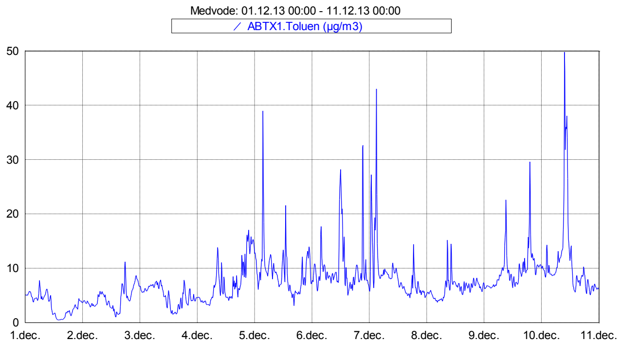
Slika 8: Imisijske koncentracije toluena med vključno 1. 12. 2013 in 10. 12. 2013.
