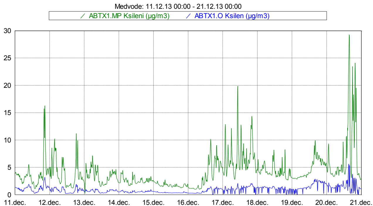
Slika 13: Imisijske koncentracije M&P in O ksilena med 11. 12. 2013 in 20. 12. 2013.
