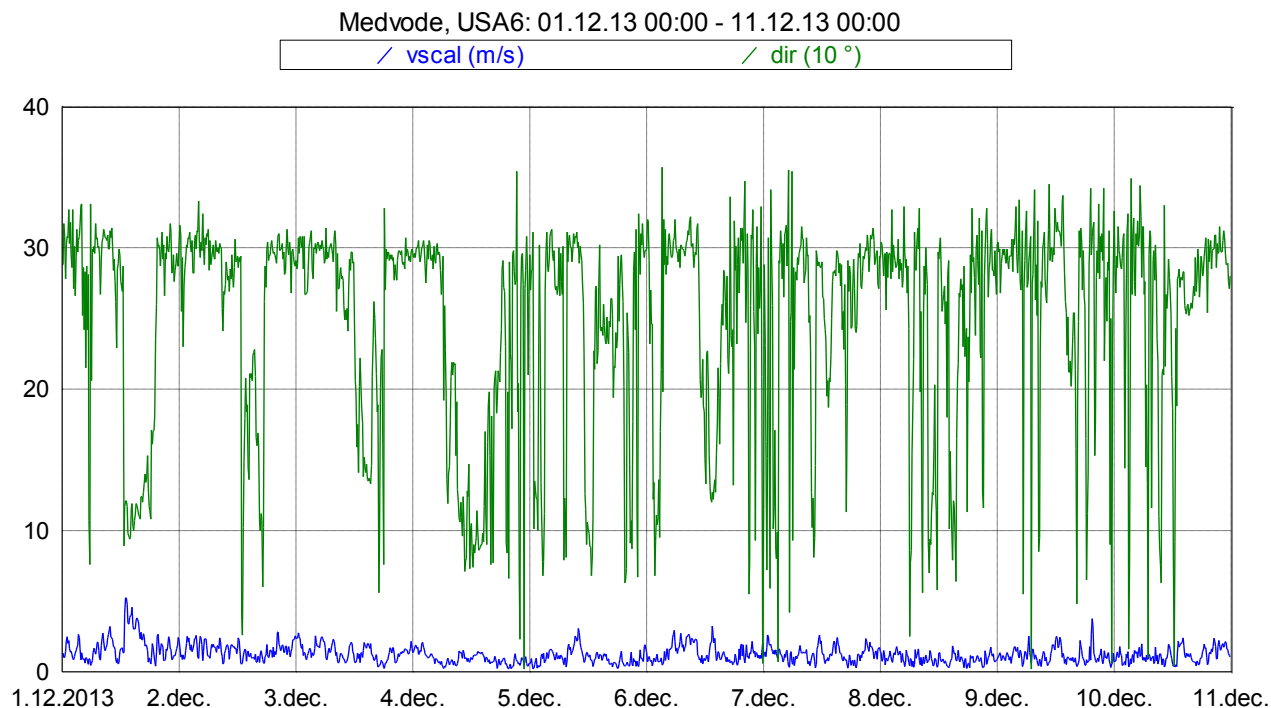
Slika 16: Smer in hitrost vetra med 1. 12. 2013 in 10. 12. 2013.
