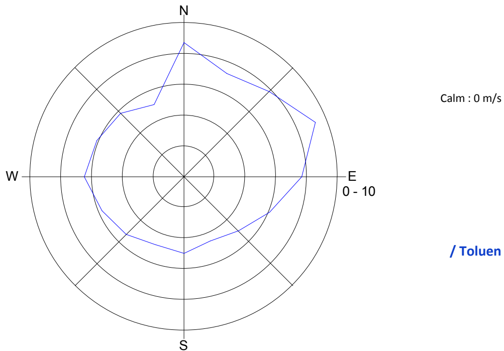
Slika 11: Roža onesnaženost - toluen, december 2013.
