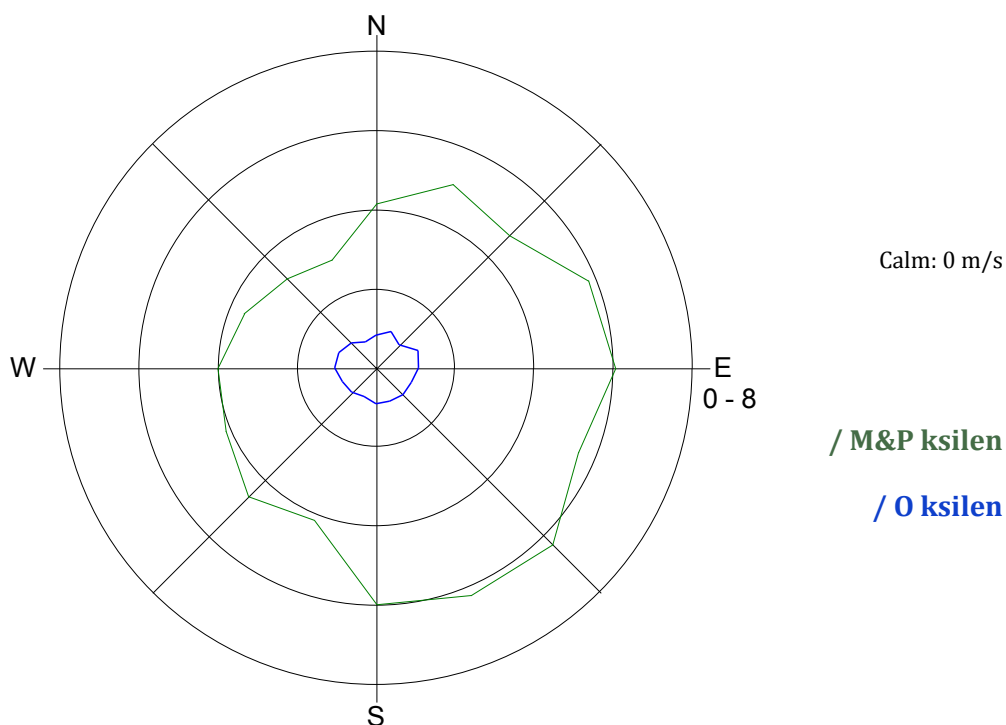
Slika 15: Roža onesnaženosti - M & P ksilen in O ksilen, december 2013.
