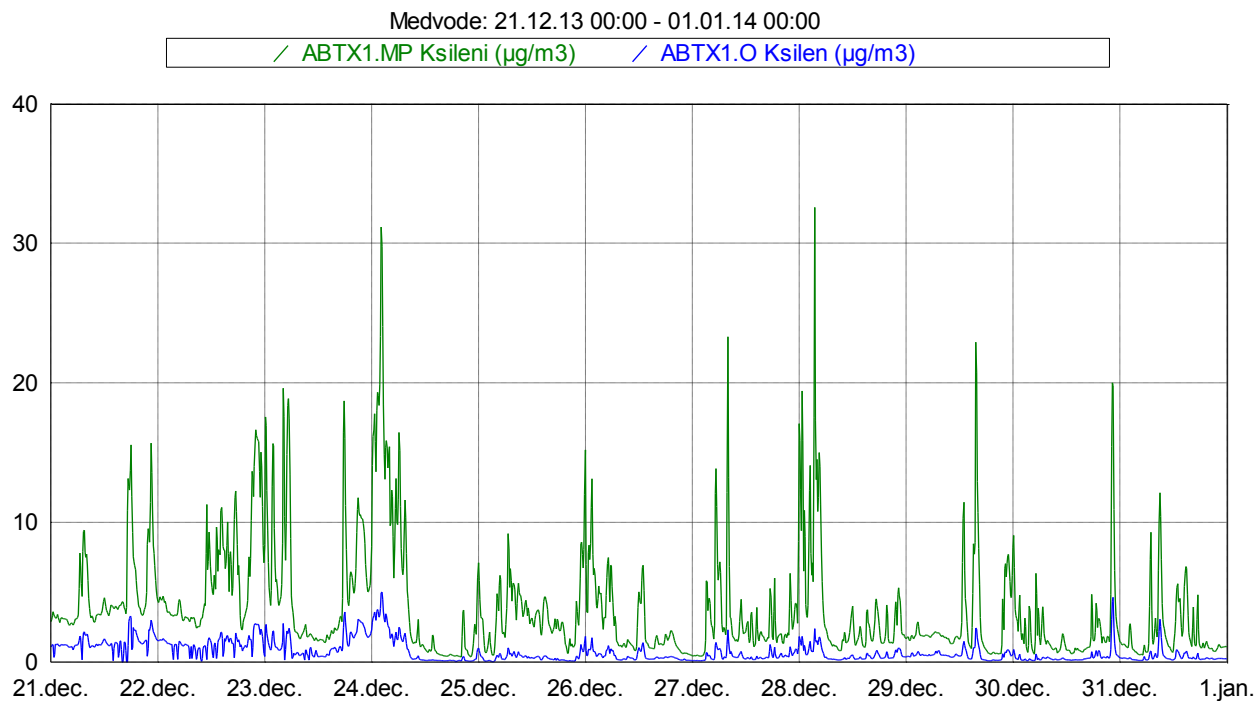
Slika 14: Imisijske koncentracije M&P in O ksilena med 21. 12. 2013 in 31. 12. 2013.
