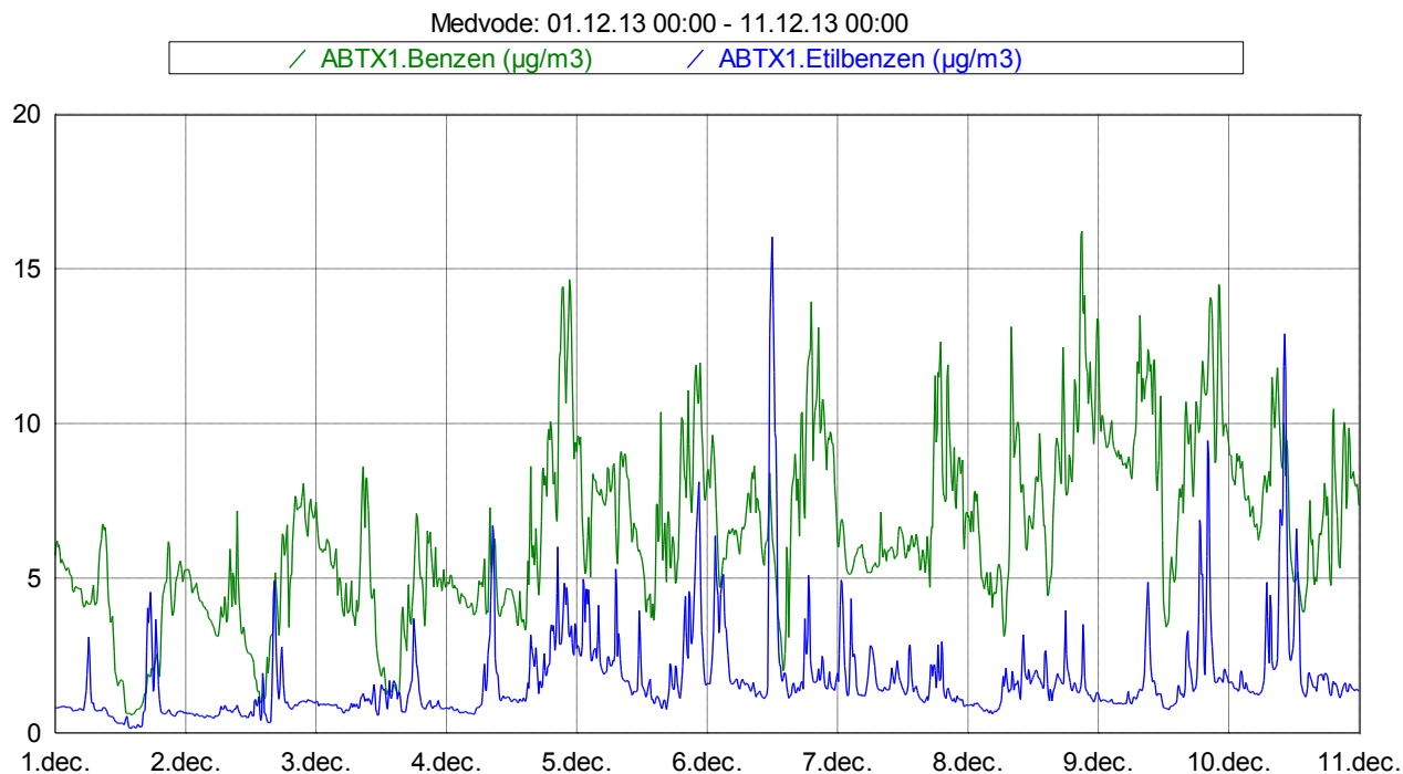
Slika 3: Imisijske koncentracije benzena in etilbenzena med vključno 1. 12. 2013 in 10. 12. 2013.
