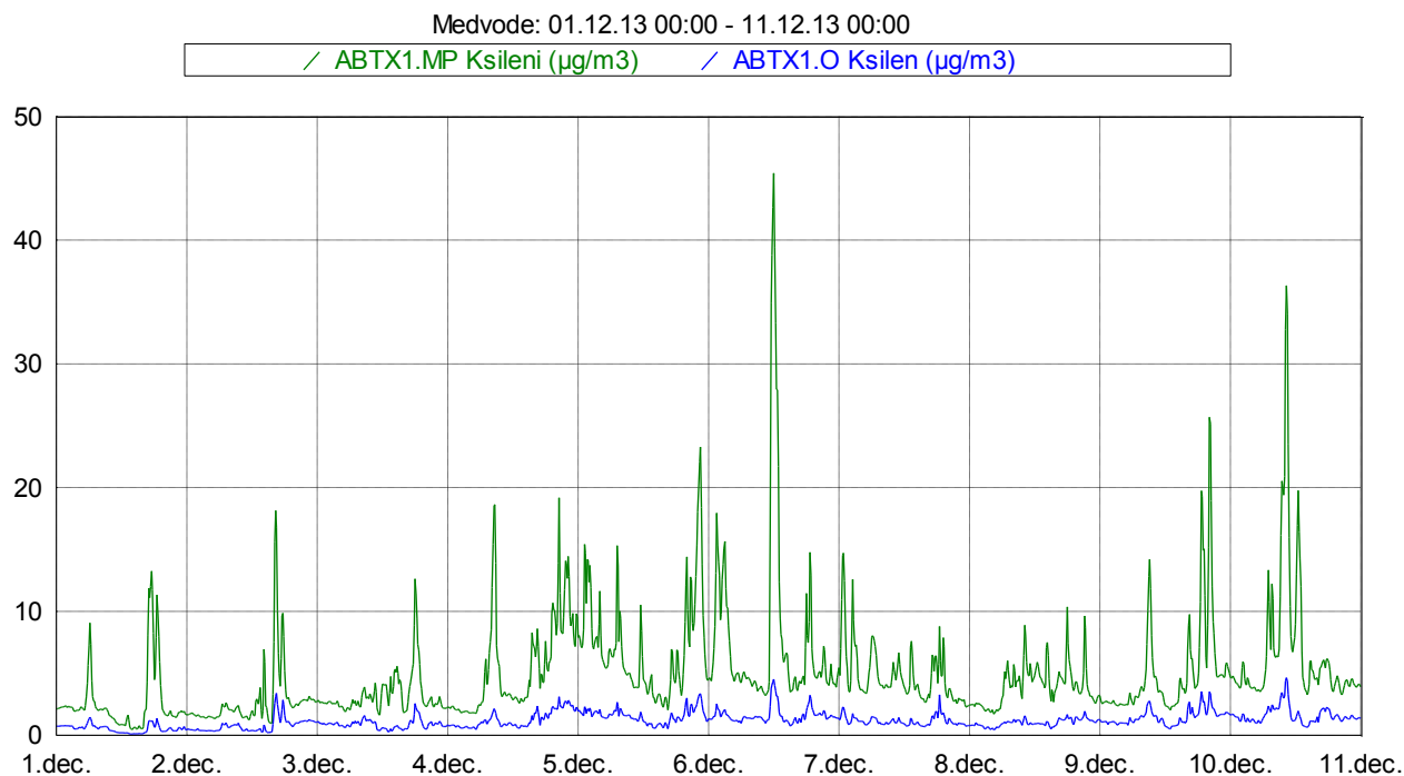
Slika 12: Imisijske koncentracije M&P in O ksilena med vključno 1. 12. 2013 in 10. 12. 2013.
