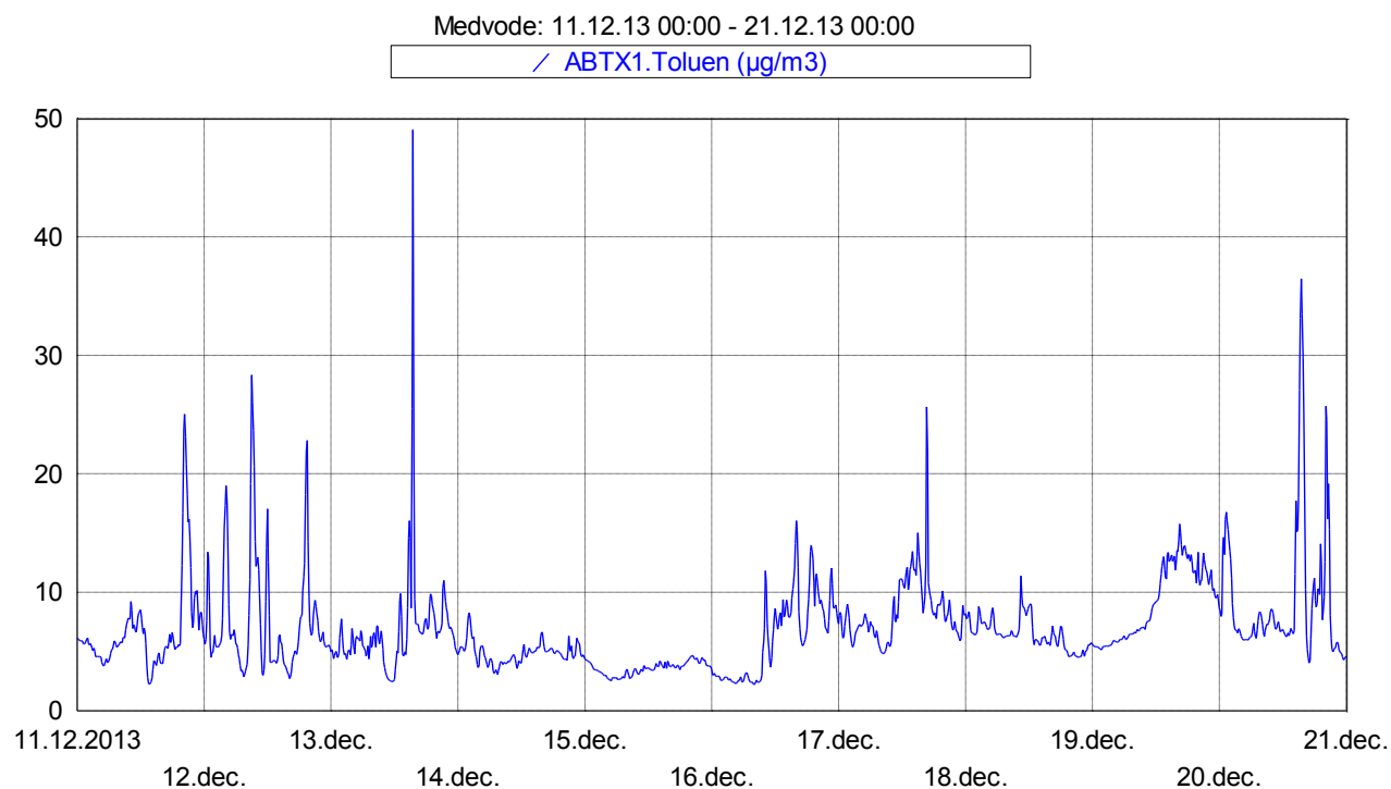
Slika 9: Imisijske koncentracije toluena med 11. 12. 2013 in 20. 12. 2013.
