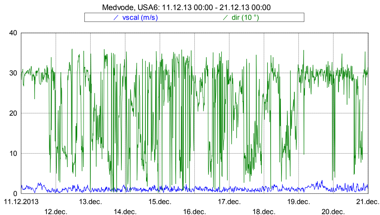
Slika 17: Smer in hitrost vetra med 11. 12. 2013 in 20. 12. 2013.
