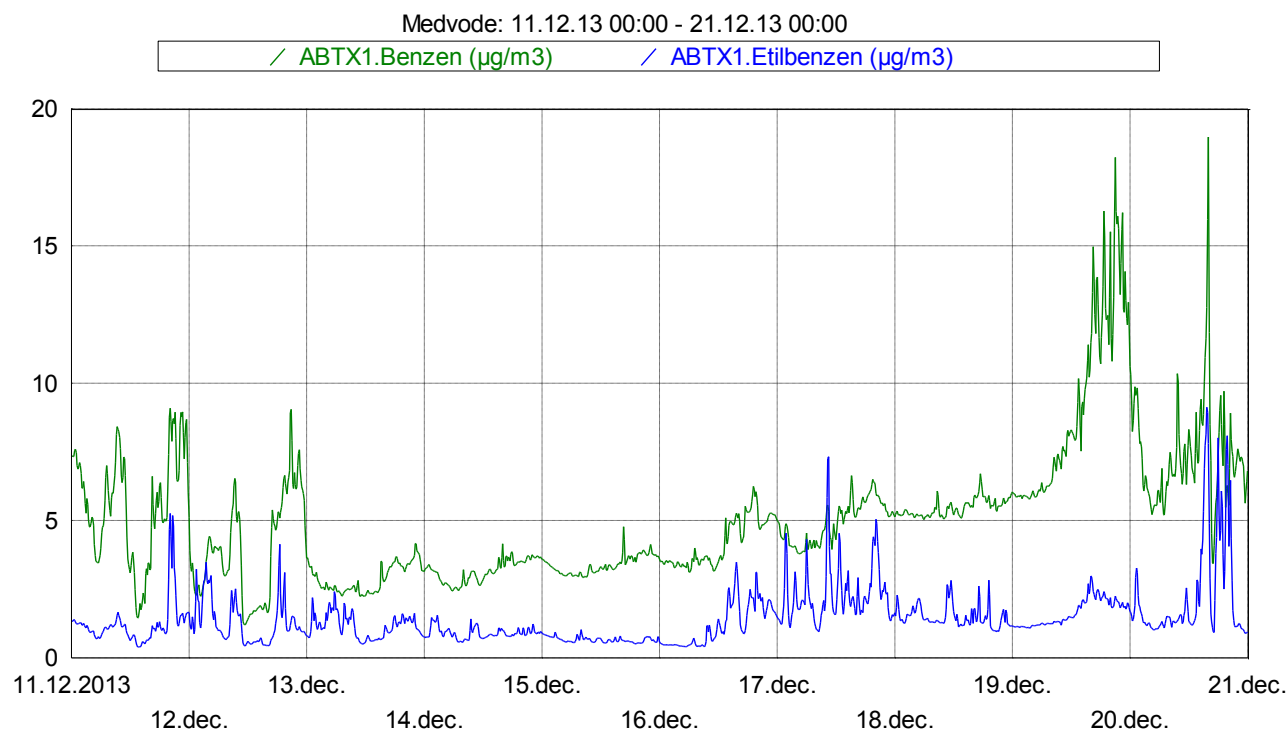
Slika 4: Imisijske koncentracije benzena in etilbenzena med 11. 12. 2013 in 20. 12. 2013.
