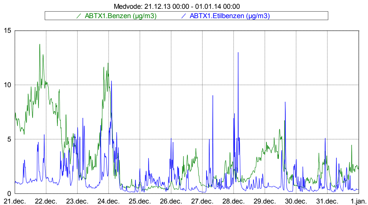
Slika 5: Imisijske koncentracije benzena in etilbenzena med 21. 12. 2013 in 31. 12. 2013.
