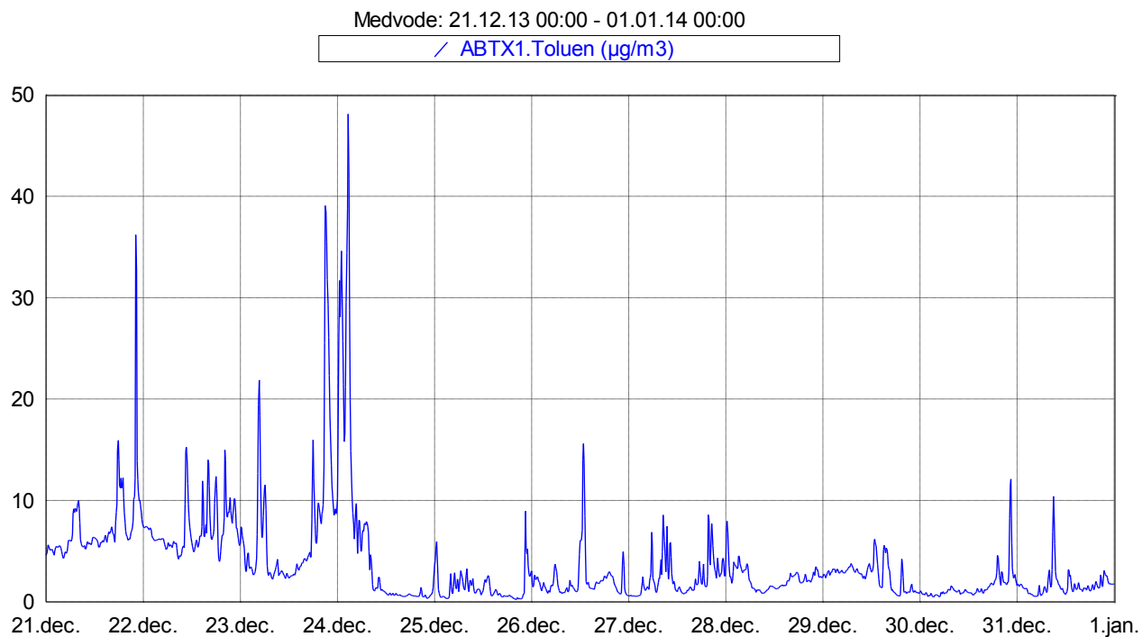
Slika 10: Imisijske koncentracije toluea med 21. 12. 2013 in 31. 12. 2013.
