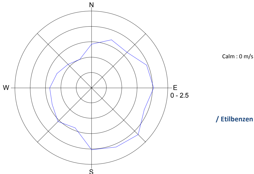
Slika 7: Roža onesnaženosti - etilbenzen december 2013.
