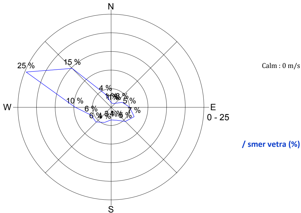
Slika 18: Smer in hitrost vetra med 21. 12. 2013 in 31. 12. 2013.
