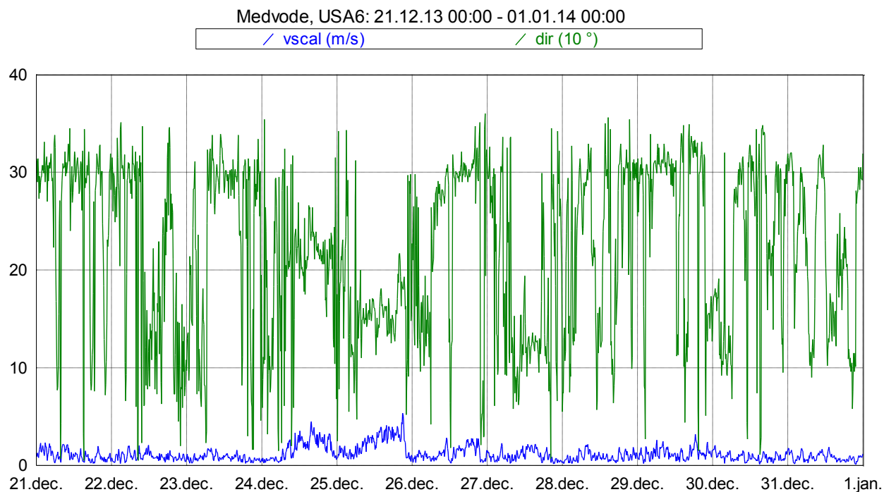
Slika 18: Smer in hitrost vetra med 21. 12. 2013 in 31. 12. 2013.
