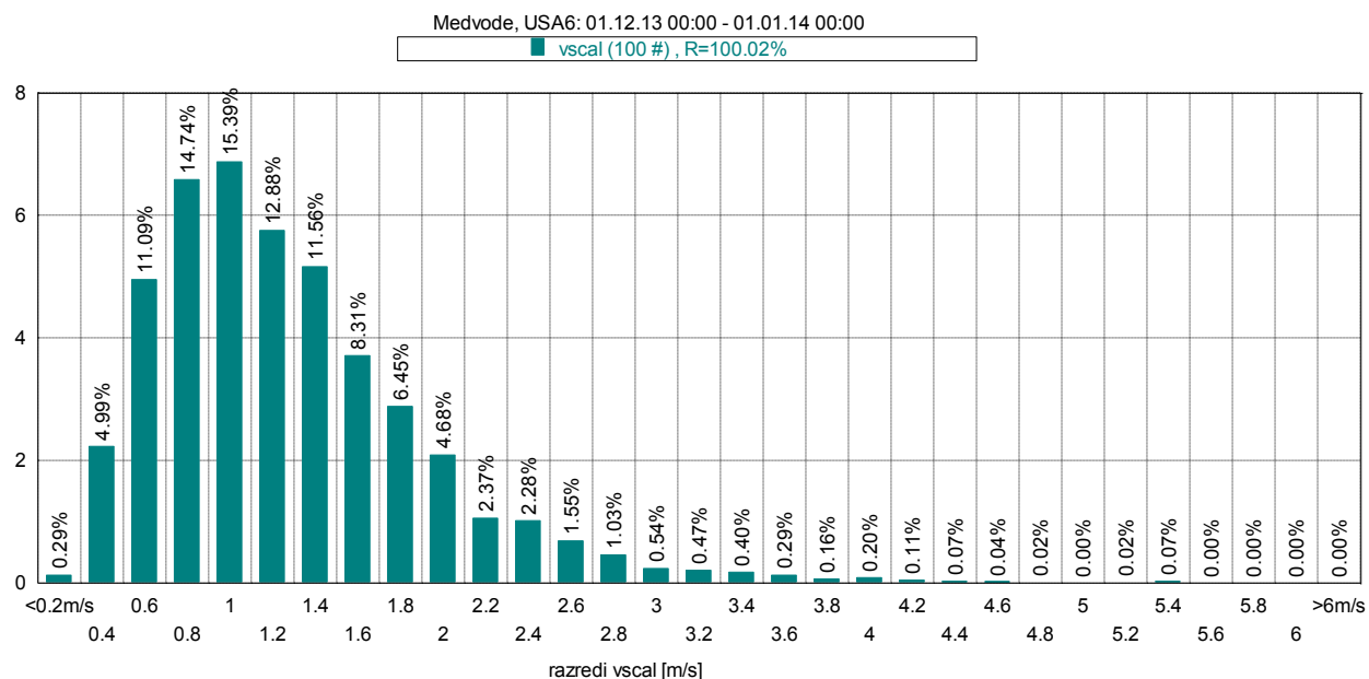
Slika 20: Frekvenčna porazdelitev po hitrosti vetra, december 2013.
