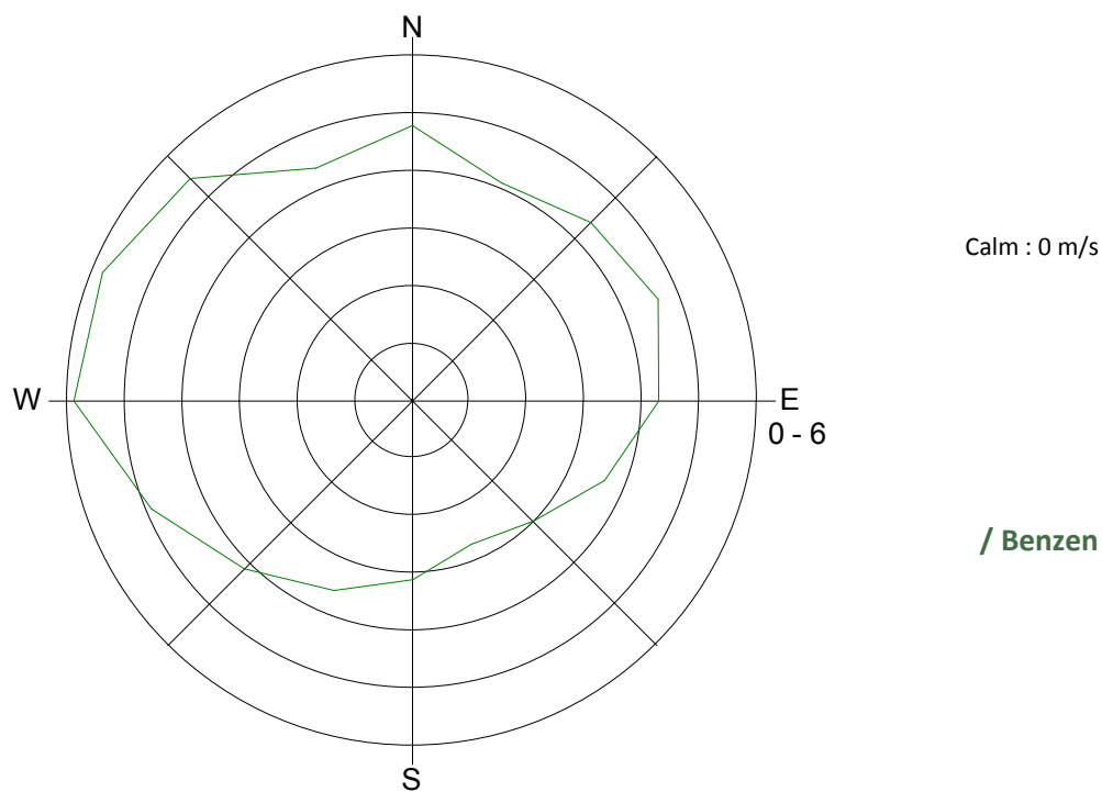
Slika 6: Roža onesnaženosti – benzen, december 2013.
