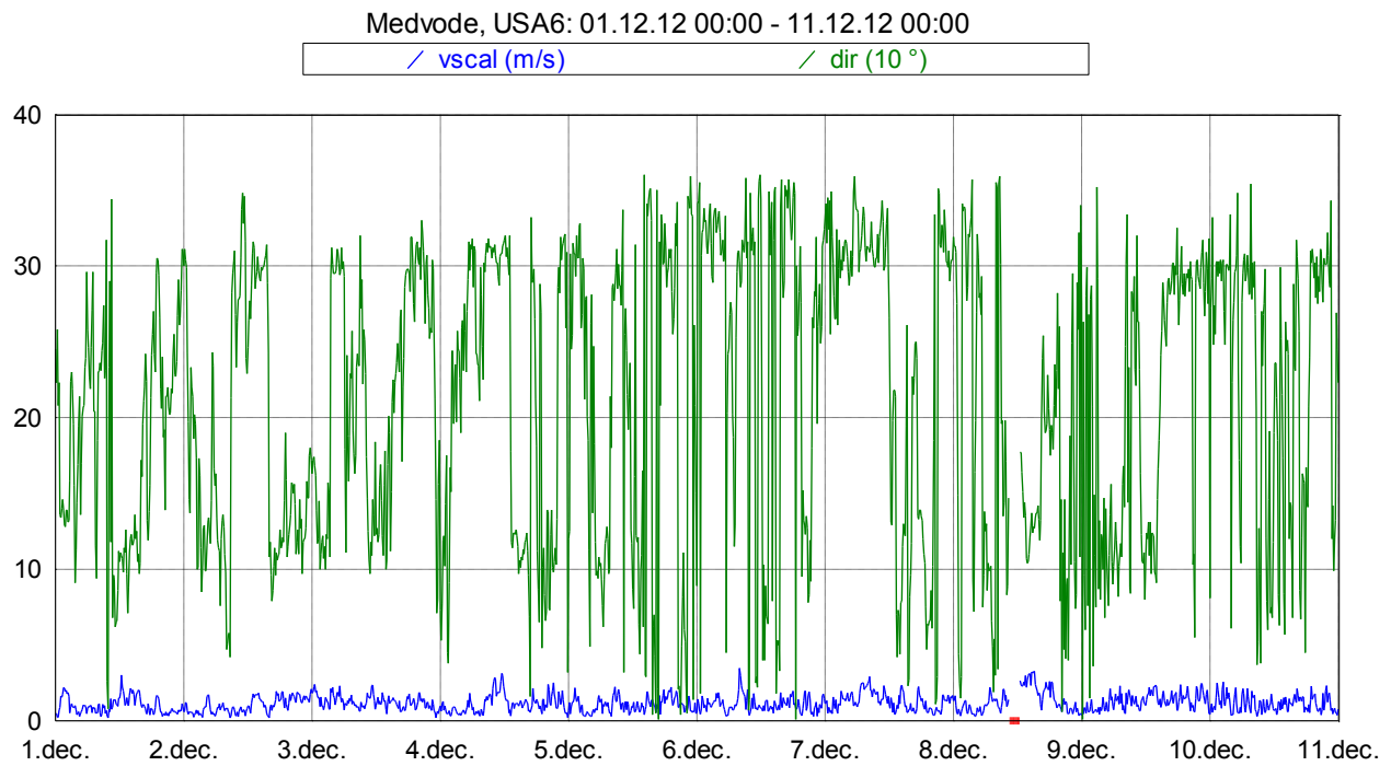
Slika 15: Smer in hitrost vetra med 1. 12. 2012 in 11. 12. 2012.
