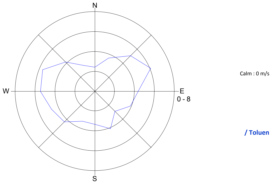
Slika 10: Roža onesnaženost - toluen, december 2012.
