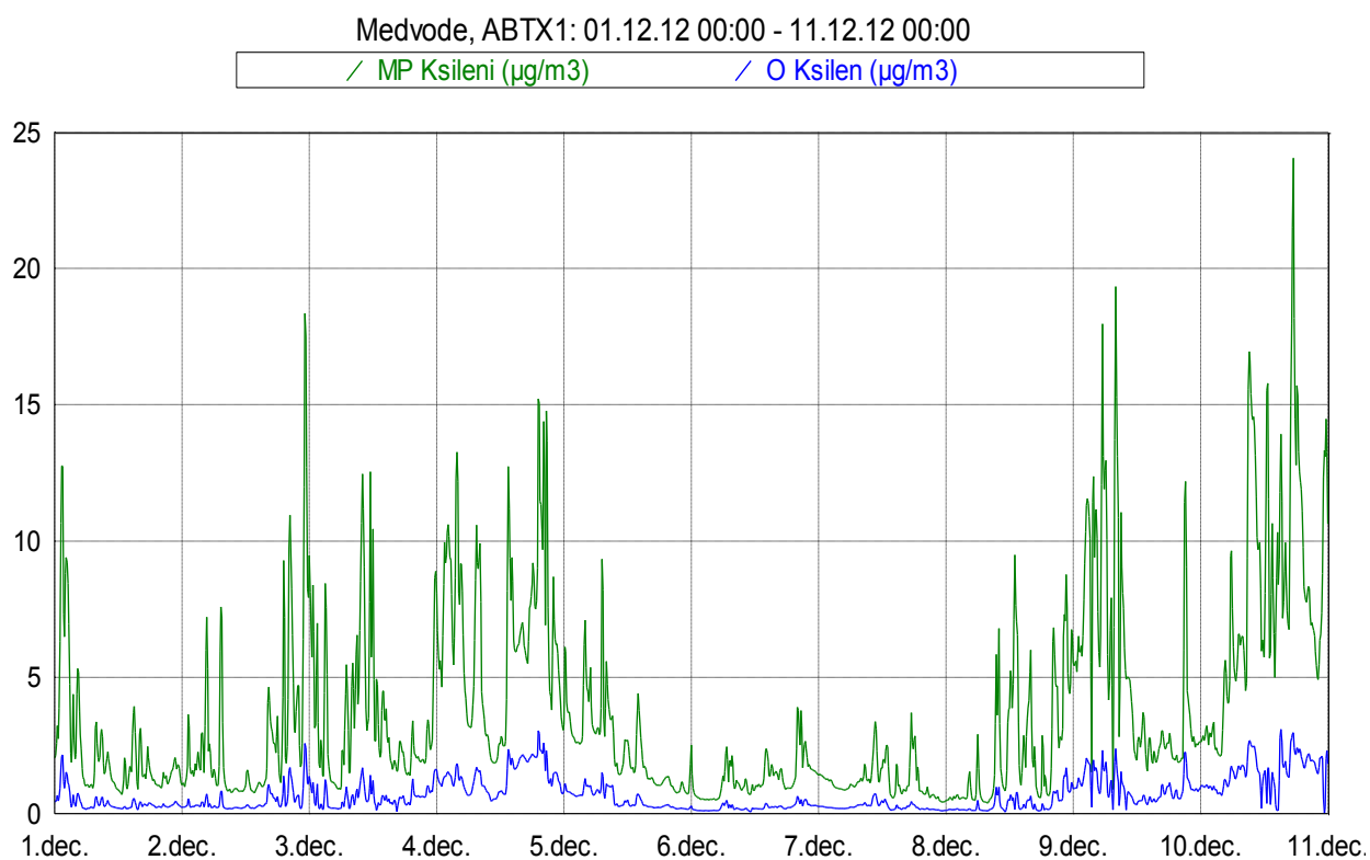
Slika 11: Imisijske koncentracije M&P in O ksilena med vključno 1. 12. 2012 in 11. 12. 2012.
