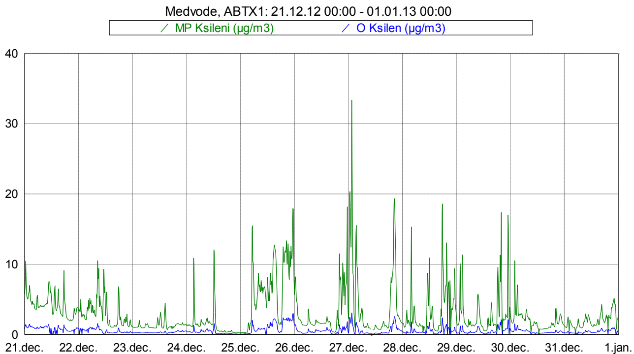
Slika 13: Imisijske koncentracije M&P in O ksilena med 21. 12. 2012 in 31. 12. 2012.
