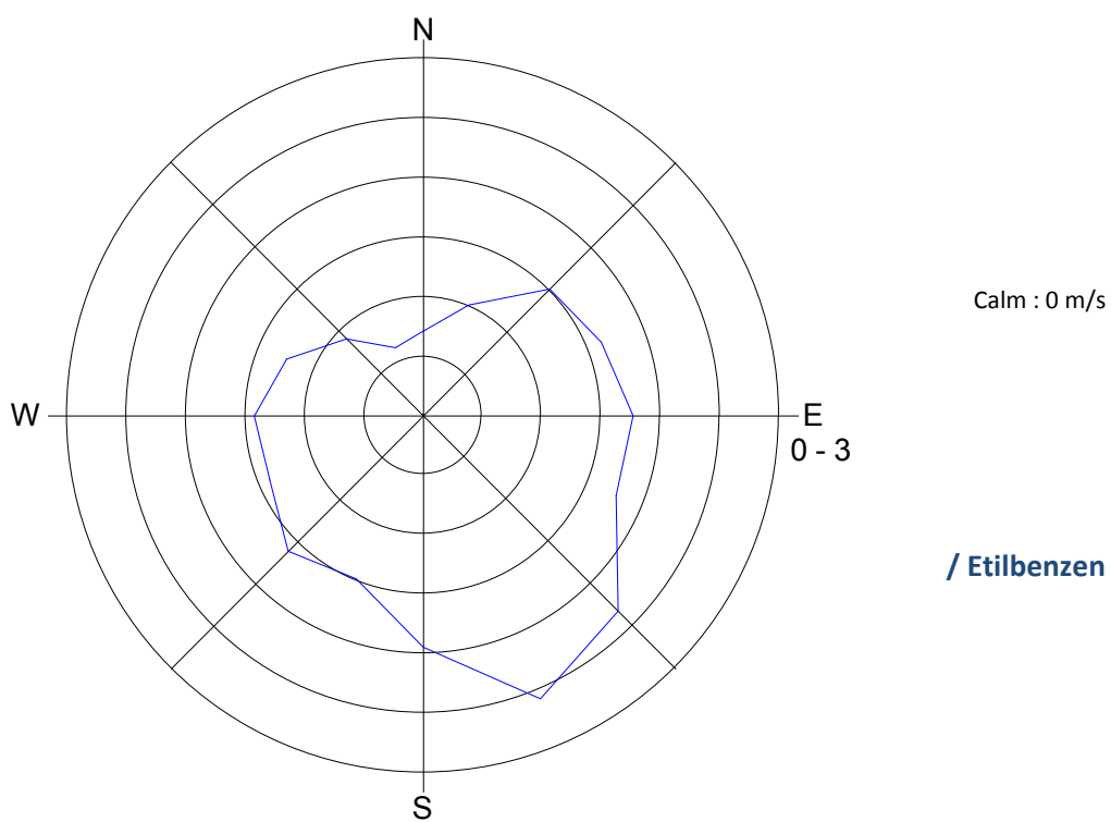
Slika 6: Roža onesnaženosti – benzen (zgoraj) in etilbenzen (spodaj), december 2012.
