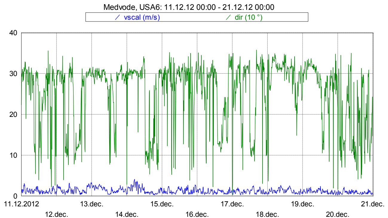
Slika 16: Smer in hitrost vetra med 11. 12. 2012 in 21. 12. 2012.
