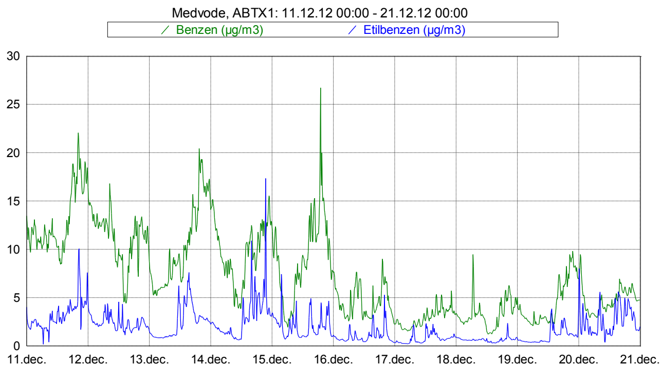
Slika 4: Imisijske koncentracije benzena in etilbenzena med 11. 12. 2012 in 21. 12. 2012.
