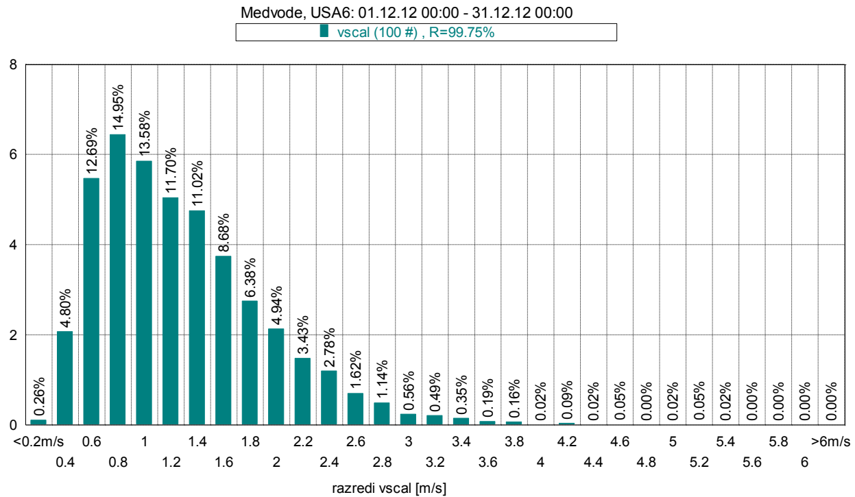
Slika 19: Frekvenčna porazdelitev po hitrosti vetra, december 2012.
