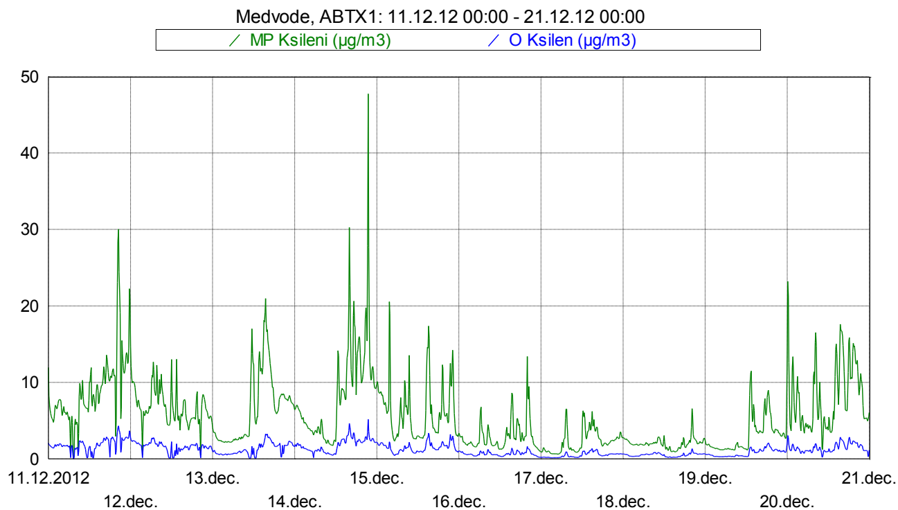
Slika 12: Imisijske koncentracije M&P in O ksilena med 11. 12. 2012 in 21. 12. 2012.
