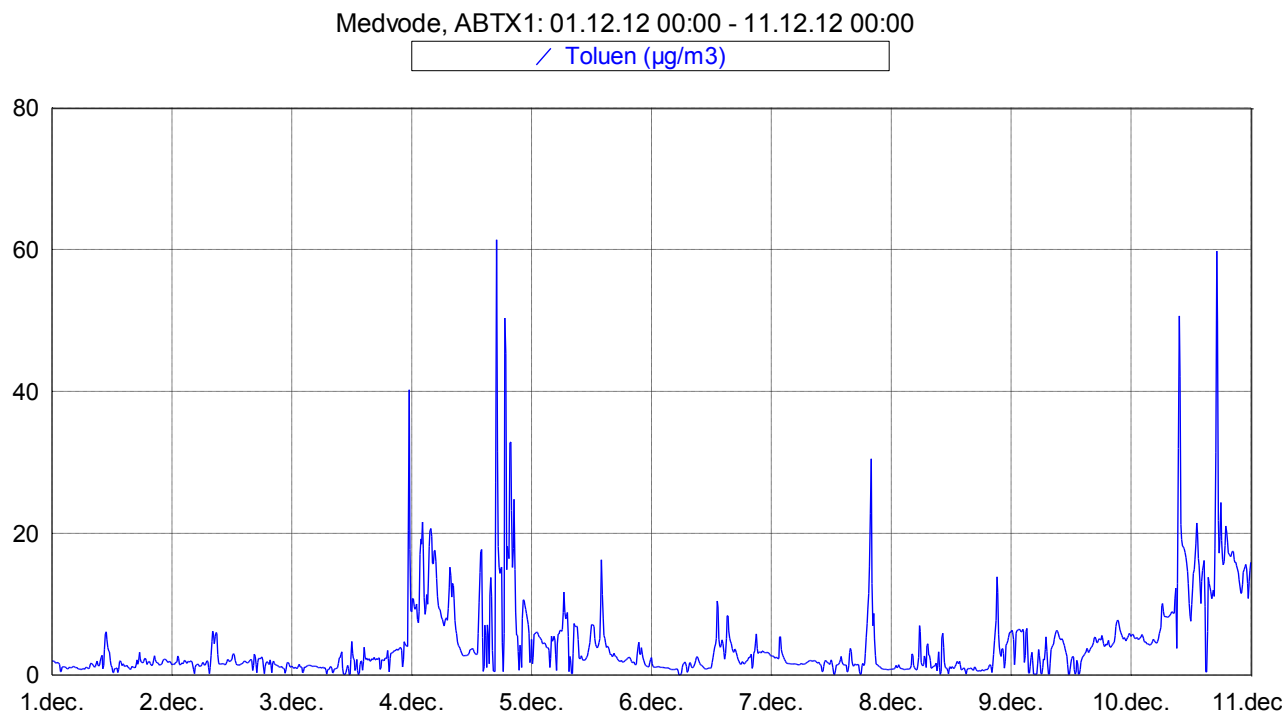
Slika 7: Imisijske koncentracije toluena med vključno 1. 12. 2012 in 11. 12. 2012.
