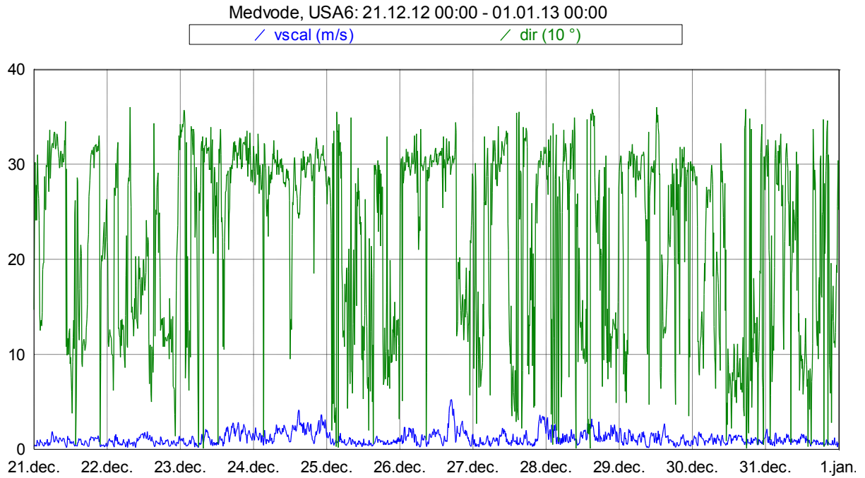
Slika 17: Smer in hitrost vetra med 21. 12. 2012 in 31. 12. 2012.
