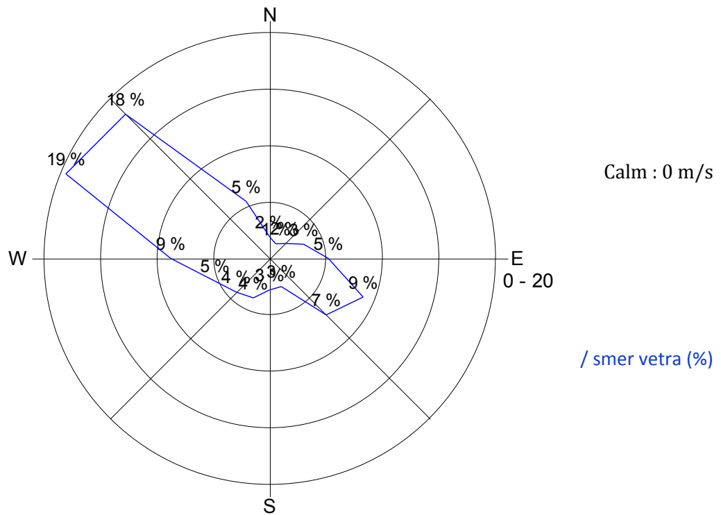
Slika 18: Roža vetrov, december 2012.
