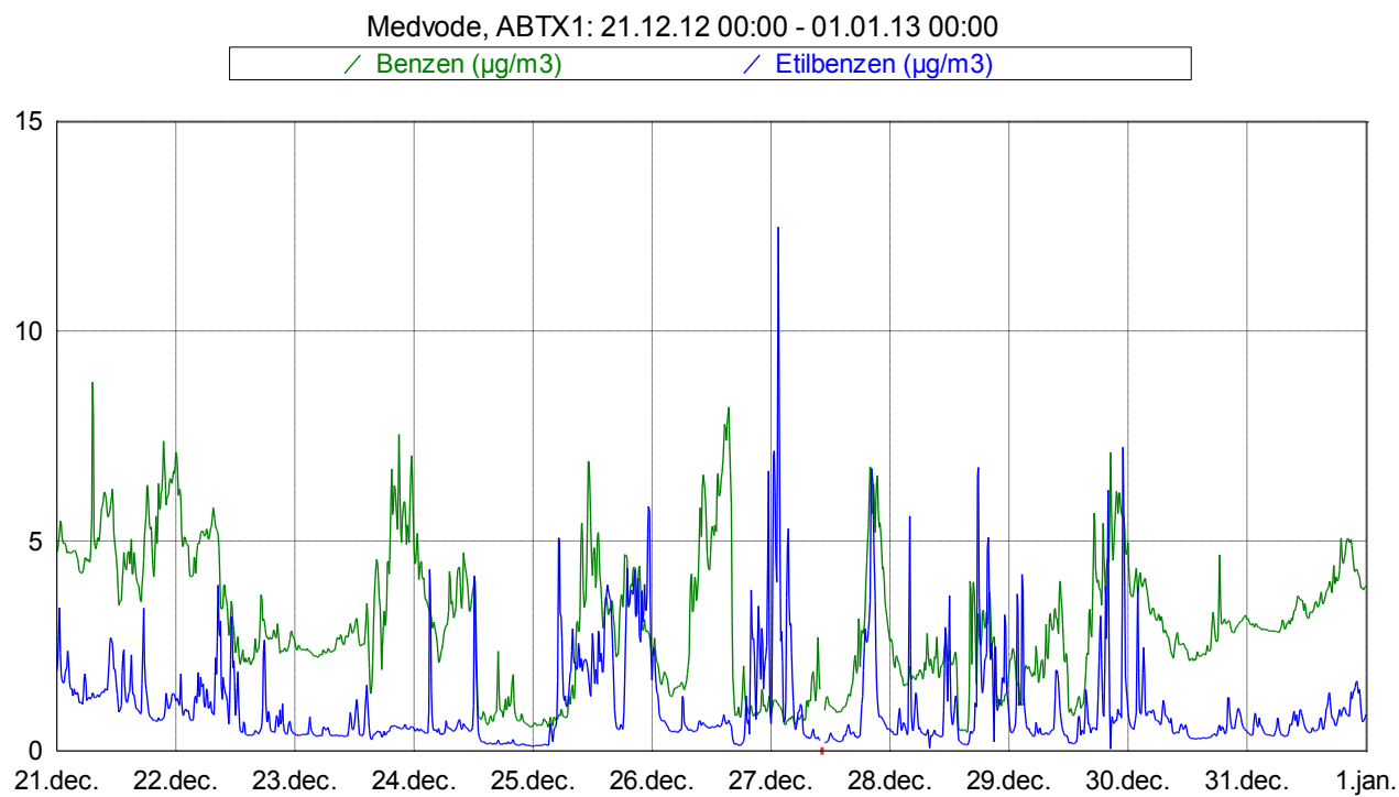
Slika 5: Imisijske koncentracije benzena in etilbenzena med 21. 12. 2012 in 31. 12. 2012.
