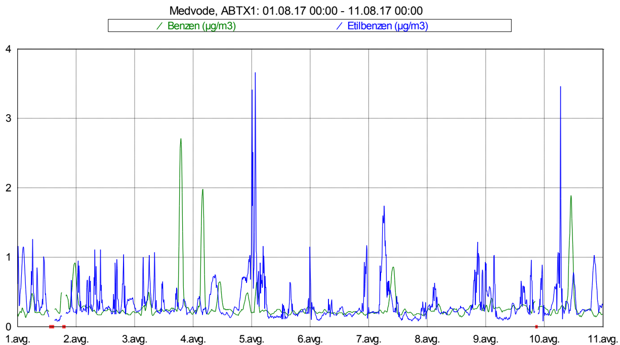
Slika 3: Imisijske koncentracije benzena in etilbenzena med vključno 1. 8. in 10. 8. 2017.
