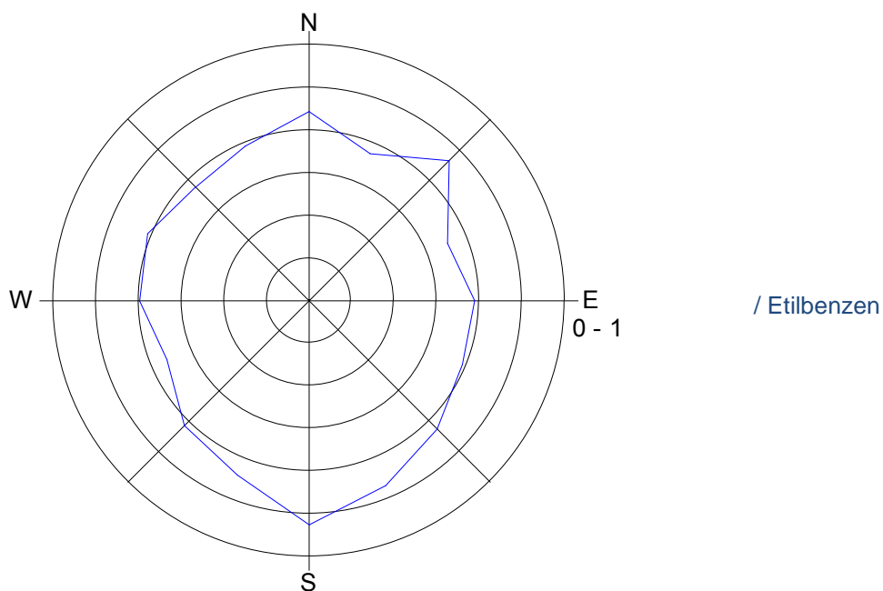
Slika 7: Roža onesnaženosti – etilbenzen, avgust 2017.
