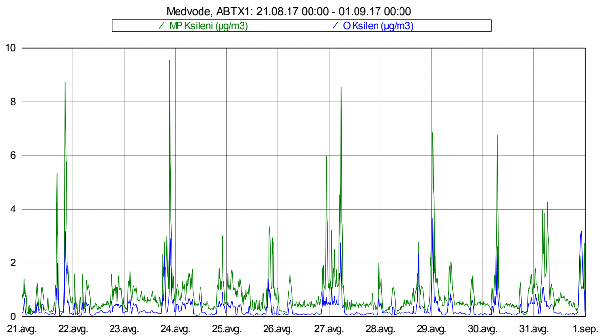
Slika 14: Imisijske koncentracije ksilenov med vključno 21. 8. in 31. 8. 2017.
