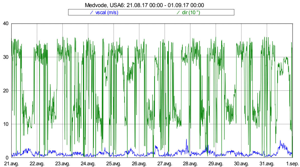
Slika 18: Smer in hitrost vetra med 21. 8. in 31. 8. 2017.
