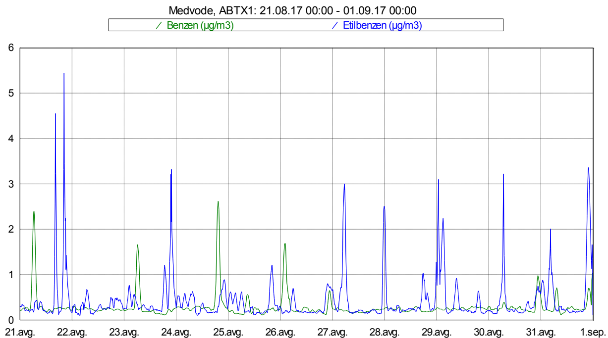
Slika 5: Imisijske koncentracije benzena in etilbenzena med vključno 21. 8. in 31. 8. 2017.
