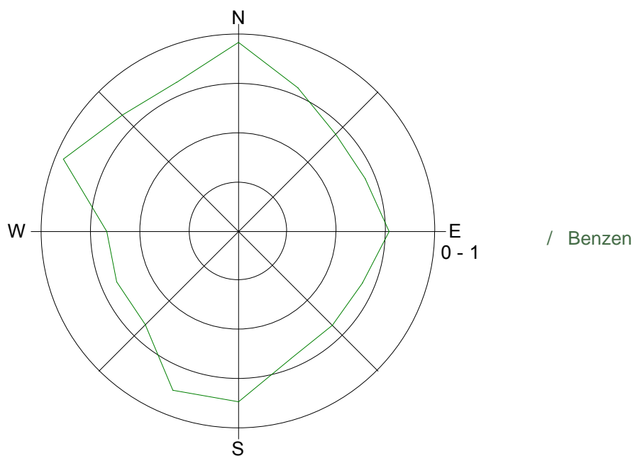
Slika 6: Roža onesnaženosti – benzen, avgust 2017.
