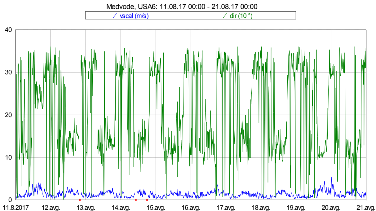
Slika 17: Smer in hitrost vetra med 11. 8. in 20. 8. 2017.
