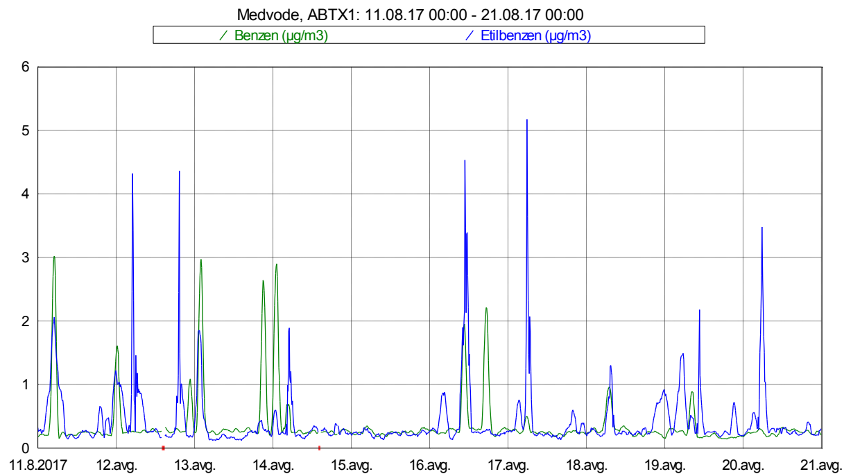
Slika 4: Imisijske koncentracije benzena in etilbenzena med vključno 11. 8. in 20. 8. 2017.
