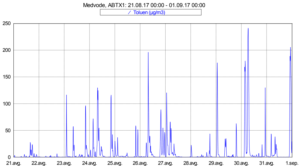
Slika 10: Imisijske koncentracije toluena med vključno 21. 8. in 31. 8. 2017.
