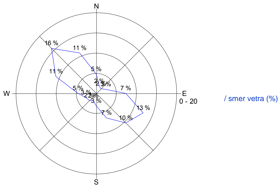
Slika 19: Roža vetrov, avgust 2017.
