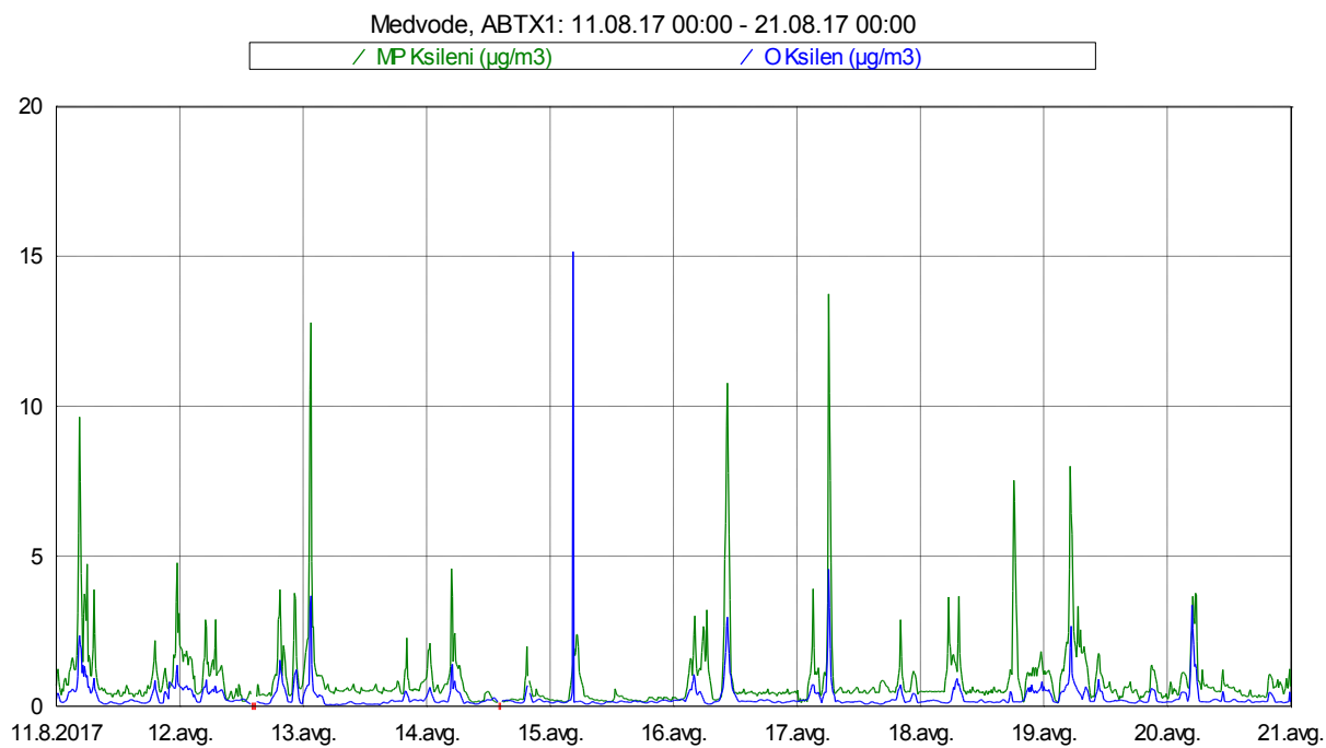
Slika 13: Imisijske koncentracije ksilenov med vključno 11. 8. in 20. 8. 2017.
