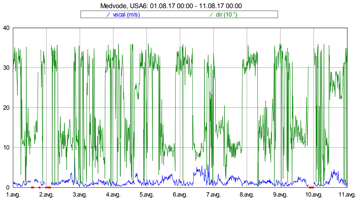
Slika 16: Smer in hitrost vetra med 1. 8. in 10. 8. 2017.
