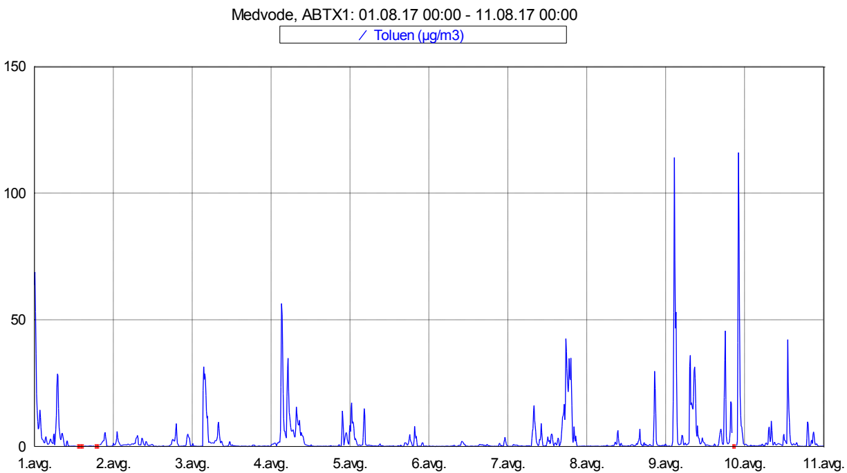
Slika 8: Imisijske koncentracije toluena med vključno 1. 8. in 10. 8. 2017.
