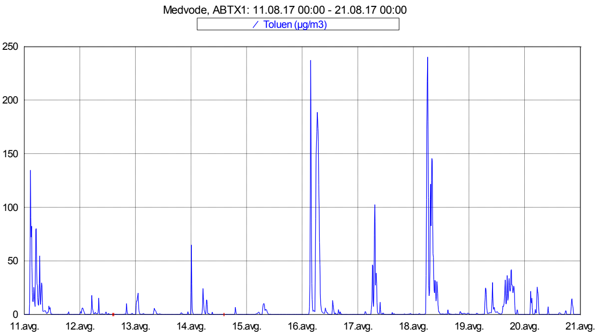
Slika 9: Imisijske koncentracije toluena med vključno 11. 8. in 20. 8. 2017.
