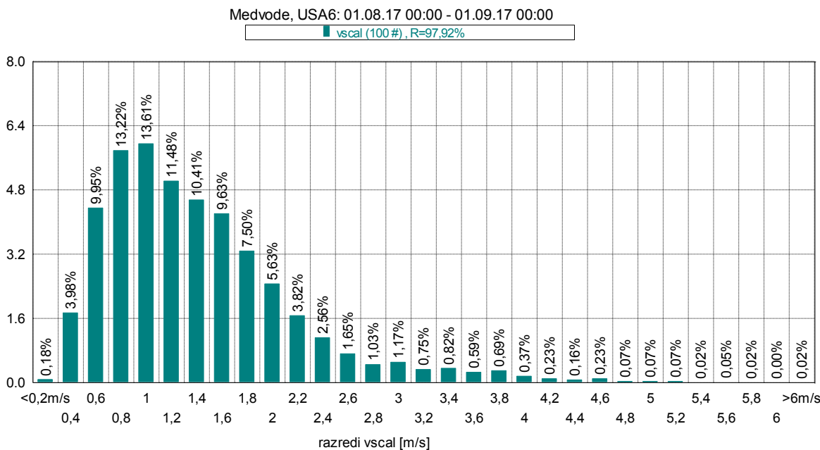
Slika 20: Frekvenčna porazdelitev po hitrosti vetra, avgust 2017.
