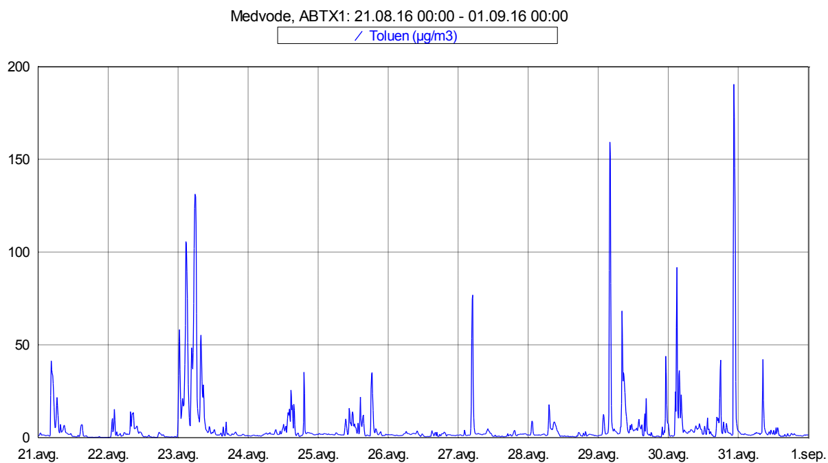
Slika 10: Imisijske koncentracije toluea med 21. 8. 2016 in 31. 8. 2016.
