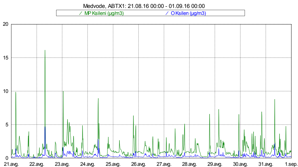
Slika 14: Imisijske koncentracije M&P in O ksilena med 21. 8. 2016 in 31. 8. 2016.
