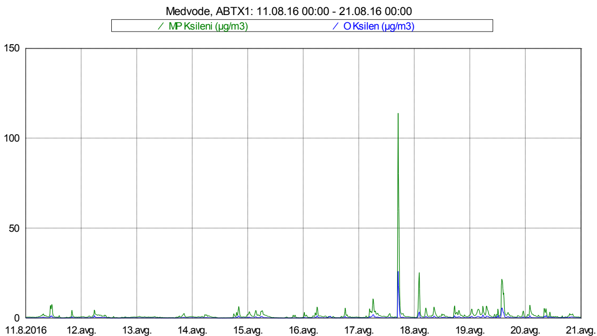
Slika 13: Imisijske koncentracije M&P in O ksilena med 11. 8. 2016 in 20. 8. 2016.
