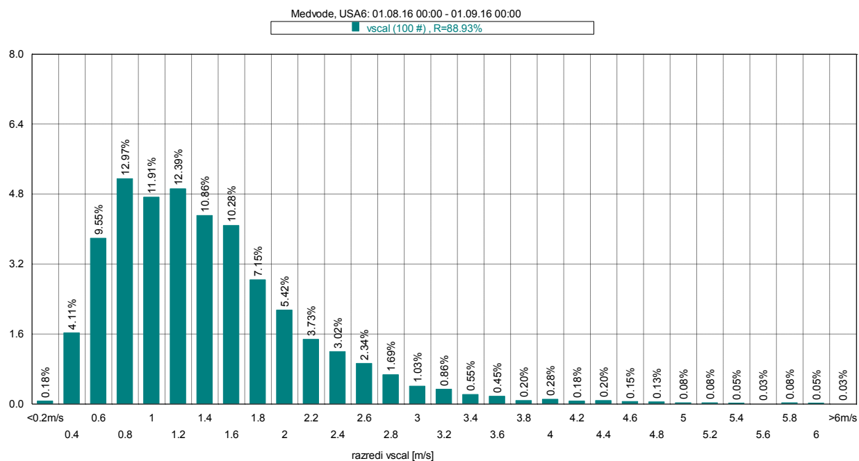
Slika 20: Frekvenčna porazdelitev po hitrosti vetra, avgust 2016.
