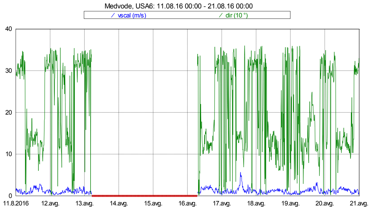
Slika 17: Smer in hitrost vetra med 11. 8. 2016 in 20. 8. 2016.
