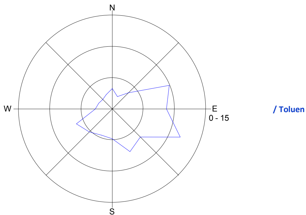
Slika 11: Roža onesnaženost - toluen, avgust 2016.
