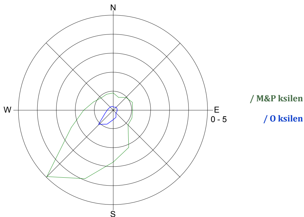
Slika 15: Roža onesnaženosti - M & P ksilen in O ksilen, avgust 2016.
