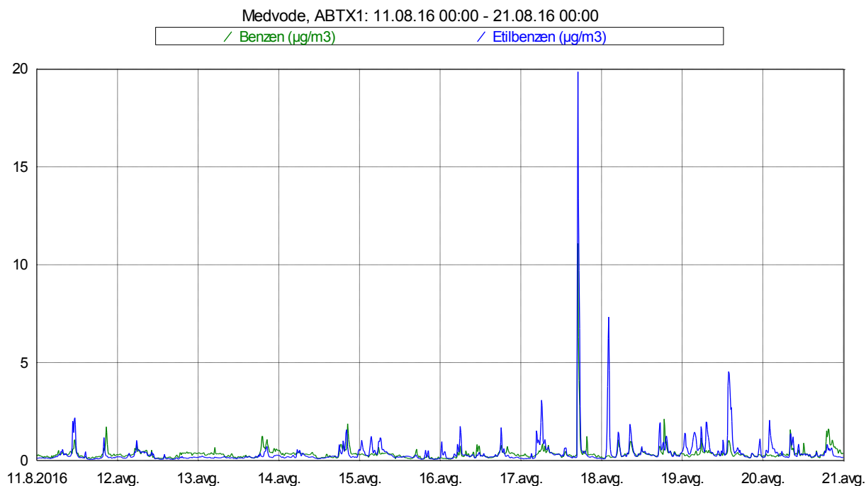
Slika 4: Imisijske koncentracije benzena in etilbenzena med 11. 8. 2016 in 20. 8. 2016.
