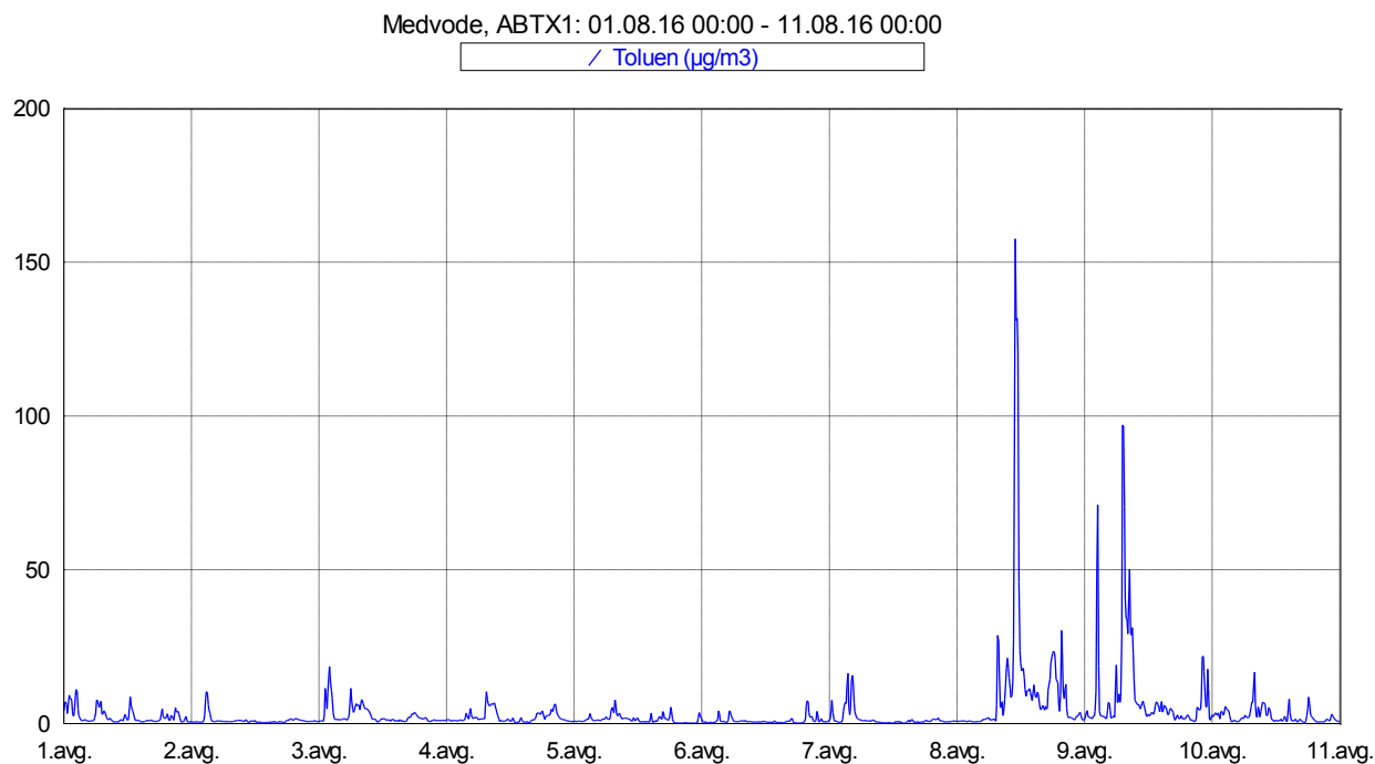
Slika 8: Imisijske koncentracije toluena med vključno 1. 8. 2016 in 10. 8. 2016.
