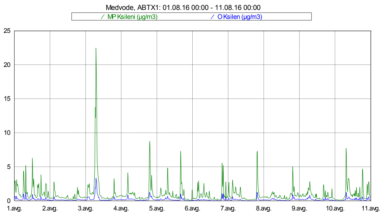
Slika 12: Imisijske koncentracije M&P in O ksilena med vključno 1. 8. 2016 in 10. 8. 2016.
