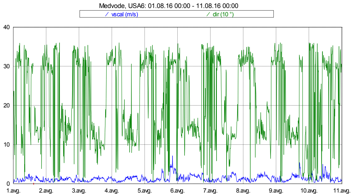
Slika 16: Smer in hitrost vetra med 1. 8. 2016 in 10. 8. 2016.
