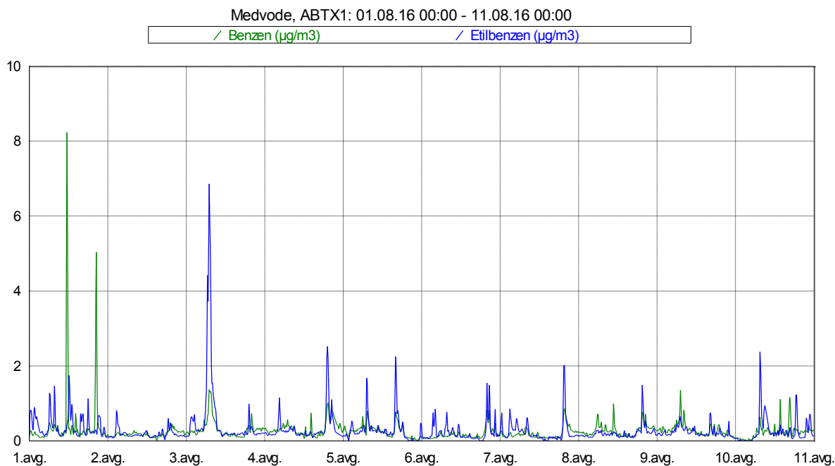
Slika 3: Imisijske koncentracije benzena in etilbenzena med vključno 1. 8. 2016 in 10. 8. 2016.
