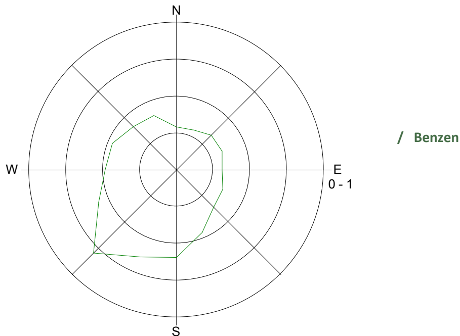
Slika 6: Roža onesnaženosti – benzen, avgust 2016.
