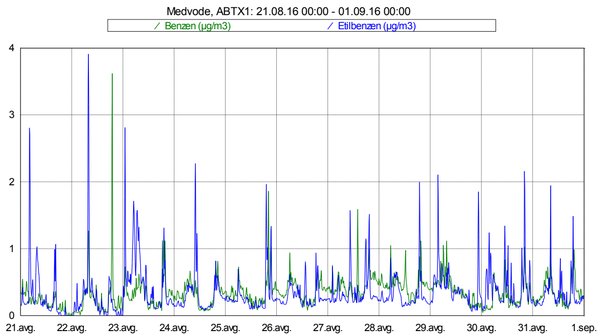
Slika 5: Imisijske koncentracije benzena in etilbenzena med 21. 8. 2016 in 31. 8. 2016.
