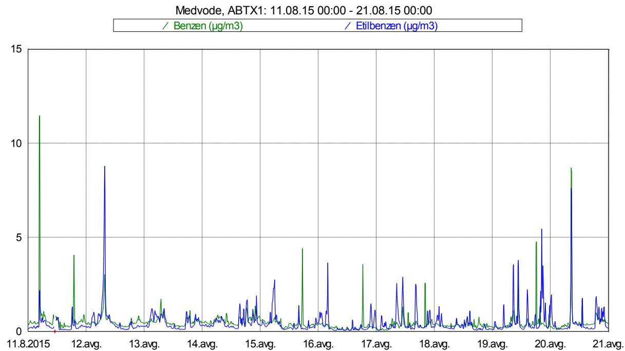
Slika 4: Imisijske koncentracije benzena in etilbenzena med 11. 8. 2015 in 20. 8. 2015.
