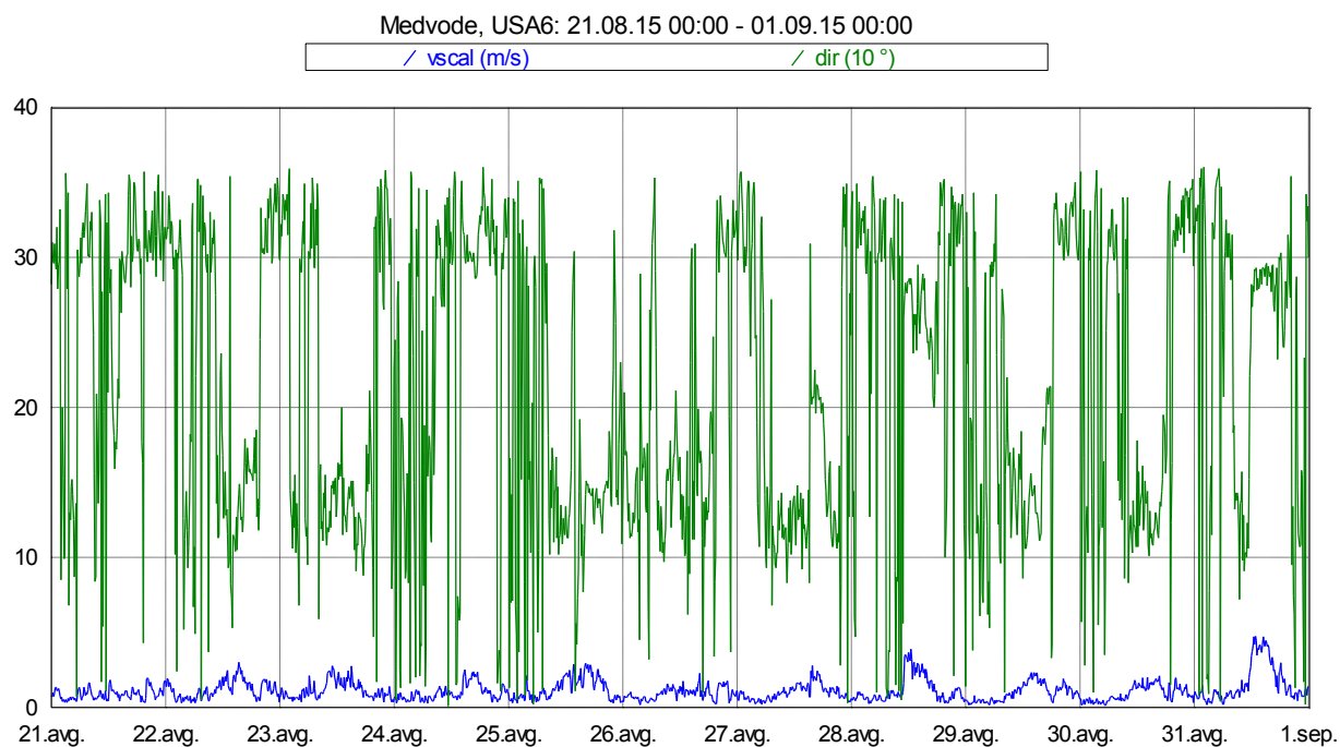
Slika 18: Smer in hitrost vetra med 21. 8. 2015 in 31. 8. 2015.
