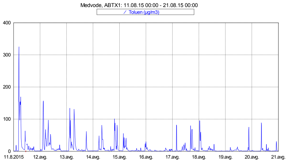
Slika 9: Imisijske koncentracije toluena med 11. 8. 2015 in 20. 8. 2015.
