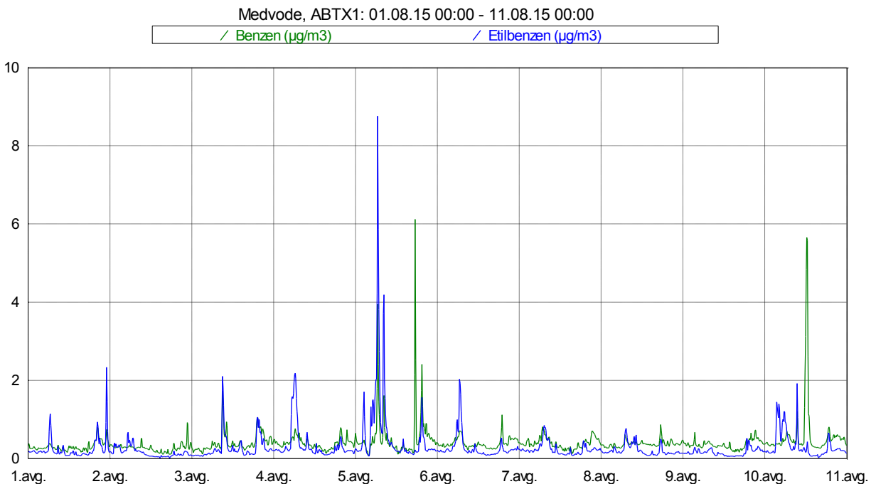
Slika 3: Imisijske koncentracije benzena in etilbenzena med vključno 1. 8. 2015 in 10. 8. 2015.
