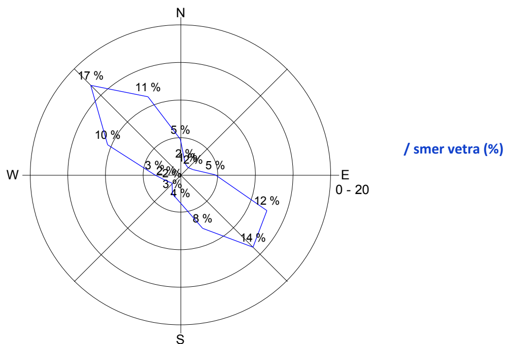
Slika 19: Roža vetrov, avgust 2015.
