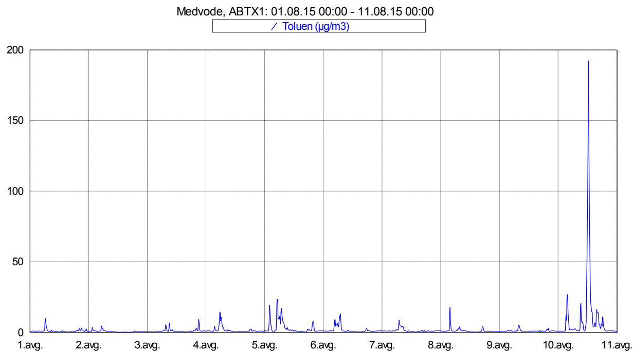
Slika 8: Imisijske koncentracije toluena med vključno 1. 8. 2015 in 10. 8. 2015.
