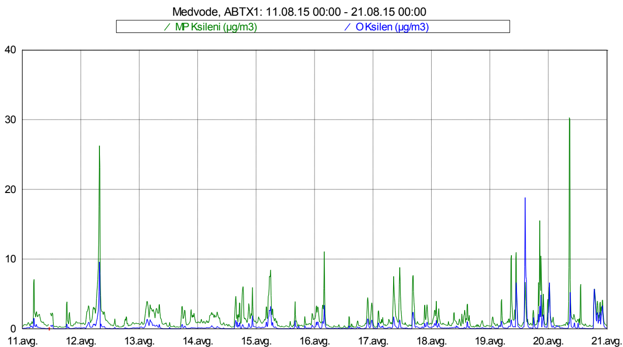
Slika 13: Imisijske koncentracije M&P in O ksilena med 11. 8. 2015 in 20. 8. 2015.
