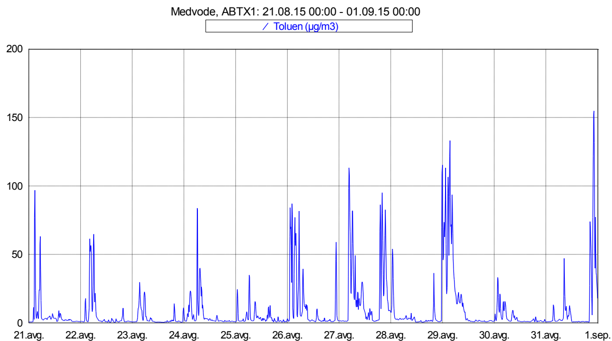
Slika 10: Imisijske koncentracije toluena med 21. 8. 2015 in 31. 8. 2015.
