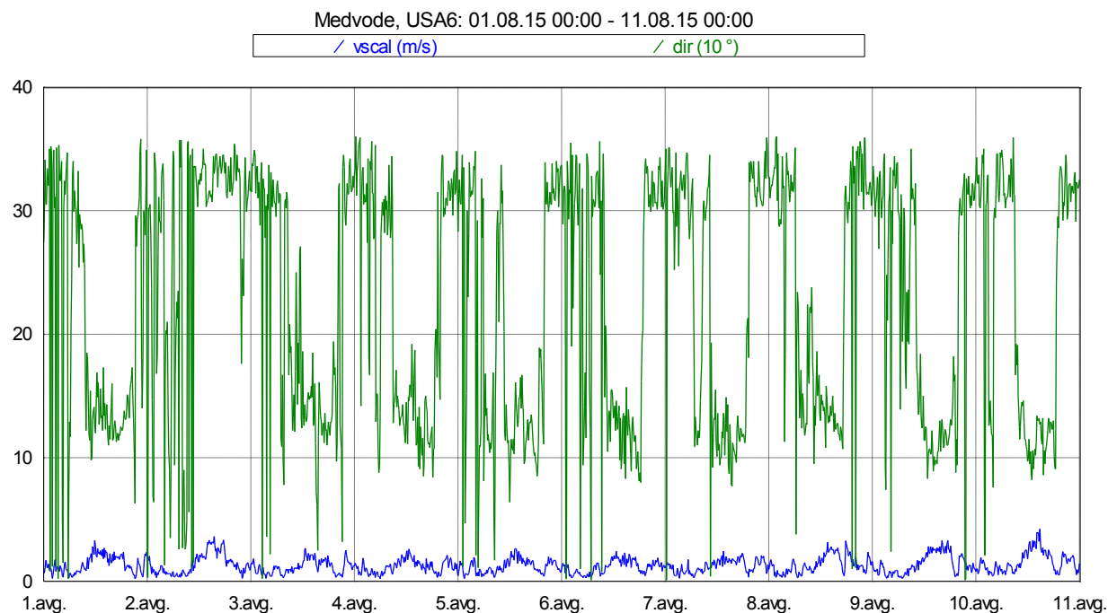
Slika 16: Smer in hitrost vetra med 1. 8. 2015 in 10. 8. 2015.
