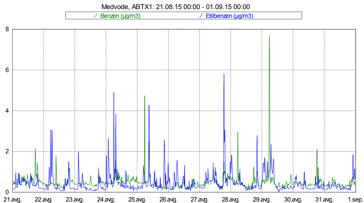
Slika 5: Imisijske koncentracije benzena in etilbenzena med 21. 8. 2015 in 31. 8. 2015.
