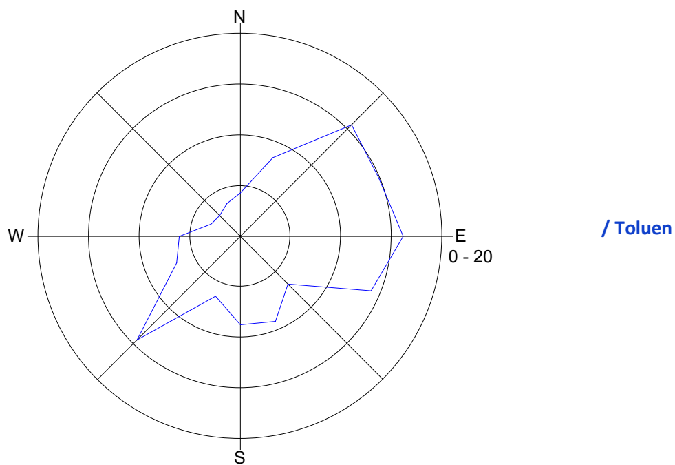
Slika 11: Roža onesnaženost - toluen, avgust 2015.
