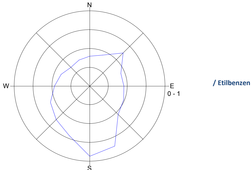
Slika 7: Roža onesnaženosti – etilbenzen, avgust 2015.
