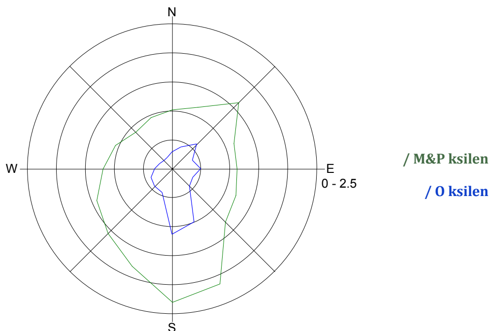
Slika 15: Roža onesnaženosti - M & P ksilen in O ksilen, avgust 2015.
