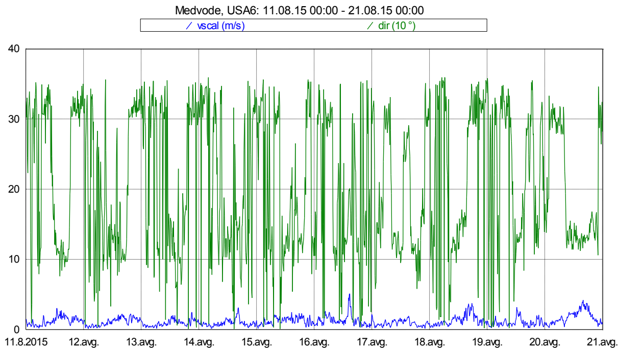
Slika 17: Smer in hitrost vetra med 11. 8. 2015 in 20. 8. 2015.
