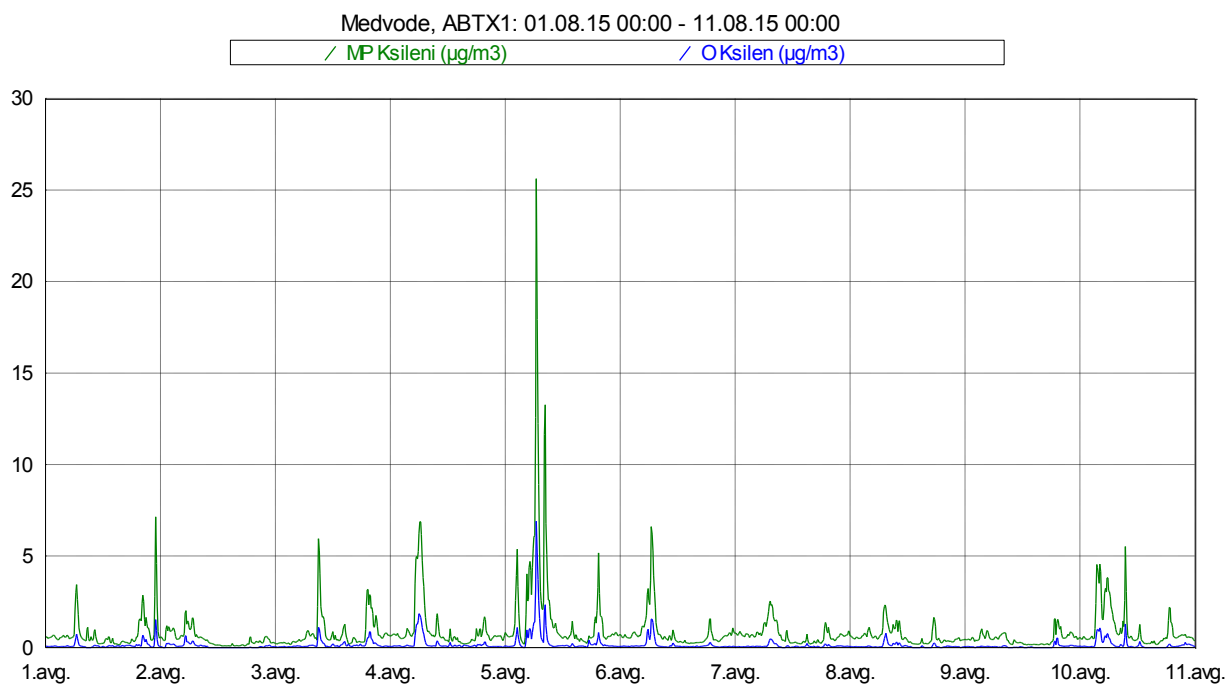
Slika 12: Imisijske koncentracije M&P in O ksilena med vključno 1. 8. 2015 in 10. 8. 2015.
