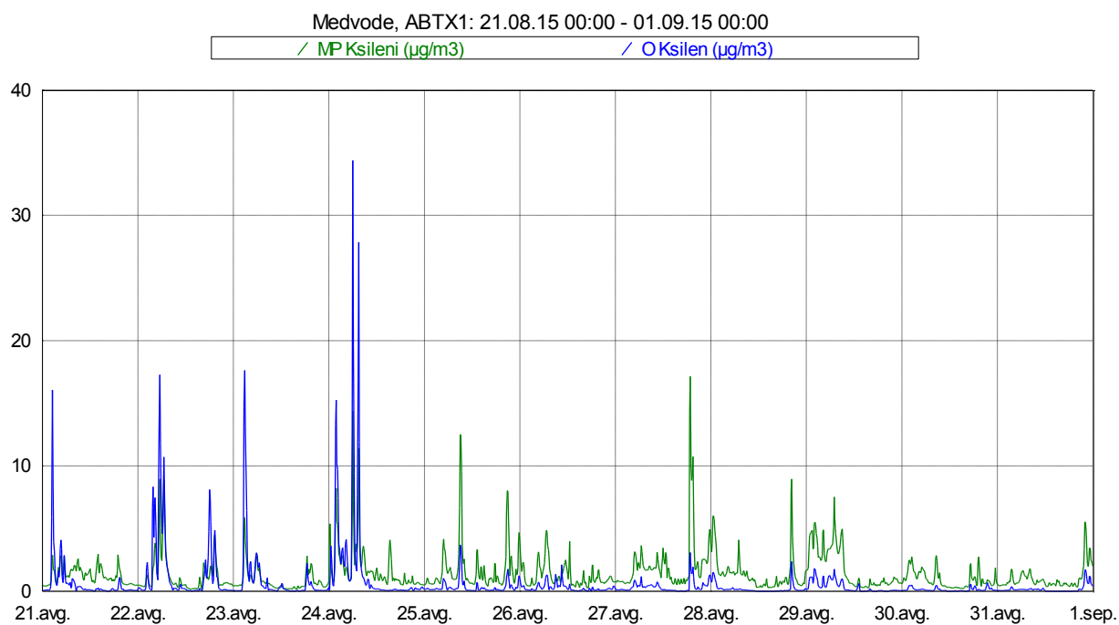
Slika 14: Imisijske koncentracije M&P in O ksilena med 21. 8. 2015 in 31. 8. 2015.
