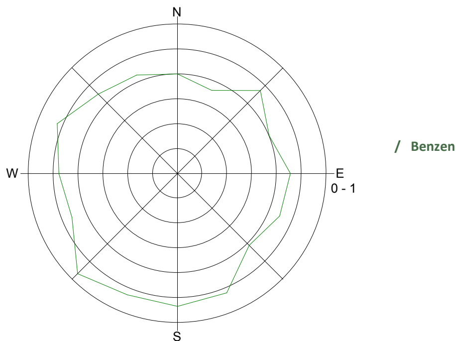
Slika 6: Roža onesnaženosti – benzen, avgust 2015.
