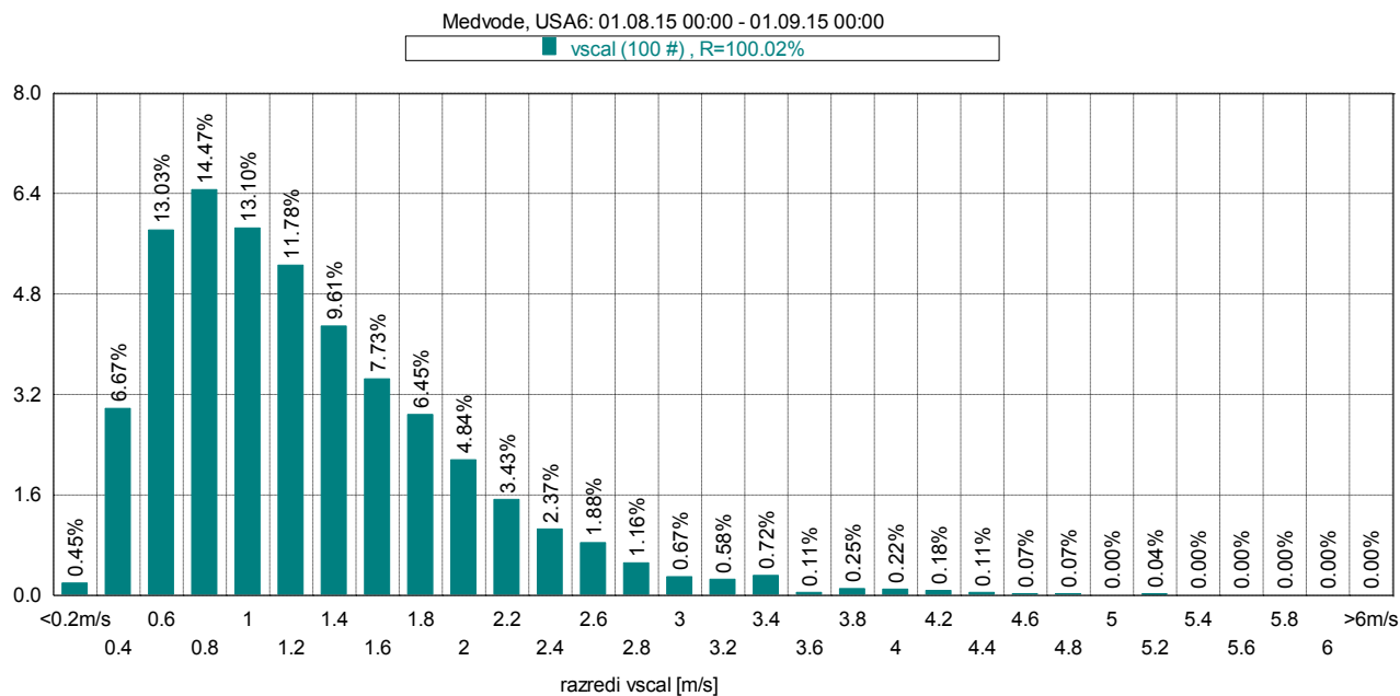
Slika 20: Frekvenčna porazdelitev po hitrosti vetra, avgust 2015.
