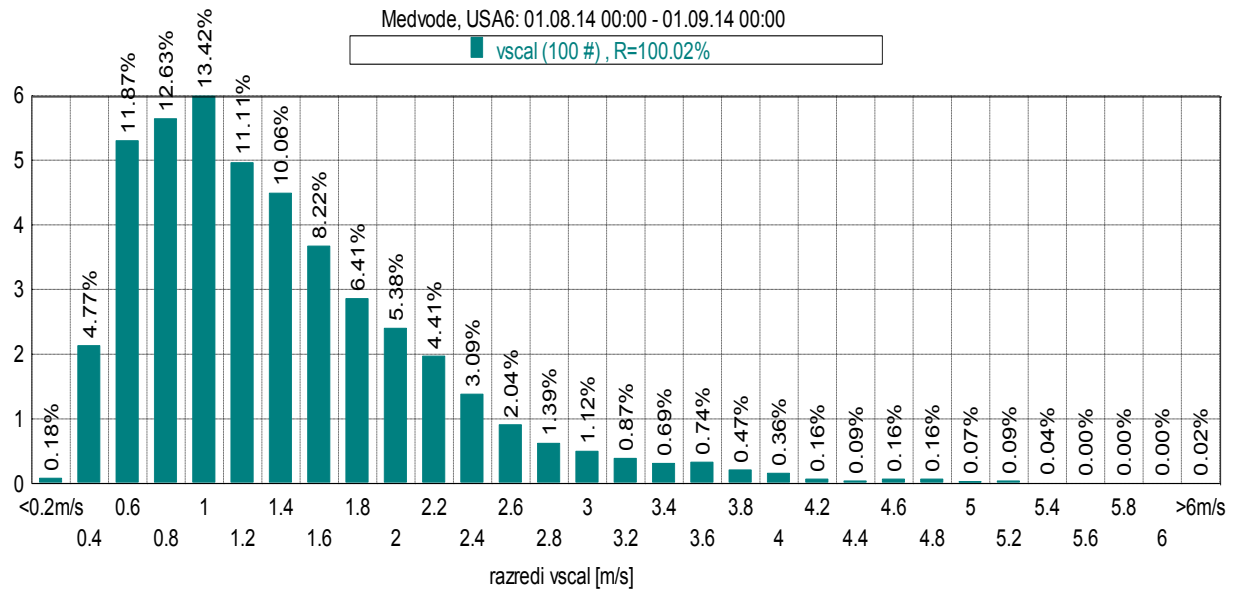
Slika 20: Frekvenčna porazdelitev po hitrosti vetra, avgust 2014.
