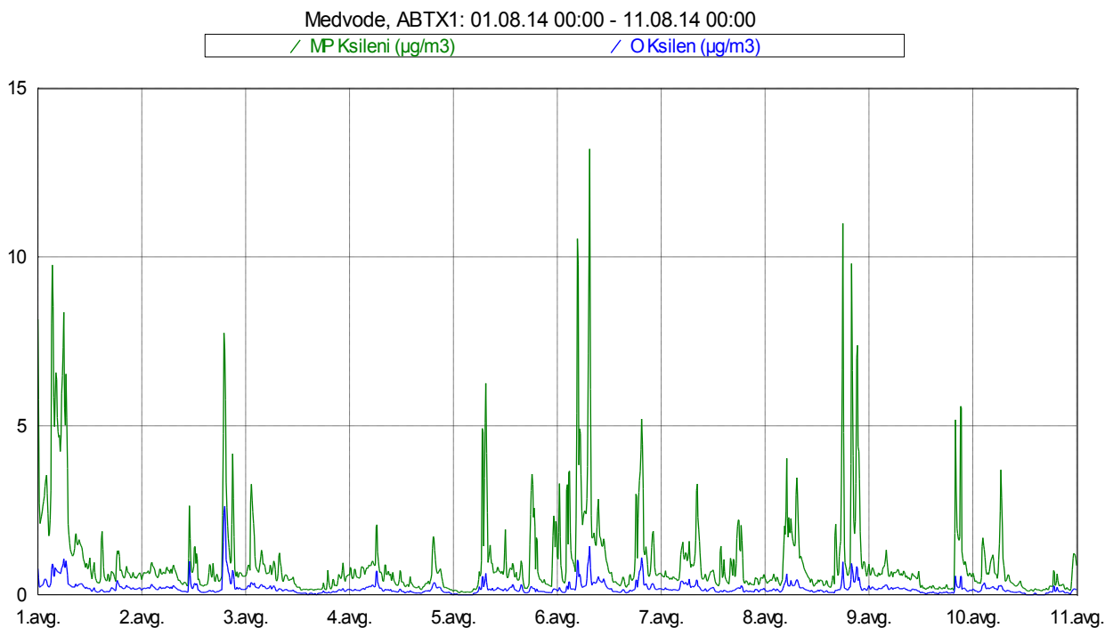
Slika 12: Imisijske koncentracije M&P in O ksilena med vključno 1. 8. 2014 in 10. 8. 2014.
