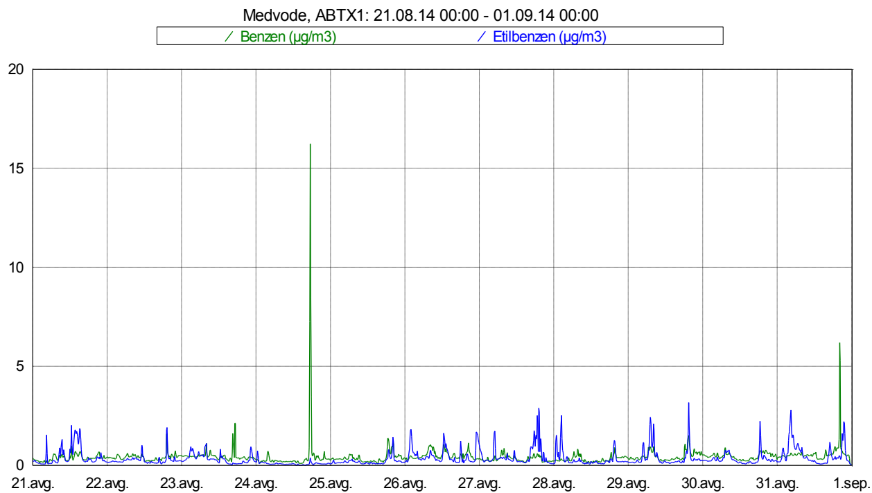
Slika 5: Imisijske koncentracije benzena in etilbenzena med 21. 8. 2014 in 31. 8. 2014.
