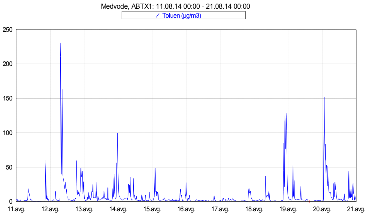
Slika 9: Imisijske koncentracije toluena med 11. 8. 2014 in 20. 8. 2014.
