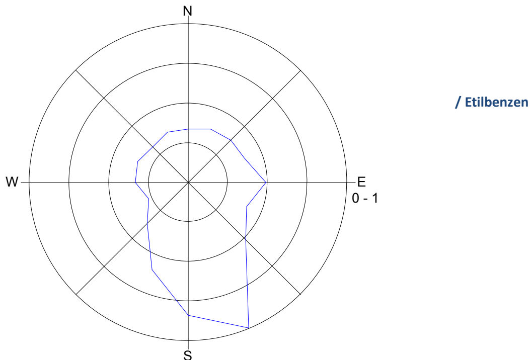
Slika 7: Roža onesnaženosti – etilbenzen, avgust 2014.
