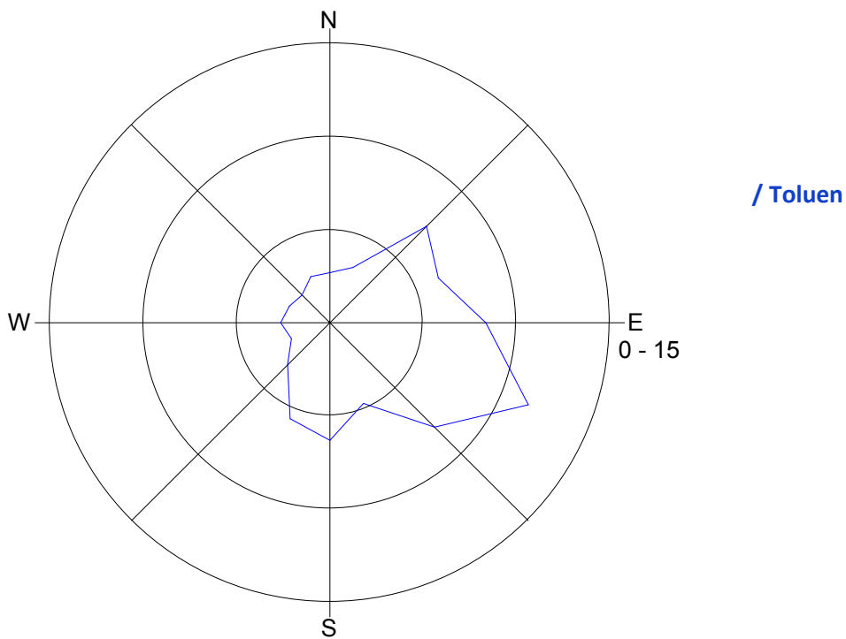
Slika 11: Roža onesnaženost - toluen, avgust 2014.
