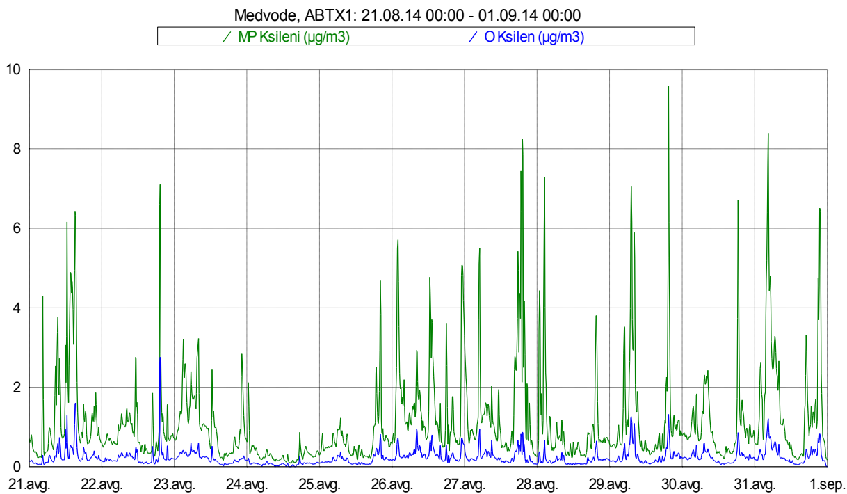
Slika 14: Imisijske koncentracije M&P in O ksilena med 21. 8. 2014 in 31. 8. 2014.
