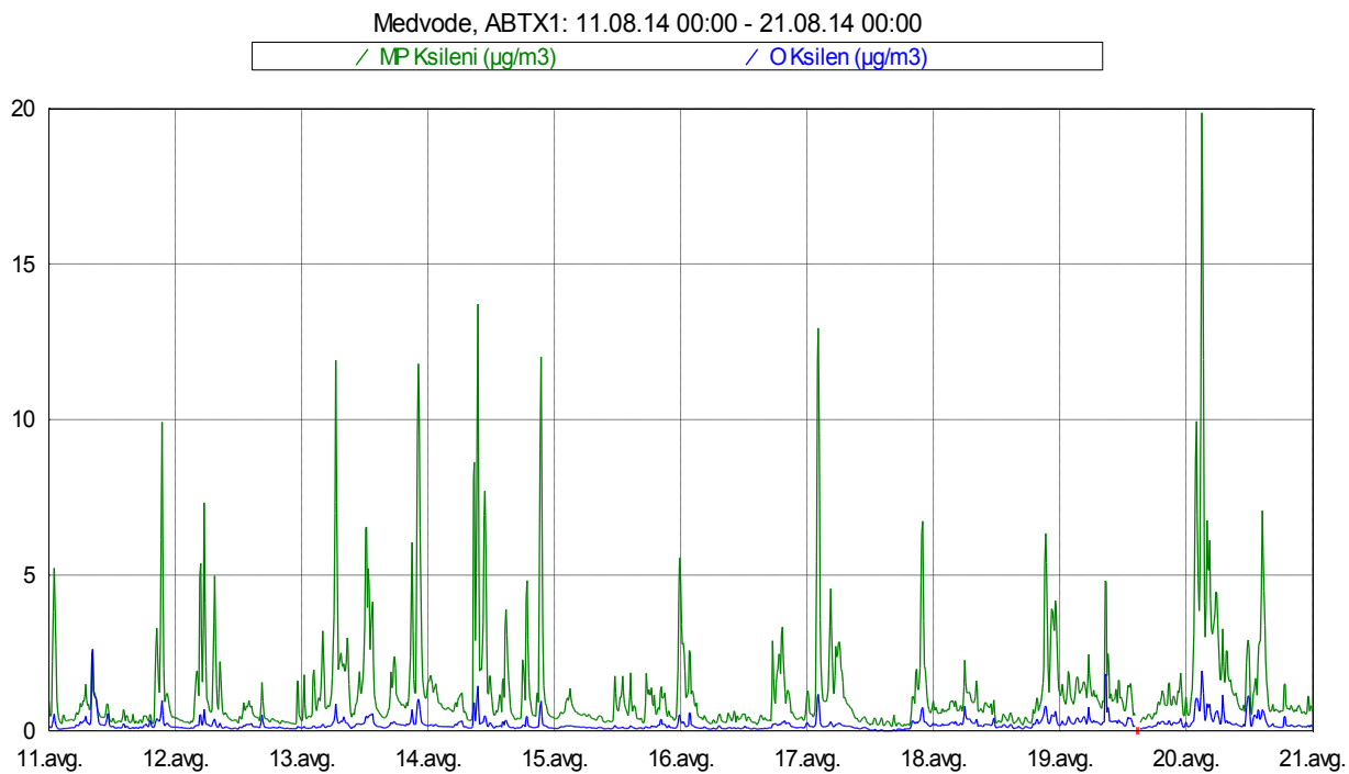
Slika 13: Imisijske koncentracije M&P in O ksilena med 11. 8. 2014 in 20. 8. 2014.
