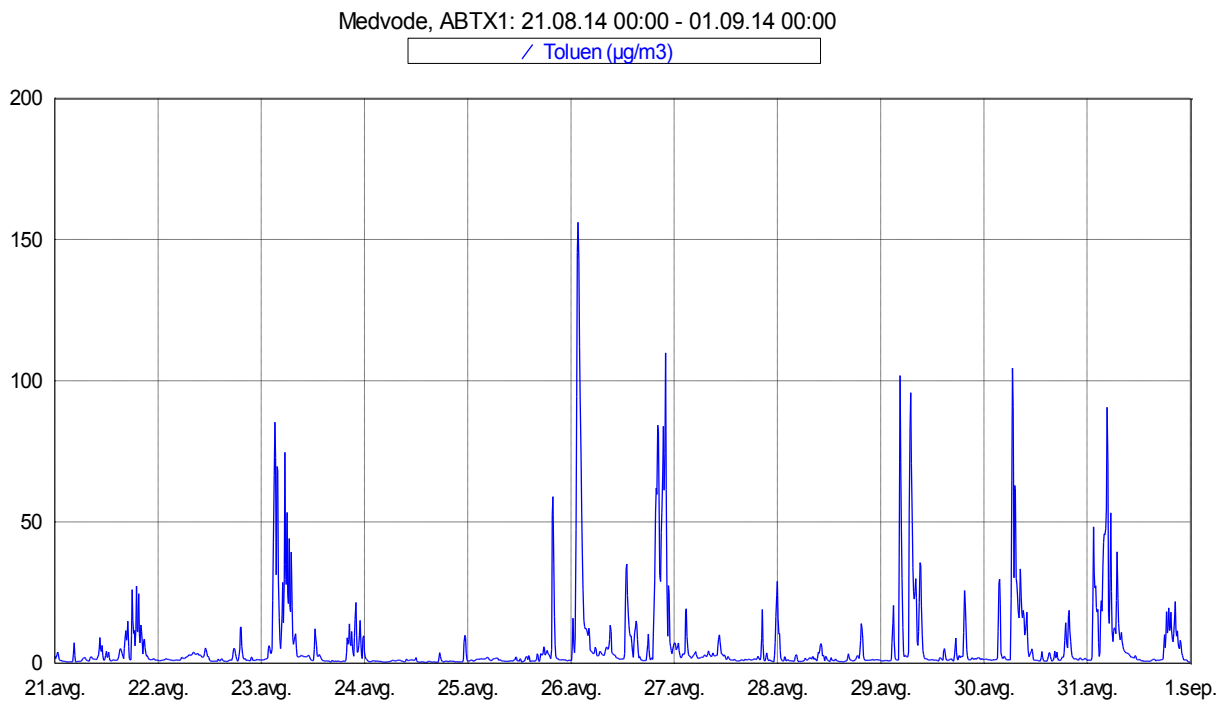
Slika 10: Imisijske koncentracije toluena med 21. 8. 2014 in 31. 8. 2014.
