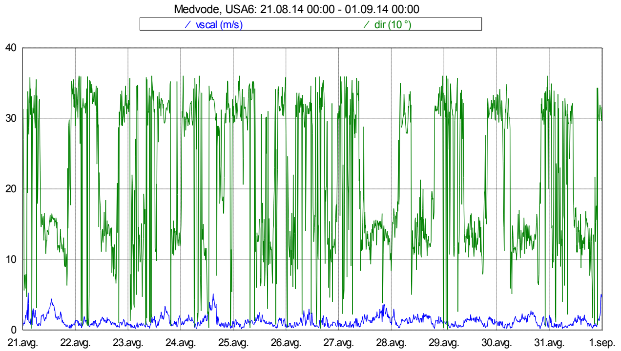
Slika 18: Smer in hitrost vetra med 21. 8. 2014 in 31. 8. 2014.
