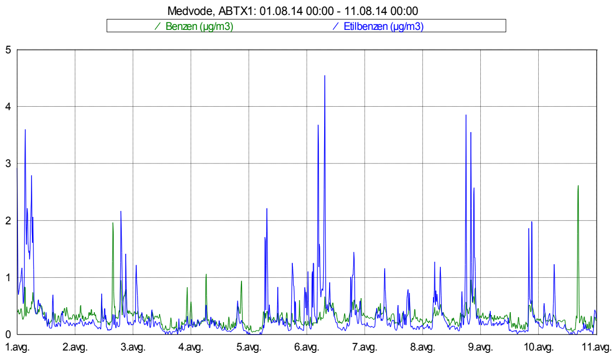
Slika 3: Imisijske koncentracije benzena in etilbenzena med vključno 1. 8. 2014 in 10. 8. 2014.
