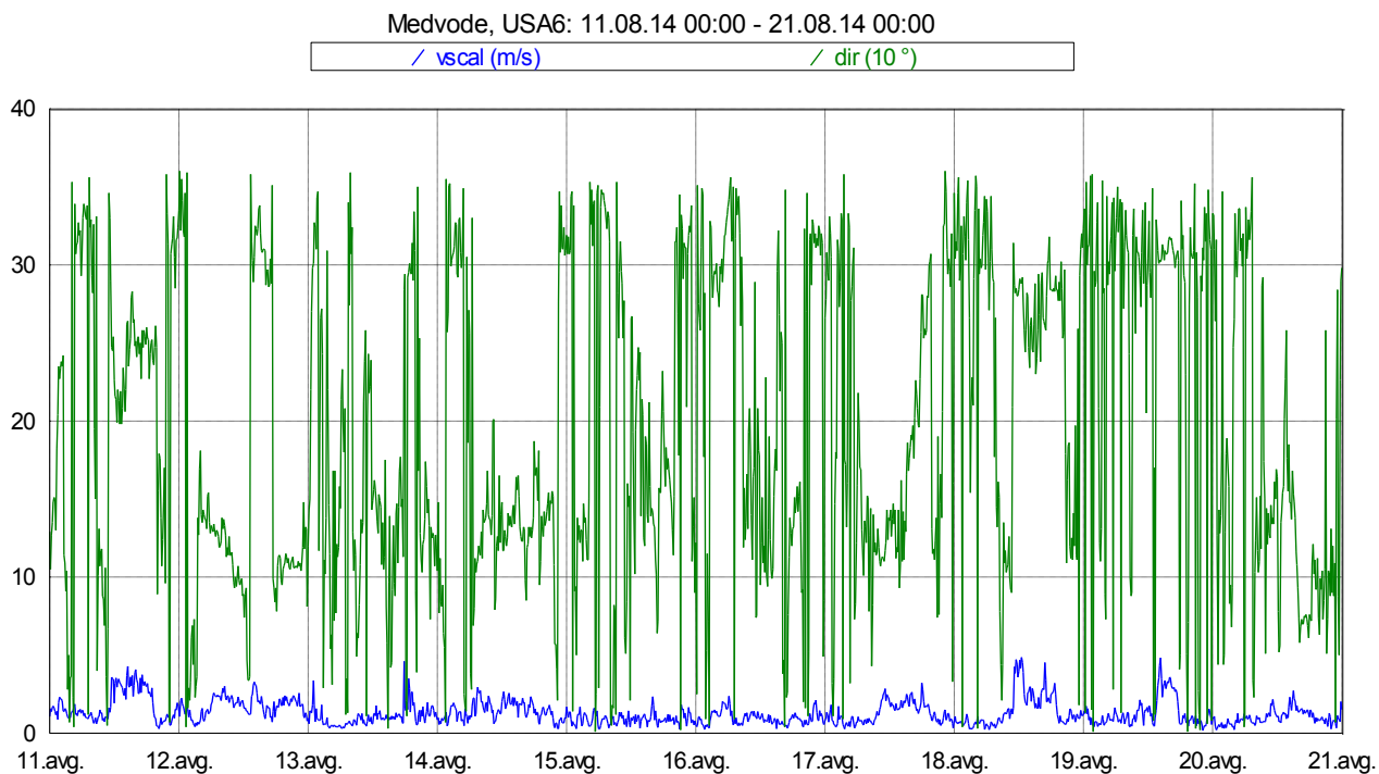
Slika 17: Smer in hitrost vetra med 11. 8. 2014 in 20. 8. 2014.
