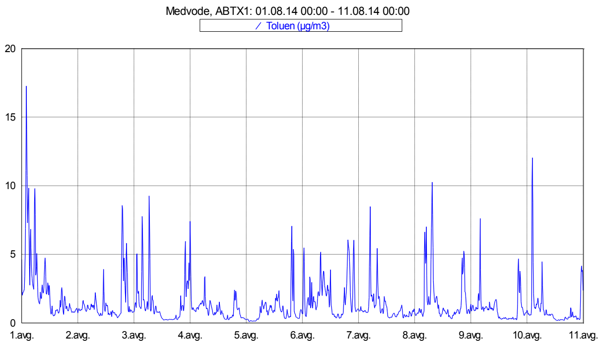
Slika 8: Imisijske koncentracije toluena med vključno 1. 8. 2014 in 10. 8. 2014.
