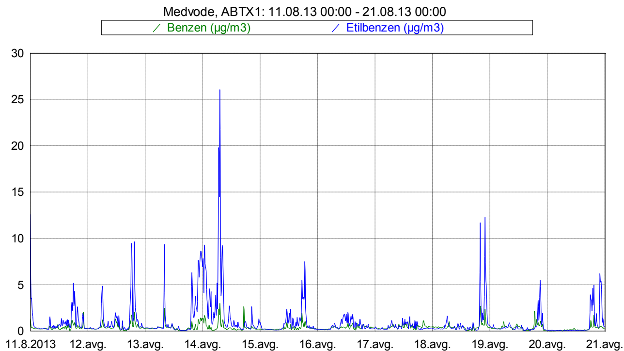
Slika 4: Imisijske koncentracije benzena in etilbenzena med 11. 8. 2013 in 20. 8. 2013.
