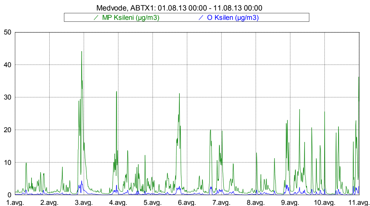
Slika 11: Imisijske koncentracije M&P in O ksilena med vključno 1. 8. 2013 in 10. 8. 2013.
