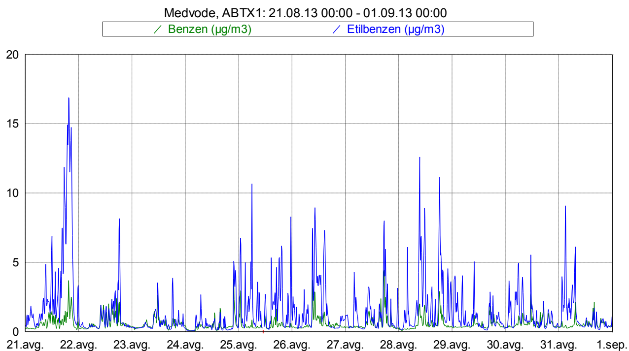
Slika 5: Imisijske koncentracije benzena in etilbenzena med 21. 8. 2013 in 31. 8. 2013.
