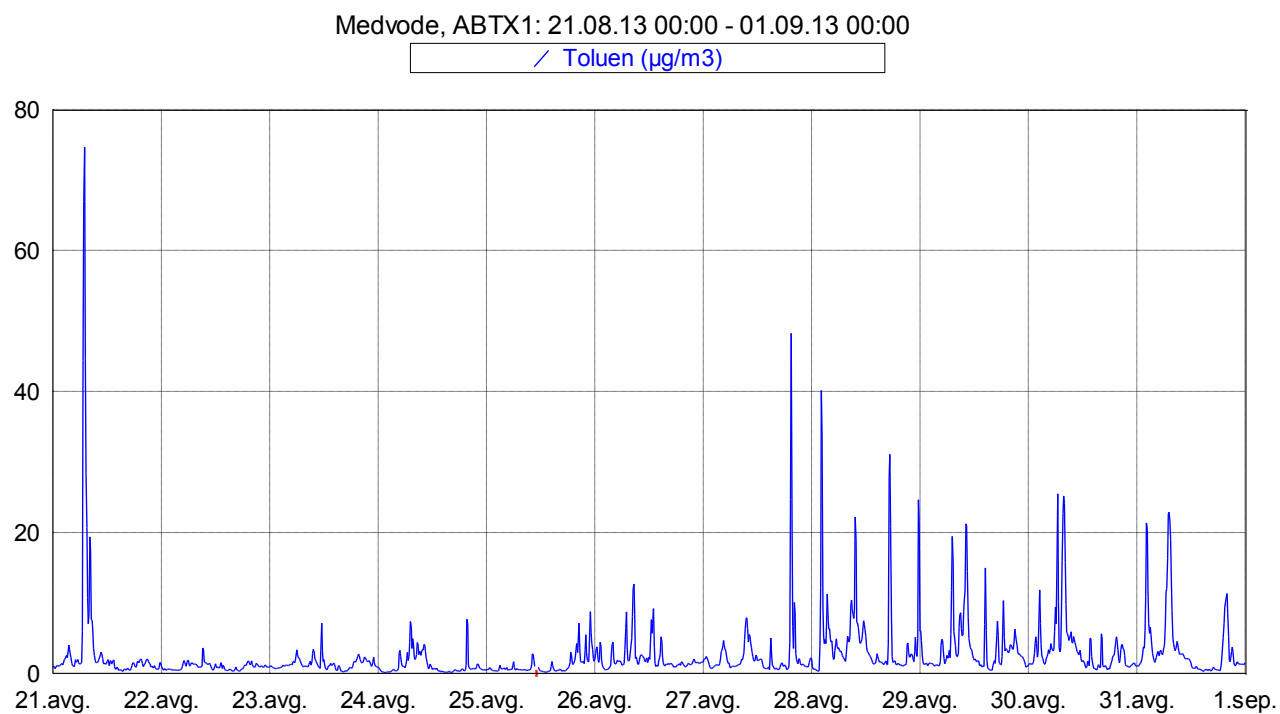
Slika 9: Imisijske koncentracije toluena med 21. 8. 2013 in 1. 8. 2013.
