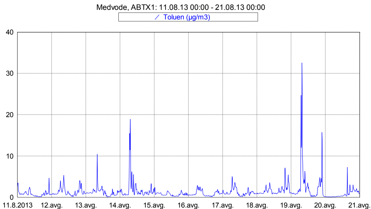
Slika 8: Imisijske koncentracije toluena med 11. 8. 2013 in 20. 8. 2013.
