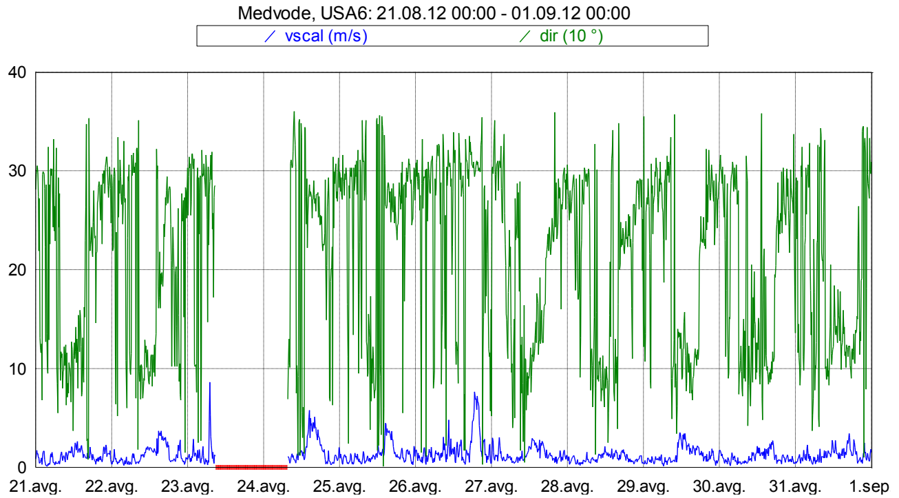
Slika 17: Smer in hitrost vetra med 21. 8. 2012 in 31. 8. 2012.
