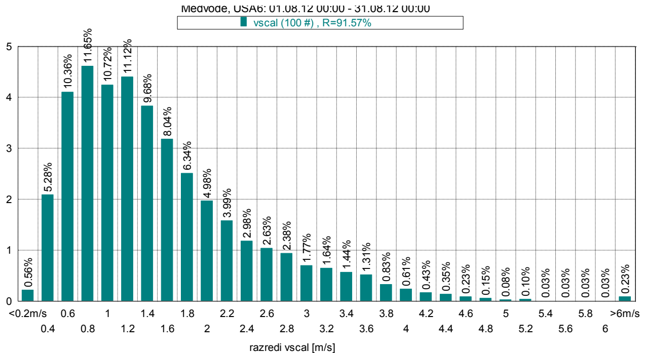
Slika 19: Frekvenčna porazdelitev po hitrosti vetra, avgust 2012.
