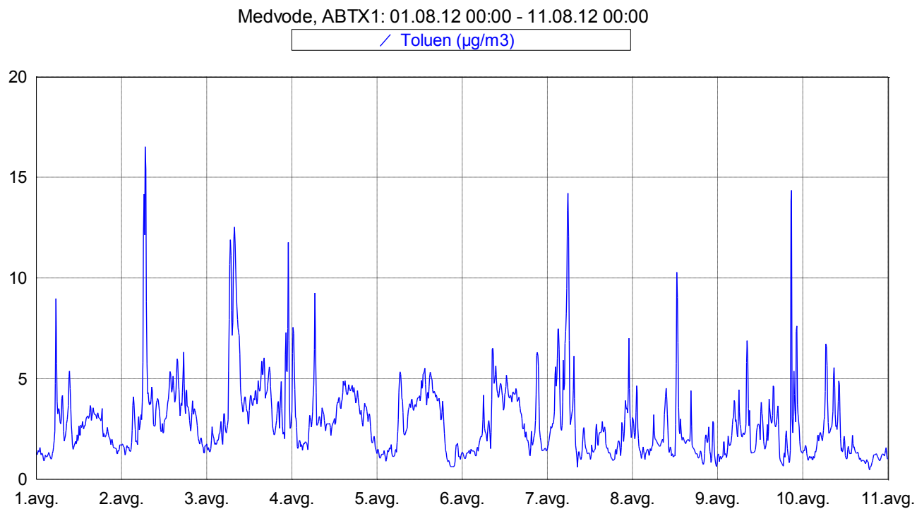
Slika 7: Imisijske koncentracije toluena med vključno 1. 8. 2012 in 10. 8. 2012.
