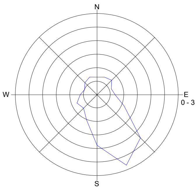
Slika 6: Roža onesnaženosti – benzen (zgoraj) in etilbenzen (spodaj), avgust 2012.
