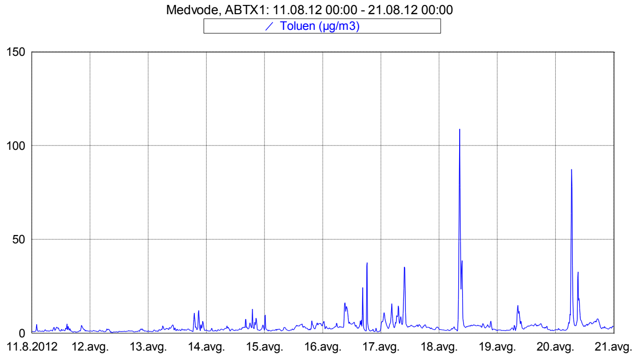
Slika 8: Imisijske koncentracije toluena med 11. 8. 2012 in 20. 8. 2012.
