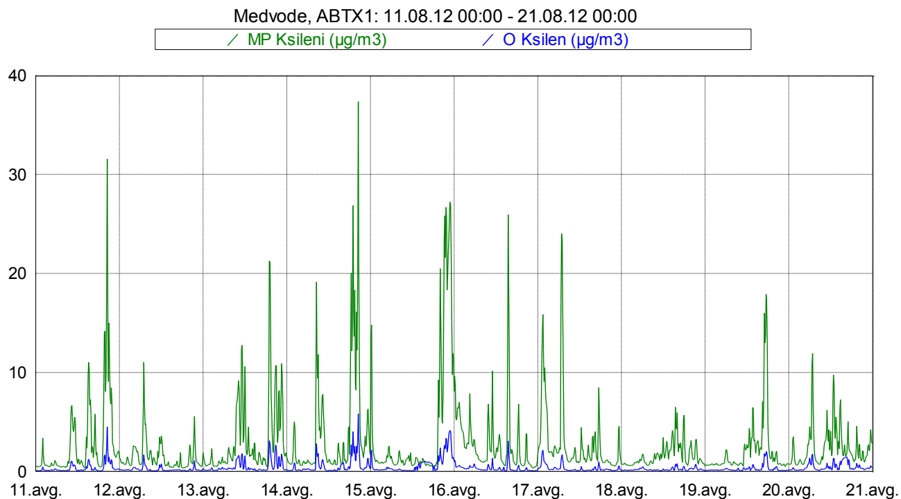
Slika 12: Imisijske koncentracije M&P in O ksilena med 11. 8. 2012 in 20. 8. 2012.
