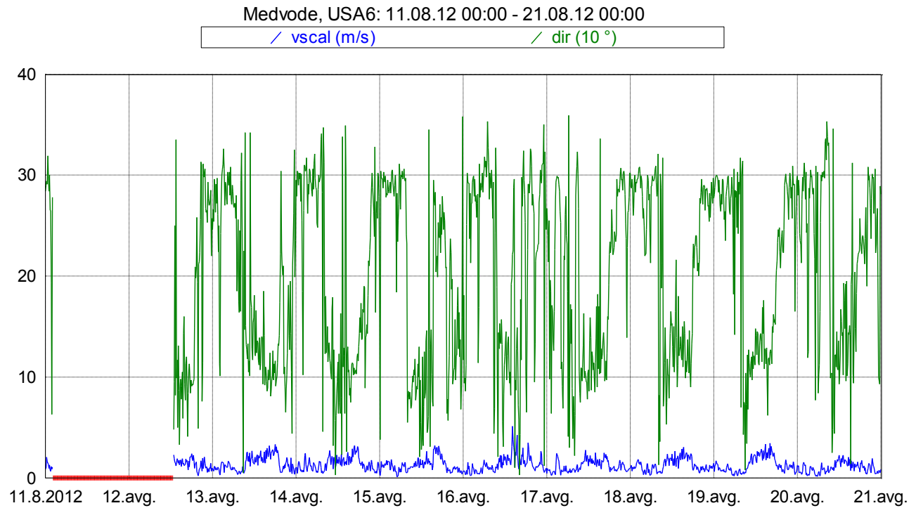
Slika 16: Smer in hitrost vetra med 11. 8. 2012 in 20. 8. 2012.
