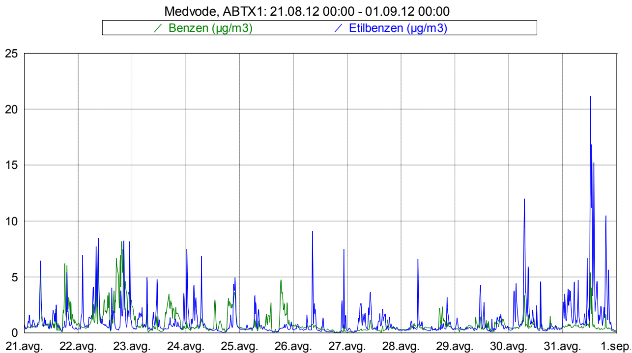
Slika 5: Imisijske koncentracije benzena in etilbenzena med 21. 8. 2012 in 31. 8. 2012.
