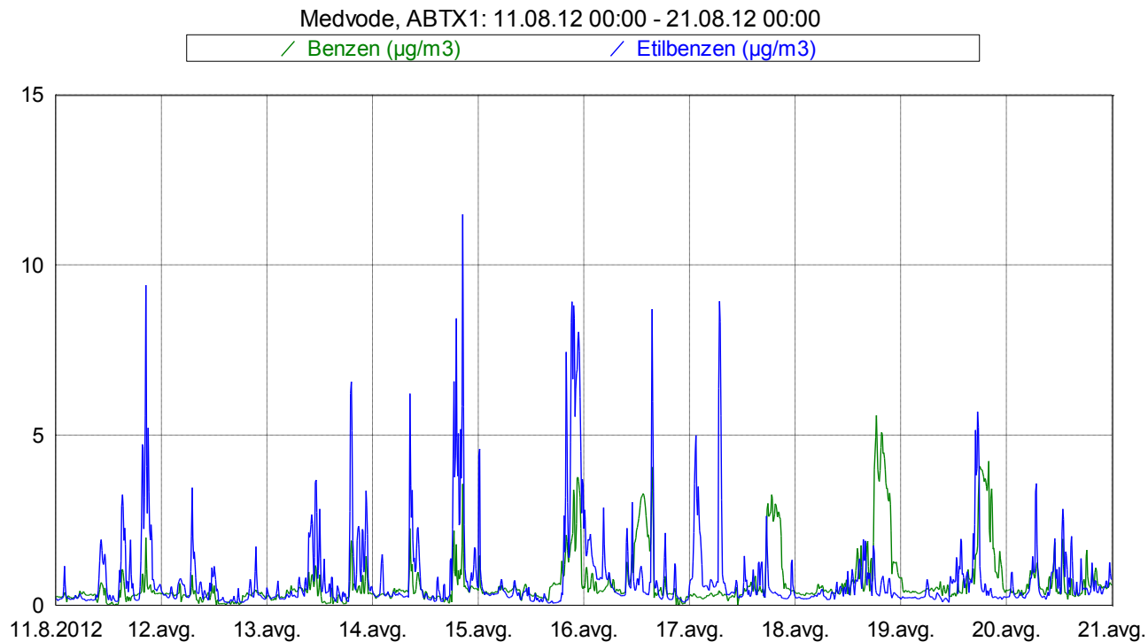
Slika 4: Imisijske koncentracije benzena in etilbenzena med 11. 8. 2012 in 20. 8. 2012.
