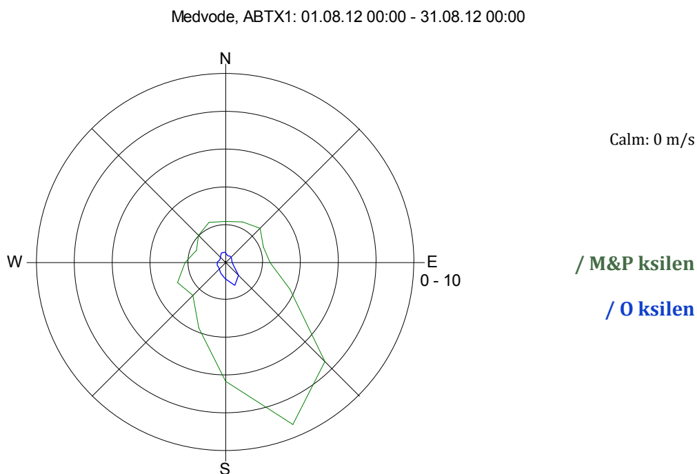
Slika 14: Roža onesnaženosti - M & P ksilen in O ksilen, avgust 2012.
