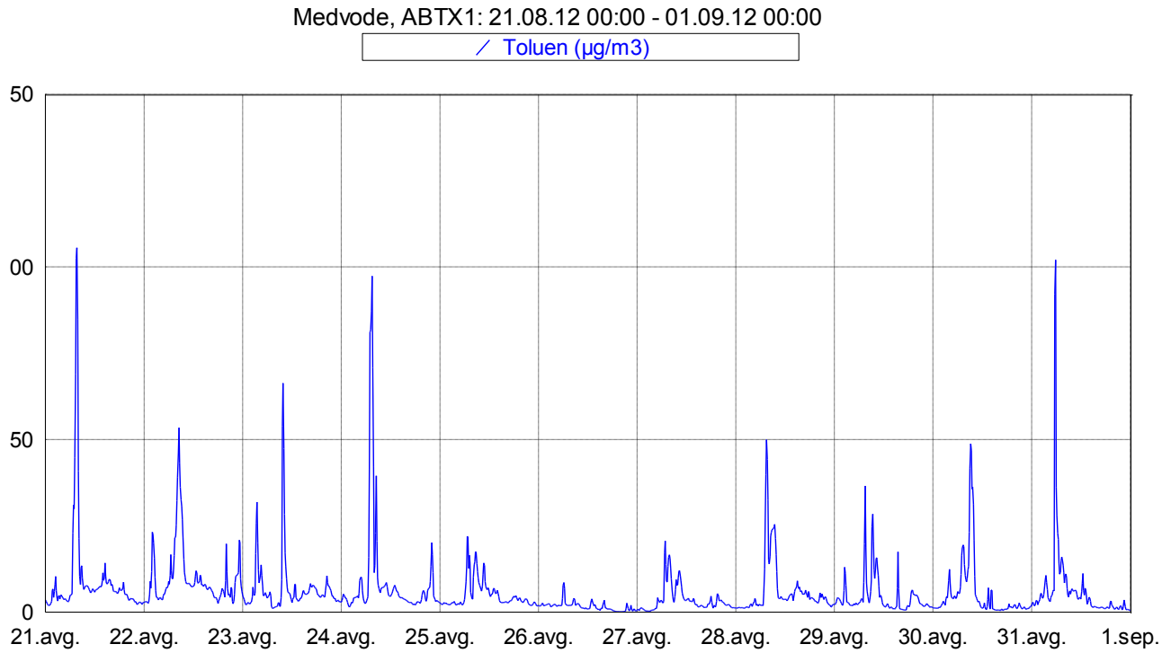
Slika 9: Imisijske koncentracije toluena med 21. 8. 2012 in 31. 8. 2012.
