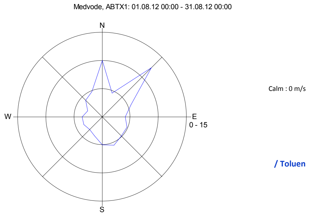
Slika 10: Roža onesnaženost - toluen, avgust 2012.
