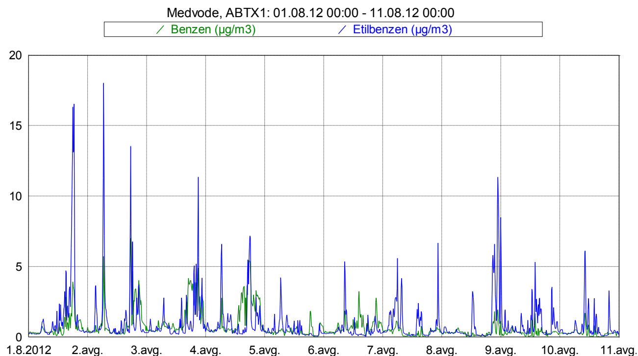
Slika 3: Imisijske koncentracije benzena in etilbenzena med vključno 1. 8. 2012 in 10. 8. 2012.
