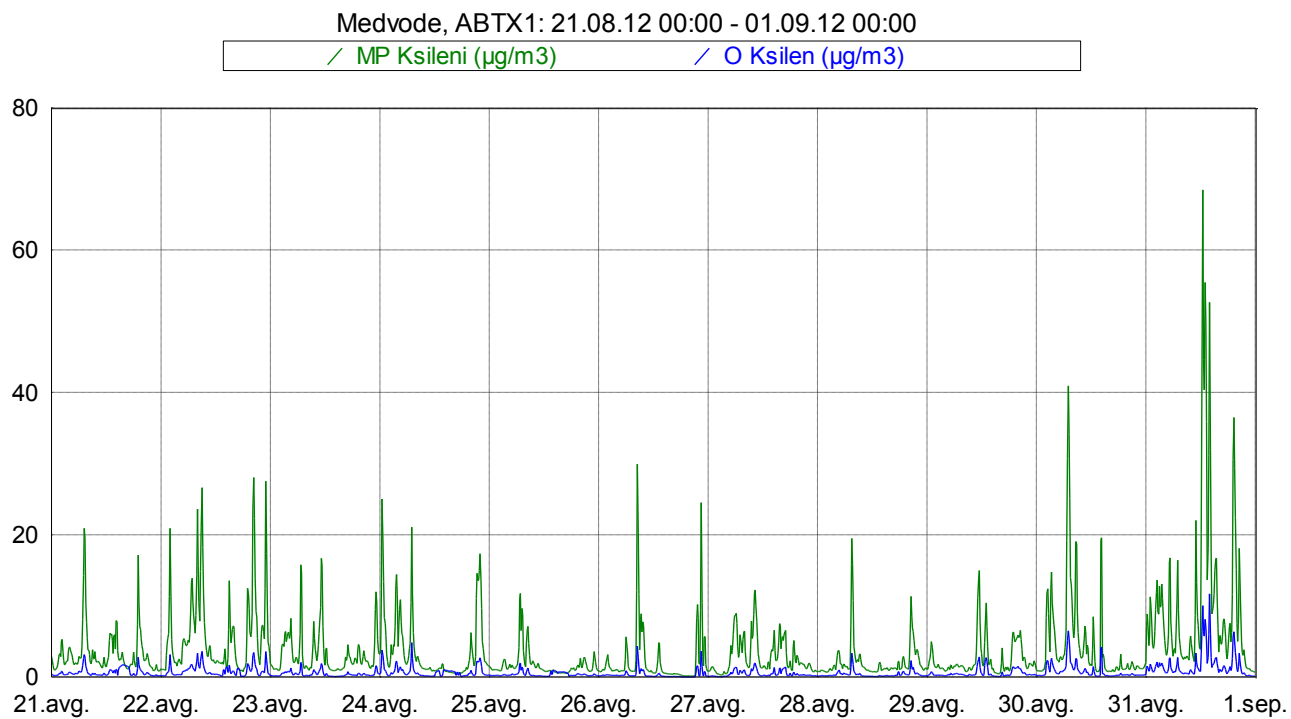
Slika 13: Imisijske koncentracije M&P in O ksilena med 21. 8. 2012 in 31. 8. 2012.
