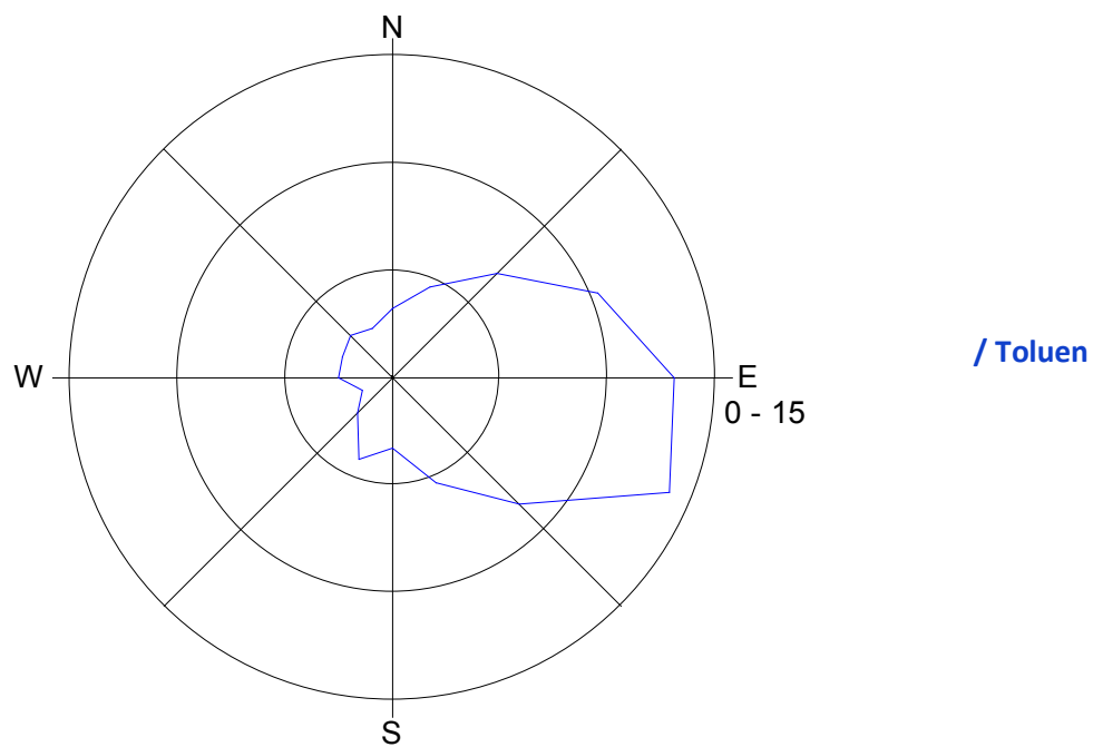
Slika 11: Roža onesnaženost - toluen, april 2016.
