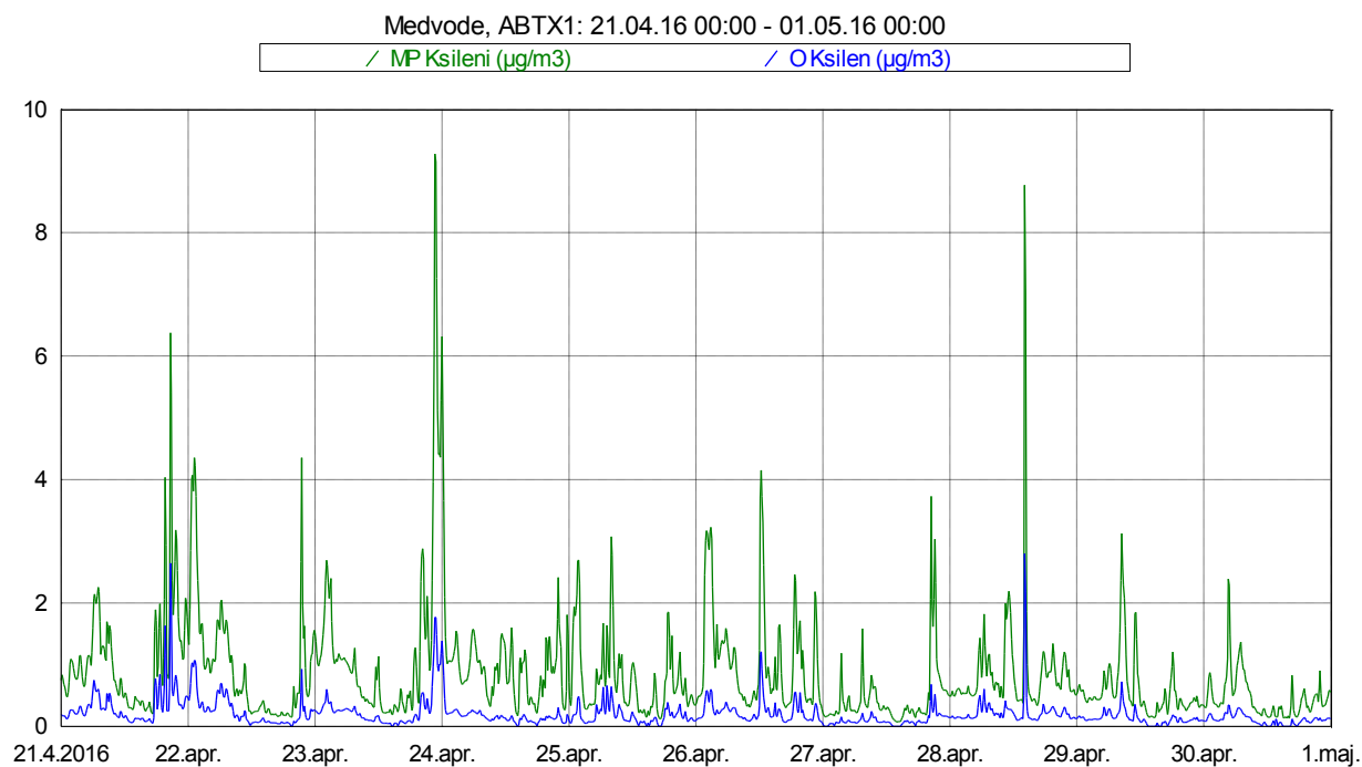
Slika 14: Imisijske koncentracije M&P in O ksilena med 21. 4. 2016 in 30. 4. 2016.
