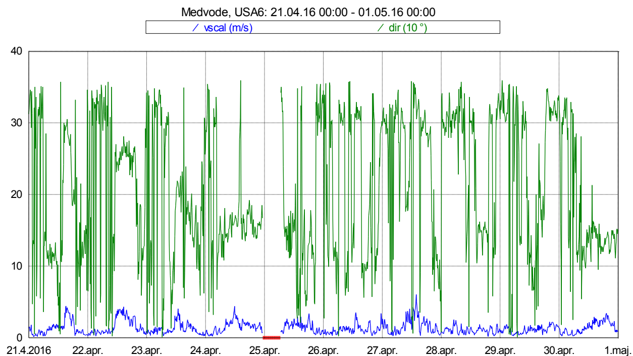
Slika 18: Smer in hitrost vetra med 21. 4. 2016 in 30. 4. 2016.
