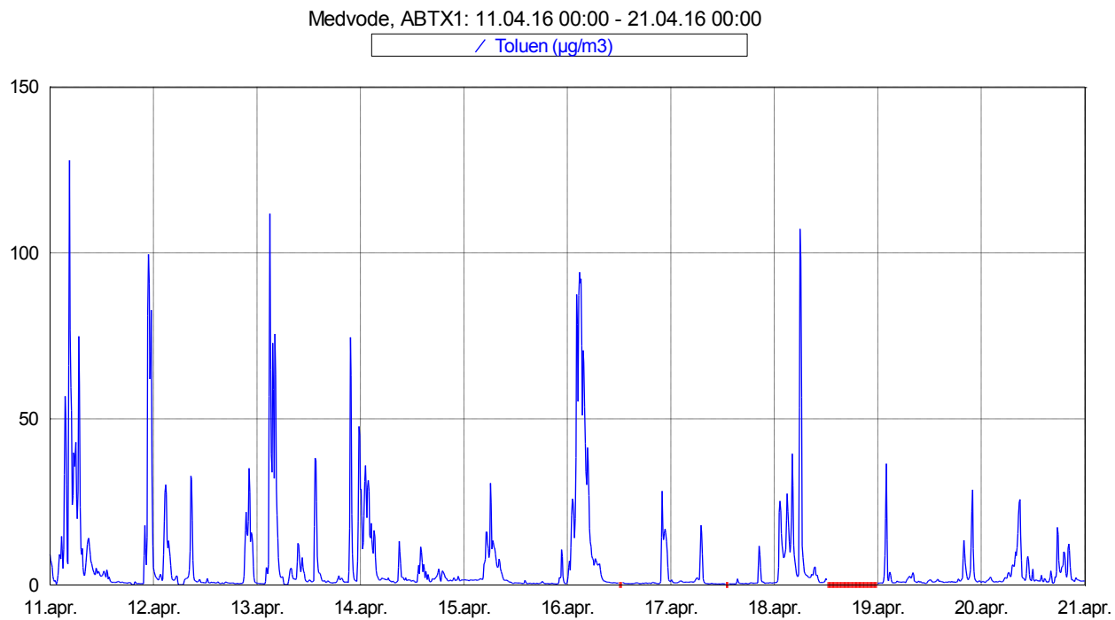
Slika 9: Imisijske koncentracije toluena med 11. 4. 2016 in 20. 4. 2016.
