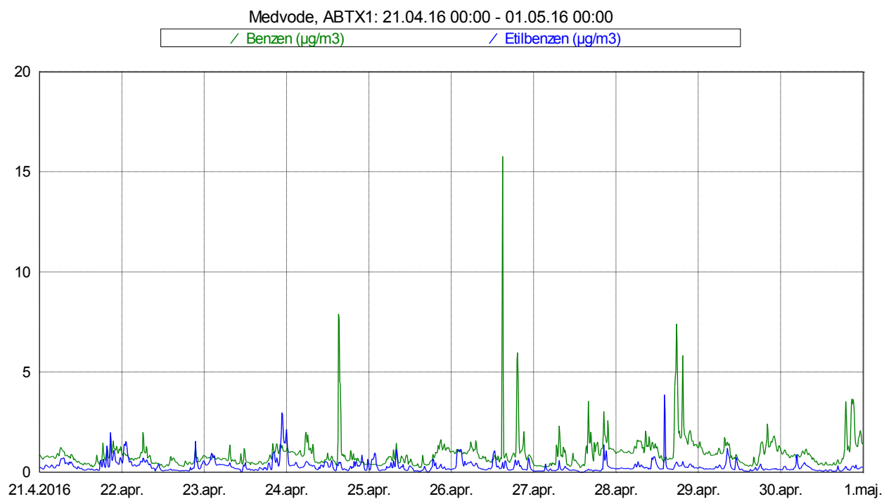
Slika 5: Imisijske koncentracije benzena in etilbenzena med 21. 4. 2016 in 30. 4. 2016.
