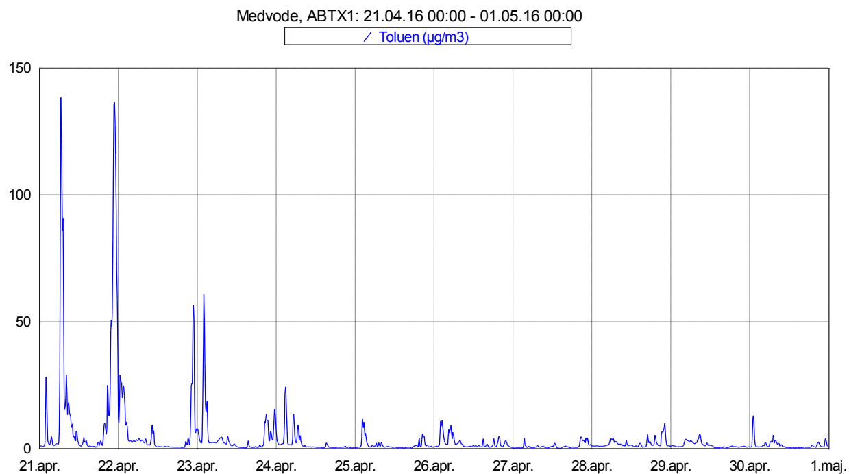
Slika 10: Imisijske koncentracije toluenta med 21. 4. 2016 in 30. 4. 2016.
