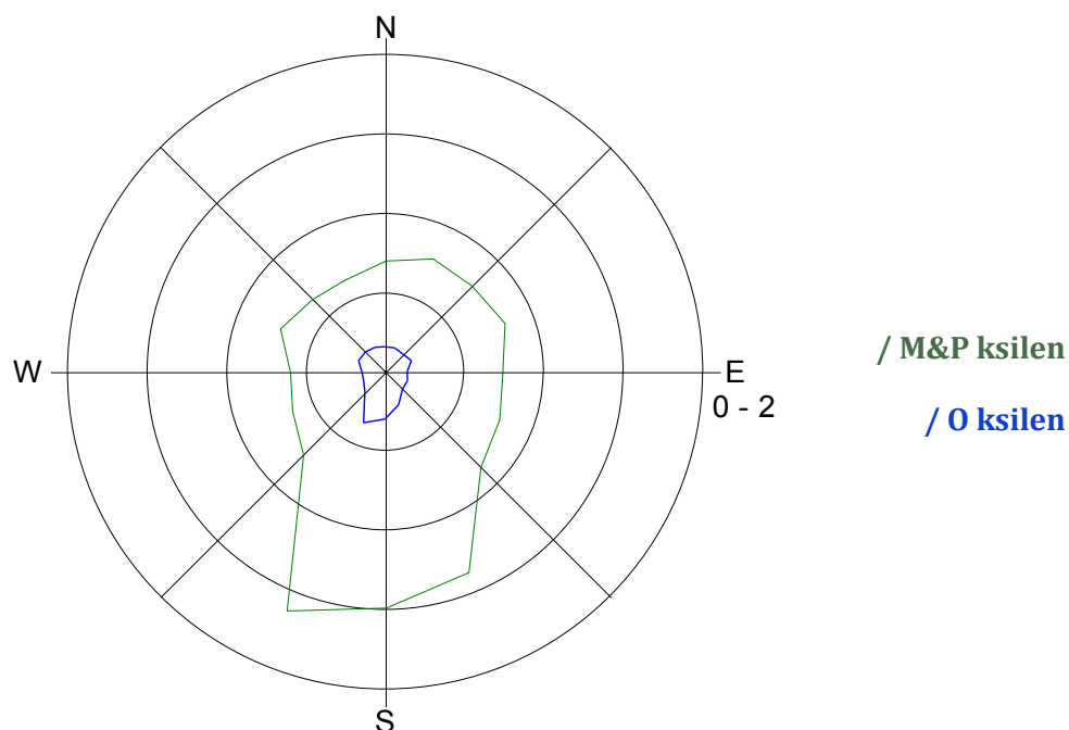
Slika 15: Roža onesnaženosti - M & P ksilen in O ksilen, april 2016.
