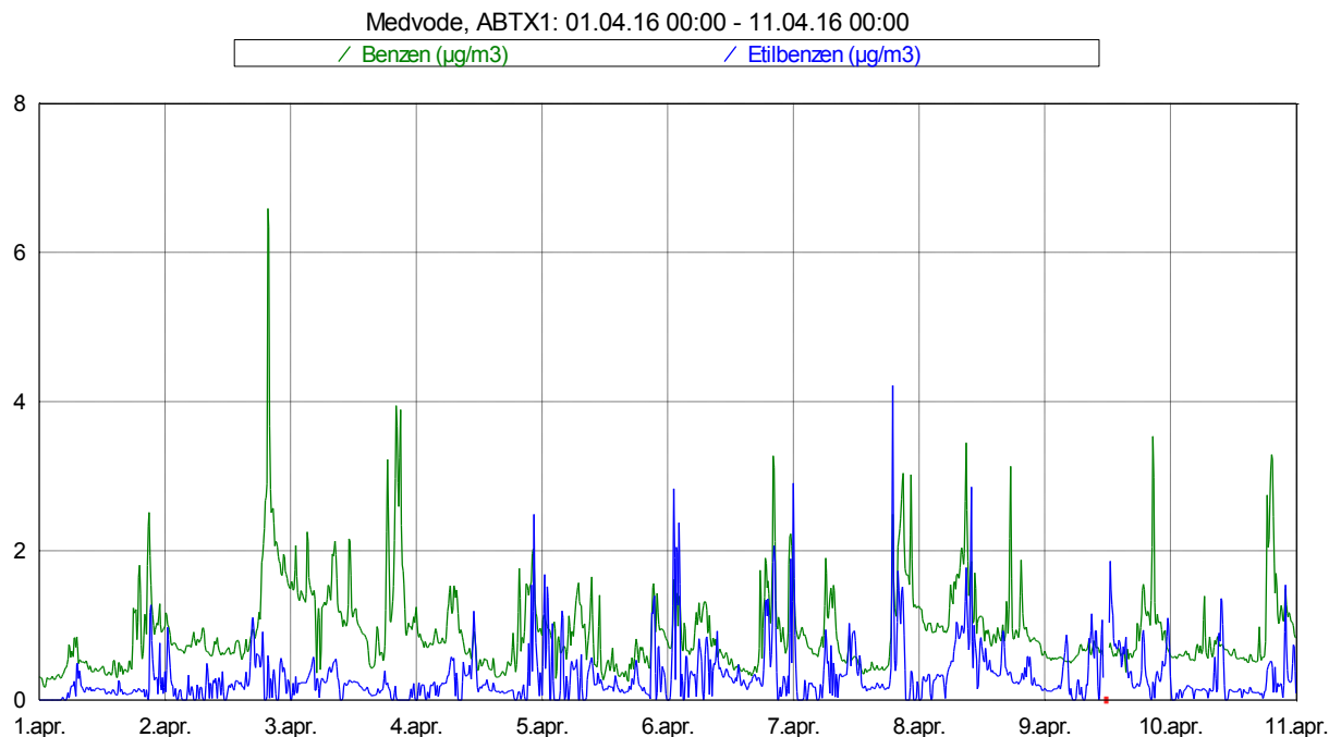
Slika 3: Imisijske koncentracije benzena in etilbenzena med vključno 1. 4. 2016 in 10. 4. 2016.
