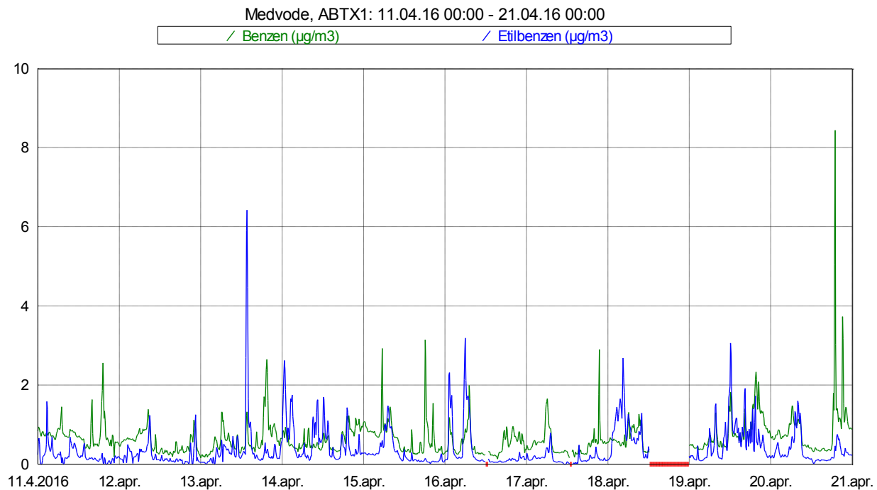
Slika 4: Imisijske koncentracije benzena in etilbenzena med 11. 4. 2016 in 20. 4. 2016.
