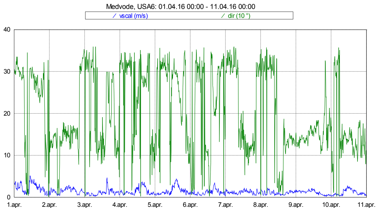
Slika 16: Smer in hitrost vetra med 1. 4. 2016 in 10. 4. 2016.
