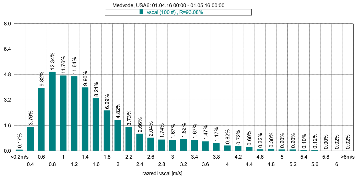
Slika 20: Frekvenčna porazdelitev po hitrosti vetra, april 2016.
