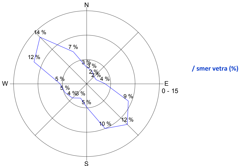
Slika 19: Roža vetrov, april 2016.
