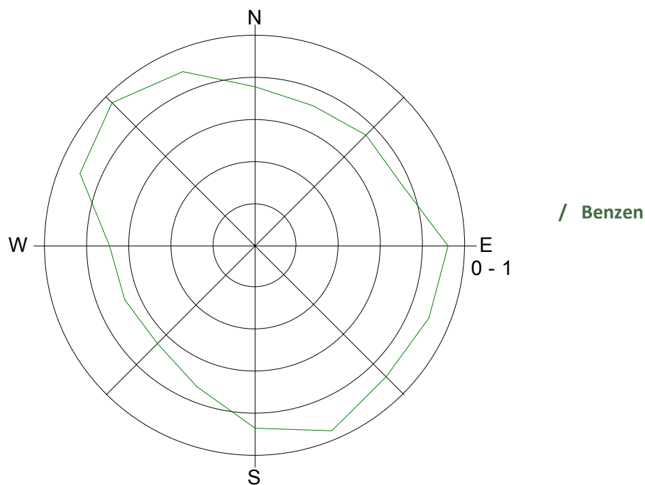
Slika 6: Roža onesnaženosti – benzen, april 2016.
