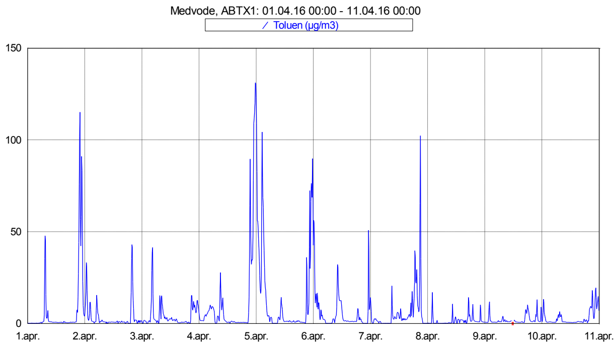
Slika 8: Imisijske koncentracije toluena med vključno 1. 4. 2016 in 10. 4. 2016.
