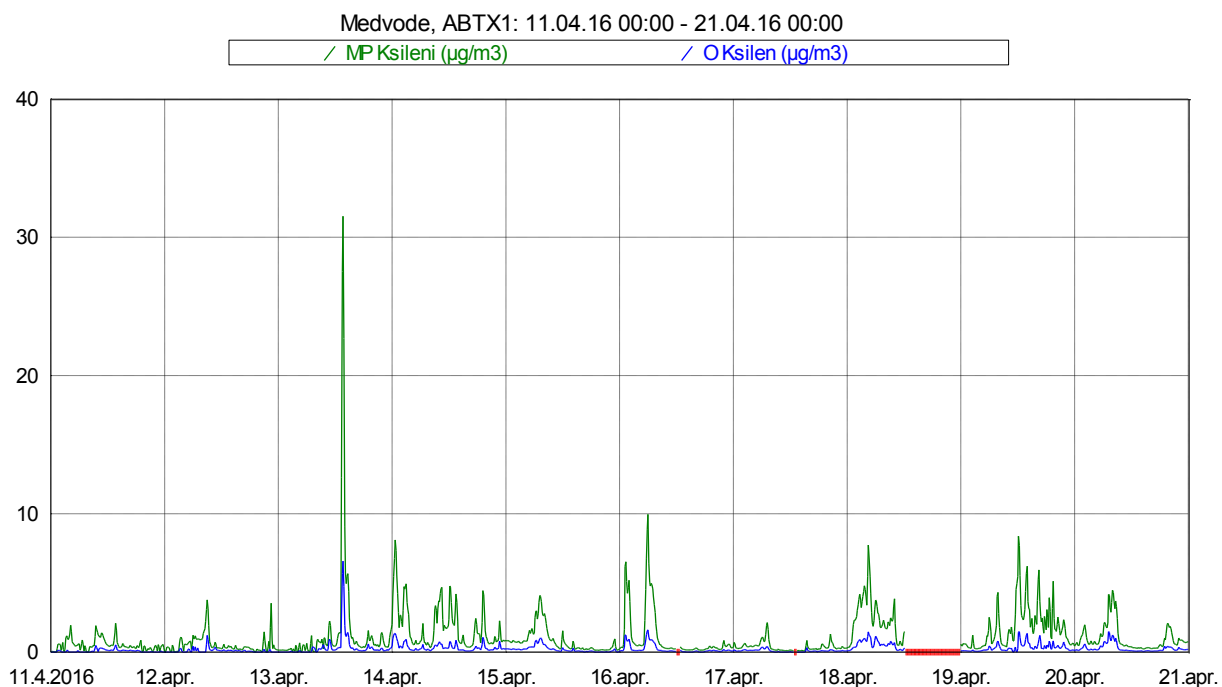
Slika 13: Imisijske koncentracije M&P in O ksilena med 11. 4. 2016 in 20. 4. 2016.
