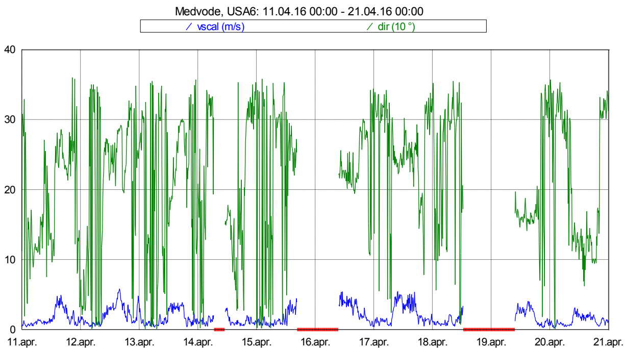
Slika 17: Smer in hitrost vetra med 11. 4. 2016 in 20. 4. 2016.
