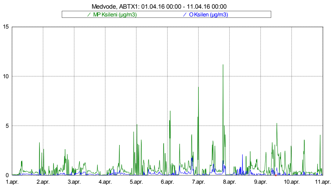
Slika 12: Imisijske koncentracije M&P in O ksilena med vključno 1. 4. 2016 in 10. 4. 2016.
