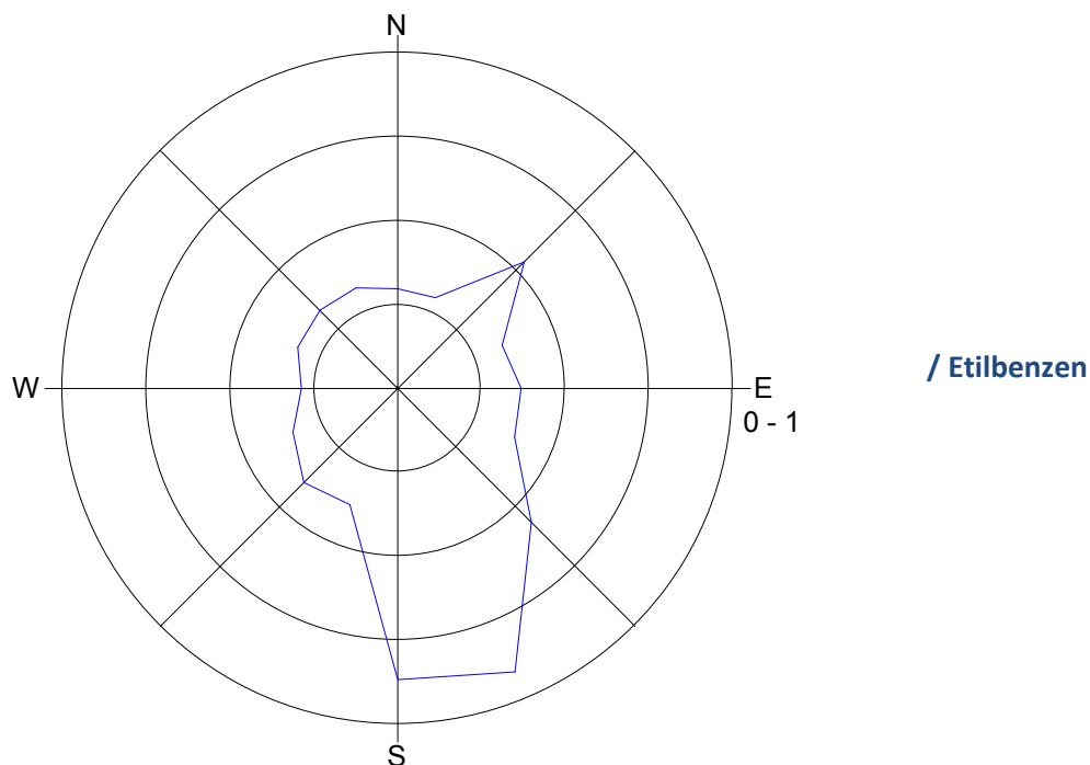
Slika 7: Roža onesnaženosti – etilbenzen, april 2015.
