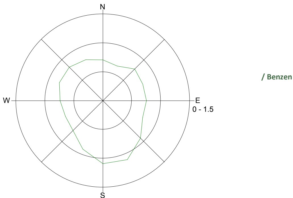
Slika 5: Imisijske koncentracije benzena in etilbenzena med 21. 4. 2015 in 30. 4. 2015.
