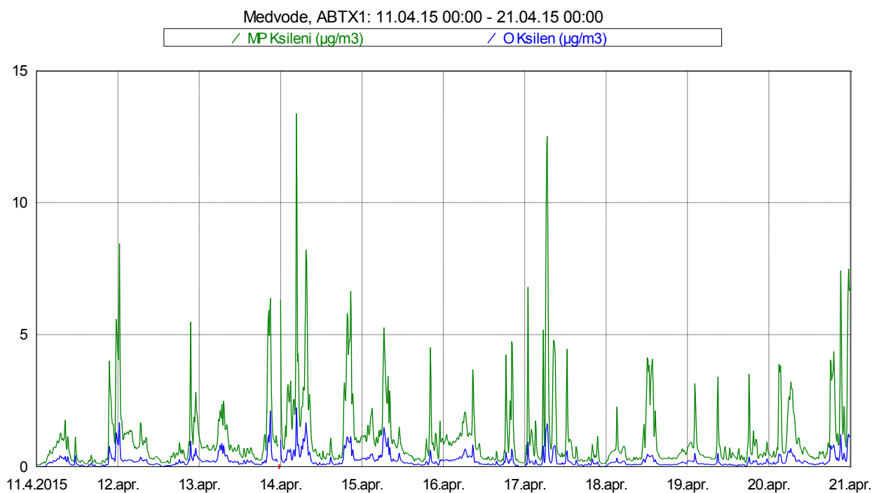
Slika 13: Imisijske koncentracije M&P in O ksilena med 11. 4. 2015 in 20. 4. 2015.
