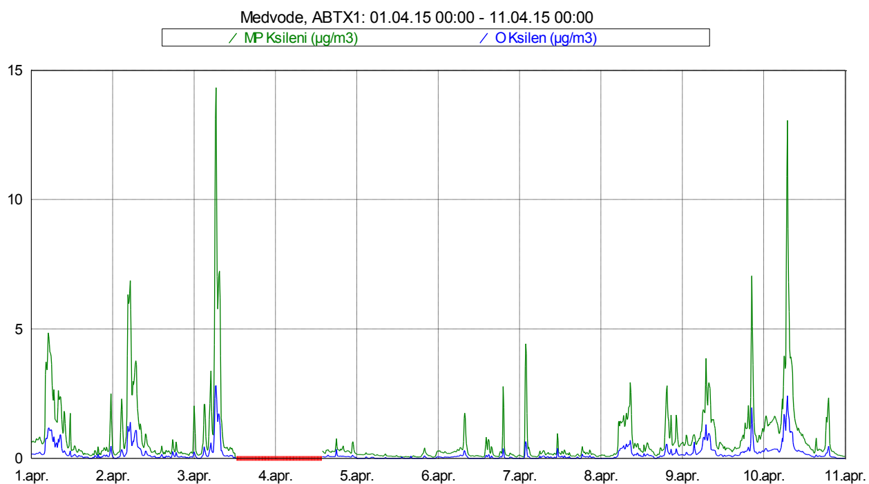
Slika 12: Imisijske koncentracije M&P in O ksilena med vključno 1. 4. 2015 in 10. 4. 2015.
