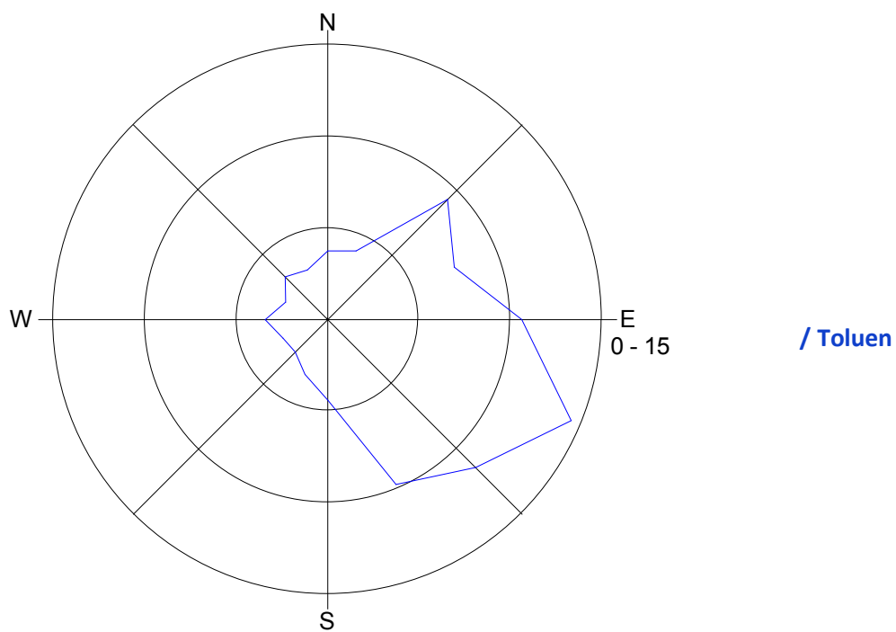
Slika 10: Imisijske koncentracije toluenta med 21. 4. 2015 in 30. 4. 2015.
