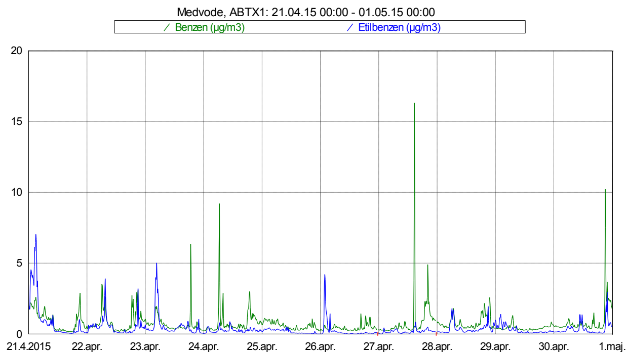
Slika 5: Imisijske koncentracije benzena in etilbenzena med 21. 4. 2015 in 30. 4. 2015.
