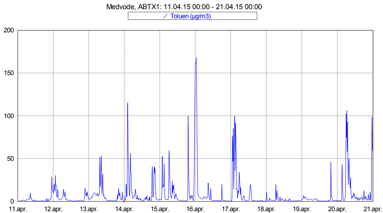
Slika 9: Imisijske koncentracije toluena med 11. 4. 2015 in 20. 4. 2015.
