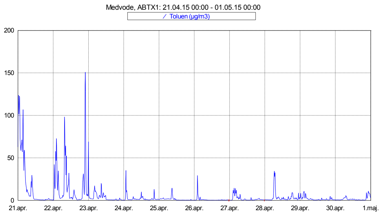
Slika 10: Imisijske koncentracije toluenta med 21. 4. 2015 in 30. 4. 2015.
