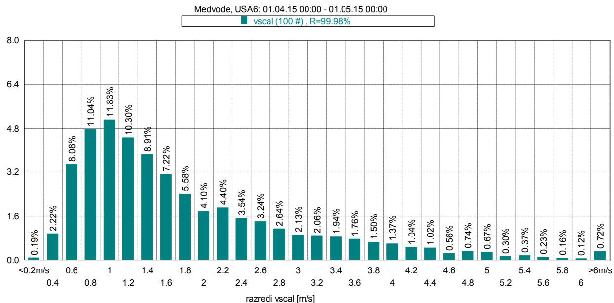
Slika 20: Frekvenčna porazdelitev po hitrosti vetra, april 2015.
