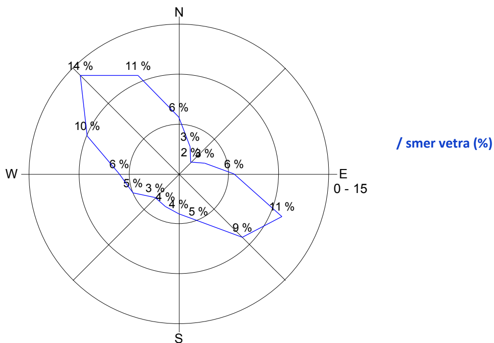
Slika 19: Roža vetrov, april 2015.
