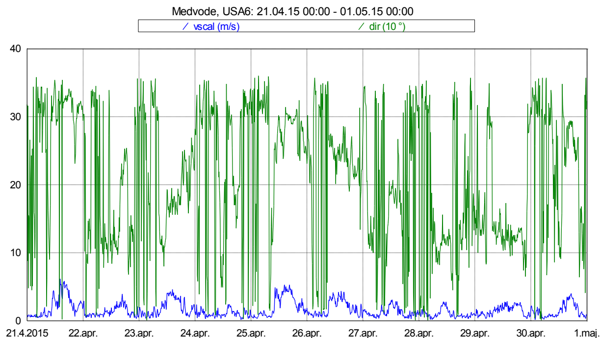
Slika 18: Smer in hitrost vetra med 21. 4. 2015 in 30. 4. 2015.
