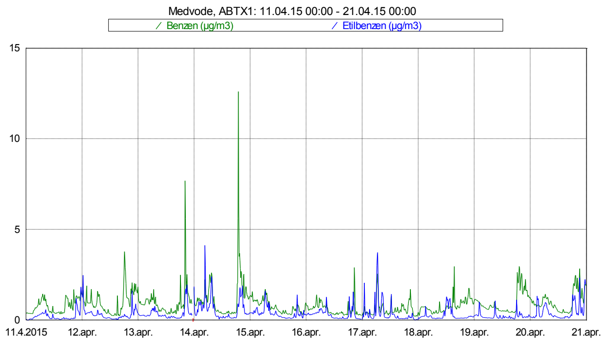
Slika 4: Imisijske koncentracije benzena in etilbenzena med 11. 4. 2015 in 20. 4. 2015.
