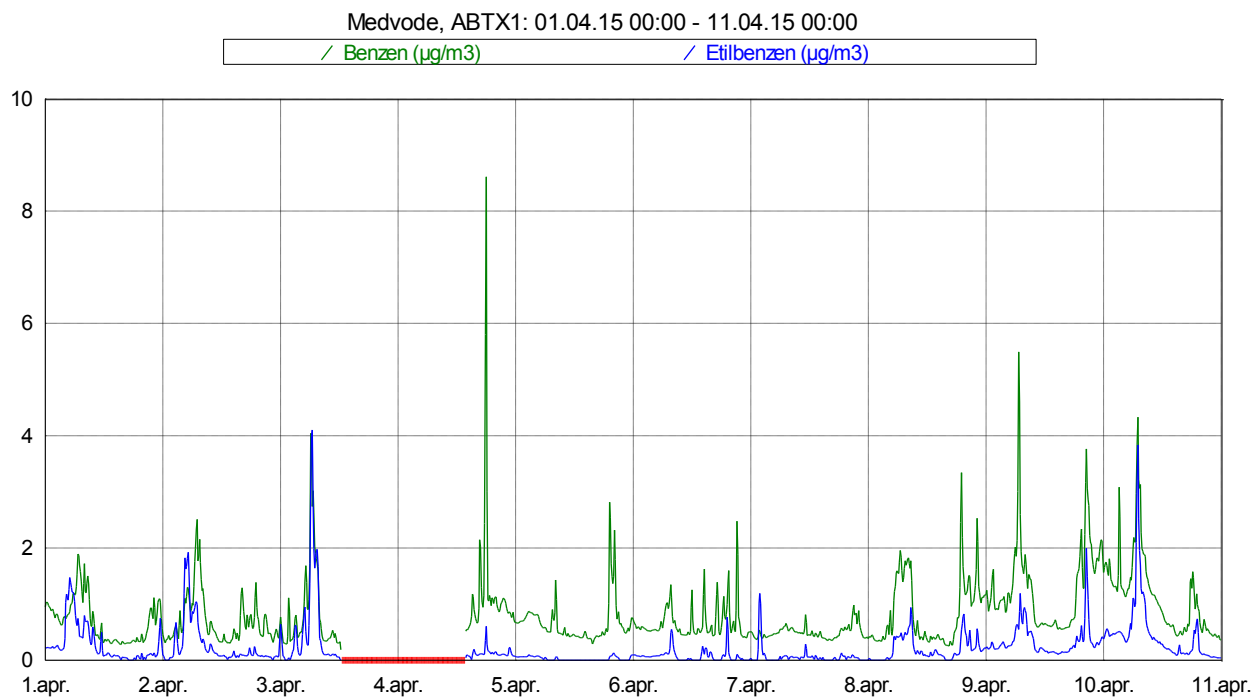
Slika 3: Imisijske koncentracije benzena in etilbenzena med vključno 1. 4. 2015 in 10. 4. 2015.
