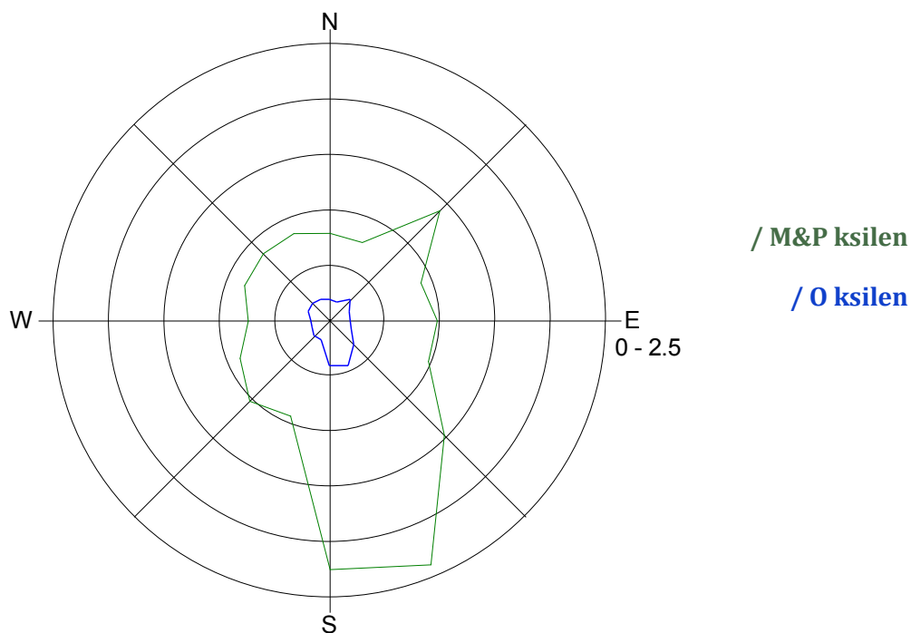
Slika 15: Roža onesnaženosti - M & P ksilen in O ksilen, april 2015.
