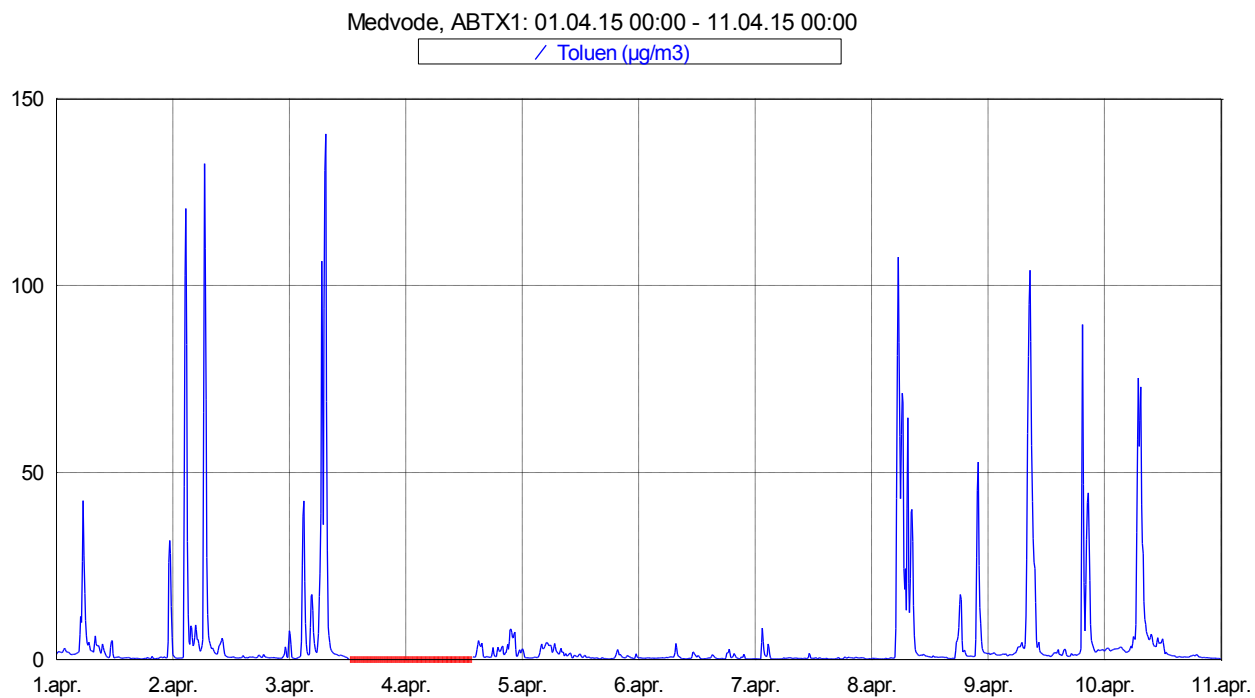
Slika 8: Imisijske koncentracije toluena med vključno 1. 4. 2015 in 10. 4. 2015.
