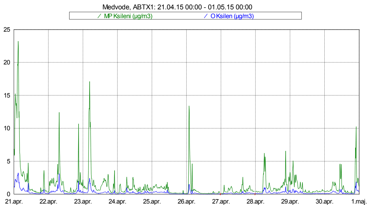
Slika 14: Imisijske koncentracije M&P in O ksilena med 21. 4. 2015 in 30. 4. 2015.
