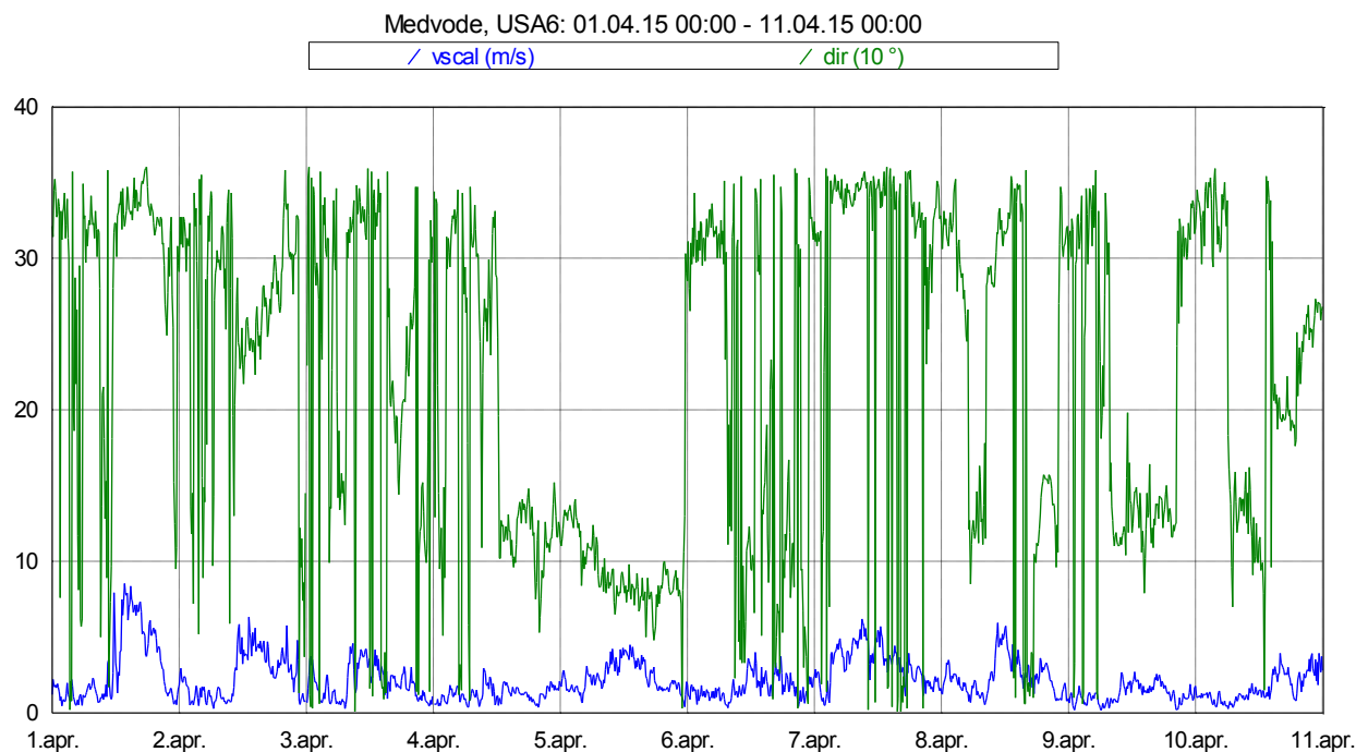
Slika 16: Smer in hitrost vetra med 1. 4. 2015 in 10. 4. 2015.
