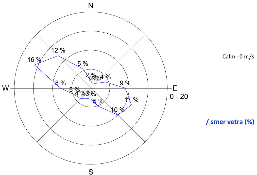
Slika 19: Roža vetrov, april 2014.
