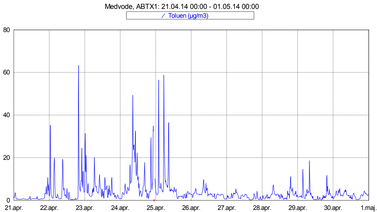
Slika 10: Imisijske koncentracije toluena med 21. 4. 2014 in 31. 4. 2014.
