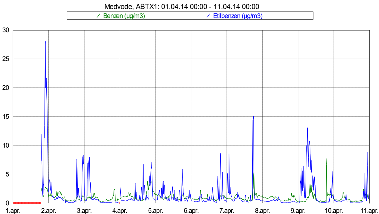
Slika 3: Imisijske koncentracije benzena in etilbenzena med vključno 1. 4. 2014 in 10. 4. 2014.
