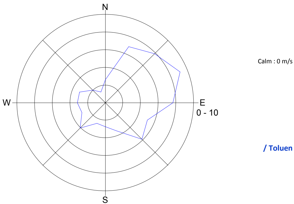
Slika 11: Roža onesnaženost - toluen, april 2014.
