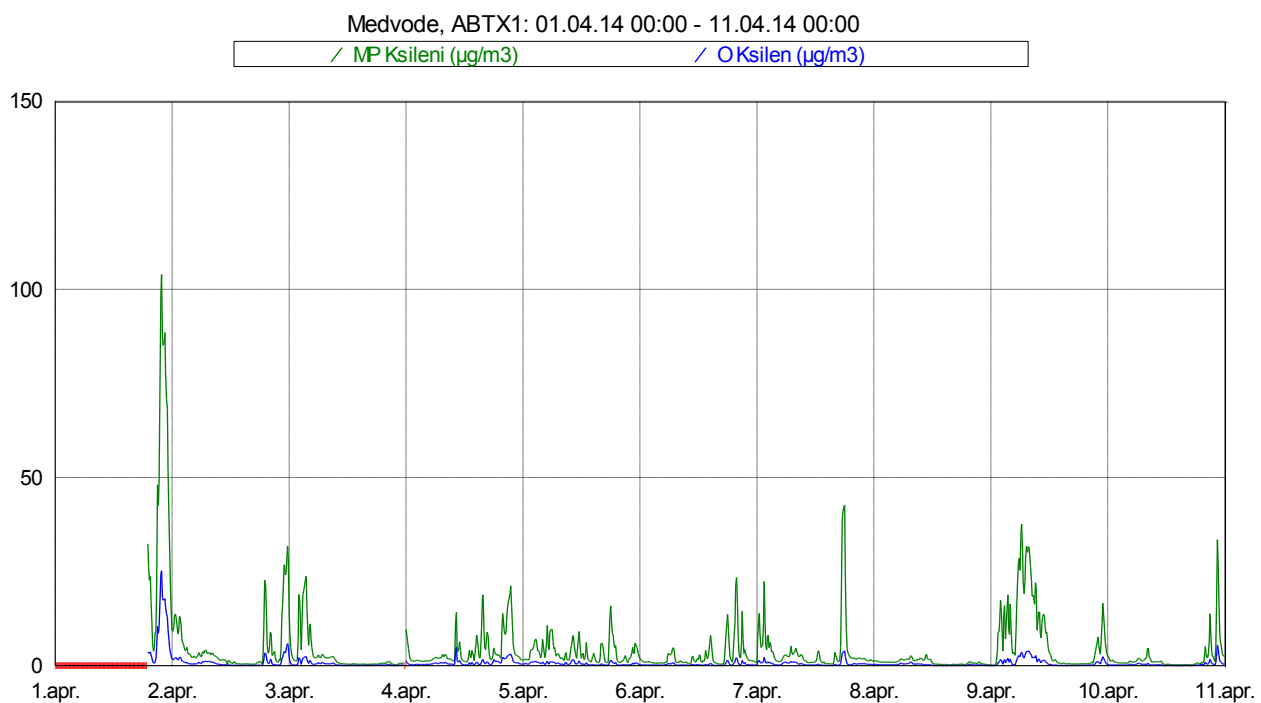
Slika 12: Imisijske koncentracije M&P in O ksilena med vključno 1. 4. 2014 in 10. 4. 2014.
