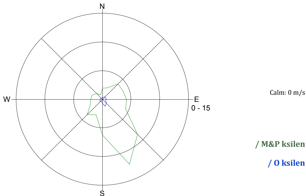
Slika 15: Roža onesnaženosti - M & P ksilen in O ksilen, april 2014.
