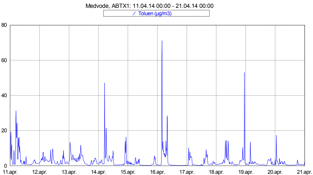
Slika 9: Imisijske koncentracije toluena med 11. 4. 2014 in 20. 4. 2014.
