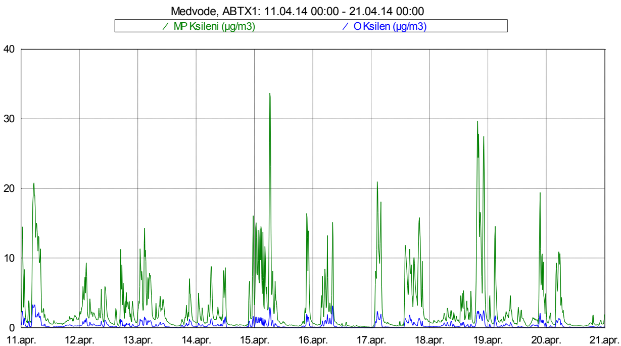
Slika 13: Imisijske koncentracije M&P in O ksilena med 11. 4. 2014 in 20. 4. 2014.
