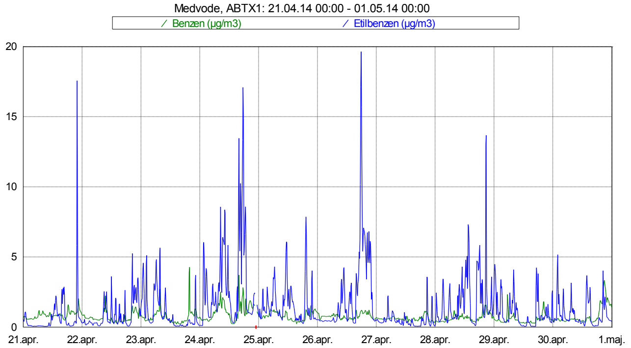
Slika 5: Imisijske koncentracije benzena in etilbenzena med 21. 4. 2014 in 31. 4. 2014.
