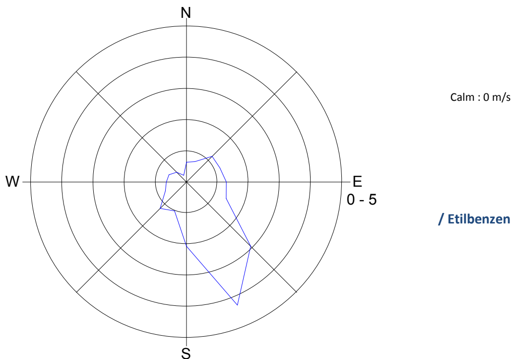
Slika 7: Roža onesnaženosti - etilbenzen april 2014.
