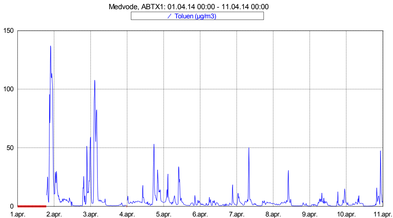
Slika 8: Imisijske koncentracije toluena med vključno 1. 4. 2014 in 10. 4. 2014.
