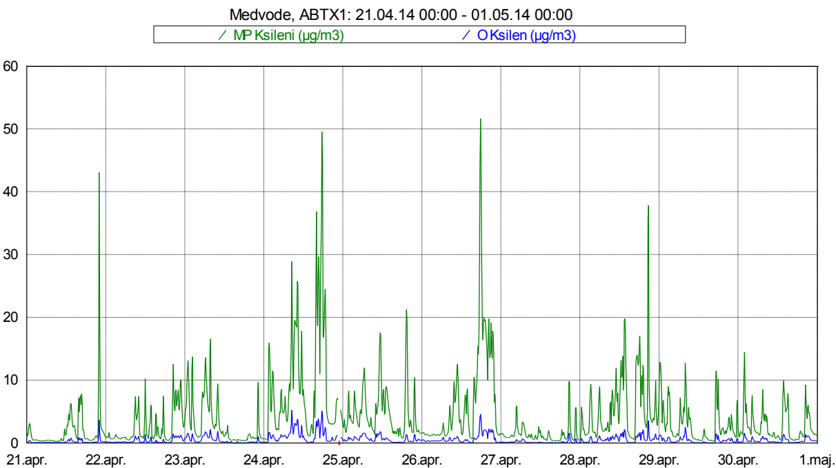
Slika 14: Imisijske koncentracije M&P in O ksilena med 21. 4. 2014 in 31. 4. 2014.
