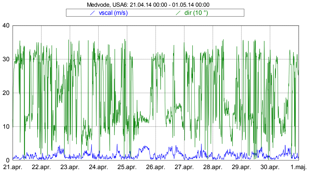
Slika 18: Smer in hitrost vetra med 21. 4. 2014 in 31. 4. 2014.
