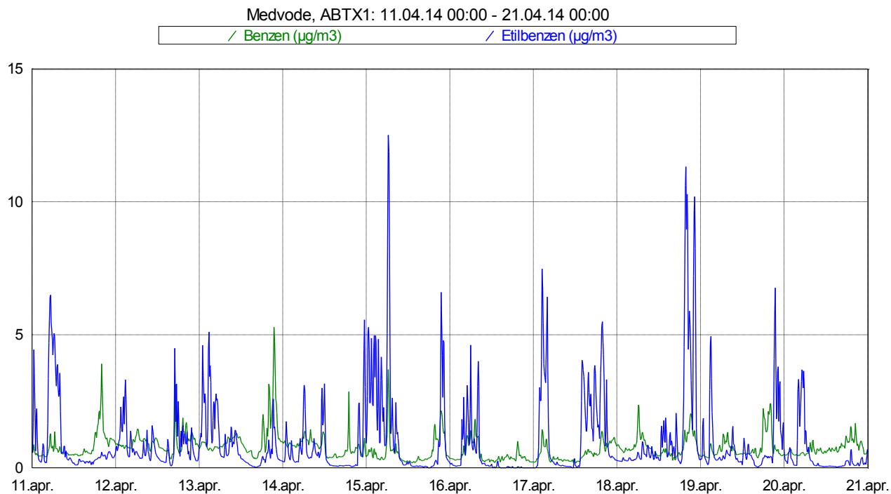
Slika 4: Imisijske koncentracije benzena in etilbenzena med 11. 4. 2014 in 20. 4. 2014.
