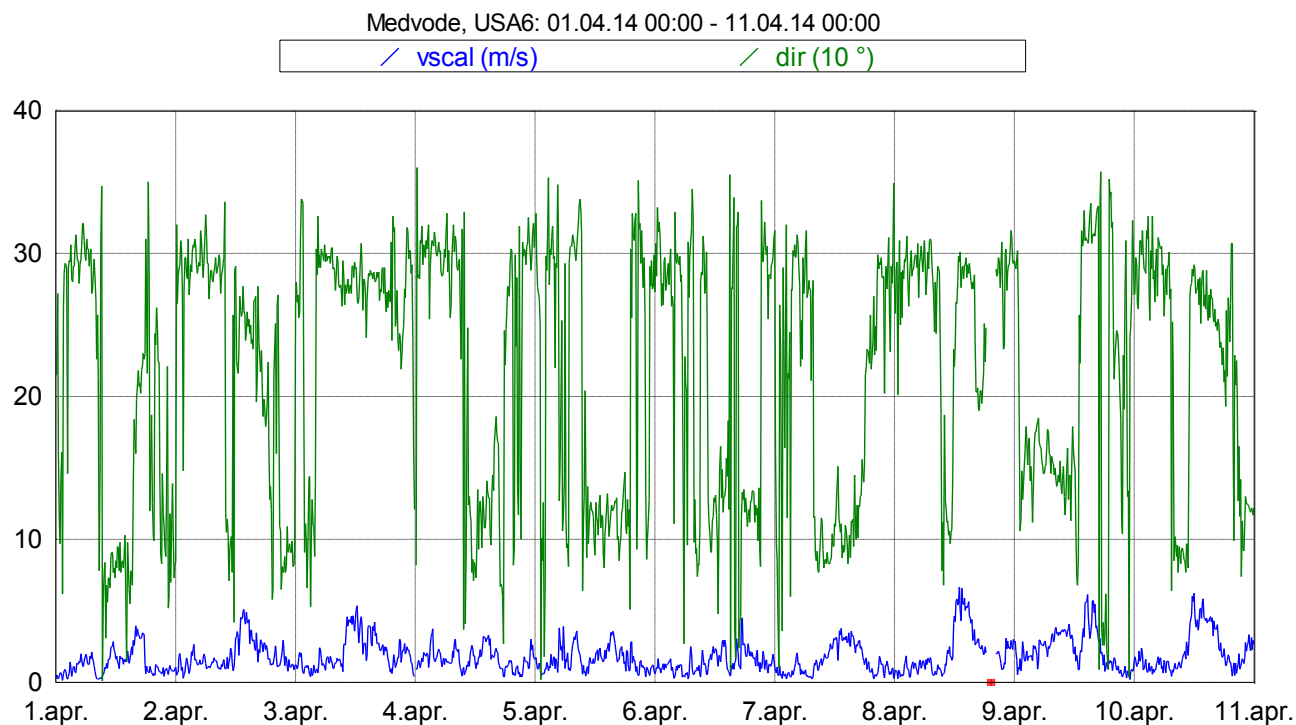
Slika 16: Smer in hitrost vetra med 1. 4. 2014 in 10. 4. 2014.
