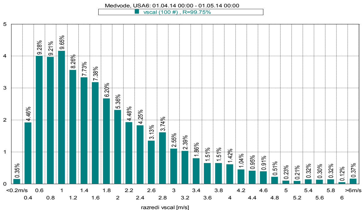
Slika 20: Frekvenčna porazdelitev po hitrosti vetra, april 2014.
