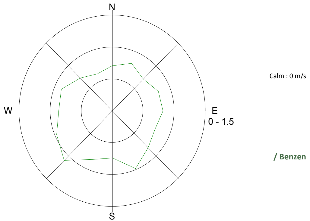
Slika 6: Roža onesnaženosti – benzen, april 2014.
