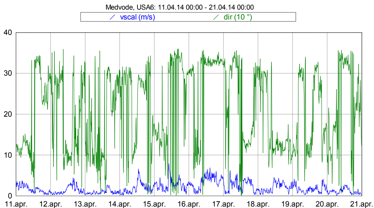
Slika 17: Smer in hitrost vetra med 11. 4. 2014 in 20. 4. 2014.
