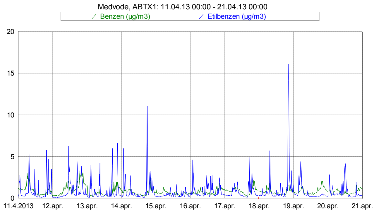
Slika 4: Imisijske koncentracije benzena in etilbenzena med 11. 4. 2013 in 20. 4. 2013.
