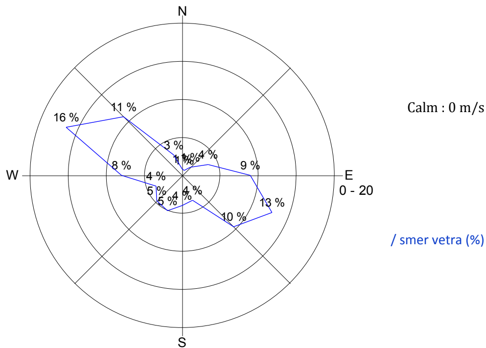
Slika 18: Roža vetrov, april 2013.
