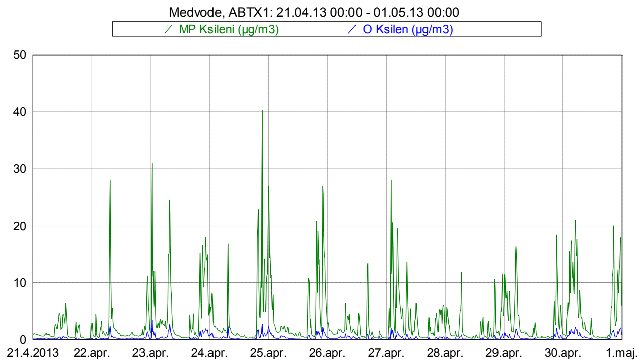
Slika 13: Imisijske koncentracije M&amp;P in O ksilena med 21. 4. 2013 in 30. 4. 2013.
