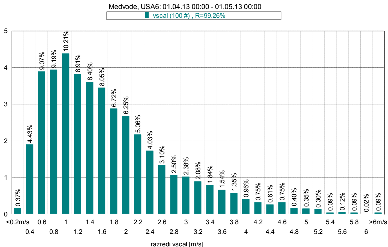
Slika 19: Frekvenčna porazdelitev po hitrosti vetra, april 2013.
