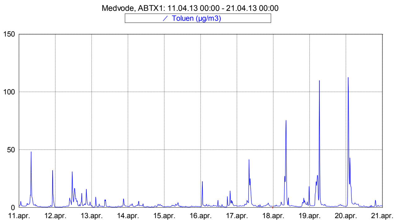
Slika 8: Imisijske koncentracije toluena med 11. 4. 2013 in 20. 4. 2013.
