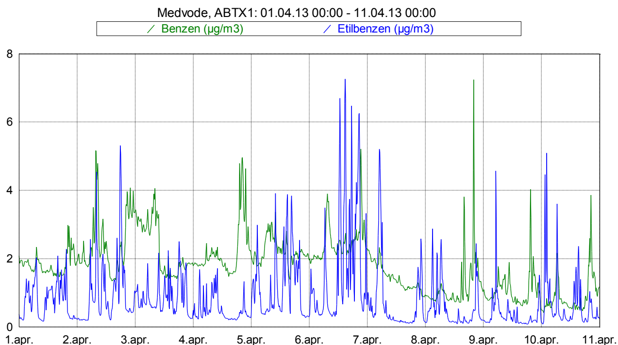
Slika 3: Imisijske koncentracije benzena in etilbenzena med vključno 1. 4. 2013 in 10. 4. 2013.
