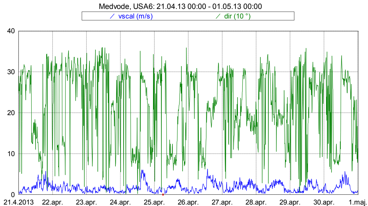
Slika 17: Smer in hitrost vetra med 21. 4. 2013 in 30. 4. 2013.
