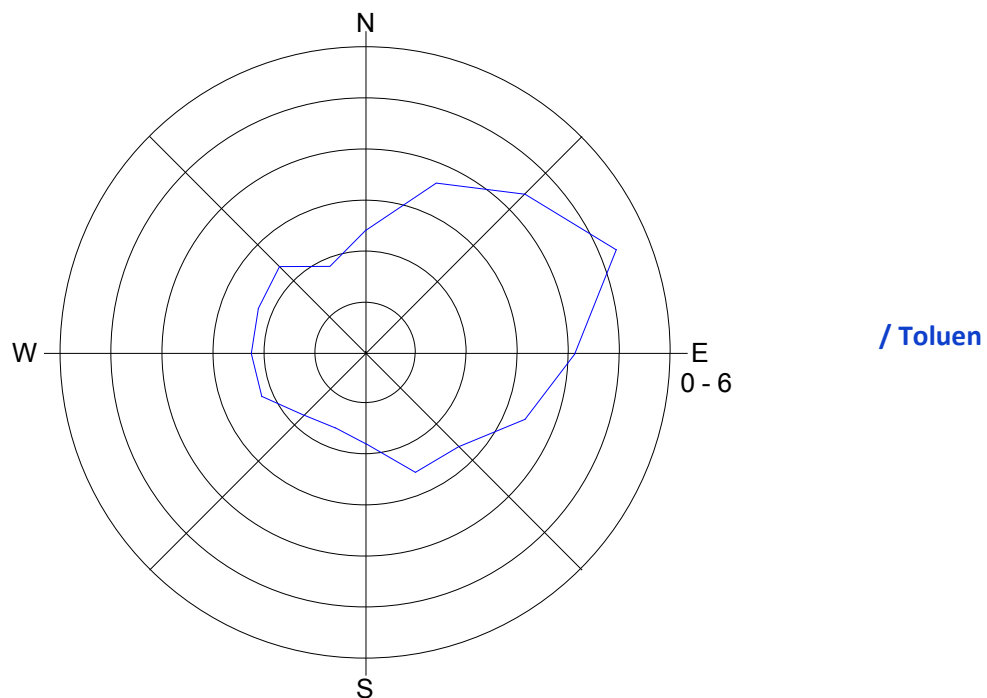
Slika 9: Imisijske koncentracije toluenta med 21. 4. 2013 in 30. 4. 2013.
