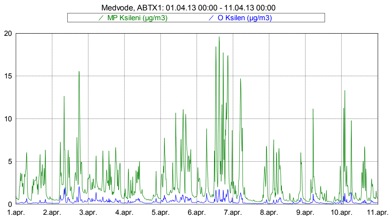
Slika 11: Imisijske koncentracije M&P in O ksilena med vključno 1. 4. 2013 in 10. 4. 2013.
