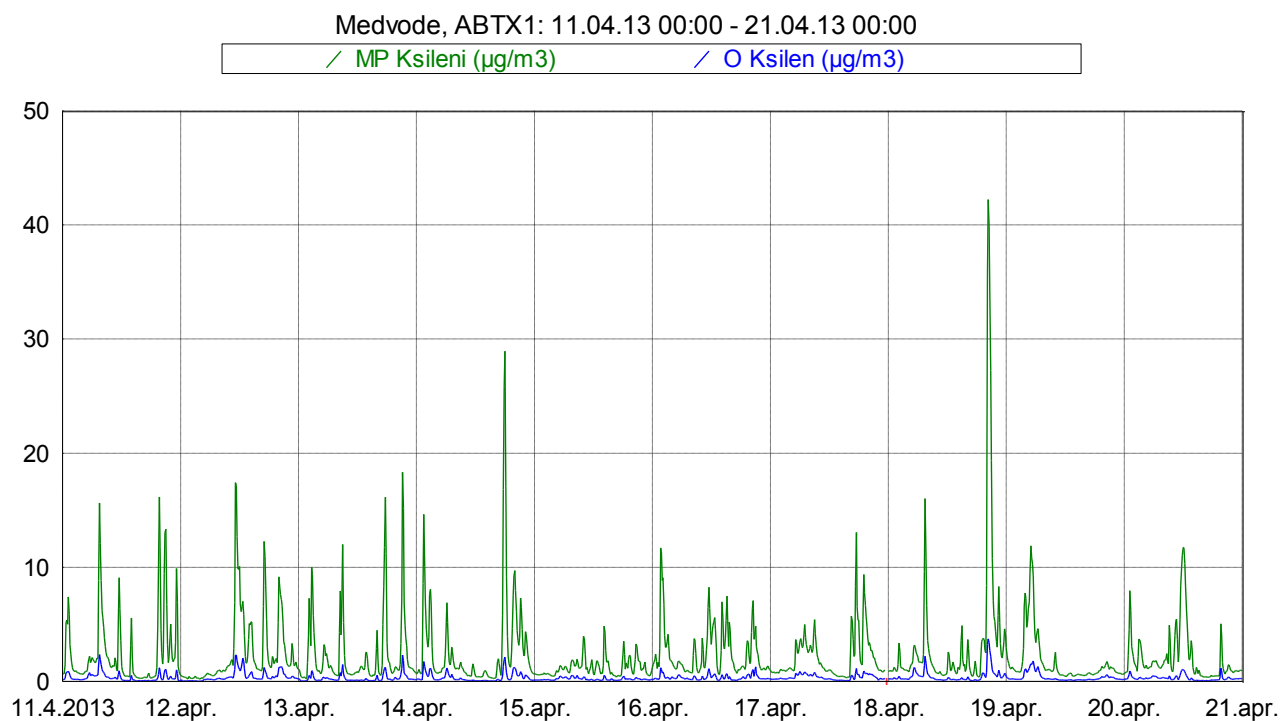
Slika 12: Imisijske koncentracije M&amp;P in O ksilena med 11. 4. 2013 in 20. 4. 2013.
