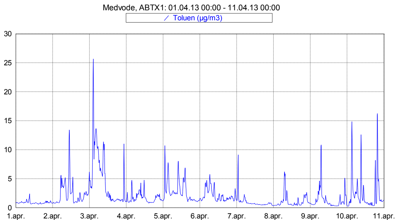
Slika 7: Imisijske koncentracije toluena med vključno 1. 4. 2013 in 10. 4. 2013.
