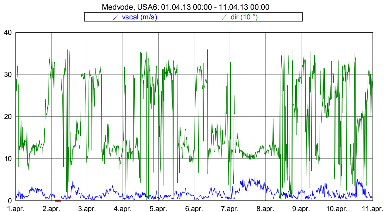
Slika 15: Smer in hitrost vetra med 1. 4. 2013 in 10. 4. 2013.
