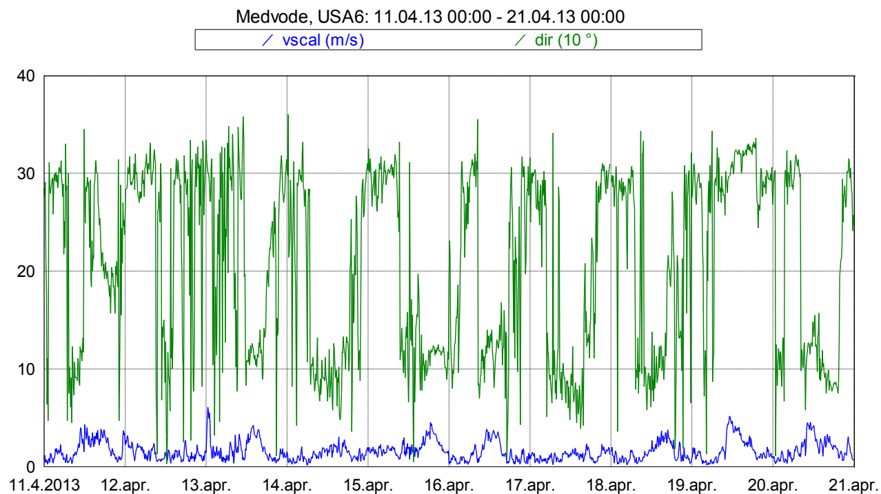
Slika 16: Smer in hitrost vetra med 11. 4. 2013 in 20. 4. 2013.
