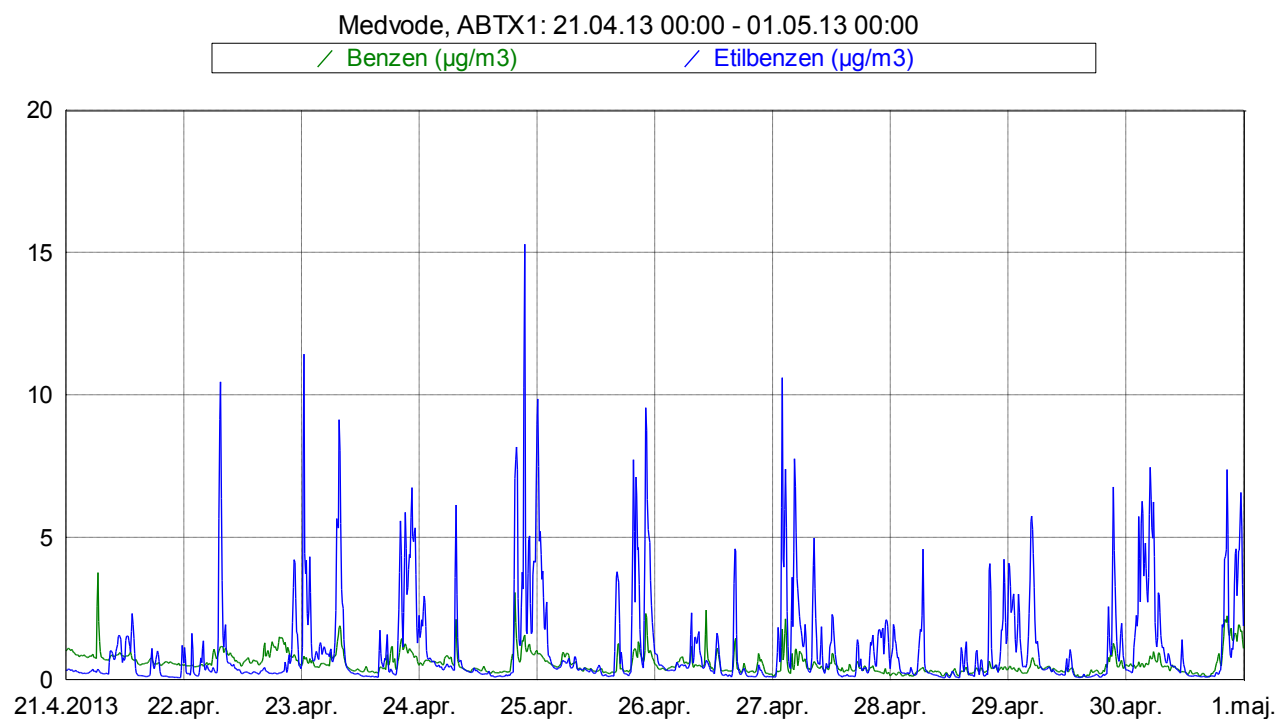
Slika 5: Imisijske koncentracije benzena in etilbenzena med 21. 4. 2013 in 30. 4. 2013.
