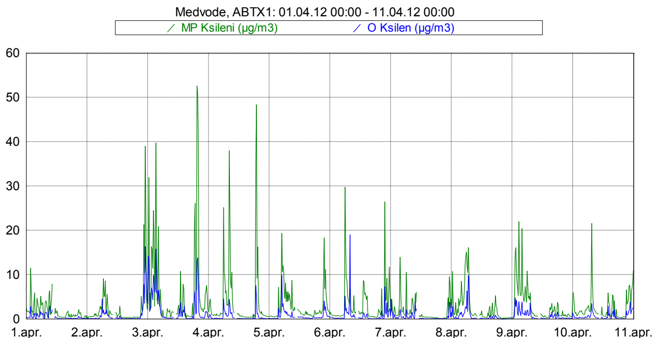
Slika 11: Imisijske koncentracije M&P in O ksilena med 1. 4. 2012 in 10. 4. 2012.
