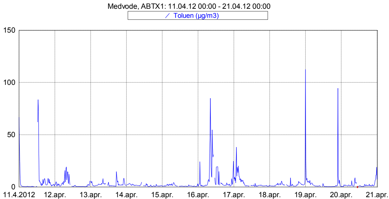
Slika 8: Imisijske koncentracije toluena med 11. 4. 2012 in 21. 4. 2012.
