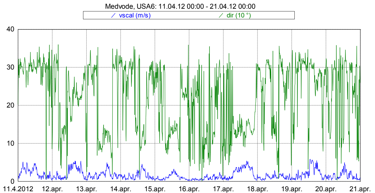
Slika 16: Smer in hitrost vetra med 11. 4. 2012 in 21. 4. 2012.
