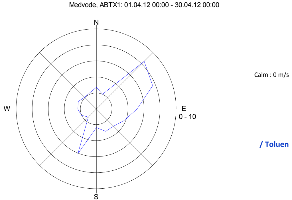
Slika 10: Roža onesnaženost - toluen, april 2012.
