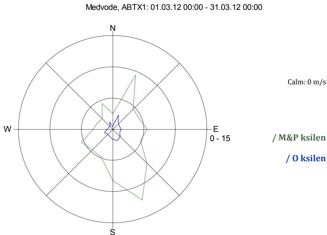
Slika 14: Roža onesnaženosti - M & P ksilen in O ksilen, april 2012.
