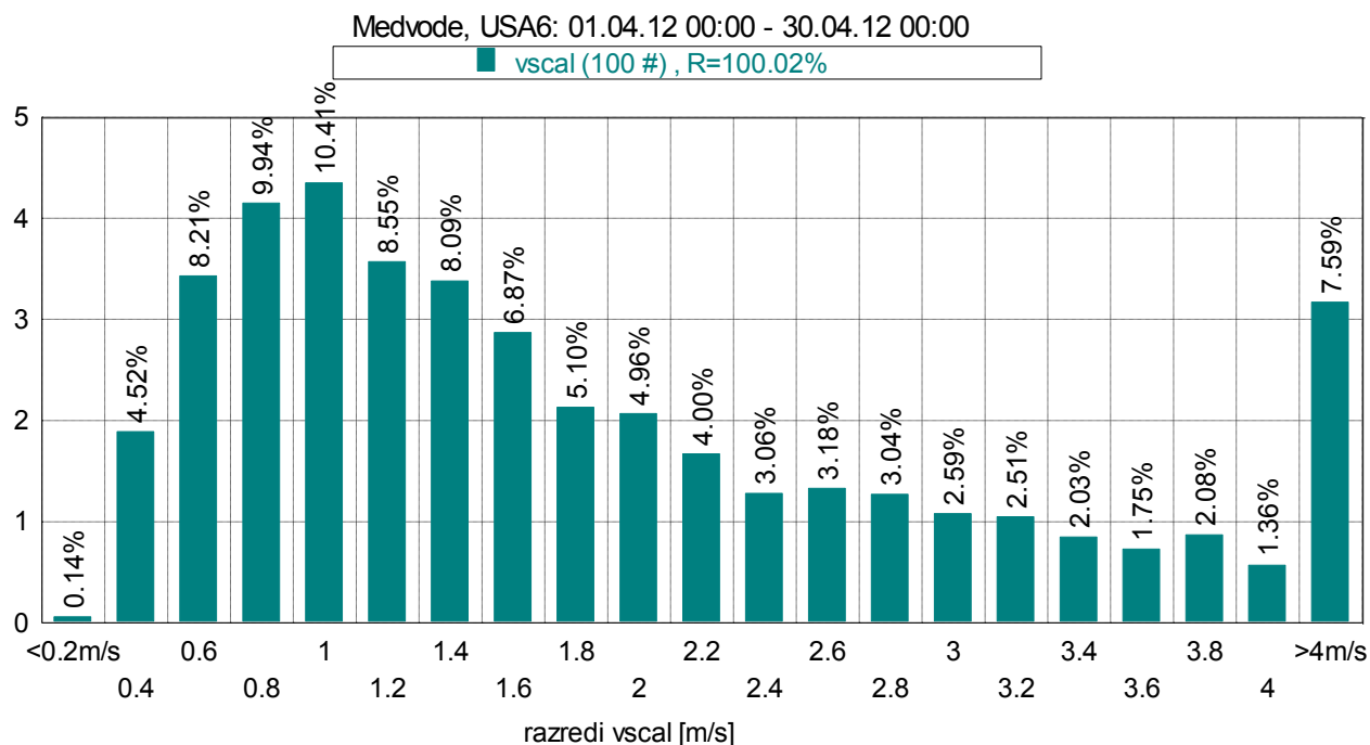
Slika 19: Frekvenčna porazdelitev po hitrosti vetra, april 2012.
