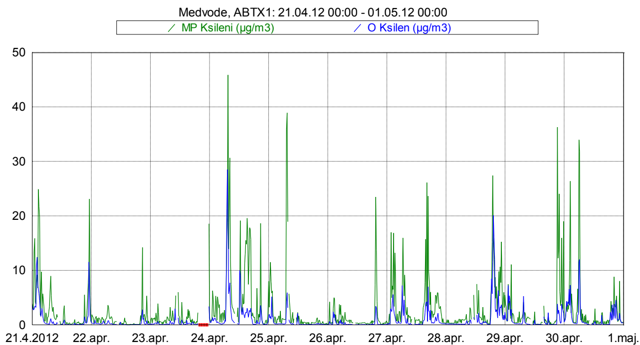
Slika 13: Imisijske koncentracije M&P in O ksilena med 21. 4. 2012 in 30. 4. 2012.
