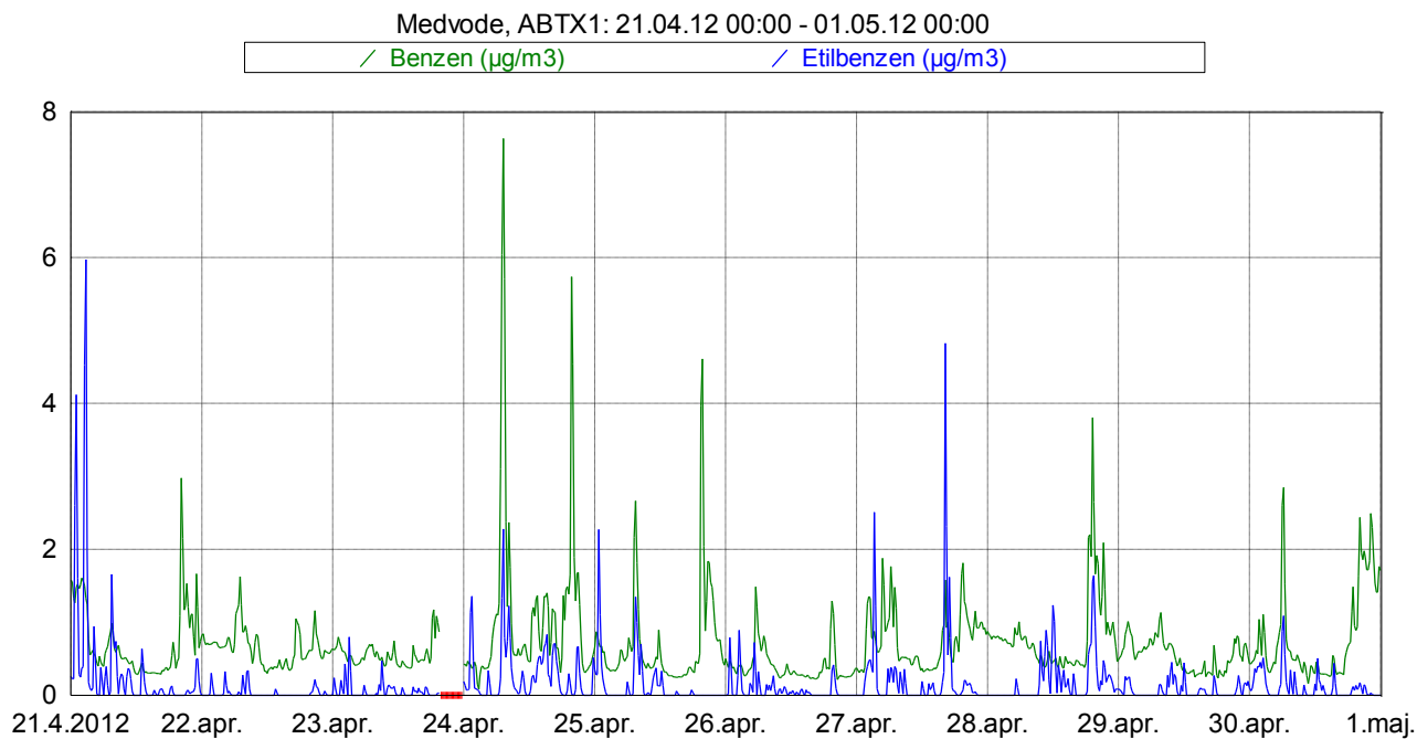
Slika 5: Imisijske koncentracije benzena in etilbenzena med 21. 4. 2012 in 30. 4. 2012.
