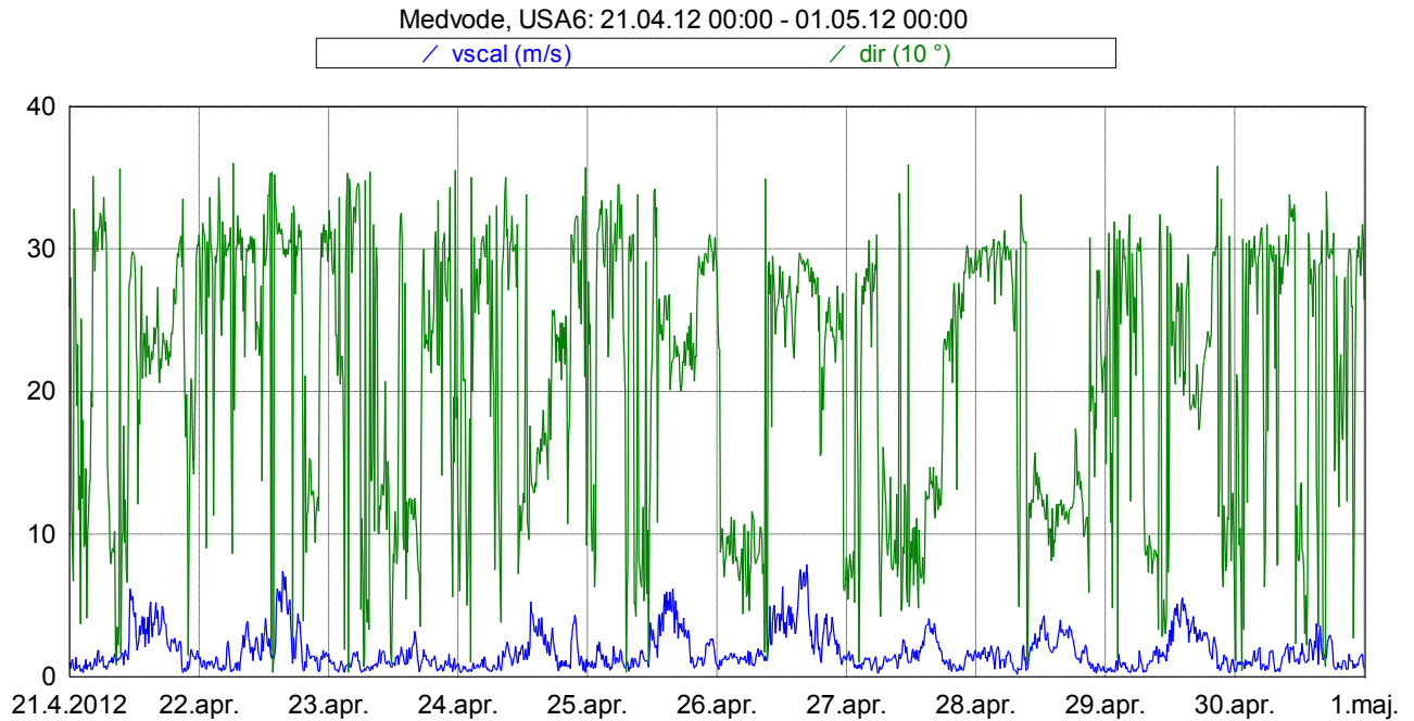
Slika 17: Smer in hitrost vetra med 21. 4. 2012 in 30. 4. 2012.
