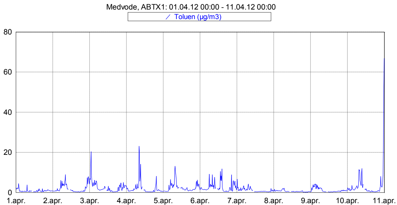
Slika 7: Imisijske koncentracije toluena med 1. 4. 2012 in 10. 4. 2012.
