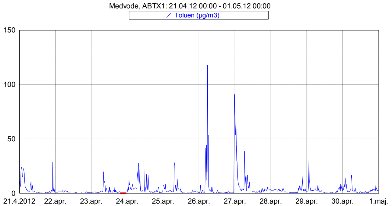
Slika 9: Imisijske koncentracije toluena med 21. 4. 2012 in 30. 4. 2012.
