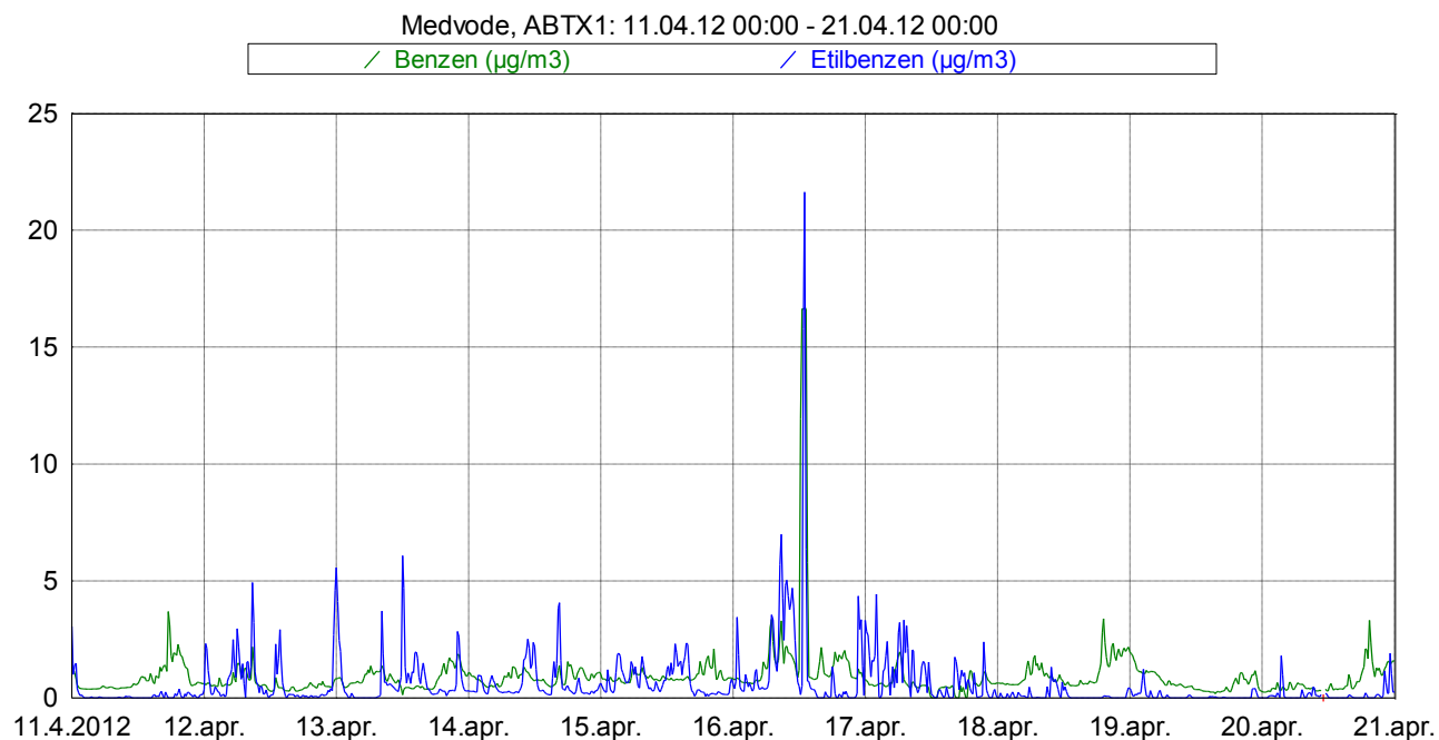
Slika 4: Imisijske koncentracije benzena in etilbenzena med 11. 4. 2012 in 21. 4. 2012.
