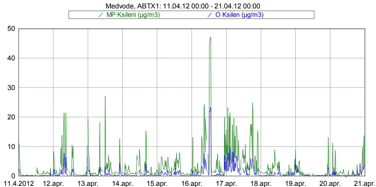
Slika 12: Imisijske koncentracije M&P in O ksilena med 11. 4. 2012 in 21. 4. 2012.
