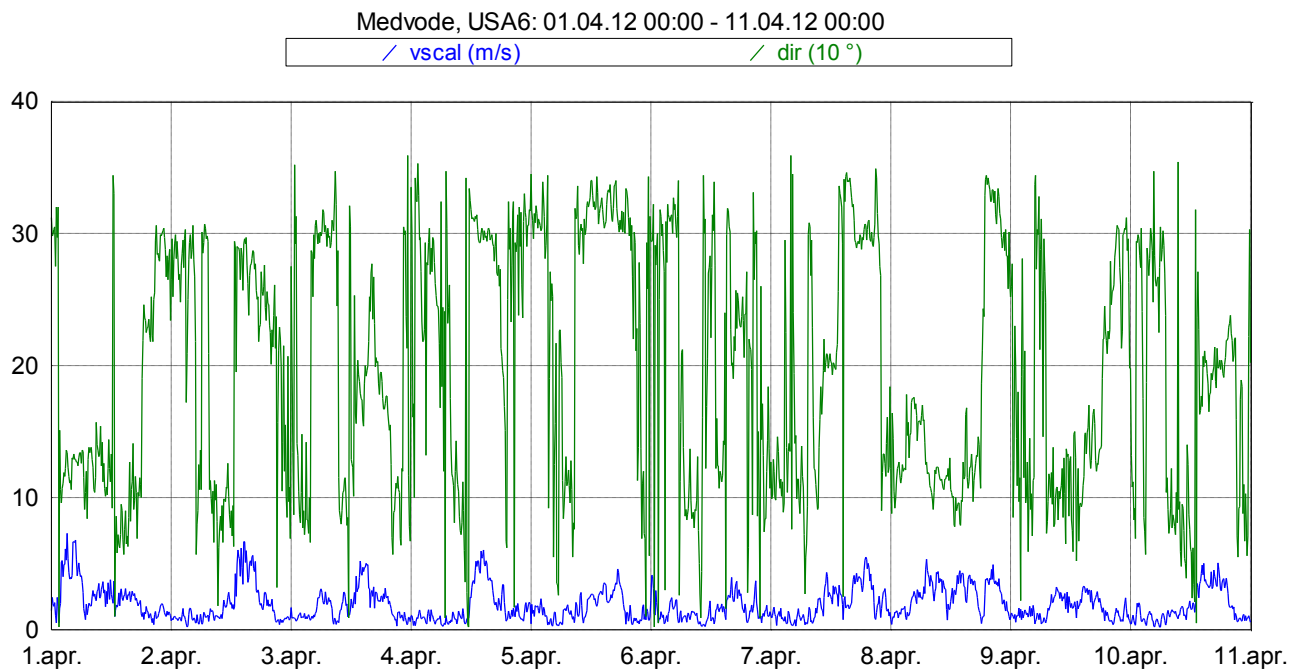
Slika 15: Smer in hitrost vetra med 1. 4. 2012 in 10. 4. 2012.
